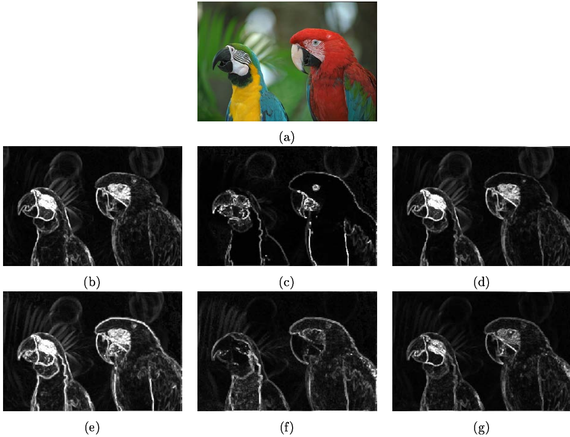
FIG. 4.2 – Gradients couleur de l'image “perroquets” : (a) image couleur initiale, f , (b) \nabla^L f , (c) \nabla^H f , (d) \nabla^S f , (e) \nabla^{\text{sup}} f , (f) \nabla^C f et (g) \nabla^P f .
