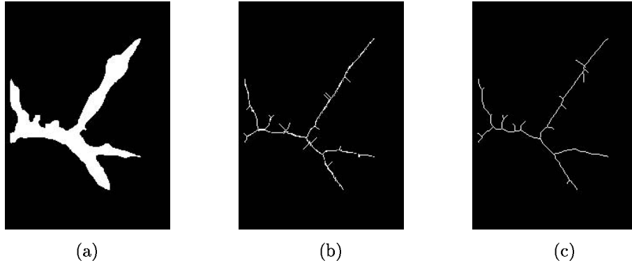
FIG. A.5 – Squelettes morphologiques : (a) Ensemble initial, (b) Squelette de Lantuéjoul, (c) Squelette par amincissement en 8-connexité. Remarquer que le squelette (b) n'est pas homotopique. Toutefois, aucun des deux n'est robuste (apparition de nombreuses ramifications non significatives).
