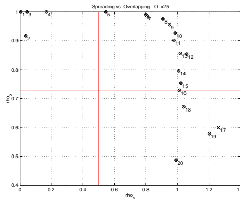
FIG. 7.9 – Diagramme de dispersion des paramètres \rho_s et \rho_o pour Frottis 0 . La zone de lecture correspond au quadrant supérieur droit.
