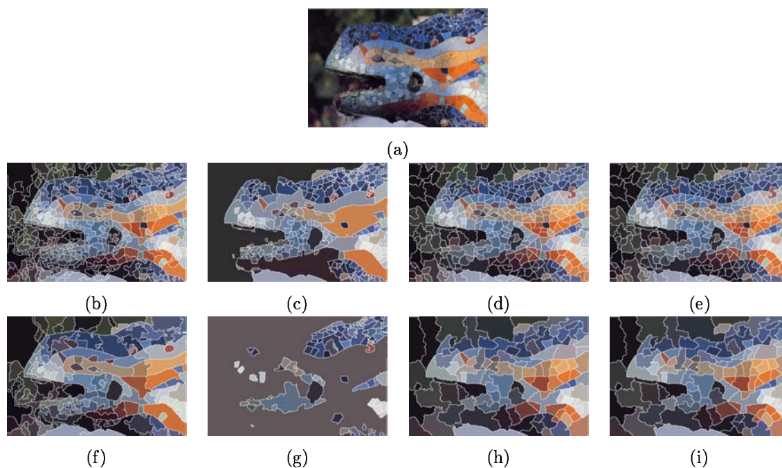
FIG. 5.9 – Comparaison de pyramides couleur de LPE non-paramétriques et paramétriques à l'aide des valeurs d'extinction sur l'image "lézard" : (a) image initiale, (b)-(f) LPE des niveaux 3 et 4 de l'algorithme de cascades (379 et 120 régions respectivement) , (c)-(g) LPE en prenant comme marqueurs les 379 et 129 minima plus contrastés, (d)-(h) LPE en prenant comme marqueurs les 379 et 129 minima avec une valeur d'extinction surfacique plus grande, (e)-(i) LPE en prenant comme marqueurs les 379 et 129 minima avec une valeur d'extinction volumique plus grande. Le gradient utilisé est \nabla^S f .
