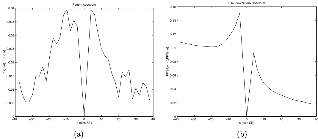
FIG. 6.3 – Exemples de courbes granulométriques pour l'exemple des figures 6.1 et 6.2 : (a) spectre de forme (densité de tailles par fermetures et ouvertures), PS(n) , (b) pseudo-spectre de forme (par dilatations et érosions), PPS(n) .
