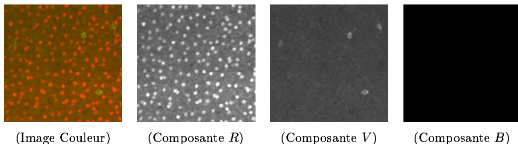
FIG. 3.22 – Image couleur de la rétine d'un singe avec deux populations de cellules qui ont été immuno-marquées avec deux fluorescences différentes.
