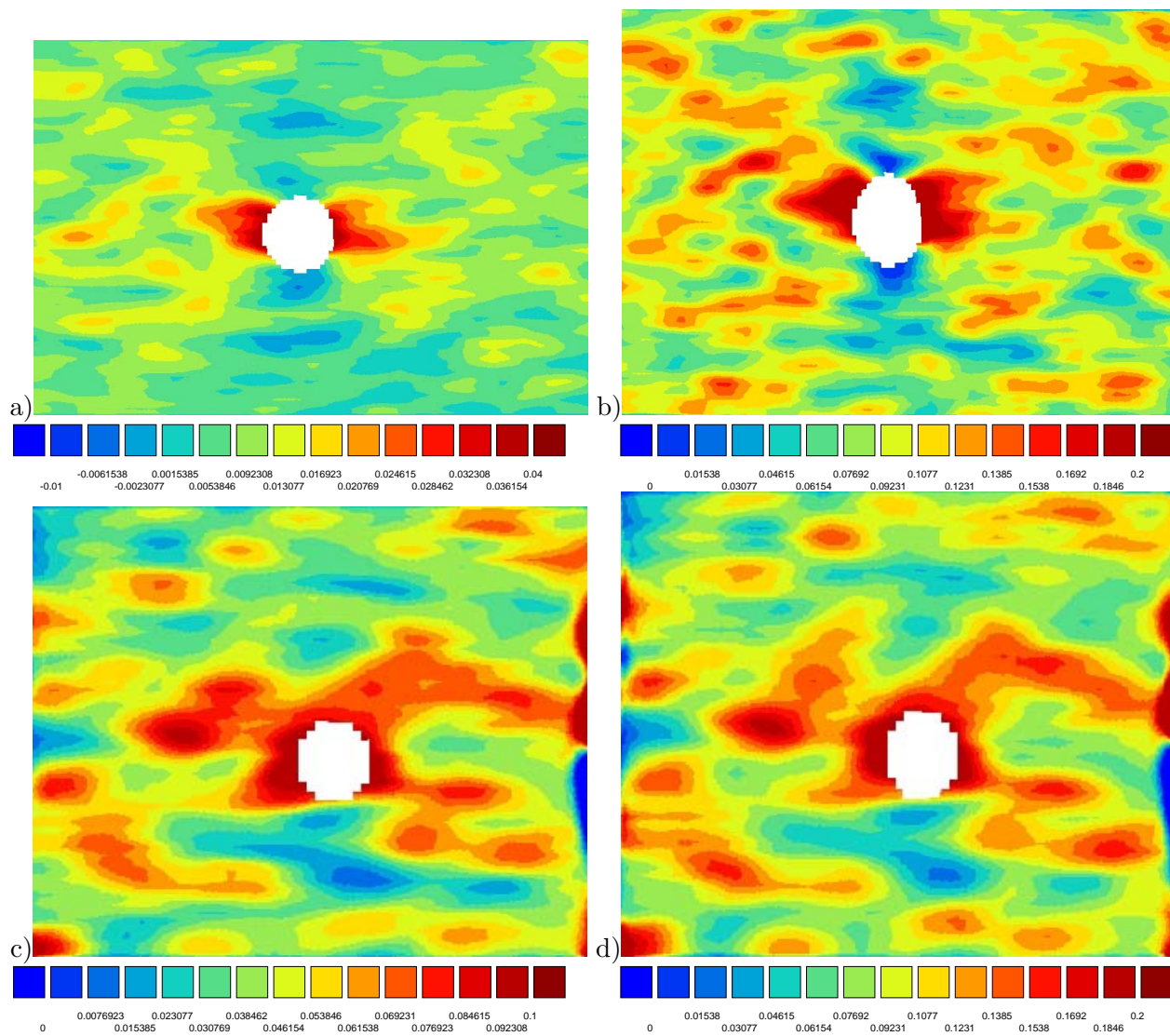
Figure V.10 : Champs des déformations axiales : a) et b) trou de 2 mm de rayon (éprouvette de 40 mm de largeur), c) et d) trou de 1 mm de rayon (éprouvette 20 mm de largeur).
