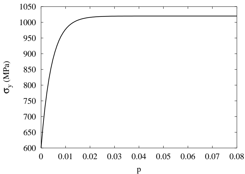
Figure IV.21 : Comportement de la couche d'oxyde de nickel.
