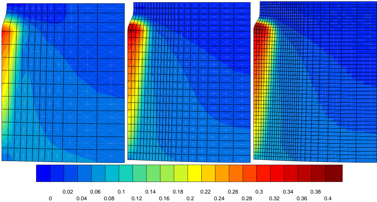
Figure VI.15 : Propagation de la fissure pour trois maillages différents avec le modèle microfoam .
