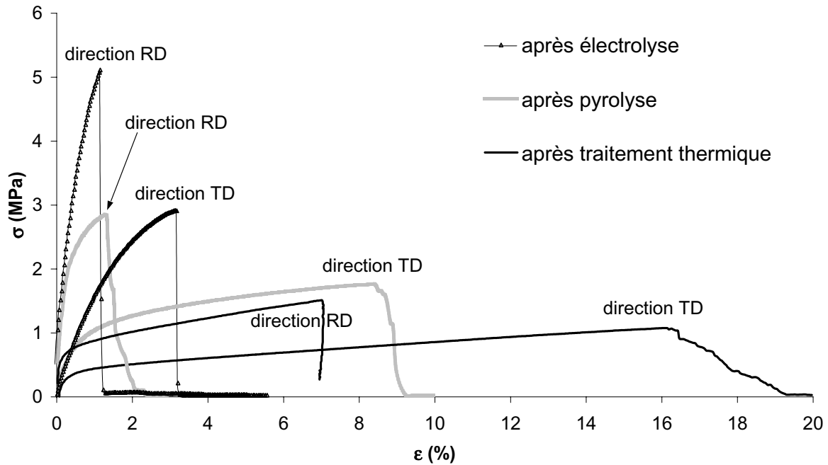
Figure .13 : Comportement mécanique des mousses de nickel après chaque étape du procédé.
