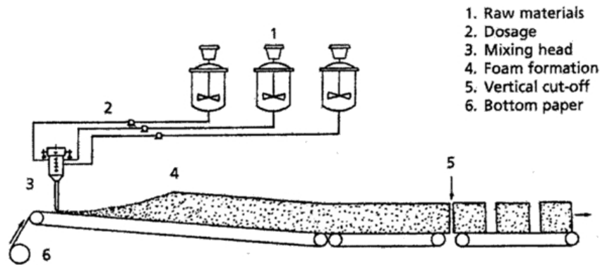
Figure .4 : Procédé de fabrication d'une mousse de polyuréthane.
