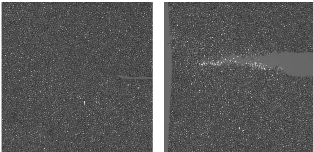
Figure VI.11 : Fissure horizontale centrale, symétrique, dans une plaque de mousse normale à la direction RD : demi-plaque initiale à gauche, et propagation de la fissure à droite.
