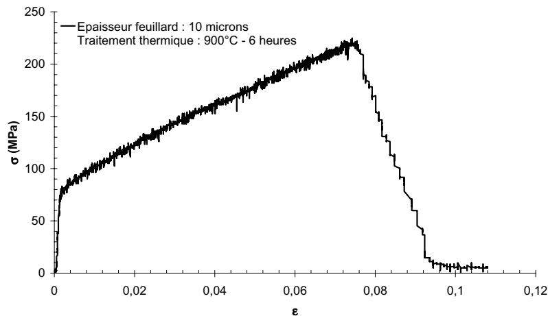
Figure III.11 : Comportement mécanique d'un feillard de nickel (Goussery, 2004).
