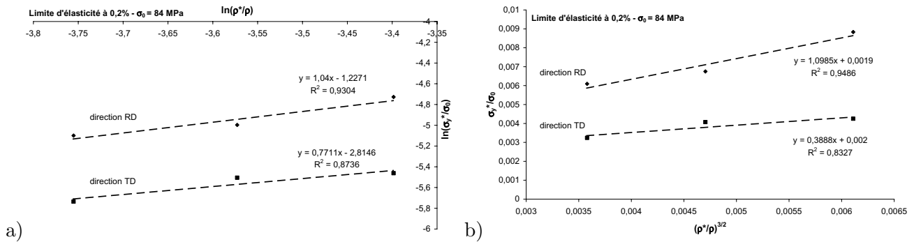
Figure III.8 : Relation entre la limite d'élasticité à 0,2 % et la densité relative de la mousse : a) détermination de la puissance, b) à puissance fixée ( n = 3/2 ).
