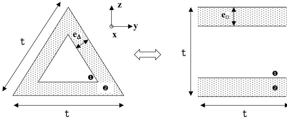
Figure IV.11 : Équivalence entre section triangulaire et carrée des brins.
