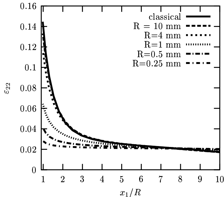
Figure VI.7 : Profil de déformations axiales le long du ligament dans une plaque micromorphe élastoplastique trouée sollicitée en traction à l'infini, en conditions de contraintes planes : influence de la taille du trou. La longueur caractéristique vaut l_c = 0,06 mm.
