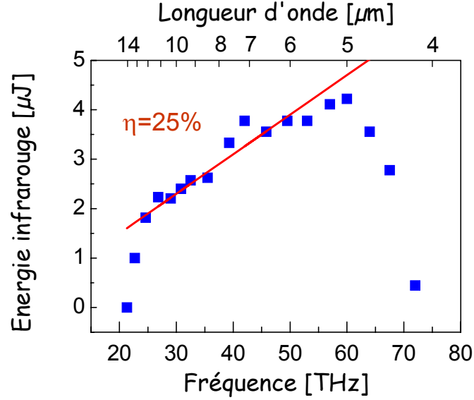
FIG. 2.9 : Energie des impulsions infrarouges engendrées dans un cristal non-linéaire de GaSe (d'épaisseur 0.5 \text{ mm} ) en fonction de leur fréquence centrale. L'accord de phase réalisé est de type II. La ligne continue correspond à un rendement quantique \eta constant égal à 25 %. (N.B. : Ce rendement quantique est égal au rapport entre le nombre de photons infrarouges engendrés et le nombre de photons signal incidents sur le cristal ; il s'agit d'un rendement externe au cristal, qui inclut les pertes par réflexions sur les faces d'entrée et de sortie).
