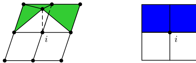
FIG. 3.4.a : \sigma_{11}^h
