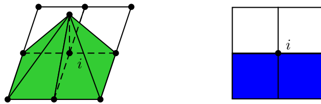
FIG. 3.4.b : \sigma_{11}^b
