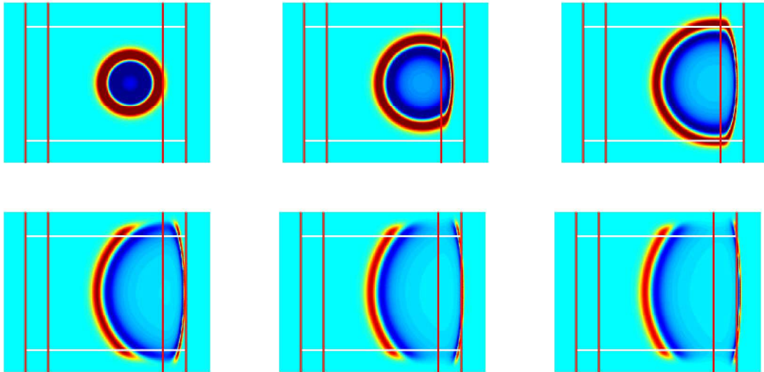
FIG. 11.10: Propagation d'une onde advective dans le cas M = 0.9 avec ajout d'une couche intermédiaire, t = 1.25, 2, 2.75, 3.75, 4.5 et 5 .
