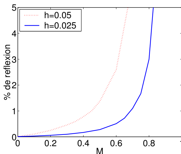
FIG. 11.8: Évolution de l'erreur en fonction de M
