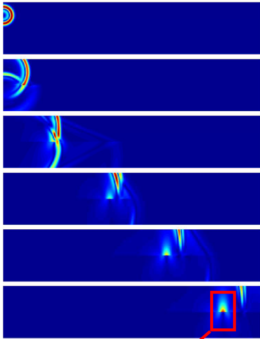
Onde de Stoneley
