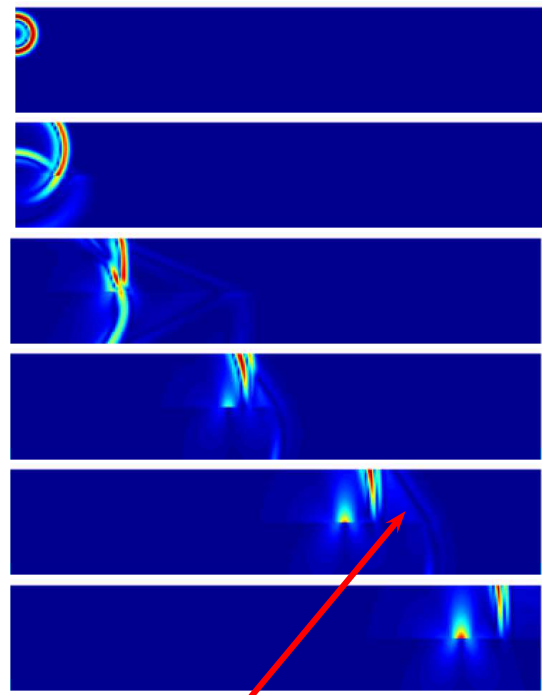
Onde de tête S
