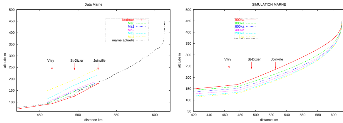
FIG. 5.45 – Comparaison entre les terrasses d'âge inférieur ou égal à 1 million d'années (à gauche) et le modèle (à droite) dans l'hypothèse d'une surrection de 90 m/Ma. La capture de la Saulx et de l'Ornain n'est pas prise en compte.
