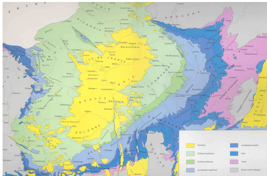
FIG. 5.2 – Carte géologique du Bassin parisien, d'après la Synthèse géologique du Bassin de Paris (Mégien et al., 1980) [132].
