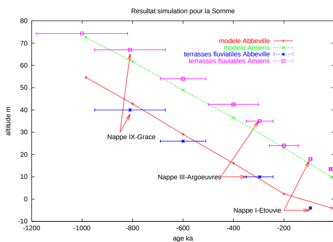
FIG. 5.29 – Hypothèse 2 : Simulation des terrasses fluviales de la Somme sur 1 million d'années en considérant un taux de surrection de 60 m par million d'années à partir d'un profil initial est proche de l'actuel. Détail. Les terrasses simulées ne sont pas incompatibles avec les terrasses réelles.
