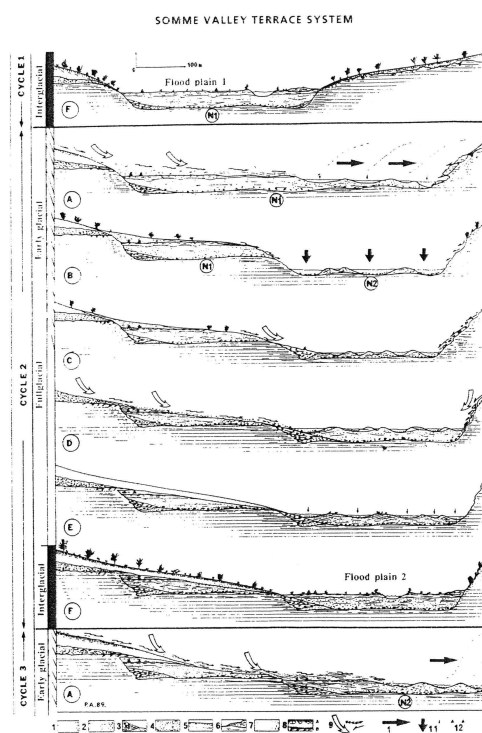
FIG. 2.9 – Schéma de synthèse sur les phases d'érosion et de sédimentation au cours du dernier cycle climatique.
