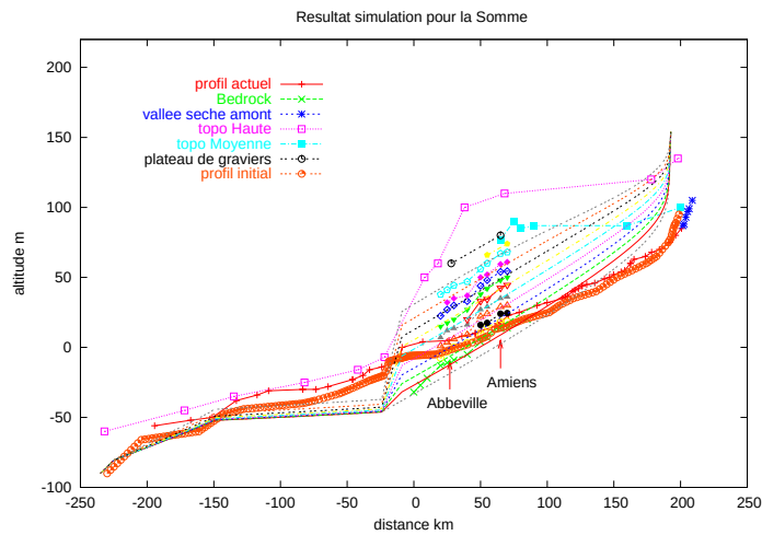
FIG. 5.27 – Hypothèse 2 sur le profil initial : celui-ci est proche du profil actuel (trait épais). Sont également représentés sur le graphique : les terrasses fluviales, le profil actuel et le relief non -incisé entourant la vallée de la Somme.
