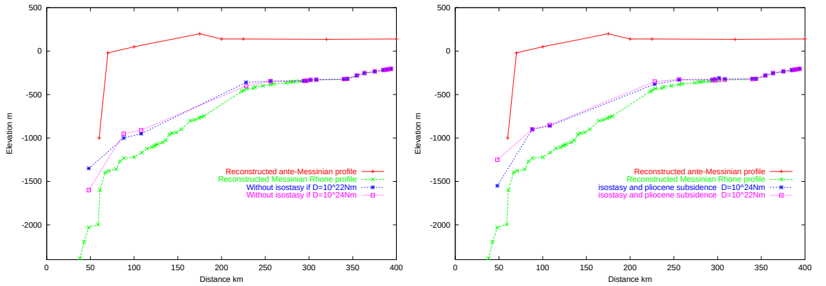
FIG. 6.20 – (A) Profils reconstruits pour des rigidités flexurales comprises entre D = 10^{22} \text{ Nm} et D = 10^{24} \text{ Nm} . Le profil précédent ne tenait pas compte de l’effet de l’isostasie durant la crise messinienne. Pas de tectonique à l’aval (on ne tient pas compte du remplissage plio-quatenaire). (B) Profils finalement reconstruits pour des rigidités flexurales comprises entre D = 10^{22} \text{ Nm} et D = 10^{24} \text{ Nm} tenant compte également du remplissage plio-quatenaire.
