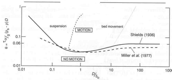
FIG. 3.8 – Diagramme de Shield représentant les contraintes adimensionnelles critiques pour du matériel non-cohésif (d'après [103]). Au dessus de la courbe, les contraintes sont suffisantes pour mettre en mouvement les particules.
