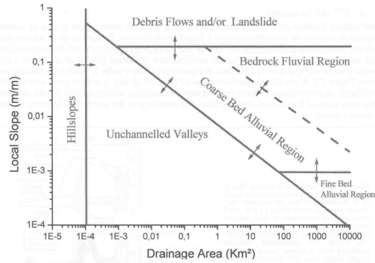
FIG. 3.5 – Relation entre la pente et l'aire de drainage (cit  dans [110]). La mesure des param tres g om triques de base permet de caract riser les diff rentes organisations g omorphologiques (les versants, le domaine non-chenalis , les parties alluviales des rivi res, les parties o  la rivi re est directement en contact avec le substrat rocheux).
