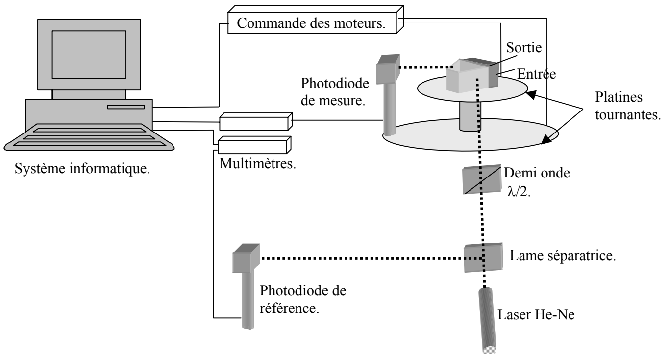
Figure 16 : Schéma du Montage mon-capteur en interrogation angulaire. Les platines tournantes, commandées par l'intermédiaire d'un programme LabView, nous permettent de varier l'angle d'incidence.
