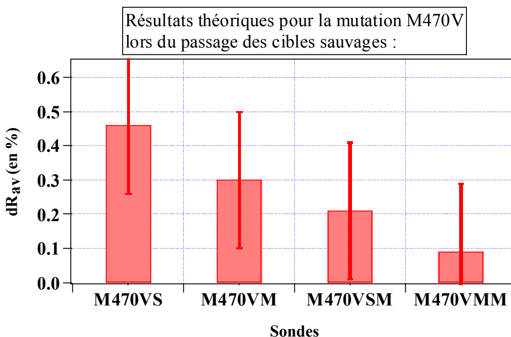
Figure 93 : Allure de la réponse théorique du multicapteur en dR av . Les résultats expérimentaux attendus varient dans une marge de ±0.2% correspondant à notre barre d'erreur. Le recouvrement de réponse des sondes M470VS et M470VM illustre le problème que nous avons cherché à résoudre en appliquant notre nouvelle stratégie de choix des sondes. Les cibles sauvages correspondent aux cibles 3* 13 bases utilisées dans les expériences précédentes.
