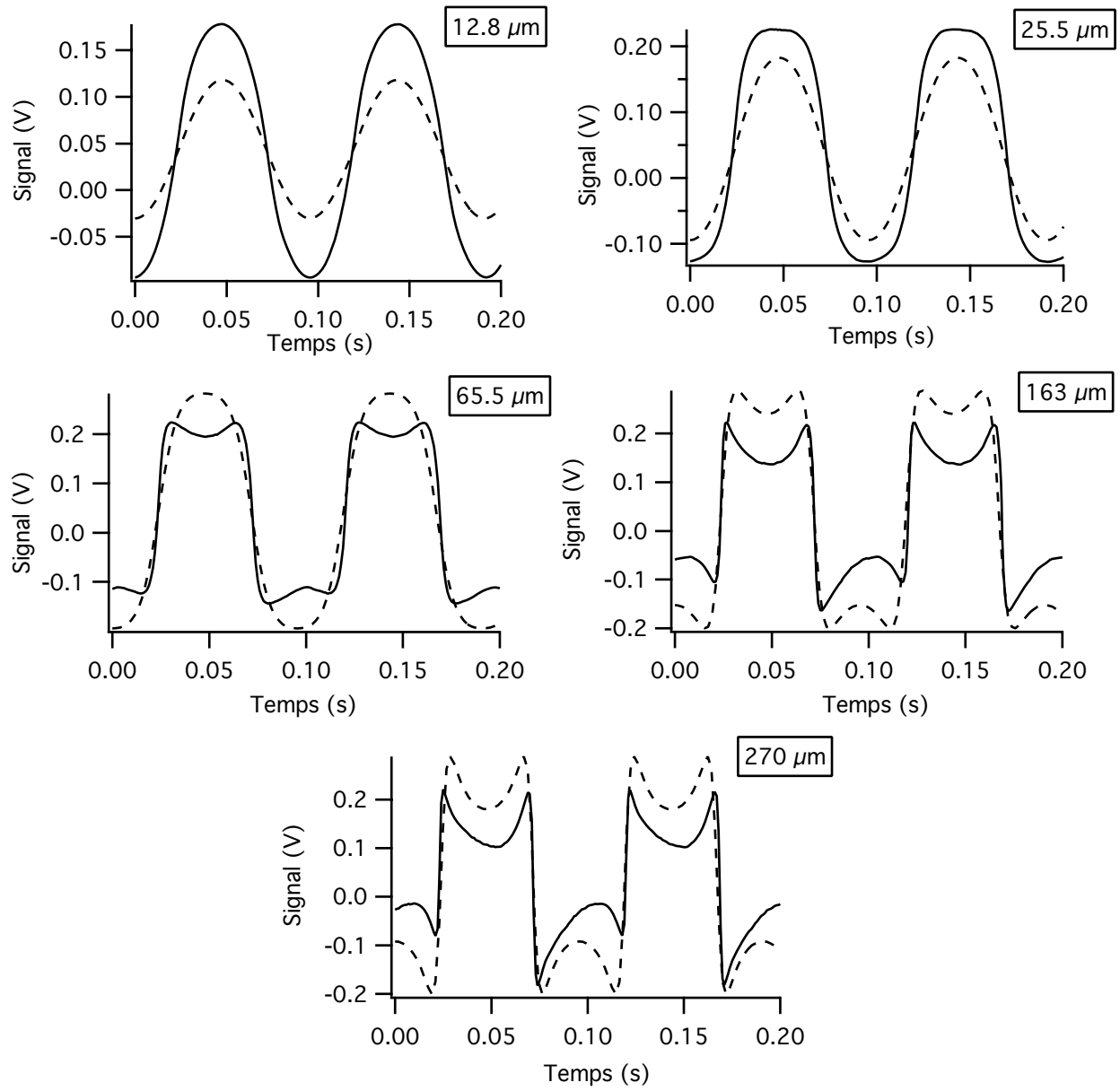
Figure III.17 : Comparaison expérience (courbe trait plein) et simulation théorique (courbe pointillée) pour \tau_o = 16 \mu\text{s} - \gamma = 0,15 \text{ cm}^{-1} - I_{s_s}^o = 1,63 \text{ V} ( f = 10 \text{ Hz} ).
