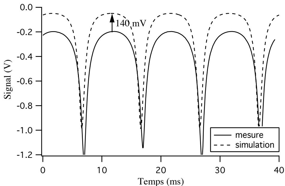
Figure IV.21 : Réponse non linéaire C théorique (courbe pointillée) et expérimentale (courbe pleine) pour un déplacement d'amplitude 36,7 \mu\text{m} .
