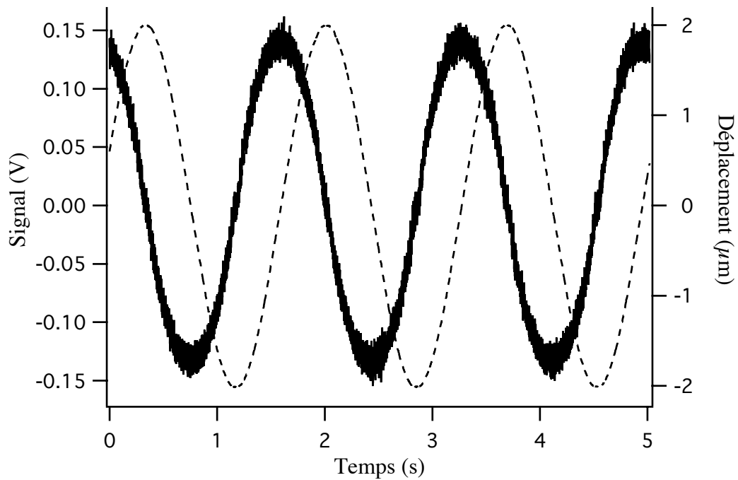
Figure III.8 : Réponse du vibromètre à une modulation de phase sinusoïdale de fréquence 0,6 Hz. La courbe en trait pointillé représente le déplacement de la cale piézo.
