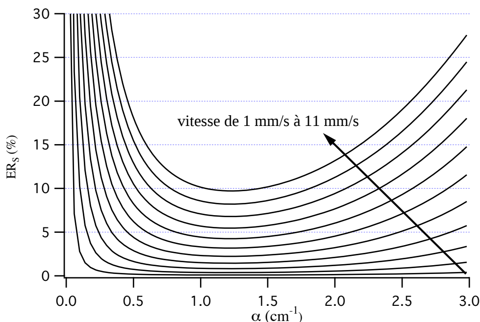
Figure III.20 : Erreur relative ER_s en fonction de l'absorption \alpha pour différentes vitesses (le temps de réponse est fixé à 1 \mu s à 1,36 \text{ cm}^{-1} ).
