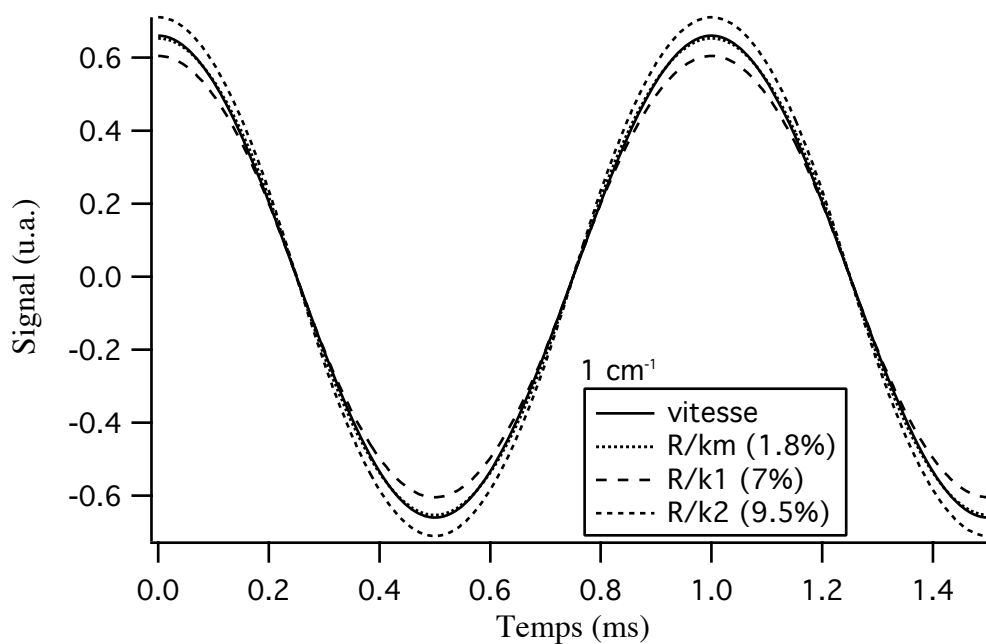
Figure IV.8 : Simulation de la réponse R normalisée pour une amplitude de 2,16 \mu\text{m} , une fréquence de 1000 \text{ Hz} , un temps de réponse de 1 \mu\text{s} et une absorption de 1 \text{ cm}^{-1} .
