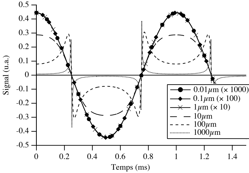
Figure III.3 : Simulation numérique de la réponse du vélocimètre à un déplacement sinusoïdal de fréquence 1 kHz à différents déplacements. Les courbes de faibles amplitudes ( 0,01 \mu\text{m} à 1 \mu\text{m} ) sont compensées. Elles se superposent exactement montrant la linéarité de la réponse du vélocimètre.
