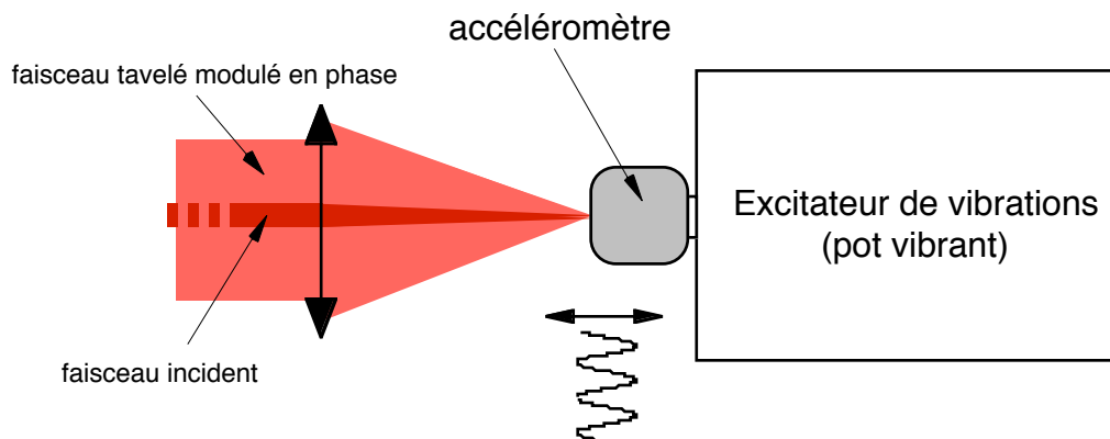
Figure III.7 : Vue du montage expérimental près de la source de vibrations.
