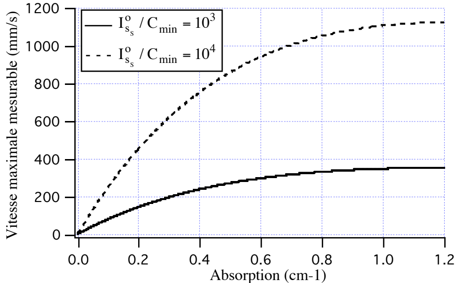
Figure IV.13 : Evolution de la vitesse maximale mesurable par le signal R en fonction de l'absorption pour un rapport signal/minimum de détection ( I_{s_s}^o/C_{\min} ) de 10^3 (trait gras) et de 10^4 (trait pointillé).
