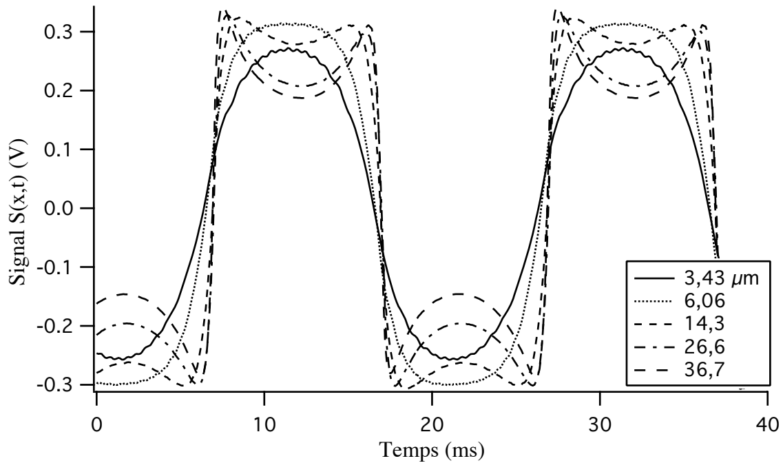
Figure IV.17 : Mesure de la réponse S(x,t) du vibromètre pour différentes amplitudes de déplacements à une fréquence de 50 Hz.
