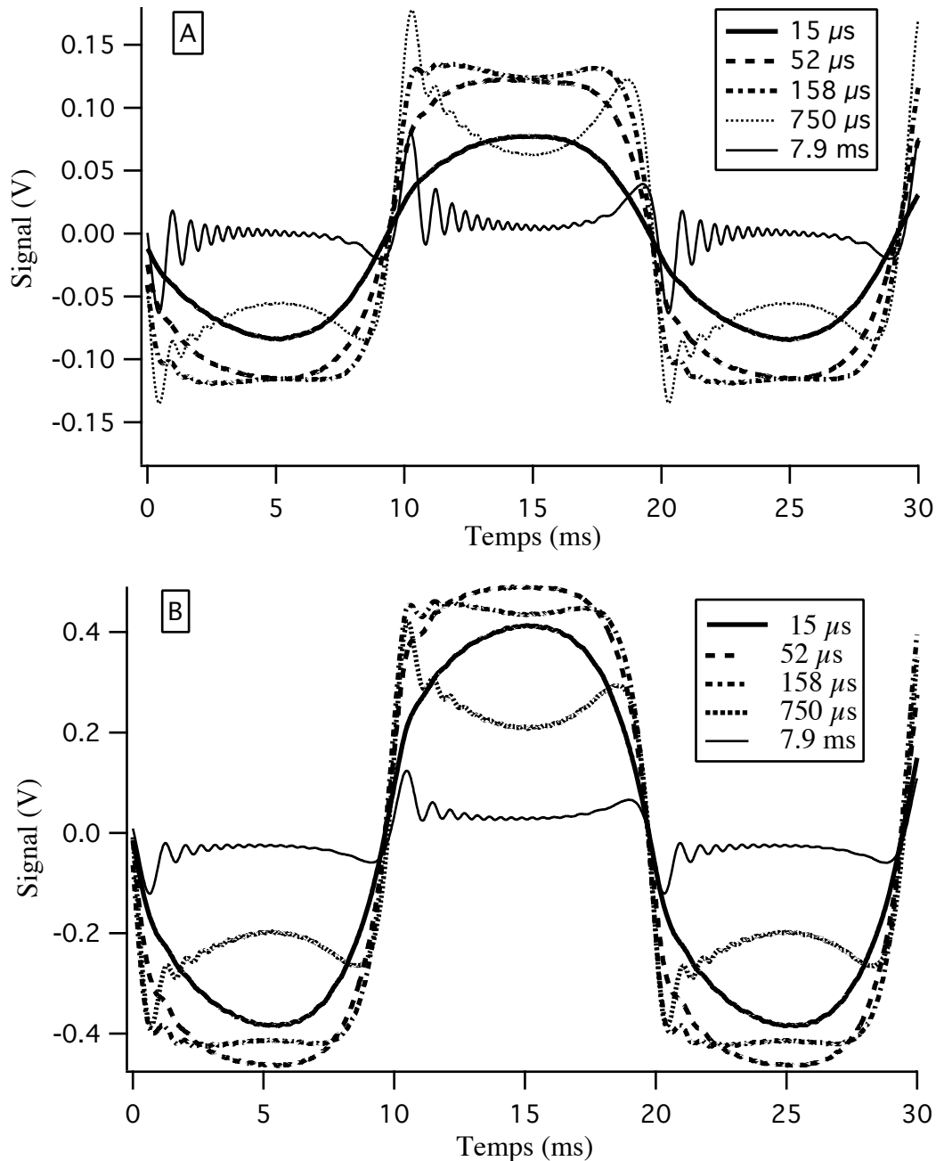
Figure III.12 : Réponse du vibromètre à une excitation sinusoïdale d'amplitude 4,5 \mu\text{m} et de fréquence 50 Hz pour différents temps de réponse du matériau. En (A) la cible est un miroir plan métallisé et en (B) une surface non polie en aluminium.
