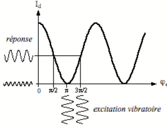
Figure I.6 : Intensité détectée lors d'une mise en quadrature \Phi_0 = 3\pi/2 ou en opposition de phase \Phi_0 = \pi/2 .
