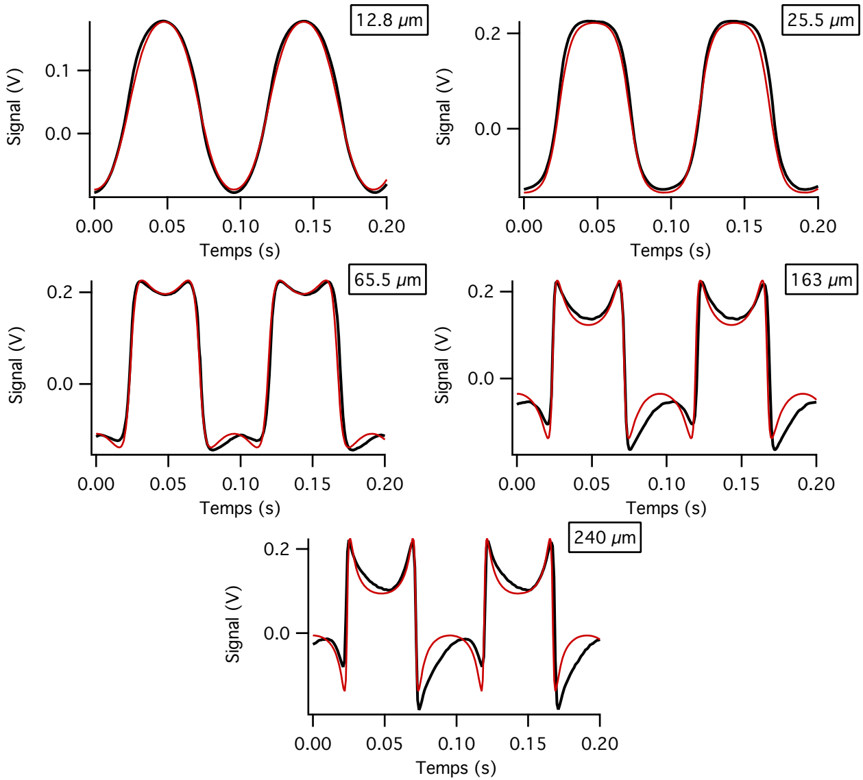
Figure III.25 : Comparaison expérience (trait épais) et simulation théorique (trait fin) pour \tau_o = 20 \mu s - \gamma = 0,12 \text{ cm}^{-1} - I_{s_s}^o e^{-\alpha x} = 1,63 \text{ V} .
