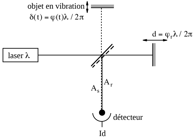
Figure I.5 : Interféromètre de Michelson.
