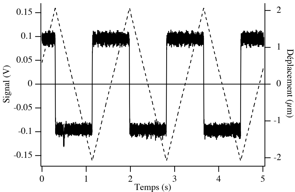
Figure III.9 : Réponse du vibromètre à une modulation de phase triangulaire de fréquence 0,6 Hz. La courbe en trait pointillé représente le déplacement de la cale piézo.
