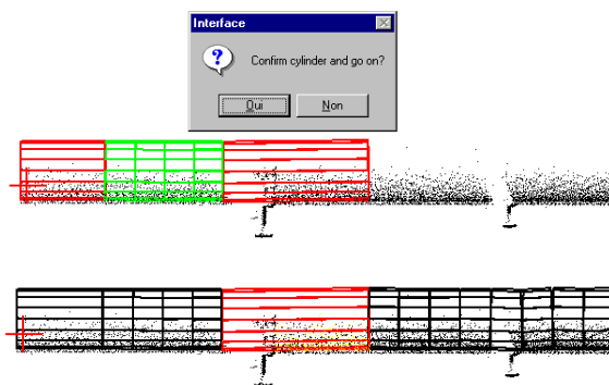
FIG. 3.26 – Adaptation de l'algorithme en présence d'ombres
