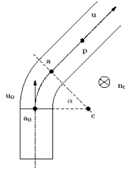
FIG. A.12 – «Cylindre après tore».
