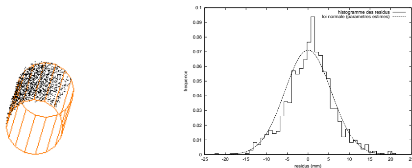
FIG. 5.14 – Histogramme des résidus et loi gaussienne (avec paramètres estimés) dans le cas d'un ajustement de cylindre sur la scène «SynthCyl2».
