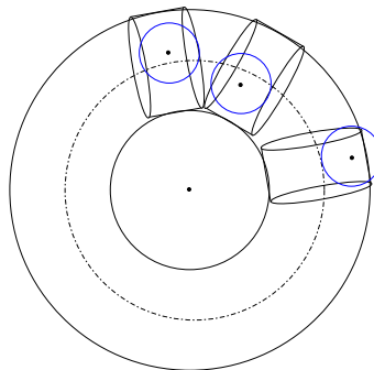
FIG. 4.21 – Principe d'initialisation des paramètres du tore par ajustement de cylindre sur des sous-nuages
