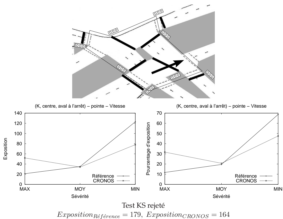
FIG. 6.13 – Courbe d'exposition en fonction de l'indicateur de proximité, dans le contexte (K, centre) pour la catégorie aval à l'arrêt, en pointe, pour les 5 échantillons traités. Les expositions totales (leur différence relative à la stratégie de Référence est supérieure à 5%) et tests KS sont aussi indiqués.
