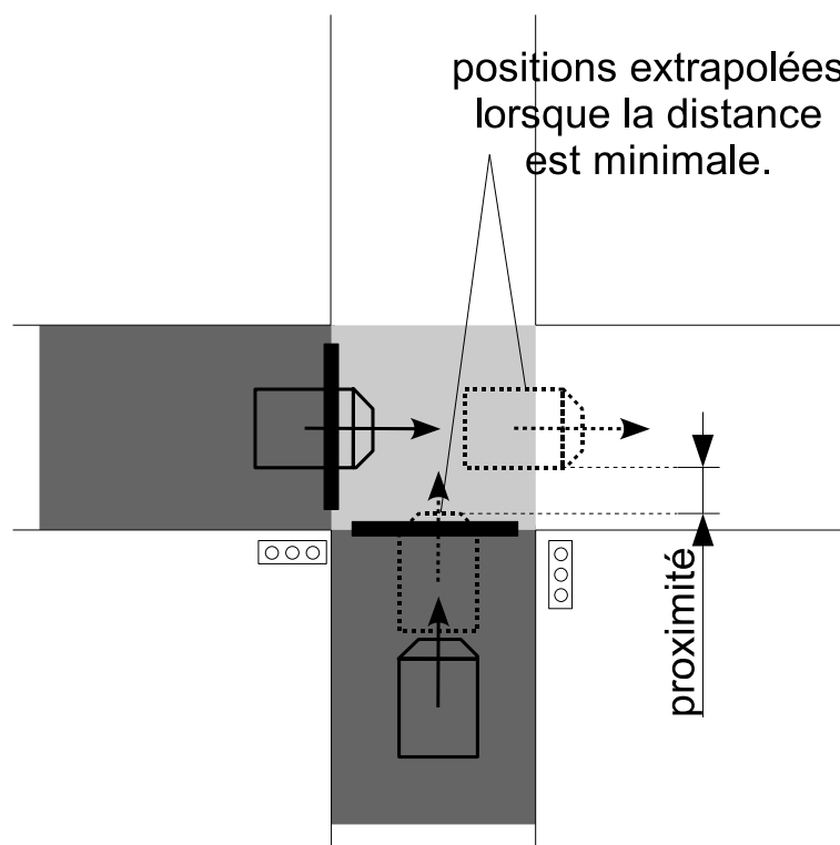
FIG. 3.5 – Illustration de l'indicateur de proximité pour une interaction de la catégorie antagoniste en mouvement.
