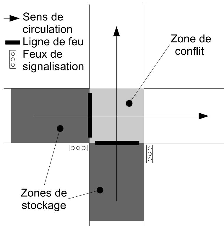
FIG. 2.1 – Une intersection : carrefour simple de deux routes à sens unique.
