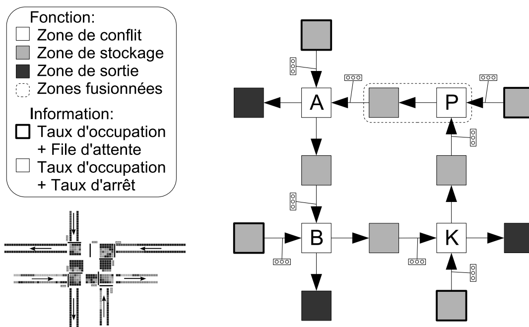
FIG. 3.4 – Schéma du carrefour au niveau de description des zones, obtenu par agrégation spatiale des pavés de chaque zone fonctionnelle du carrefour. Les informations indiquées sont celles qui alimentent CRONOS.
