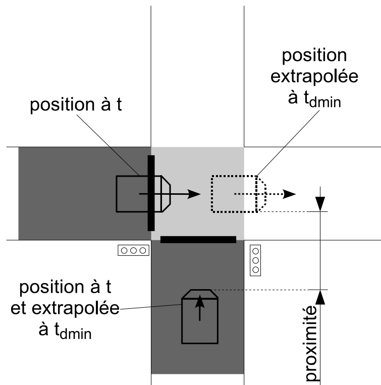
FIG. 4.6 – Illustration de l'indicateur de proximité pour une interaction de la catégorie antagoniste en mouvement et des hypothèses simplifiées d'extrapolation des trajectoires.
