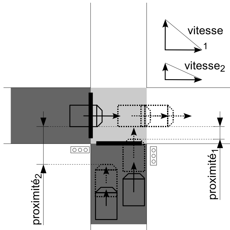
FIG. 3.7 – Illustration de la qualification d'un instant selon les indicateurs de sévérité pour deux interactions de la catégorie antagoniste en mouvement. Les mobiles en pointillés indiquent leurs positions extrapolées lorsque les distances des mobiles en interaction sont minimales. Les indicateurs d'indice 1 sont les plus sévères.
