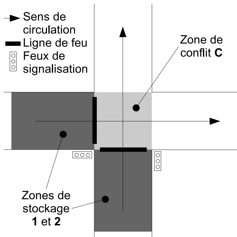
FIG. 4.2 – Plan d'une intersection simple de notre carrefour, avec la zone de conflit notée C , et les deux zones de stockage amont notées 1 et 2.
