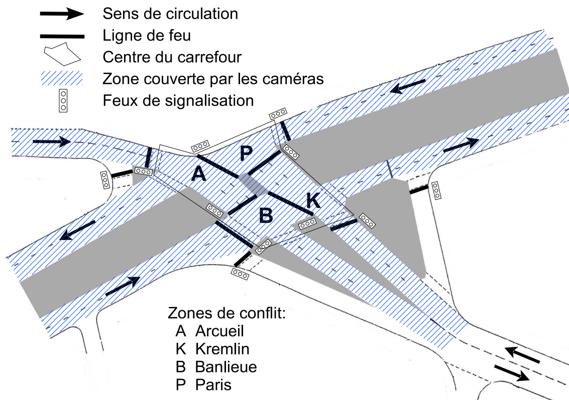
FIG. 3.2 – Site expérimental : plan du carrefour équipé.
