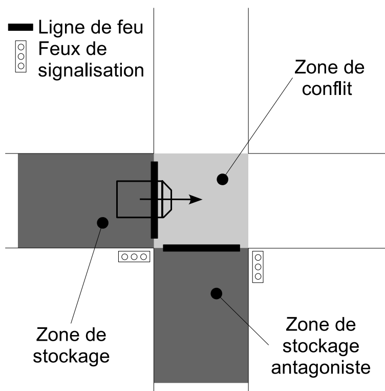
FIG. 3.1 – Une intersection : carrefour simple de deux routes à sens unique. La zone de stockage antagoniste est définie par rapport à la zone de stockage dont provient un mobile qui entre dans la zone de conflit.
