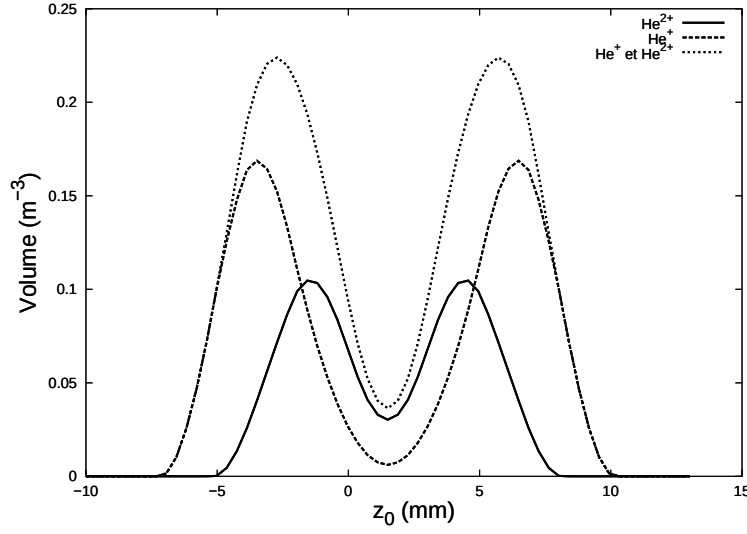
FIG. 7.8 – Evolution des volumes de \text{He}^{2+} , de \text{He}^+ , et de \text{He} au moins une fois ionisé, en fonction de la position du foyer laser z .
