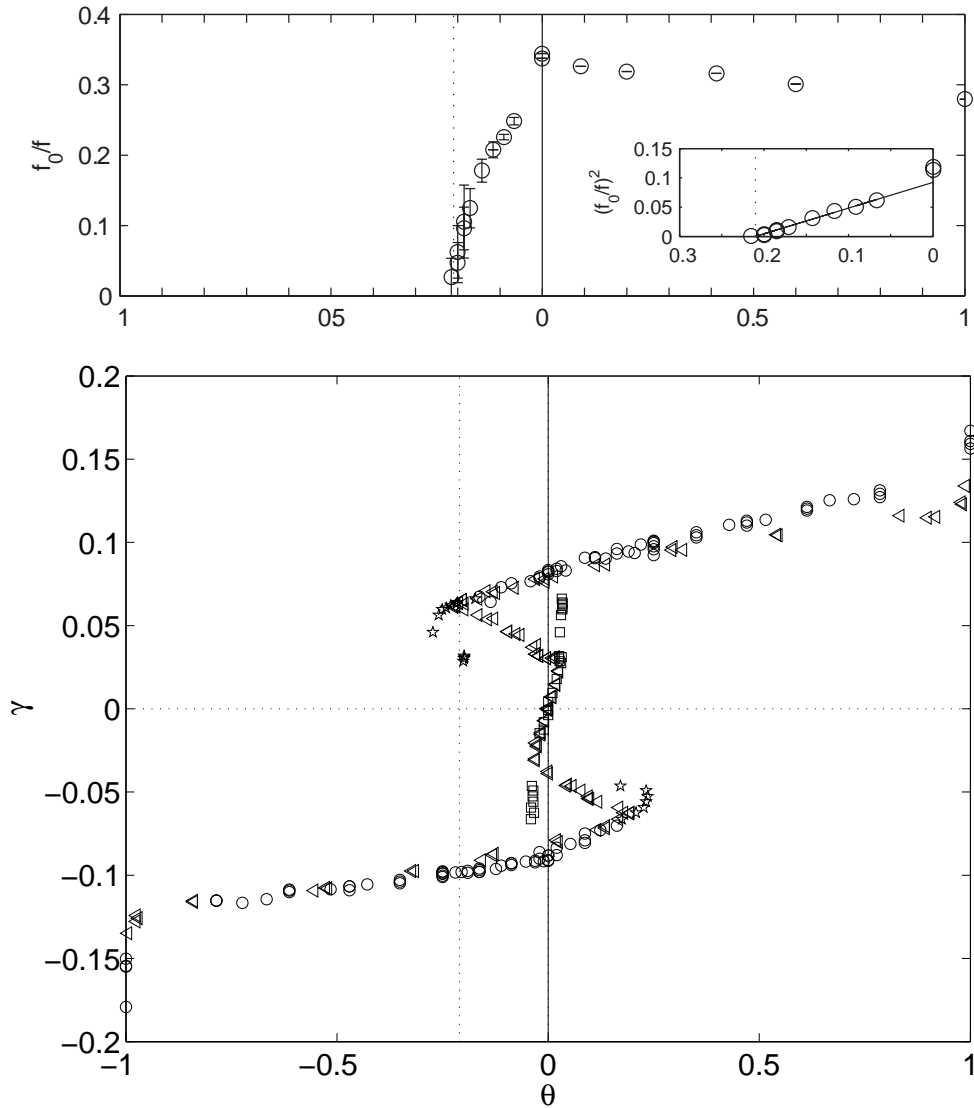
FIG. 3.43: Figure de synthèse des cycles effectués à vitesses de rotation imposées ( \circ ) ou à couples imposés ( \square , \triangle et \star ) pour les turbines TM60 2 en sens (-), dans un cylindre lisse. La figure du haut est une reproduction de la figure 3.21 page 96. Dans le cas des cycles à couples imposés, les ( \triangle ) représentent la moyenne brute de \theta , les ( \star ) représentent les états à une cellule visités de manière intermittente, et les ( \square ) représentent les états à deux cellules visités de manière intermittente.
