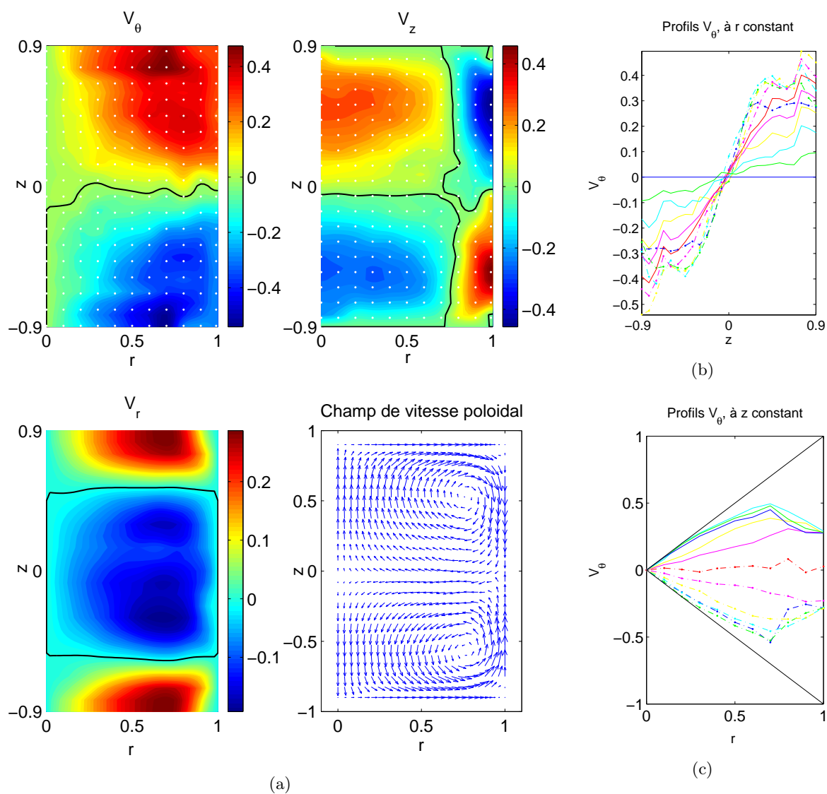
FIG. D.3: (a) Champ de vitesse adimensionnel, turbines TM73_2 en contrarotation dans le sens positif à f = 6\text{Hz} , Re = 4.7 \times 10^5 . Cylindre lisse. (b) Coupes en z de V_\theta . (c) Coupes en r de V_\theta .
