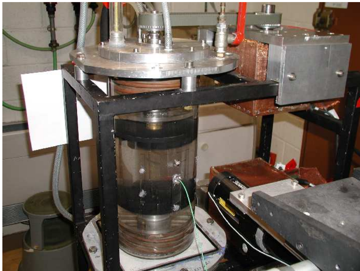
FIG. 1.3: Photographie du dispositif expérimental : les turbines sont peintes en noir. On distingue également les plaques de plexiglas de part et d'autre des turbines, ainsi que les serpentins de cuivre permettant la régulation thermique. En haut, sur la platine en aluminium, un tuyau est relié à un vase d'expansion suspendu au plafond. La courroie relie la poulie de la cage à roulements au moteur, enchâssé dans la cage en tissu de cuivre visible en haut à droite. Le fil vert relie un capteur de pression piézoélectrique monté en paroi à un amplificateur de charges. Le passage de capteur sert également aux mesures de températures par thermorésistance de platine (Pt100). Un thermomètre à alcool monté dans un doigt de gant et situé sur la platine supérieure permet un contrôle de la température.
