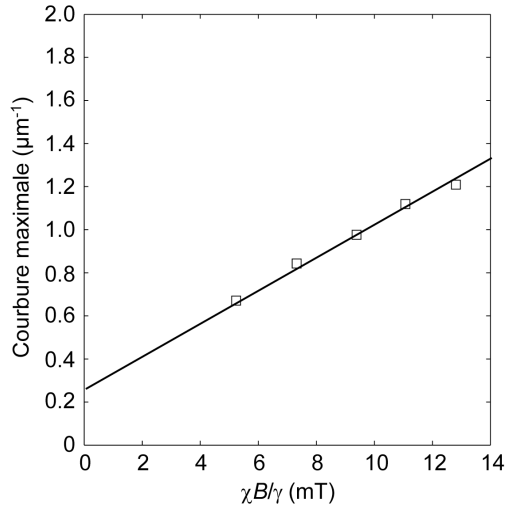
Figure 85 : relation affine entre la courbure maximale d'une épingle et le champ magnétique appliqué pour une chaîne PAA ( K_b=2.6 \cdot 10^{-22} \text{ J.m} ).
