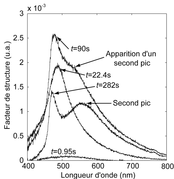
Figure 41 : croissance du pic de diffraction pris à différents temps après avoir appliqué le champ magnétique. Le pic de diffraction commence par croître car la taille moyenne des chaînes croît. Il décroît ensuite. Un pic secondaire apparaît, qui se décale vers la droite au cours du temps. On constate également le décalage du pic de diffraction vers la gauche au cours du temps.
