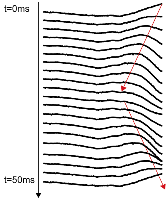
Figure 98 : illustration de ce que serait un mouvement réversible.
