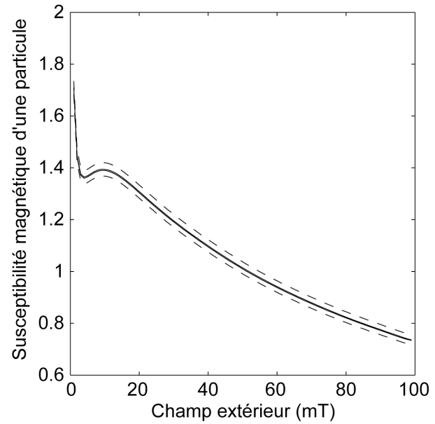
Figure 27 : susceptibilité magnétique d'une particule magnétique sphérique en fonction du champ magnétique extérieur appliqué. Les courbes en pointillées indiquent l'erreur commise sur la mesure de \chi .
