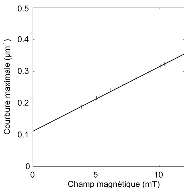
Figure 83 : relation affine entre la courbure maximale d'une épingle et le champ magnétique appliqué pour une chaîne ADN ( K_b=2.6.10^{-22}\text{J.m} ).
