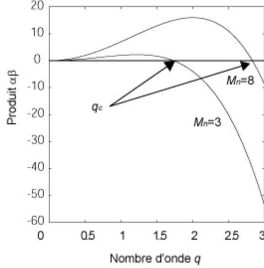
Figure 80 : représentation de la relation de dispersion.
