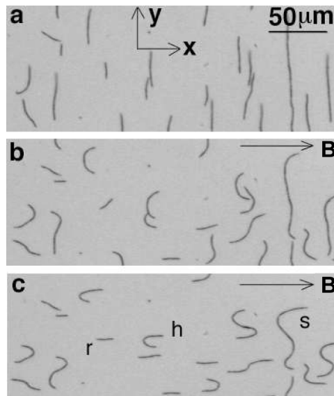
Figure 75 : déstabilisation d'un ensemble de filaments de PAA, les petites chaînes basculent en bloc (r) ou bien basculent en formant une ou plusieurs arches (h et s). Images prises par P. Jop.
