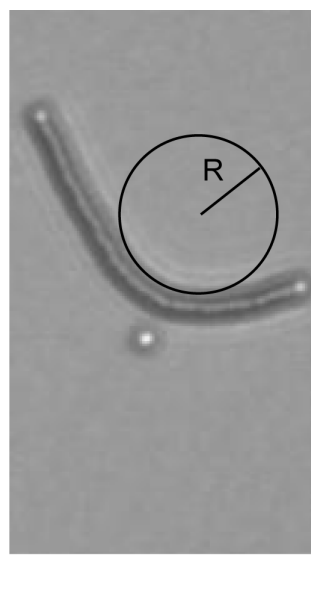
Figure 84 : courbure résiduelle d'un filament à champ magnétique nulle.
