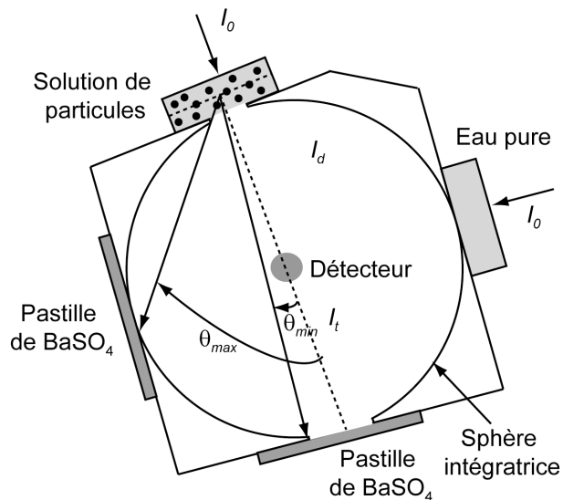
Figure 110 : définition des angles \theta_{min} et \theta_{max} utilisés dans le calcul des intensités diffusées et transmises.
