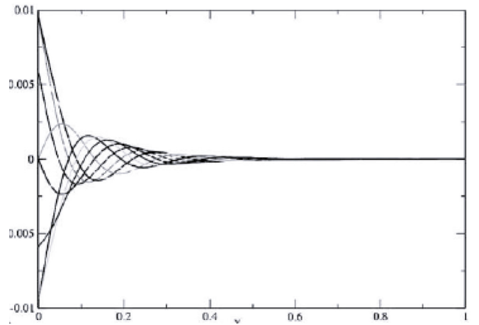
Figure 63 : filament à haut S_p . Seule une portion du filament se déforme [Lagomarsino, 2003].
