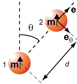
Figure 16 : définition des notations qui apparaissent dans l'expression du champ magnétique créé par le dipôle 1 à l'endroit où se trouve le dipôle 2.
