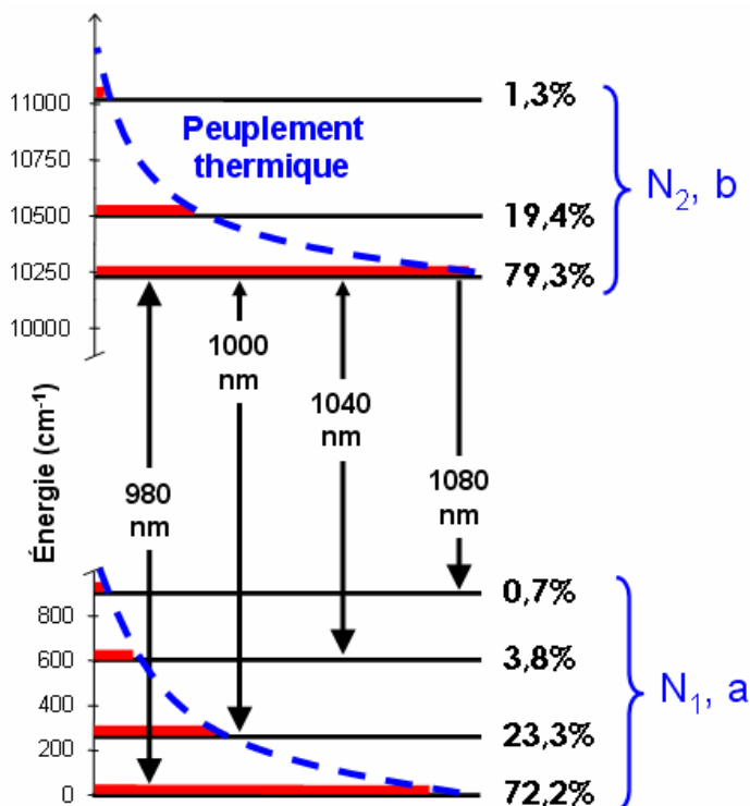
Figure B-4 : Répartition des niveaux d'énergie et des populations de chaque sous-niveau pour le site d'accueil n°2 dans Yb:YSO (pour les transitions d'absorption et d'émission du champ selon la polarisation X) sous l'influence d'un champ de pompe (pour que le multiplet excité soit peuplé). Les longueurs d'ondes correspondant aux maxima des transitions sont reportées. Les facteurs de peuplements f_a et f_b sont reportés à côté de chaque sous-niveau a ou b pour une température de 300\text{ K} . La population totale du multiplet fondamental est notée N_1 et la population totale du niveau excité est notée N_2 .
