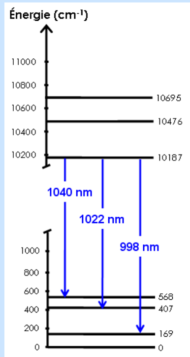
Niveaux énergétiques et transitions possibles pour \text{Yb:KYW} .
