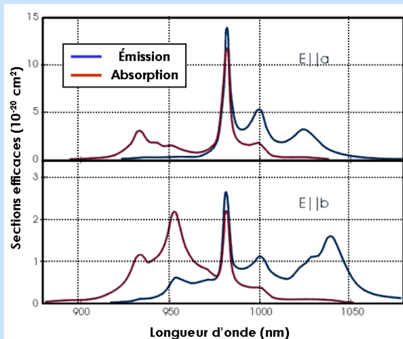
Spectres d'absorption (en rouge) et d'émission (en bleu) selon les deux polarisations accessibles ( a et b ) de \text{Yb:KYW} .
