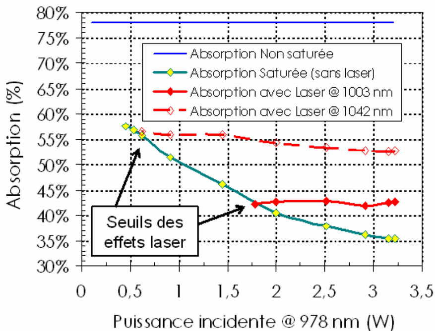
Figure B-8 : Graphique représentant l'absorption du faisceau de pompe à 978 nm par un cristal de Yb:YSO pour différents régimes, avec ou sans effet laser. On retrouve la valeur de l'absorption non saturée et l'évolution de l'absorption saturée en fonction de la puissance de pompe avec et sans effet laser pour 2 longueurs d'ondes d'émission différentes.
