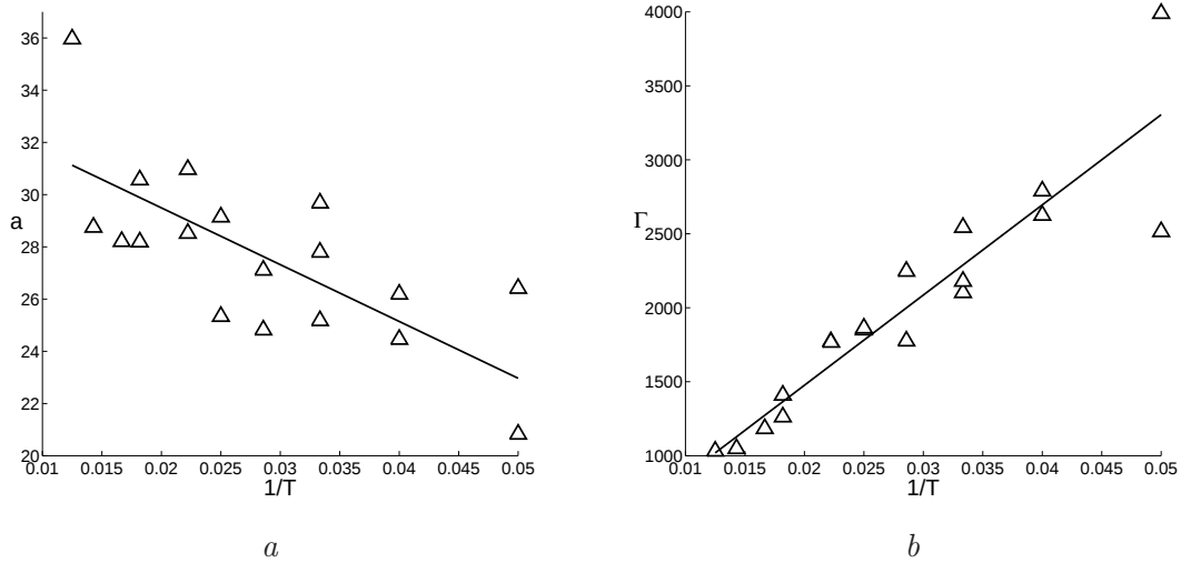
FIG. 5.13 – Évolution de (a) la taille des coeurs des tourbillons a (en mm ) et (b) de leur circulation \Gamma (en mm^2s^{-1} ) en fonction de la vitesse de rotation des flaps. a_i et \Gamma_i sont représentés par les symboles \triangle . Les fits a_f et \Gamma_f sont représentés en traits pleins.
