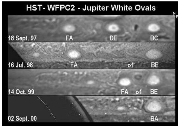
FIG. 1.4 – Quatre images des tempêtes appelées Ovaes Blanches de Jupiter prises entre septembre 1997 et septembre 2000 par le télescope Hubble. Le diamètre des Ovaes Blanches varie entre 8000 km et 12000 km. Sur l'image du haut, on distingue trois Ovaes Blanches. En 1998, les deux tempêtes les plus à l'est se sont appariées. En octobre 1999, les dernières images montrent que les deux Ovaes Blanches restantes se rapprochent et s'apparient. D'après le Space Telescope Science Institute of Baltimore, NASA, ESA.
