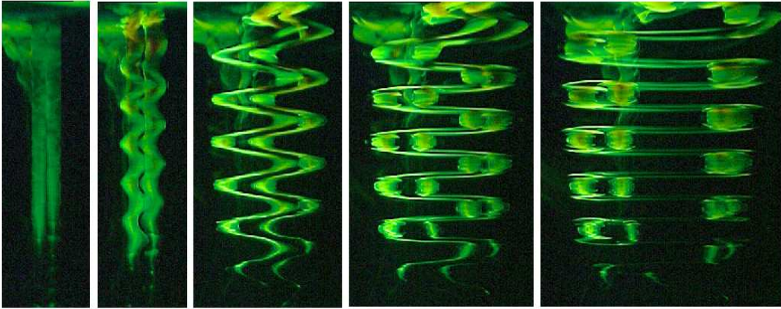
FIG. 1.22 – Développement de l'instabilité zigzag agissant sur une paire de tourbillons contra-rotatifs verticaux dans un fluide fortement stratifié. Les tourbillons sont visualisés par de la fluorescéine. D'après Billant & Chomaz (2000 a ).
