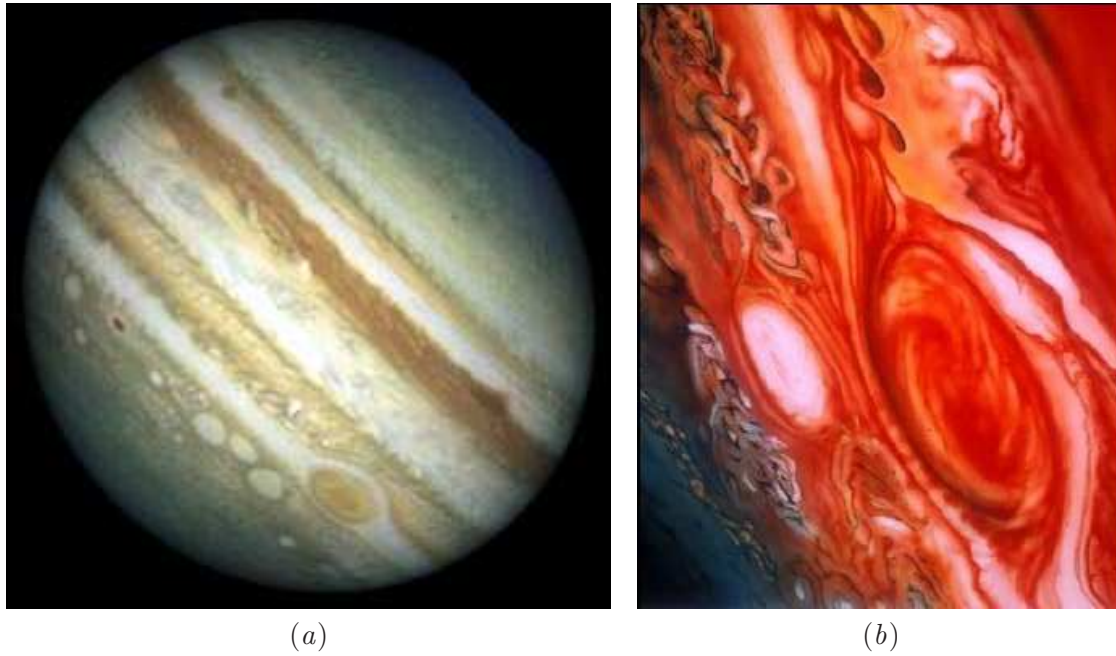
FIG. 1.1 – (a) Image de Jupiter montrant ses trois Ovaux Blanches et son Point Rouge (en bas à droite). (b) Zoom sur le Point Rouge et une Ovale Blanche. D'après Hubble, NASA.
