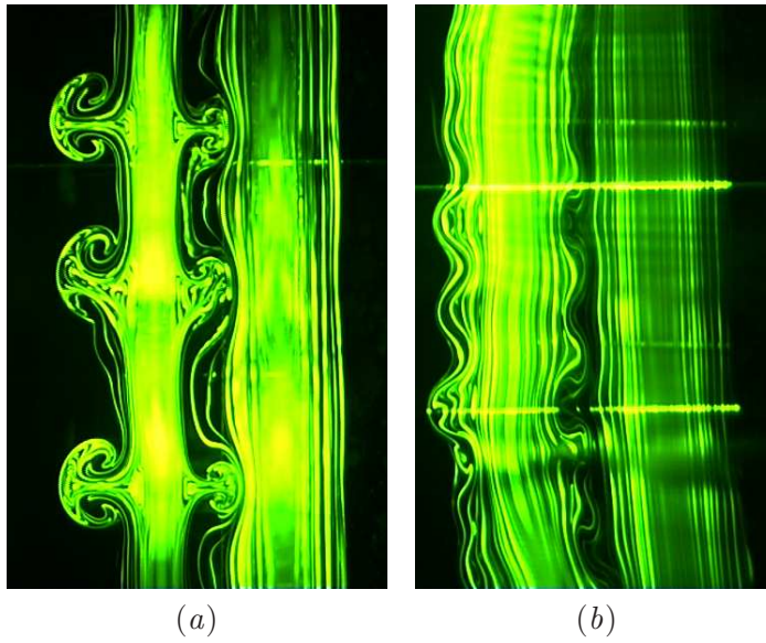
FIG. 2.7 – (a) Exemple d’instabilité centrifuge agissant sur un tourbillon anticyclonique (à gauche) dans une cuve tournante. Un tourbillon cyclonique (à droite), moins visible car moins chargé en fluorescéine est stable centrifuge. (b) Instabilité centrifuge asymétrique oscillante correspondant à m=1 . D’après Billant et al. (2004).
