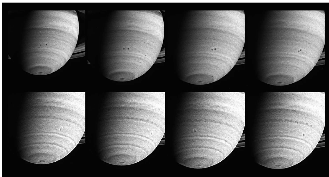
FIG. 1.5 – Appariement de deux tempêtes d'environ 1000 km de diamètre dans l'atmosphère de l'hémisphère sud de Saturne. Photos prises entre le 22 février et le 22 mars 2004. Dans les quatres images du haut, les deux tempêtes s'approchent lentement avant de s'apparier. En bas, les quatre images ont été prises à quatre jours d'intervalle et montrent la rapide axisymétrisation de la structure appariée. D'après le Space Science Institute of Boulder, NASA, ESA, ISA.
