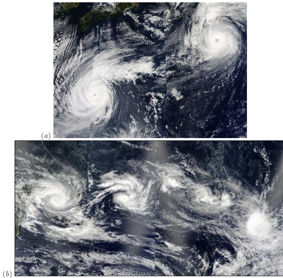
FIG. 1.8 – (a) Typhons Parma (à droite, vents de 170 km/h) et Ketsana (à gauche, vents de 250 km/h) au Sud du Japon le 24 octobre 2003. (b) Cyclones Gerry, Hape, 18S et Fiona sur l’océan Indien à l’est de Madagascar (visible à gauche) le 12 février 2003. D’après J. Schmaltz, MODIS, satellites Terra et Aqua de la NASA.
