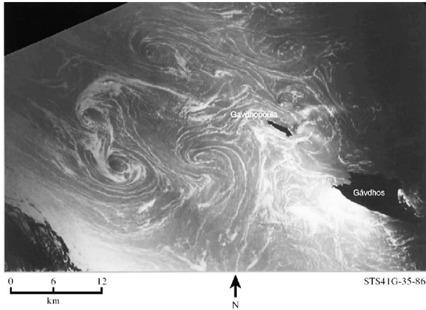
FIG. 1.14 – Mer Méditerranée au sud de la Crète. Une paire de spirales interconnectées se distingue en particulier à gauche. On distingue clairement le point de stagnation entre ces deux tourbillons. Les images ont été prises par des navettes volant entre 200 et 400km d'altitude et la visualisation des spirales est rendue possible par la réflexion des rayons du soleil. D'après Munk et al. (2000).
