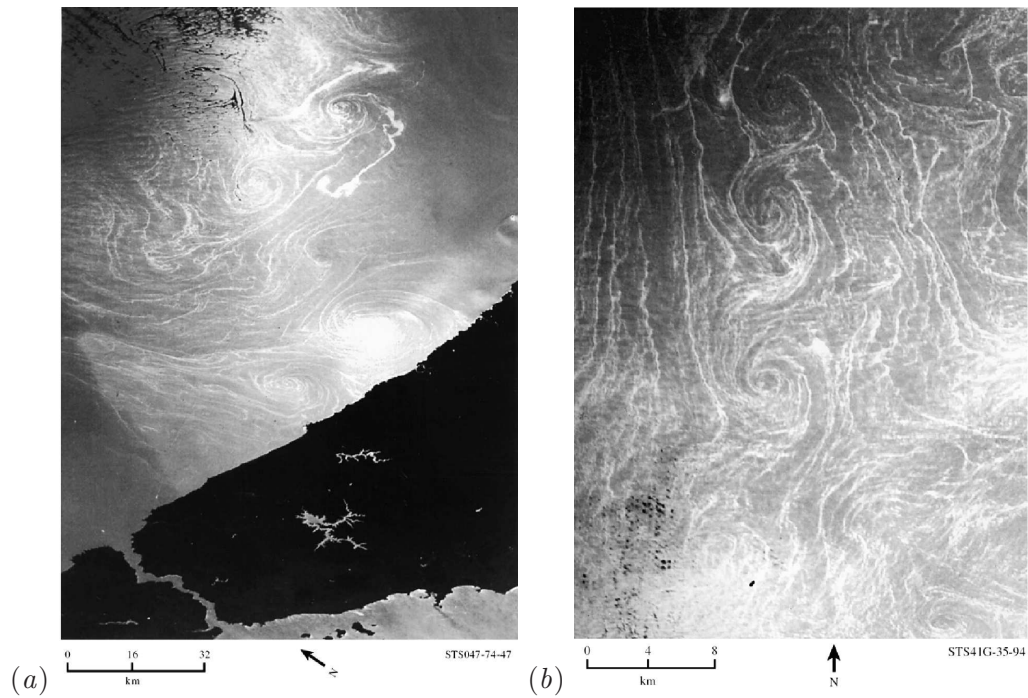
FIG. 1.15 – (a) Spirales dans la Mer Noire au large d’Istanbul le 18 septembre 1992. Une première paire à 20km de la côte, une deuxième paire à 50km. (b) Quatre spirales interconnectées en Mer Méditerranée au large de l’Egypte le 7 octobre 1984. D’après Munk et al. (2000).
