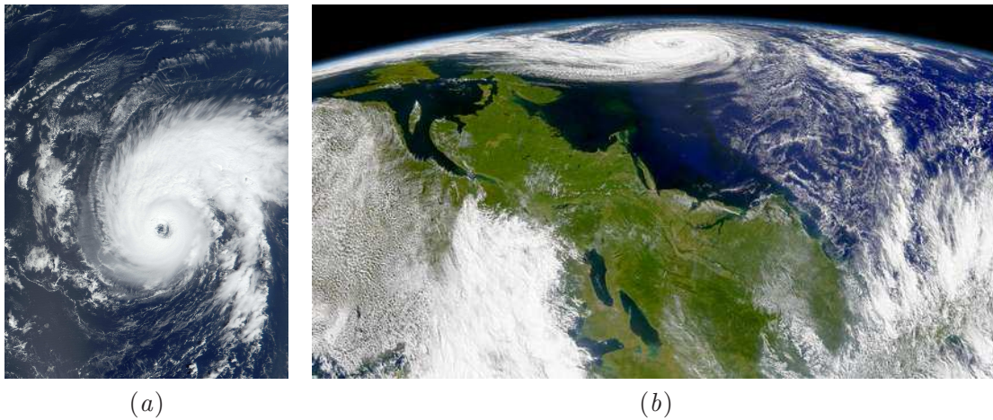
FIG. 1.11 – Ouragan Erin (a) vue de dessus à l'est des Bermudes le 12 septembre 2001 ; (b) vue de côté le 9 septembre 2001. La côte nord-est de l'Amérique est visible. D'après J. Descloitres, MODIS et Goddard Space Flight Center et ORBIMAGE, NASA.
