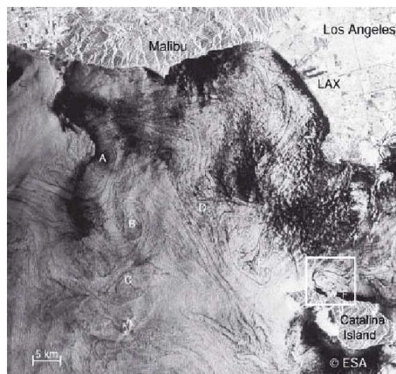
FIG. 1.16 – Petits tourbillons côtiers dans la Baie de Santa Monica en Californie le 19 décembre 1994. Les tourbillons A et B sont les plus gros (rayon de 8\text{km} environ), les tourbillons C, D, E et F sont plus petits (rayon de 3\text{km} environ). D’après ERS-1 SAR, DiGiacomo & Holt (2001).
