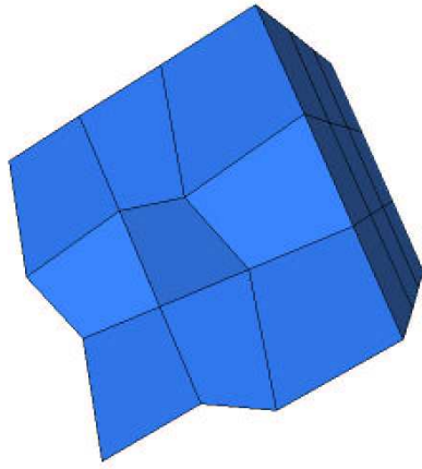
FIG. 3.4 – Maillage hexaédrique légèrement modifié
