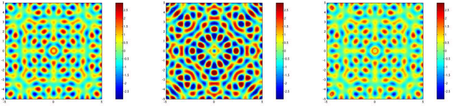
FIG. 7.2 – Point source dans une cavité. À gauche, solution numérique de référence, au milieu solution numérique avec une intégration exacte, à droite avec une intégration approchée. Quadrilatères de la première famille, maillés avec 60 points par longueur d’onde.
