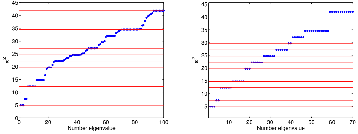
FIG. 5.14 – Distribution des valeurs propres en utilisant les points de Gauss à gauche, et les points de Gauss-Lobatto à droite. Les lignes horizontales symbolisent les valeurs propres analytiques.
