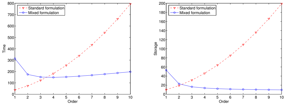
FIG. 2.3 – A gauche temps de calcul, à droite stockage
