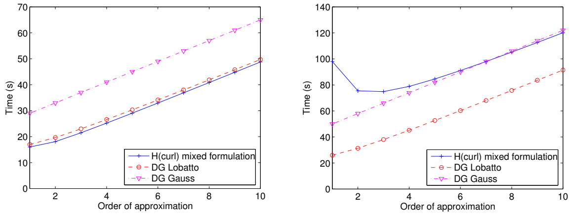
FIG. 6.2 – À gauche temps de calcul en fonction de l'ordre d'approximation pour le cas 2-D, à droite cas 3-D. Nombre de ddl constant.
