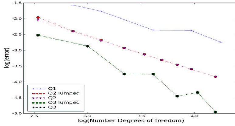
FIG. 3.7 – Convergence du mode numérique vers le mode analytique en fonction du nombre de ddl. Echelle log-log, norme L^2 , maillages réguliers.
