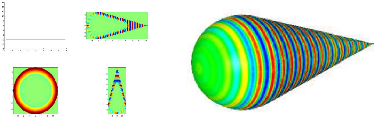
FIG. 3.22 – Partie réelle du champ total pour un cone sphère. A gauche, coupe intérieure, à droite valeur du champ sur la surface extérieure.
