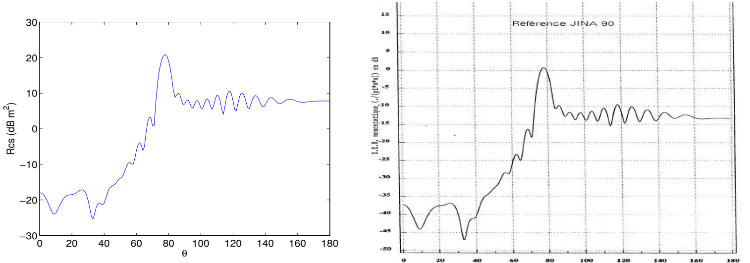
FIG. 9.25 – Ser pour un cône-sphère revêtu. A gauche, résultat fourni par notre code, à droite référence du JINA. Polarisation HH
