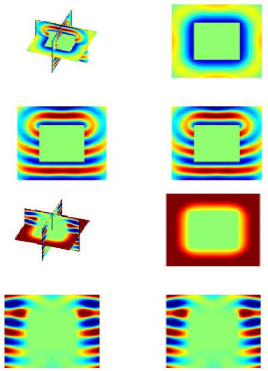
FIG. 1.20 – En haut, partie réelle du champ diffracté, en bas, partie réelle du champ total
