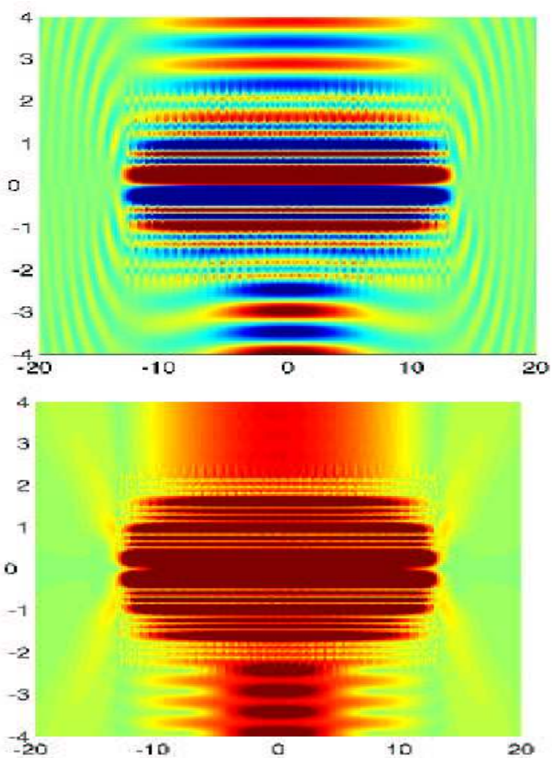
FIG. 1.27 – Solution pour un diamètre D=40.2\mu m , une fréquence relative F de 1.0001 (décalage de la longueur d'onde de -0.1548452nm ), waist w = 9.92\mu m . En haut, partie réelle du champ total, en bas, le module. Les unités sont comptées en \lambda_0 = 1.55\mu m : les longueurs physiques sont obtenues en multipliant par 1.55\mu m .
