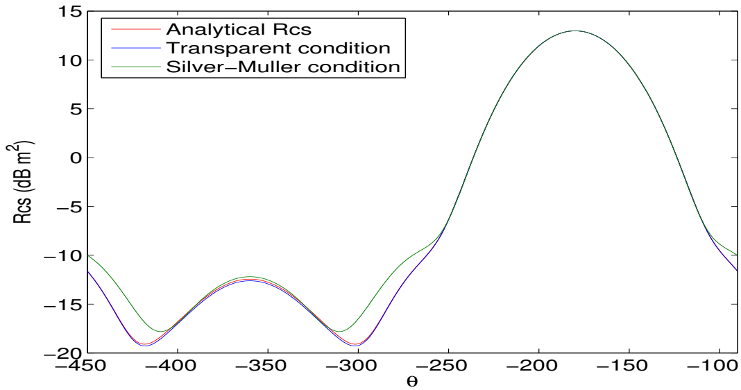
FIG. B.3 – SER d’une sphère diélectrique de rayon 1.0 . k = \pi , \epsilon_r = 1.5 , la frontière extérieure du domaine de calcul est placée sur une sphère de rayon 1.5 . En rouge, SER avec la condition transparente. En bleu, SER obtenue analytiquement. Le maillage utilisé compte 11\,000 degrés de liberté.
