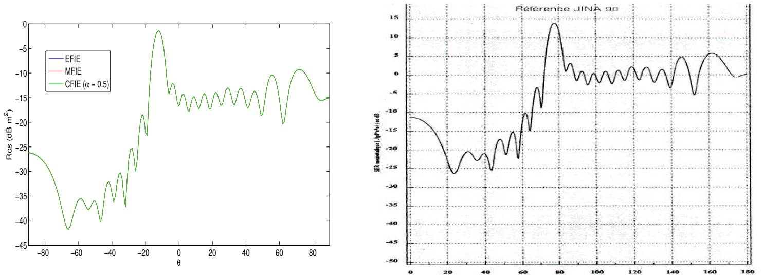
FIG. 9.18 – Ser pour un cône-sphère parfaitement conducteur. A gauche, résultat fourni par notre code, à droite référence du JINA. Polarisation HH
