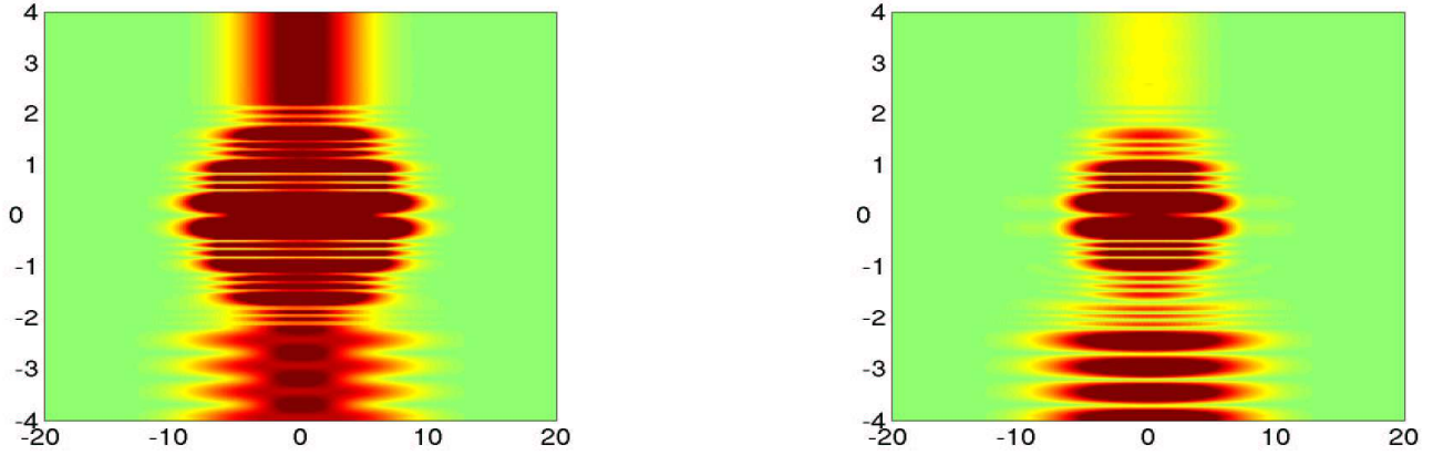
FIG. 1.30 – Solution pour un diamètre D=40.2\mu\text{m} , une fréquence relative F de 1.000732 (longueur d'onde de 1.548866\mu\text{ m} ), waist w = 9.92\mu\text{m} . A gauche, solution de référence ; à droite solution pour Q_2 avec 10 points par longueur d'onde
