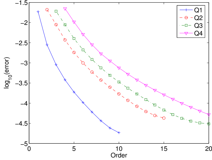
FIG. 9.4 – Evolution de l'erreur L^\infty sur l'intégrale extérieure en fonction de k ( k + 1 points de quadrature) pour divers ordres d'approximation
