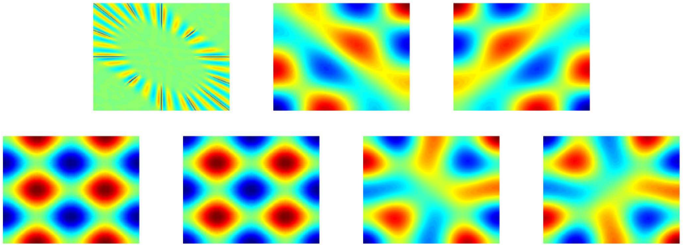
FIG. 6.16 – Quelques modes propres pour un maillage triangulaire découpé (approximation Q_5 ). Utilisation des points de Gauss
