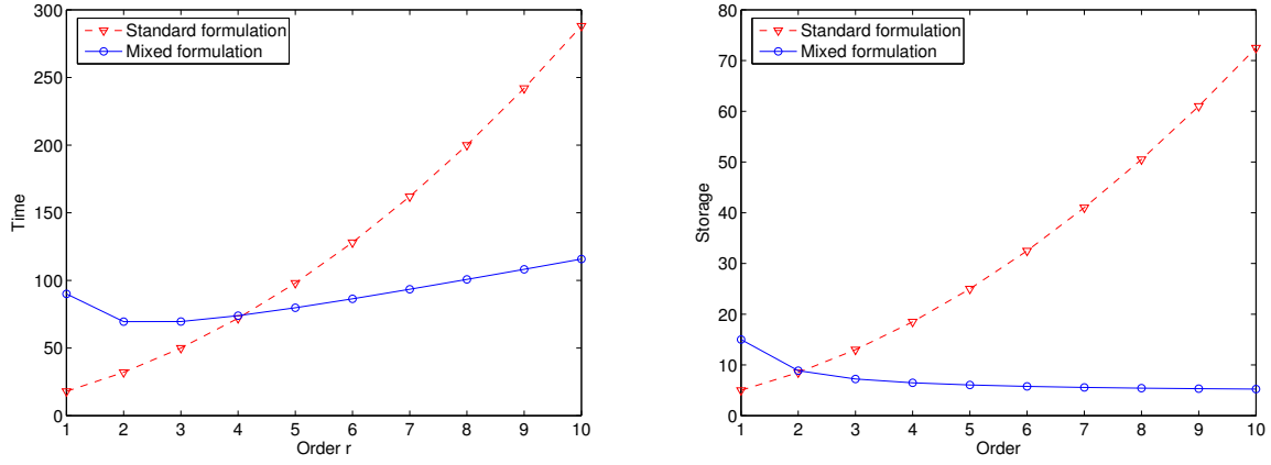
FIG. 2.2 – A gauche temps de calcul en fonction de l'ordre d'approximation, à droite stockage
