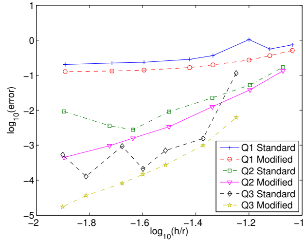
FIG. 8.3 – Evolution de l'erreur L^2 pour la FV E, E_\theta et la FV U, E_\theta . Courbes en échelles log-log. Maillages triangles découpés et intégration exacte ((r+1)^2 points de Gauss)
