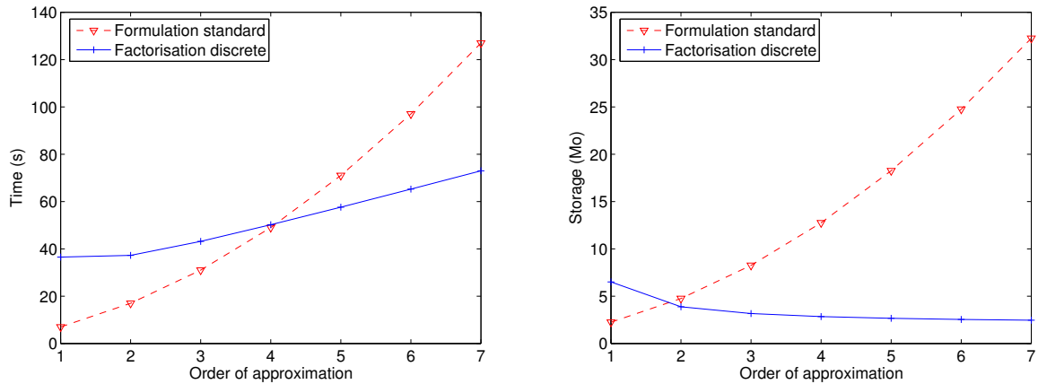
FIG. 5.9 – À gauche temps de calcul en fonction de l'ordre d'approximation, à droite stockage. Première famille sur les quadrilatères. Nombre ddl constant.
