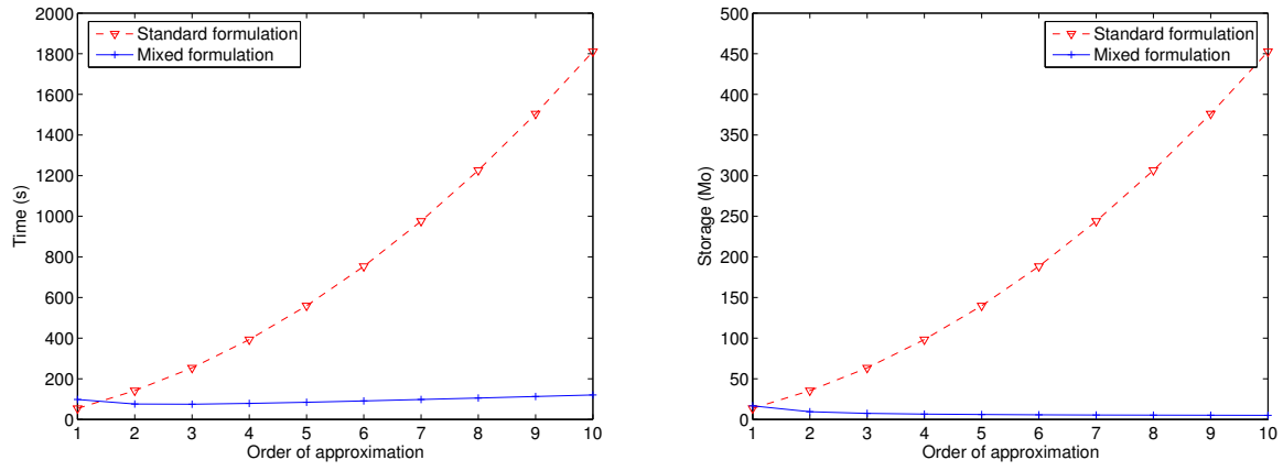
FIG. 4.3 – A gauche temps de calcul en fonction de l'ordre d'approximation, à droite stockage. Nombre ddl constant.
