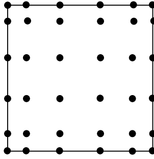
FIG. 1.3 – Les 36 points de Gauss-Lobatto pour des éléments spectraux Q_5 en 2D
