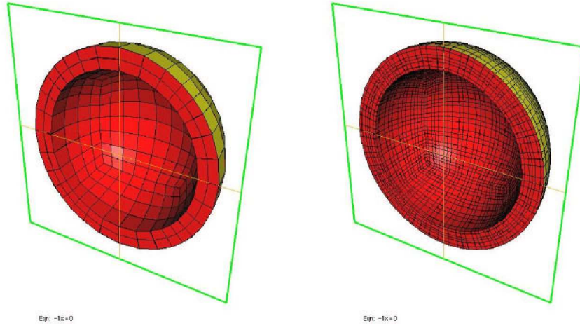
FIG. 2.11 – À gauche, maillage Q_3 , à droite sous-maillage Q_1
