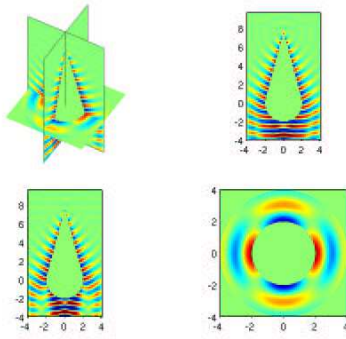
FIG. 8.6 – Partie réelle du champ diffracté par une onde plane pour un cone-sphère parfaitement conducteur. L’onde plane est axiale, elle vient par le haut.
