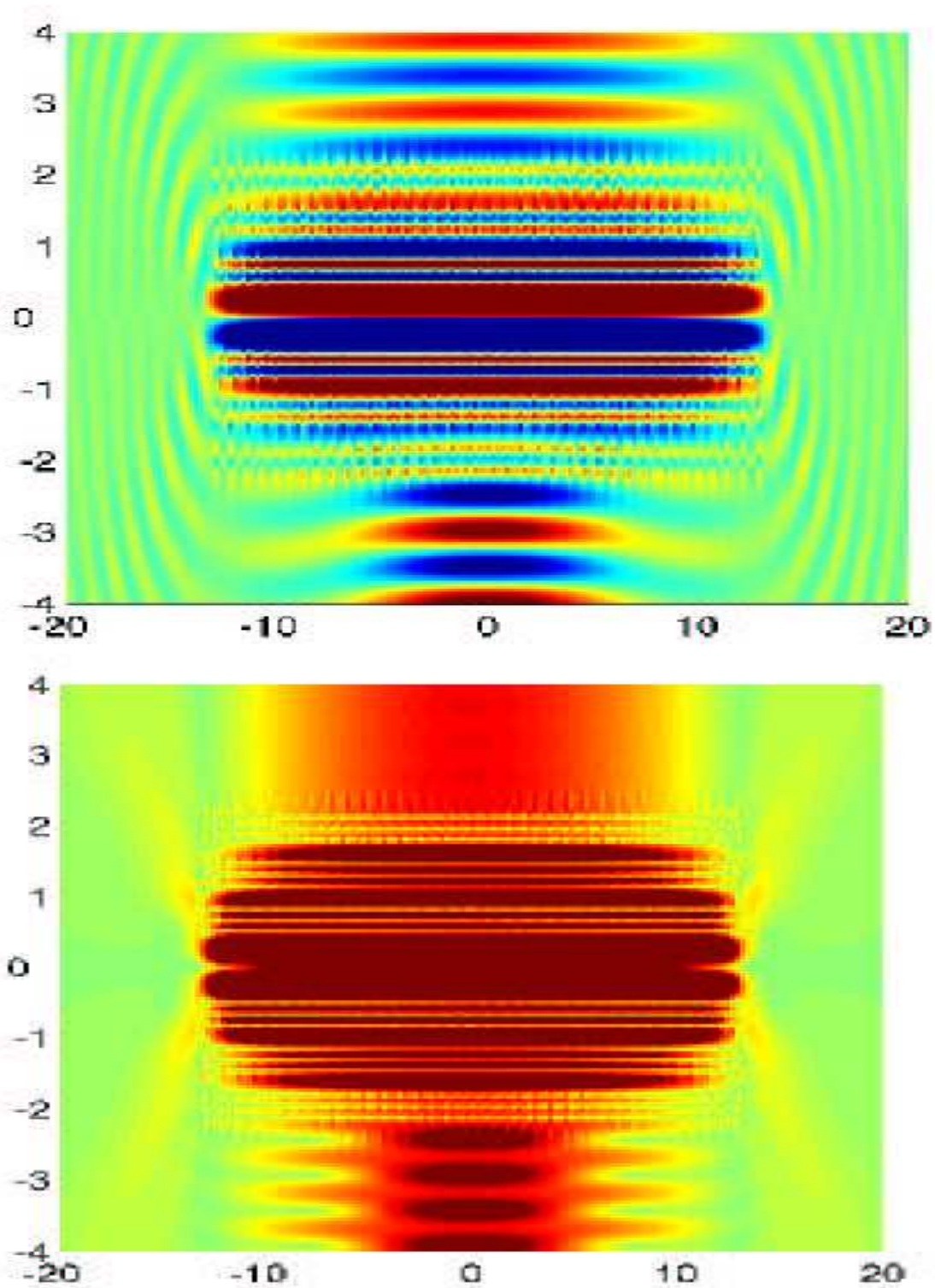
FIG. 1.27 – Solution pour un diamètre D=40.2\mu m , une fréquence relative F de 1.0001 (décalage de la longueur d'onde de -0.1548452\text{ nm} ), waist w = 9.92\mu m . En haut, partie réelle du champ total, en bas, le module. Les unités sont comptées en \lambda_0 = 1.55\mu m : les longueurs physiques sont obtenues en multipliant par 1.55\mu m .
