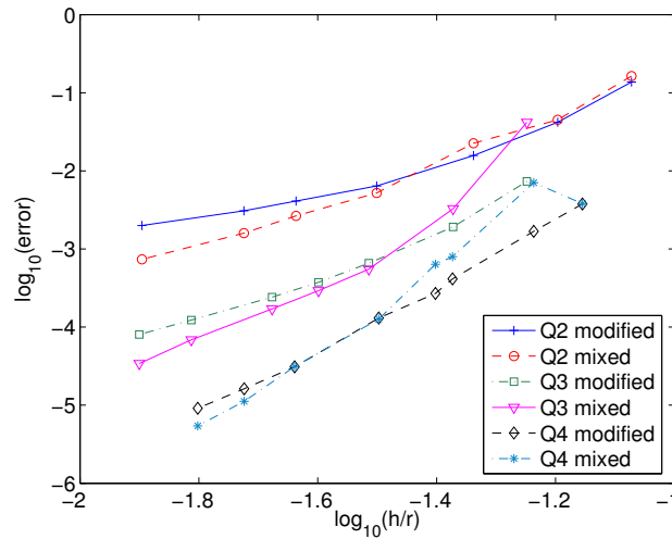
FIG. 8.4 – Evolution de l’erreur L^2 pour la FV mixte E, E_\theta et la FV mixte U, E_\theta . Courbes en échelles log-log, maillages triangles découpés et intégration exacte.
