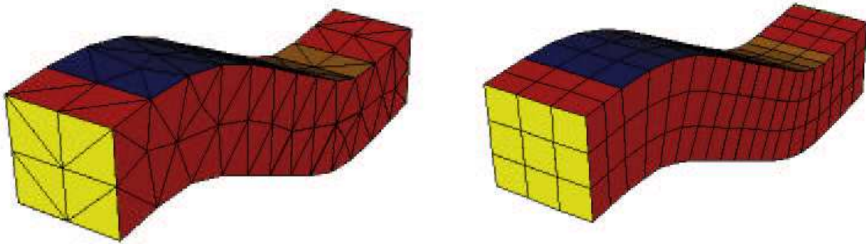
FIG. 3.19 – Maillage de la cavité en tétraèdres à gauche, en hexaèdres à droite
