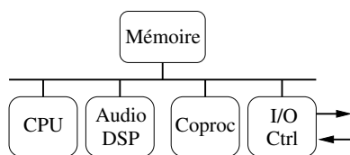
FIG. 2.1 – Architecture typique d'un système pour portable.
