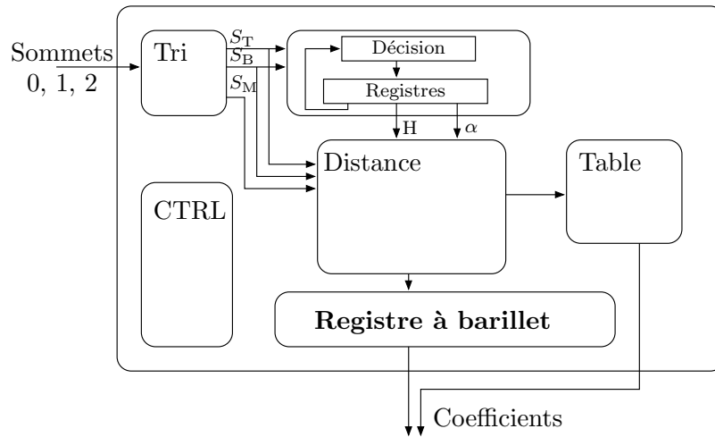
FIG. 8.17 – Diagramme en bloc d'un opérateur d'initialisation.
