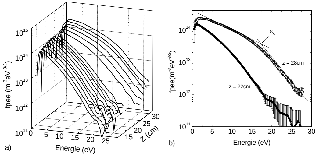
FIG. 4.5 : Fonction de probabilité en énergie des électrons dans le cas de la double couche statique ( C = 8\% , 0,13 \text{ Pa} , 600 \text{ W} ) . (a) Evolution axiale des eepf (tronquées à 23 \text{ eV} pour les altitudes z < 25 \text{ cm} ). (b) Eepf à 3 \text{ cm} au-dessus et 3 \text{ cm} au-dessous de la double couche statique (mêmes conditions).
