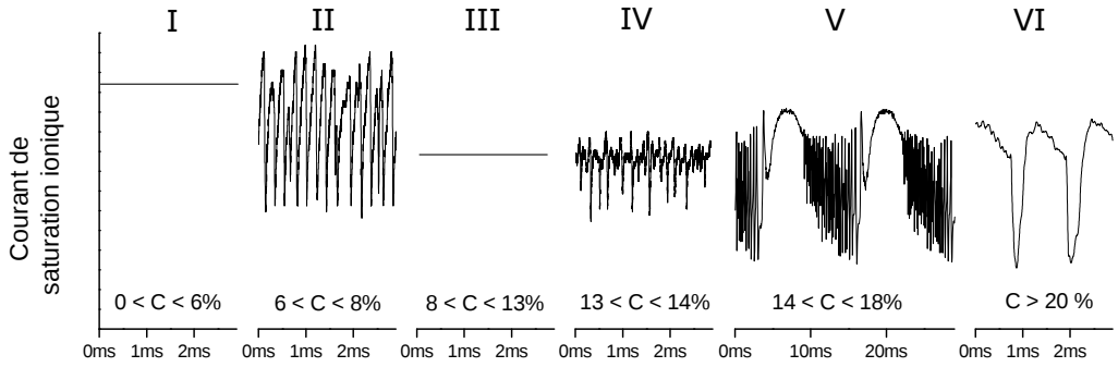
FIG. 3.12 : Évolutions typiques du courant de saturation ionique pour des concentrations C croissantes de \text{SF}_6 pour une position z = 23 cm à puissance constante. Régime I : diffusion continue du plasma (régime indépendant du temps). Régime II : diffusion continue et ondes acoustiques ioniques. Régime III : diffusion non linéaire ; double couche statique (régime indépendant du temps). Régime IV : déstabilisation de la double couche statique. Régime V : Double couche propagative (très lente) et ondes acoustiques ioniques. Régime VI : Double couche propagative (décrite en section 3.3)
