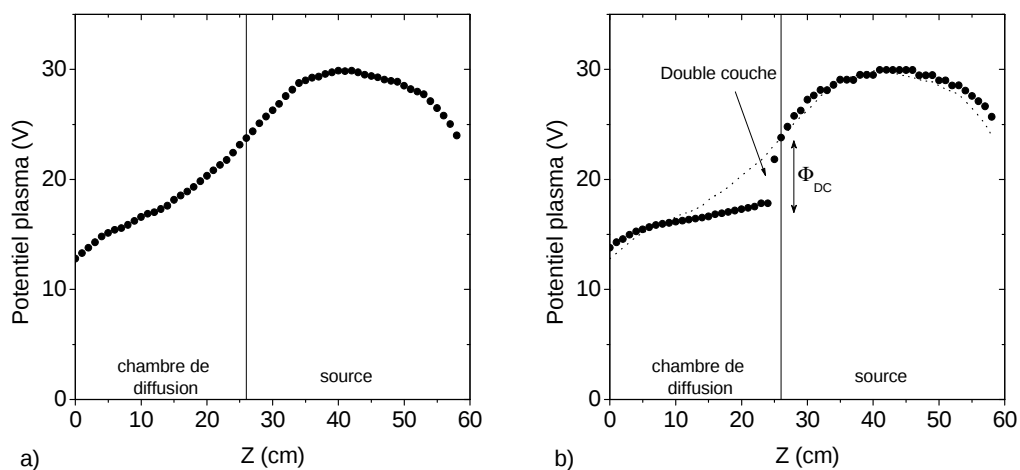
FIG. 4.1 : Évolution axiale du potentiel plasma en mélange \text{Ar}/\text{SF}_6 : (a) Concentration C = 4\% (b) C = 8\% . La ligne pointillée reprend le cas argon pur. Pression 0,13 Pa, puissance 600 W
