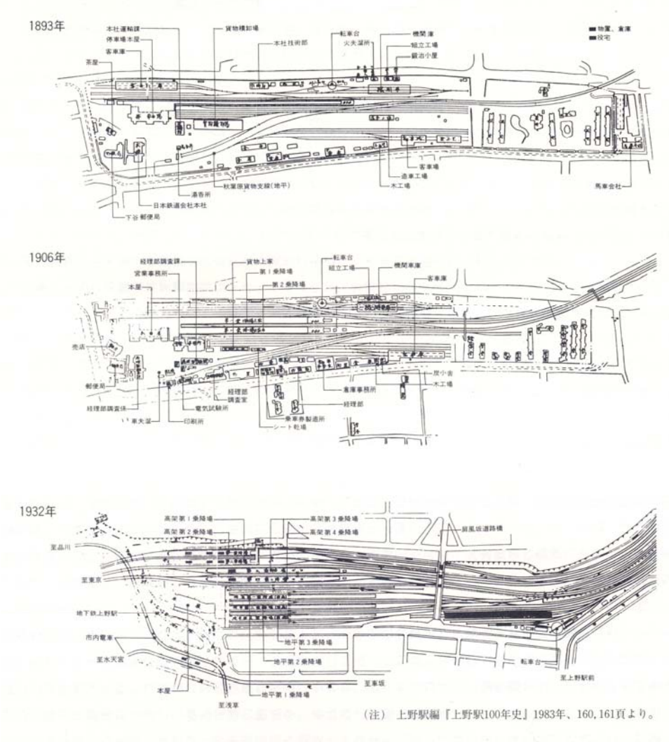
Figure 454 Transition de type de gare à Ueno (1892, 1906, 1932)
