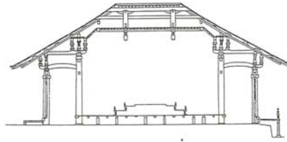
图 3-1 東大寺法華堂側面断面図、正堂正面断面図
