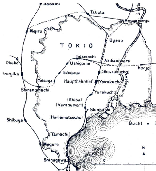
Figure 450 Plan du réseau des chemins de fer à Tokyo proposé par Bartzer (1903)
