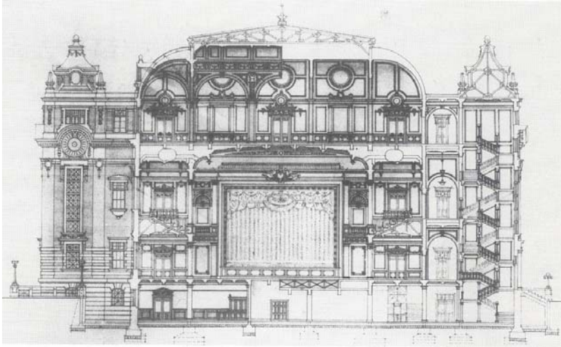
Figure 804 Auditorium de la ville d'Osaka (1918) : ferme avec 8 contrefiches inclinées
