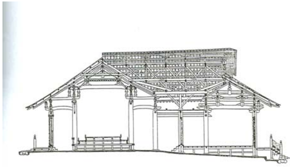
图 3-1 東大寺法華堂側面断面図、正堂正面断面図
