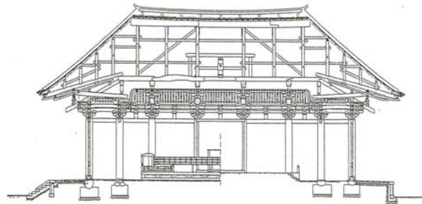
图 3-2 興福寺東金堂側面、正面断面図
