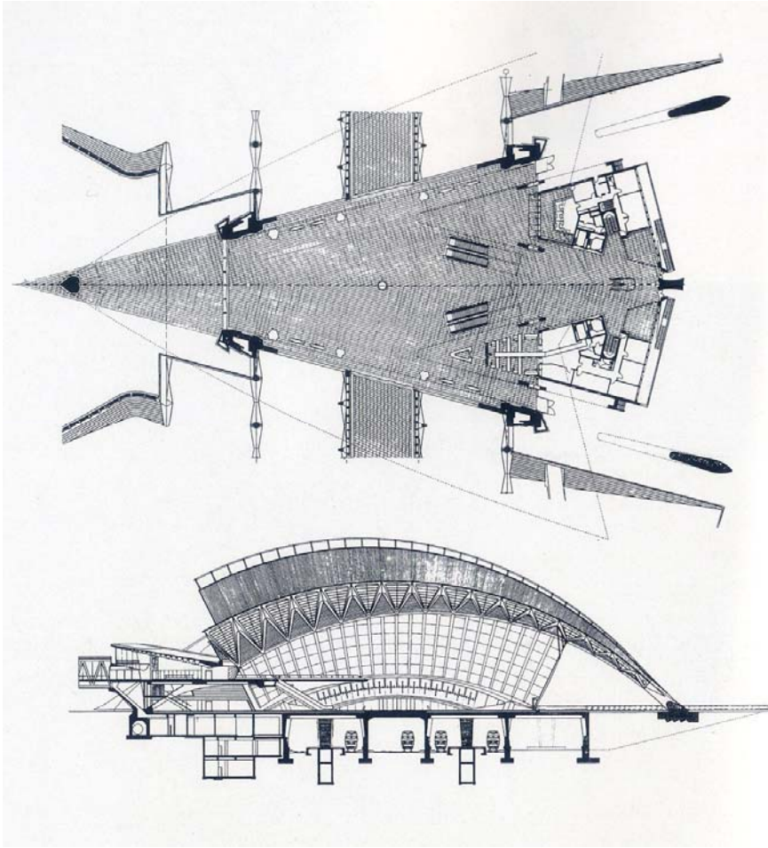
Figure 879, 880 Plan et coupe de Satolas
