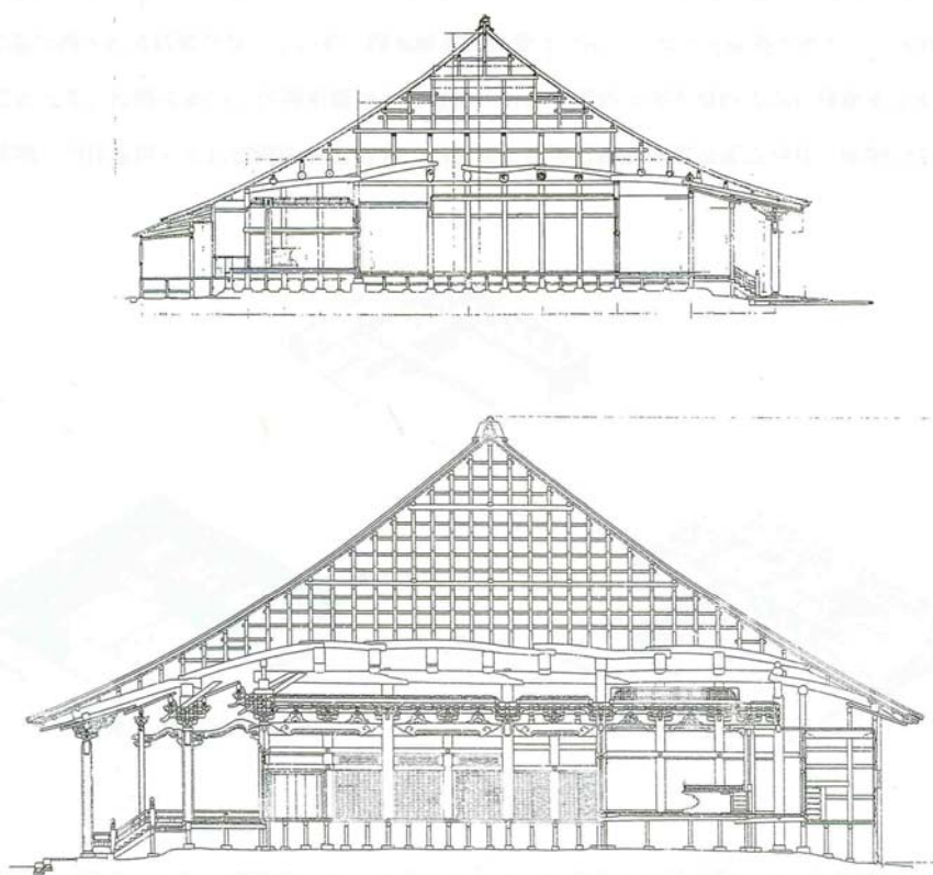
Figure 837 Sections comparatives du Hondô du temple de la secte de Jôdoshinshû, Temples de Daitshûji, de Nishihonganji, 1/400
