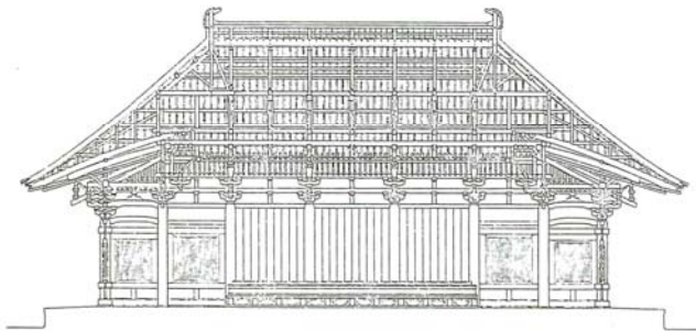
图 3-2 興福寺東金堂側面、正面断面図
