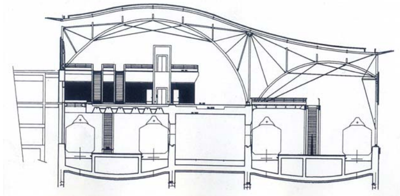
Figure 884 Coupe de Lille Europe
