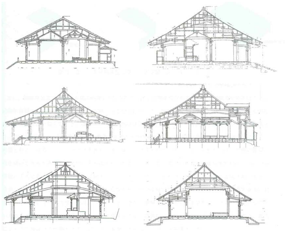
Figure 834 Coupes des temples avec le « Kondô » et le « Raidô » aux différents systèmes de plafond, Temples de Taimadera, de Kongôrinji, de Saimyôji, de Jôgonin, de Jôrokuji, de Daigoji, 1/400
