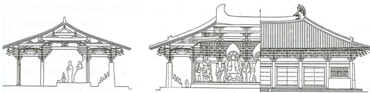
Figure 833 Coupes comparatives des temples de Tôshôdaiji (776, Japon) et de Bukkôji (Chine, 857), 1/400
