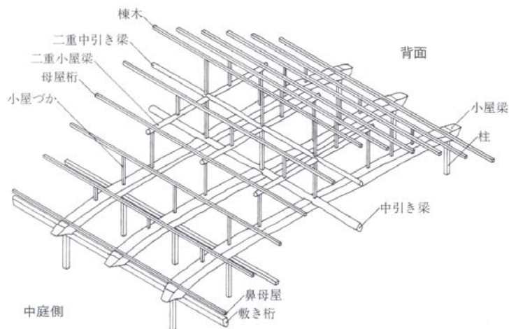
Figure 779 Charpente japonaise « wagoya » de l'Hôtel de la préfecture de Mie
