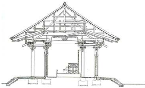
图 3-2 興福寺東金堂側面、正面断面図
