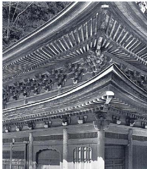
Figure 781 Détail de l'ogidaruki du hall de Shariden du Temple d'Enkakuji (1398)
