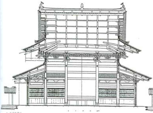
Figure 838 Halls (Butsuden) de la secte de Zenshū, Les temples de Daitokuji, de Myōshinji, de Manpukuji, 1/400
