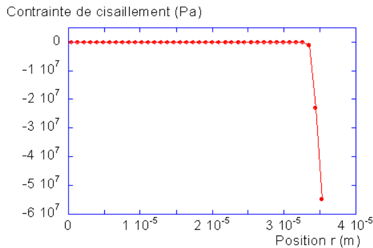
FIG. II.13 – La contraite de cisaillement de surface dans le cas d'une sphère tronquée et un chargement linéairement réparti.
