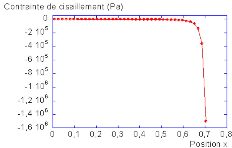
FIG. II.12 – La contraite de cisaillement de surface sur un talus.
