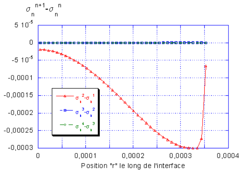
FIG. II.27 – La différence \sigma_n^{i+1} - \sigma_n^i entre deux itérations.
