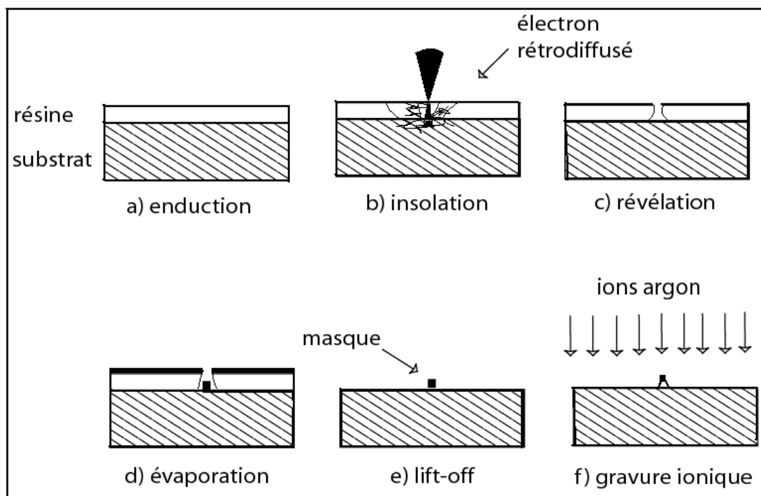
FIG. VI.3: Schéma des différentes étapes de la fabrication.
