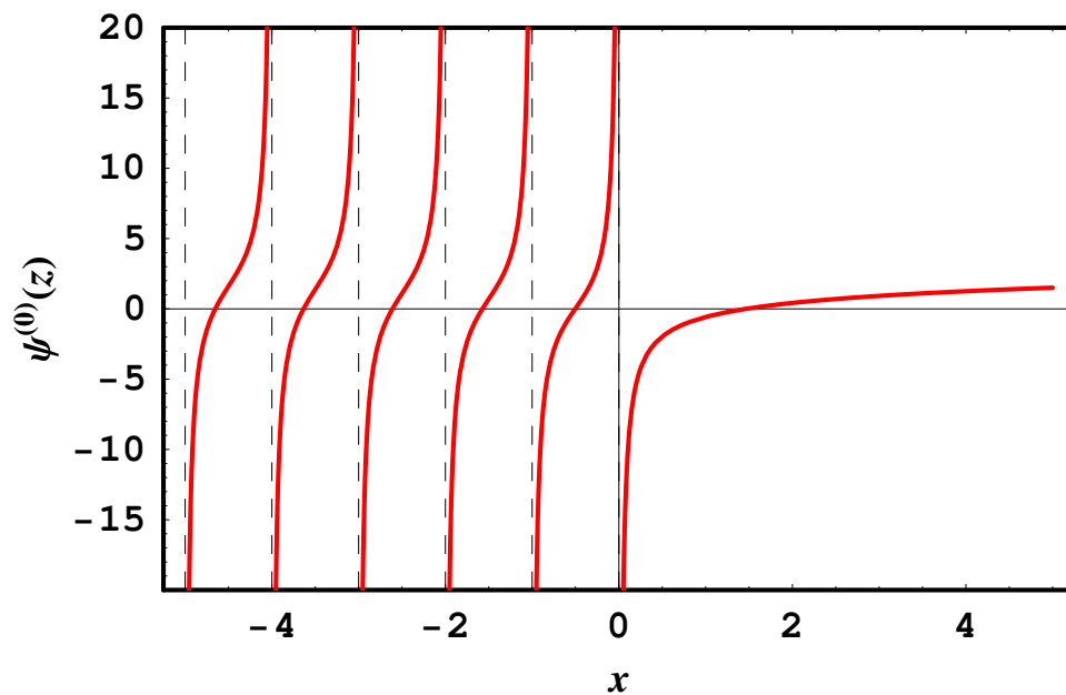
FIG. C-1: Fonction Digamma.
