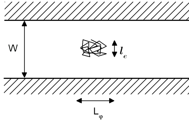
FIG. V.4: La trajectoire fermée typique des électrons contribue à la localisation faible dans le régime diffusif bidimensionnel l_e \ll L_\varphi \ll W \ll L .
