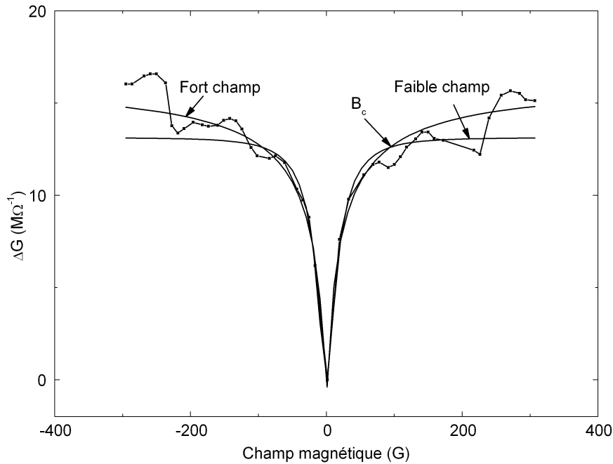
FIG. VI.11: La magnétoconductance des fils de largeur nominale L=620 nm à la tension de la grille V_g=0 V, à T=50 mK et les deux courbes ajustées par l'équation V.42 pour deux cas : faible champ magnétique et fort champ magnétique. La flèche indique le champ magnétique de "cross-over".
