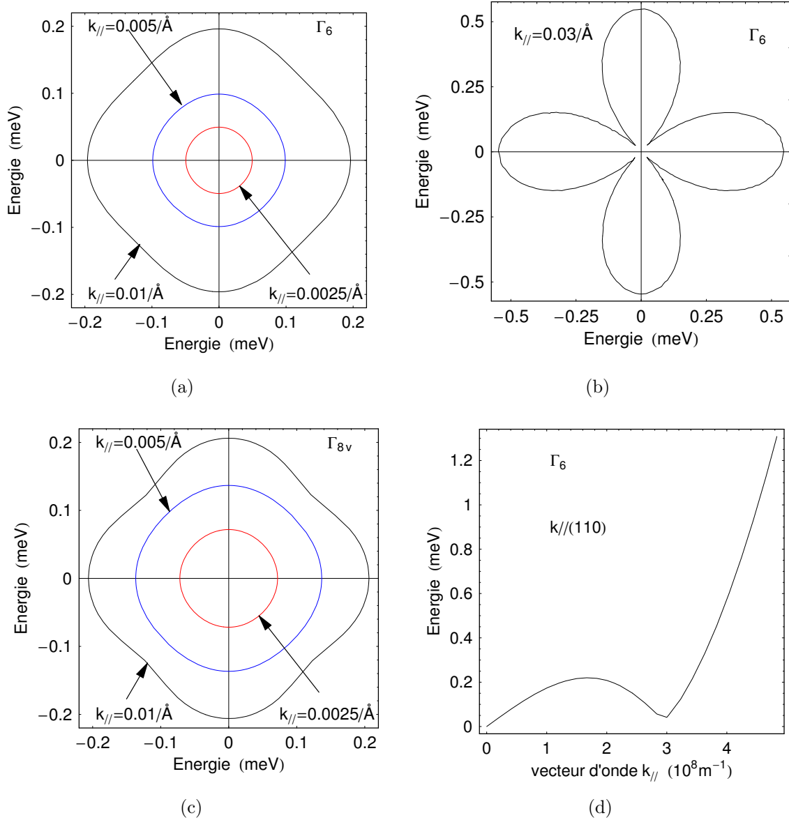
FIG. III.3: La variation angulaire du splitting de spin dans la bande de conduction pour un vecteur d'onde transverse k_{\perp} = 0.01 \text{ \AA}^{-1} (a); pour un vecteur d'onde k_{\perp} = 0.03 \text{ \AA}^{-1} (b) dans la bande de valence (c) du puits quantique Al 0.3 Ga 0.7 As/GaAs 100 Å de large; et la variation du splitting de spin en fonction du vecteur d'onde transverse k_{\perp} suivant la direction [110] ( \theta = \pi/4 ) (d). Le calcul est effectué sans tenir compte du terme d'interface.
