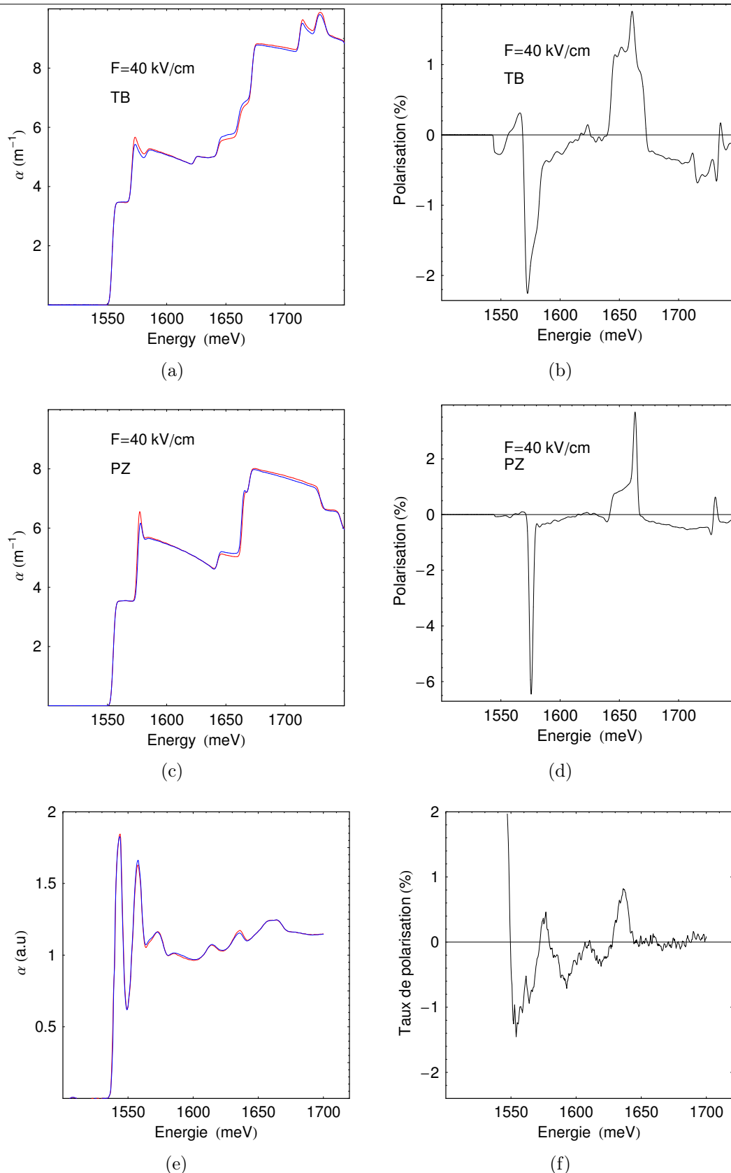
FIG. III.6: Absorption et taux de polarisation d'un puits quantique GaAs/ \text{Al}_{0.3}\text{Ga}_{0.7}\text{As} 100 Å de large sous 40 kV/cm, calculées en utilisant l'ensemble des paramètres TB (figures a et b), l'ensemble des paramètres PZ (figures c et d) et les mesures en photocourant (figures e et f) (d'après la thèse de Sébastien Cortez [11]). Les courbes rouges et bleues correspondent respectivement aux directions [110] et [1-10].
