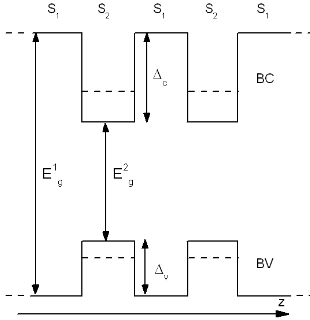
FIG. I.3: Profil de bande pour un multipuits quantique (ou super-réseau). Les niveaux d'énergies des états d'électron et de trous sont indiqués par les traits pointillés. Les notations \Delta_c et \Delta_v représentent l'offset de conduction et l'offset de valence.
