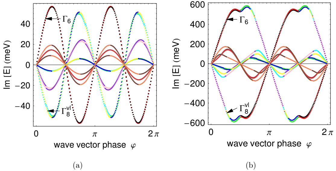
FIG. II.4: La partie imaginaire de l'énergie propre de toutes les bandes en fonction de la phase \varphi du vecteur d'onde \mathbf{k} , pour |\mathbf{k}|=0.02 ( 2\pi/a ) (a) et pour un vecteur plus grand |\mathbf{k}|=0.06 ( 2\pi/a ) (b). La figure II.4(b) montre la disparition de l'intersection près de \pi/2 (ou 3\pi/2 ) entre deux courbes rouge et noir correspondant à la bande de conduction \Gamma_{6c} et l'axe Ox.
