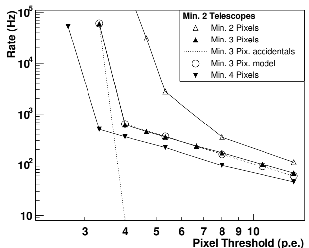
FIG. 6.4: Taux de déclenchement en fonction du seuil individuel par pixel pour différentes conditions de seuils par secteur. La courbe pointillée correspond au déclenchement fortuit attendu par le bruit de fond de ciel. Les ronds vides correspondent aux simulations du taux de déclenchement pour cette configuration. Cette figure est tirée de la référence [33].
