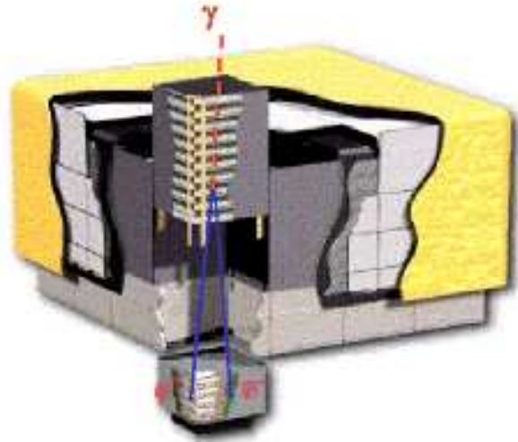
FIG. 2.7: Vue en coupe de GLAST.
