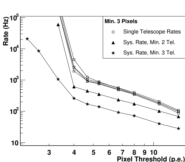
FIG. 6.3: Taux de déclenchement en fonction du seuil par pixel (déclenchement sur 3 pixels) pour plusieurs multiplicités de télescopes. Les 4 courbes du haut (carrés vides) montrent le taux pour chaque télescope individuel. Cette figure est tirée de la référence [33].
