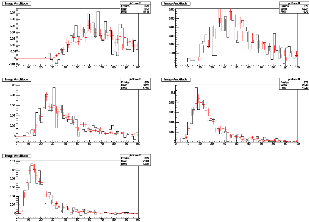
FIG. 10.9: Distribution en intensité (échelle arbitraire) des 5 pixels les plus brillants pour des simulations gamma suivant une loi de puissance d'indice spectral -2,6 à 46^\circ (points rouge) et pour les événements gamma observés sur la Nébuleuse du Crabe.
