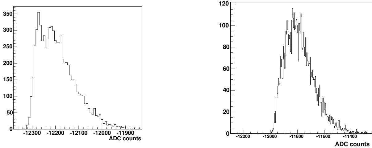
FIG. 8.3: gauche Spectre obtenu après nettoyage dans une région sombre du ciel (M 87). droite Spectre obtenu dans une région brillante du ciel (SN 1006).
