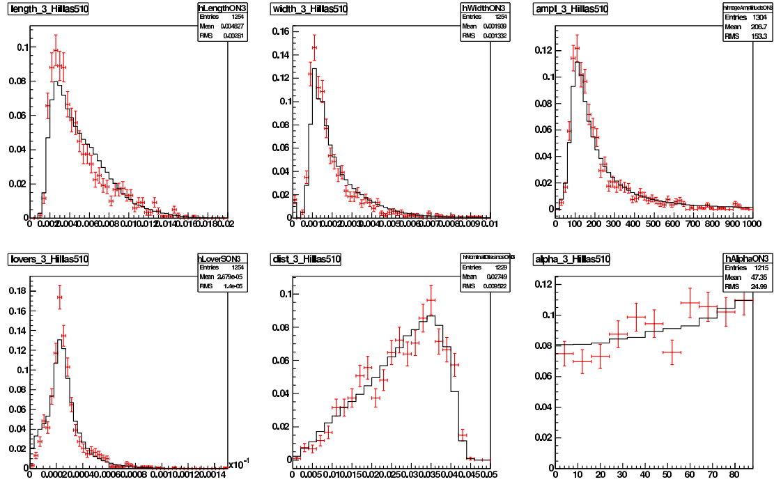
FIG. 10.8: Distributions des paramètres de Hilla (échelle arbitraire) pour des simulations de hadrons (points rouge) et des données réelles (trait noir). De gauche à droite et de haut en bas : longueur, largeur, amplitude d'image, LoverS, distance nominale et paramètre \alpha .
