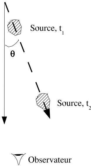
FIG. 11.2: Géométrie pouvant expliquer un mouvement apparent superluminique.
