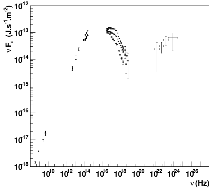
FIG. 12.1: Distribution spectrale en énergie de PKS 2155-304. Les données dans le domaine des X correspondent à plusieurs états enregistrés par les satellites Beppo-SAX et RXTE. Les points à plus basses énergies sont tirés de la base de données extragalactiques NED [109].
