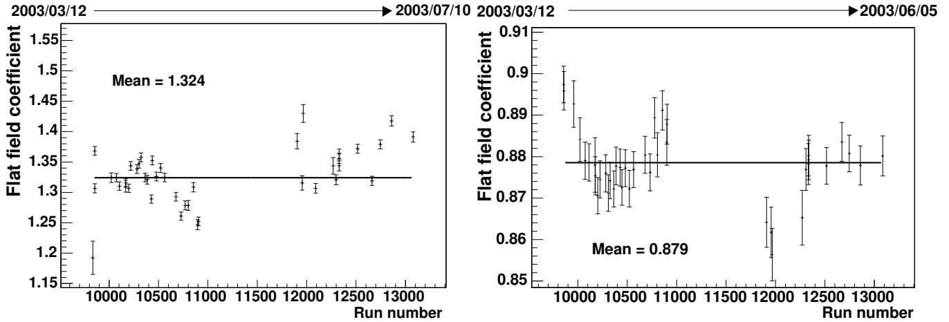
FIG. 8.26: Evolution des coefficients de correction d'inhomogénéité pour deux PMS sur 4 mois.
