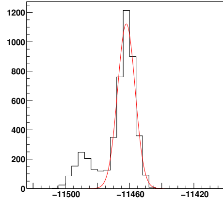
FIG. 8.12: Piédestal pour ARS non verrouillé.
