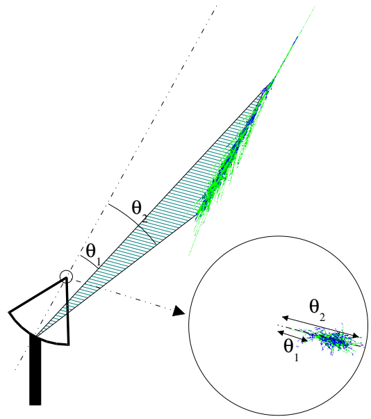
FIG. 2.10: Principe d'un imageur à effet Tcherenkov, comme H.E.S.S. Cette figure est tirée de [11].
