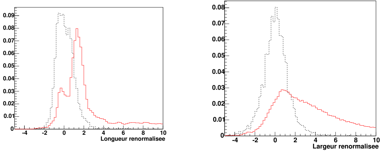
FIG. 10.11: Distribution des paramètres de longueurs et de largeurs d'images renormalisées. Le trait pointillé noir correspond à une simulation de photons gamma et le trait continu rouge à une acquisition sur une région de contrôle hors source (hadrons).
