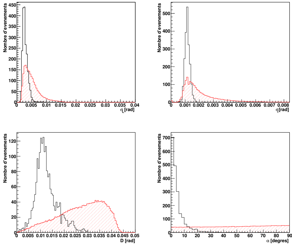
FIG. 10.4: Distributions des paramètres de Hillas pour des simulations \gamma (histogrammes grisés) et pour des données réelles à un même angle zénithal en mode mono-télescope.
