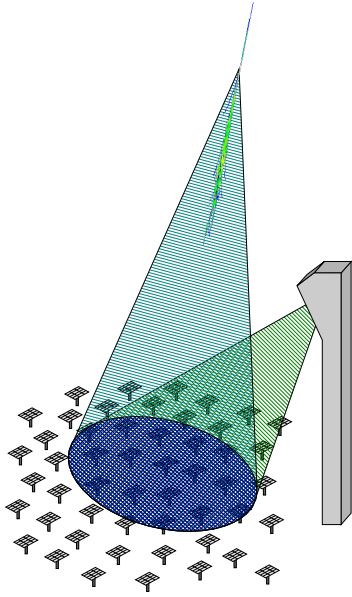
FIG. 2.9: Principe d'un échantillonneur Tcherenkov, comme CELESTE. Cette figure est tirée de [11].
