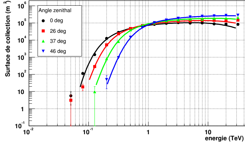
FIG. 12.5: Surfaces de collection pour la stéréoscopie en déclenchement monotélescope (stéréo soft).
