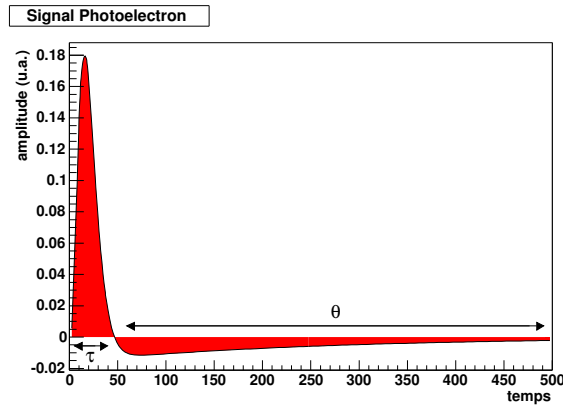
FIG. 8.2: Amplitude du signal d'un photoélectron ( \times -1 ) au cours du temps. La contribution négative correspond au rebond du circuit RC. Cette figure n'est pas à l'échelle.
