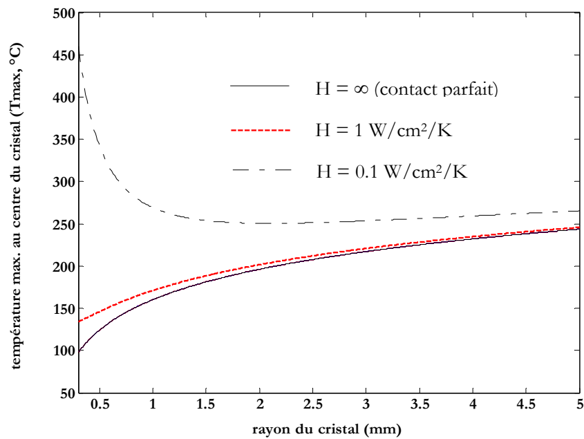
Figure I.2.7 : Température maximale au centre du cristal T(r=0, z=0) en fonction du rayon r_0 du cristal. Pour simplifier, le calcul est effectué avec l'hypothèse qu'il n'y a pas de saturation de l'absorption, et la divergence de la pompe est négligée. D'autre part : T_c=15^\circ\text{C} , \eta_h=6.5 \% , \alpha_{NS}=7.4 \text{ cm}^{-1} , K_c=2.1 \text{ W/m/K} (valeurs du GdCOB), P_{inc}=15 \text{ W} , w_p=100 \text{ }\mu\text{m} .
