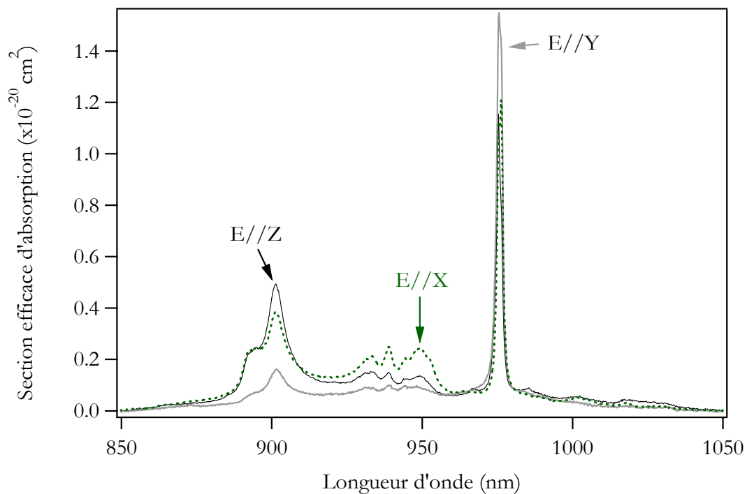
Figure III.2.1 : Spectre d'absorption en lumière polarisée de l' \text{Yb:GdCOB} . X, Y, Z sont les axes cristallographiques. E désigne le champ électrique de l'onde. D'après [Mongel 99].
