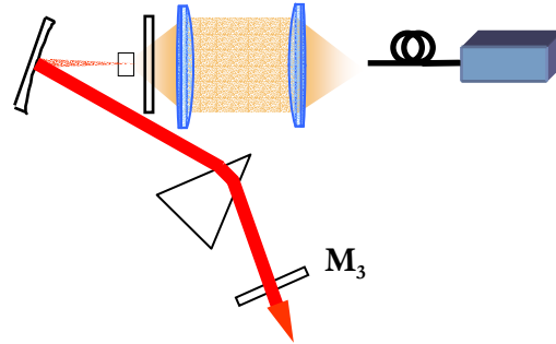
Figure II.2.4 : schéma d'une cavité avec prisme (voir aussi figure II.1.2)
