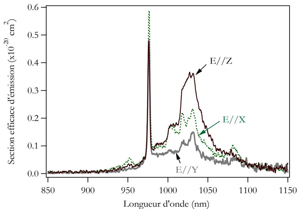
Figure III.2.2 : Spectres d'émission en lumière polarisée de l' \text{Yb:GdCOB} . D'après [Mongel 99].
