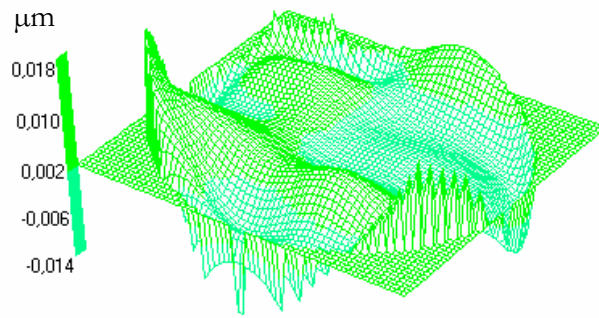
Figure III.5.1 : Evaluation de l'exactitude de mesure de la phase : l'écart-type est de 0,004 \mu\text{m} ( \approx \lambda/150 ) sur l'étendue de la pupille (diamètre : 2,3 \text{ mm} ). L'écart « pic-vallée » du front d'onde est de 0,032 \mu\text{m} ( \lambda/20 ). Ici le front d'onde est obtenu par moyennage de 10 acquisitions.
