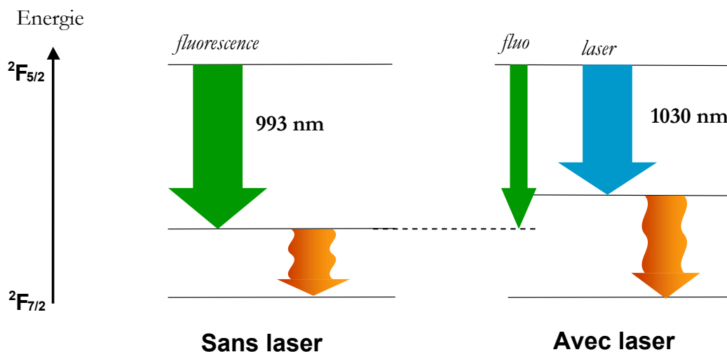
Fig. IV.3.8 : illustration (simplifiée) du comportement observé dans le KGW : en supposant les désexcitations non radiatives négligeables ( \eta_r = 1 ) la lentille thermique plus forte en présence d'effet laser peut être attribuée à une longueur d'onde moyenne de fluorescence très basse (993 nm). Lorsque le laser fonctionne (à 1030 nm), le défaut quantique devient plus grand, et par conséquent la charge thermique aussi.
