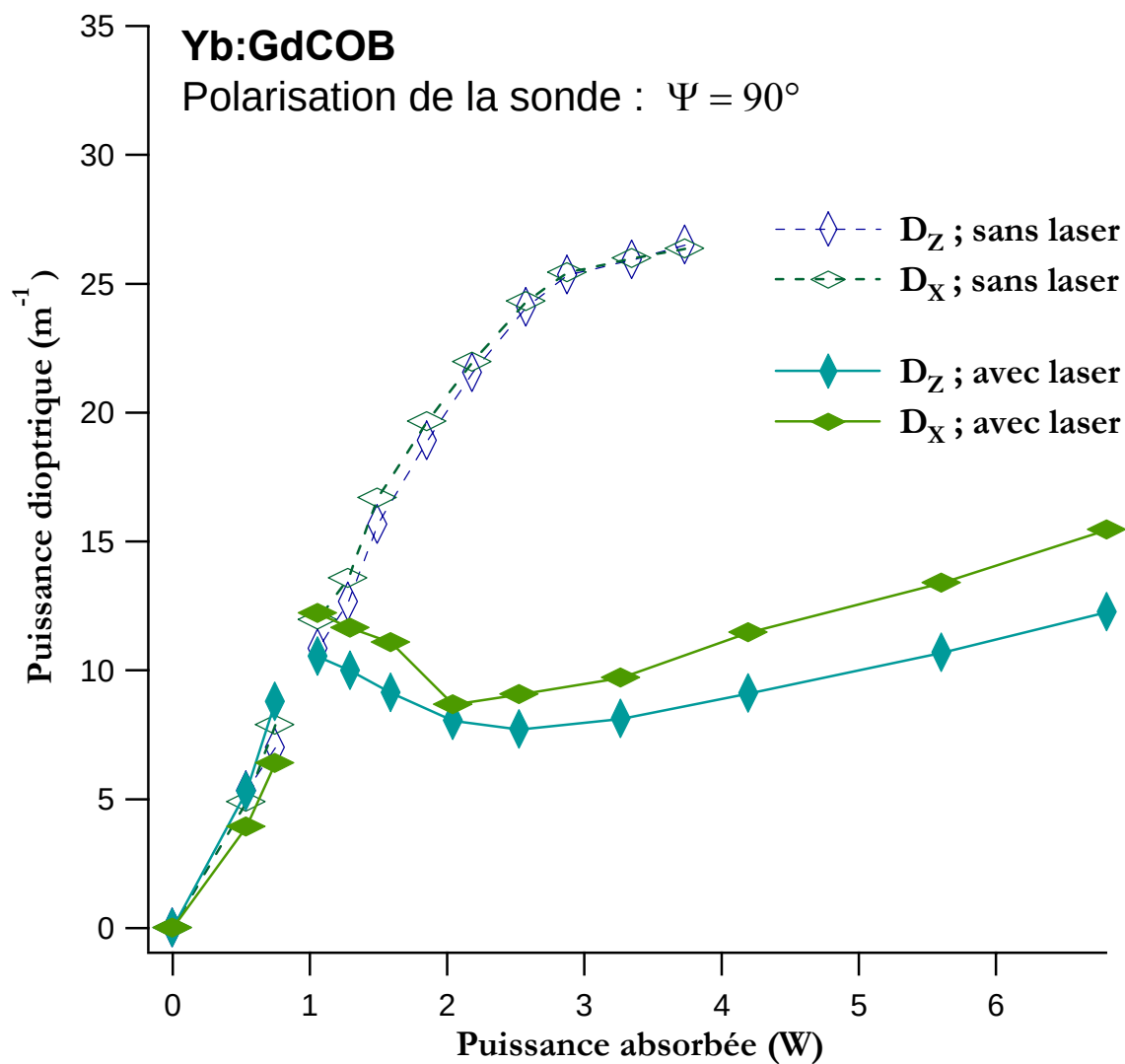
Figure IV.7.5 : puissance dioptrique mesurée avec et sans effet laser avec un faisceau de sonde polarisé parallèlement à l'axe cristallophysique X ( \Psi = 90^\circ ).
