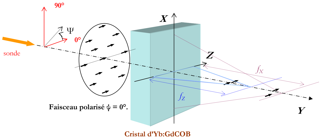
Figure IV.7.1 : position des axes cristallographiques (X, Y, Z) du cristal (biaxe) de GdCOB : le faisceau laser est naturellement polarisé selon Z. La direction de polarisation de la sonde est définie par l'angle \Psi . Quand \Psi=0^\circ la polarisation est parallèle à l'axe Z. On a également représenté la signification des focales f_Z et f_X (dans le texte on se référera à leurs inverses, D_Z et D_X respectivement), ici avec un faisceau polarisé \Psi=0^\circ .
