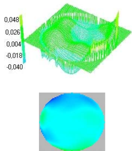
Figure IV.2.1 : Fronts d'onde enregistrés avec un cristal d' \text{Yb:YAG} . À gauche : la zone sondée est plus grande que la zone pompée (diamètre de pompe : 200 \mu\text{m} ; diamètre de sonde à 1/e^2 : 320 \mu\text{m} ). Sur une pupille d'analyse de 3.38 mm de diamètre, les coefficients d'aberration non négligeables sont : C_3 = -0.118 \mu\text{m} et C_8 = +0.046 \mu\text{m} . À droite : la zone sondée et la zone pompée ont des tailles comparables (diamètre de sonde à 1/e^2 : 220 \mu\text{m} ). Sur une pupille d'analyse de 2.3 mm de diamètre, le seul coefficient non négligeable est la courbure : C_3 = -0.085 \mu\text{m} ( C_8 = +0.001 \mu\text{m} ).
