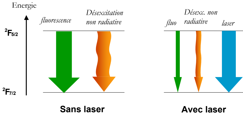
Fig. IV.3.7 : illustration du comportement observé dans le GdCOB, l'YCOB, l'YSO, le YAG et le GGG : les effets non radiatifs sont mis en évidence par une diminution du débit qui leur est associé lorsque l'oscillation laser a lieu. Le débit d'émission stimulée « court-circuite » alors la fluorescence et les effets non radiatifs.
