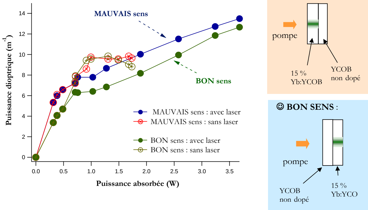
Figure IV.8.3 : influence du sens d'utilisation du matériau composite sur la puissance de la lentille thermique.
