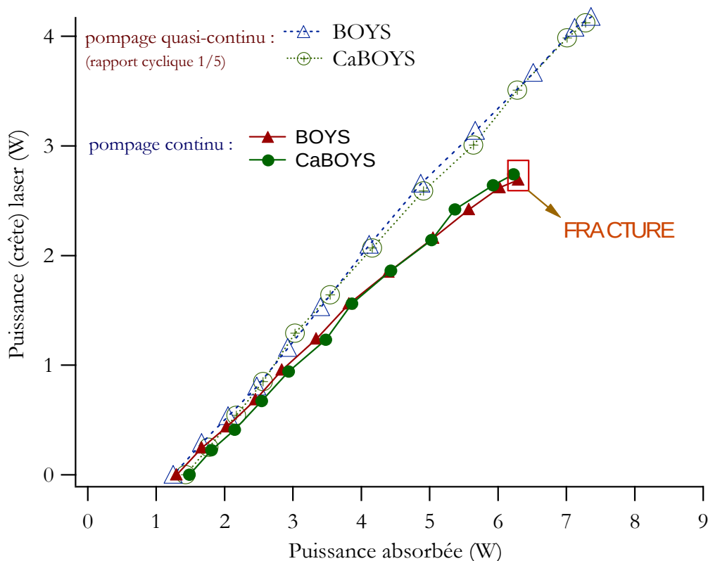
Figure III.3.11 : Comparaison des performances de l'Yb:CaBOYS (dopé 15 at.% Yb, e = 2.51 mm, \kappa//c ) et de l'Yb:BOYS (dopé 20 at.% Yb, e = 2.38 mm, \kappa//c ) en pompage par diode LIMO (12.5 W incidents à 975 nm).
