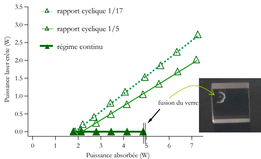
Figure III.3.8 : Performances comparées de l'Yb:BOYS, Yb:GdCOB et Yb:verre en régime quasi-continu (rapport cyclique 1/17 et 1/5) et continu.
