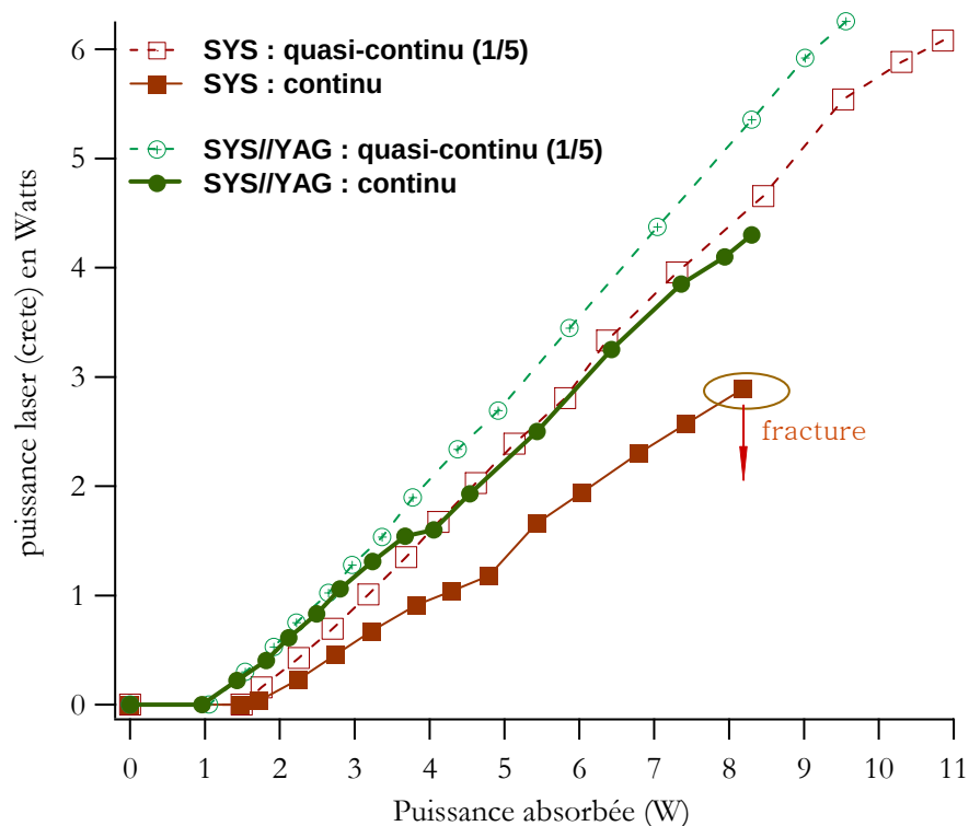
Figure III.4.3. : performances du cristal composite Yb:SYS//YAG ; comparaison avec le cristal d'Yb:SYS simple (fig. III.4.2).
