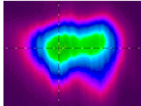
Figure III.3.5 : Profil du faisceau de pompe (diode Optopower sans sa fibre) au niveau du cristal.
