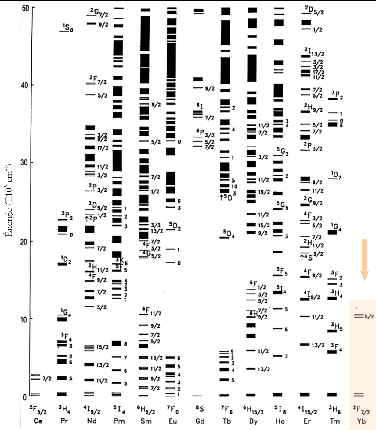
Niveaux d'énergie des ions lanthanide trivalents (ici dans les chlorures), d'après [Handbook of lasers].
