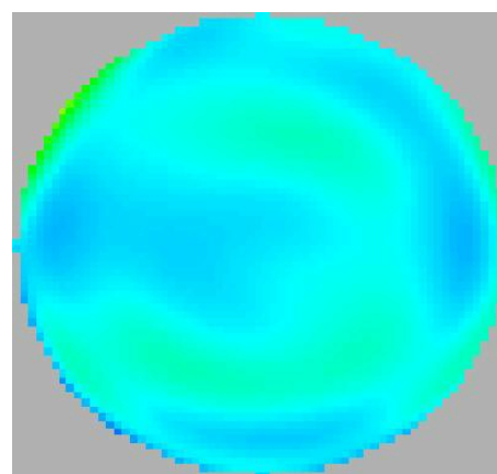
Front d'onde résidu obtenu après soustraction de la courbure (écart-type : 0.010 \mu m )
