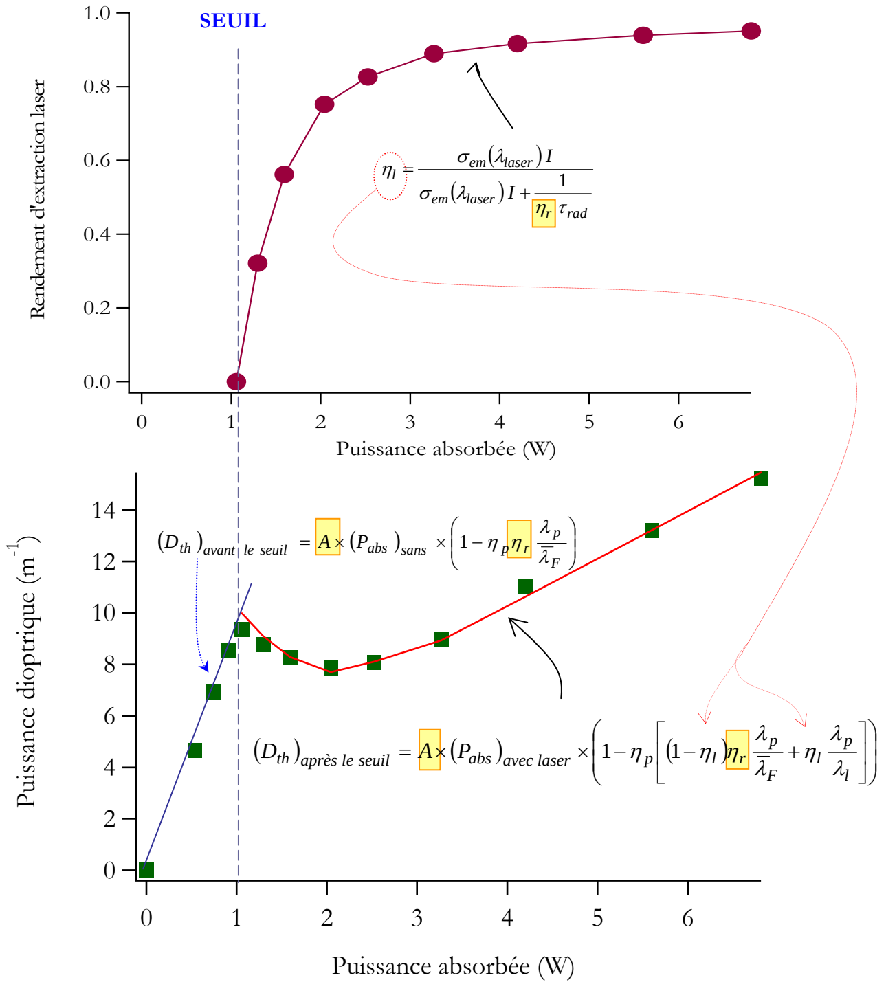
Figure IV.3.9 : illustration de la démarche adoptée pour déduire le rendement quantique de fluorescence, dans le cas de l'Yb:GdCOB. En haut : le rendement d'extraction laser \eta_l est tracé en fonction de la puissance absorbée : il est calculé à partir de l'intensité I , donc de la puissance laser expérimentale (éq. IV.3.4). Il s'exprime aussi en fonction du rendement quantique de fluorescence \eta_r . Cette expression est ensuite réinjectée (voir en bas ) dans l'expression complexe de (D_{th})_{avec\ laser} . On n'a donc plus que deux paramètres ajustables : A et \eta_r (surlignés) qui sont choisis pour que les courbes donnant (D_{th})_{après\ le\ seuil} et (D_{th})_{avant\ le\ seuil} (cette dernière étant une droite) correspondent au mieux aux points expérimentaux. La formule donnant (D_{th})_{avant\ le\ seuil} est simplement déduite de l'expression de (D_{th})_{après\ le\ seuil} mais avec \eta_l = 0 . Il n'y a aucun autre paramètre ajustable que A et \eta_r .
