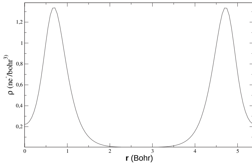
FIG. 5.2 – Densité des électrons de semi-cœur dans la phase \alpha du titane en DFT-LDA, quand ils sont traités explicitement dans la valence. La coupe de la densité est faite suivant \mathbf{a} le premier vecteur de base du réseau direct.
