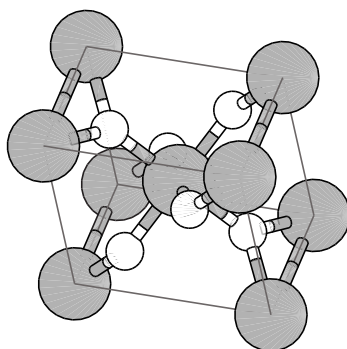
FIG. 2.3 – Structure de la phase rutile de \text{TiO}_2 . Grandes sphères : Ti. Petites sphères O.
