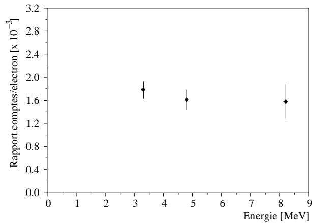
FIG. C.5: Rapport du nombre de comptes mesurés sur la caméra CCD et du nombre d'électrons contenus pour 3.0, 4.8 et 8.5 MeV. Les barres d'erreur tiennent compte des fluctuations statistiques du rapport à chaque énergie et de l'incertitude provenant de la méthode d'analyse.
