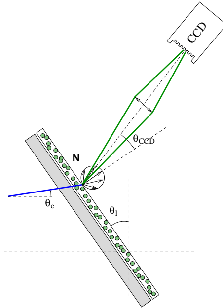
FIG. C.2: (Couleur) Scintillateur, système optique d'imagerie et paramètres associés.
