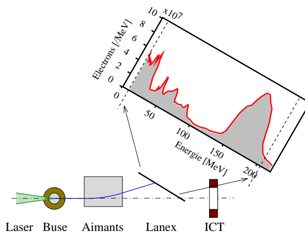
FIG. B.1: (Couleur) Dispositif expérimental pour la mesure du spectre des électrons.
