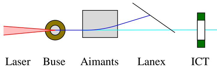
FIG. 2.1: (Couleur) Dispositif expérimental. Le laser est focalisé sur l'avant du jet de gaz. Les électrons accélérés lors de l'interaction sont déviés par le champ magnétique d'un aimant permanent et traversent ensuite un scintillateur. La lumière émise par la face arrière de ce scintillateur est collectée sur une caméra CCD. L'intégrateur de charge (ICT) sert à mesurer le nombre d'électrons qui le traversent.
