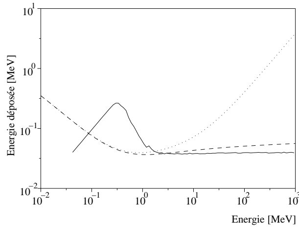
FIG. C.1: Dépôt d'énergie dans du Gadolinium Oxysulfide pur à partir : des tables de valeurs du pouvoir d'arrêt collisionnel (ICRU) (tirets), du pouvoir d'arrêt total (points) et des résultats de la simulation Monte-Carlo (ligne).
