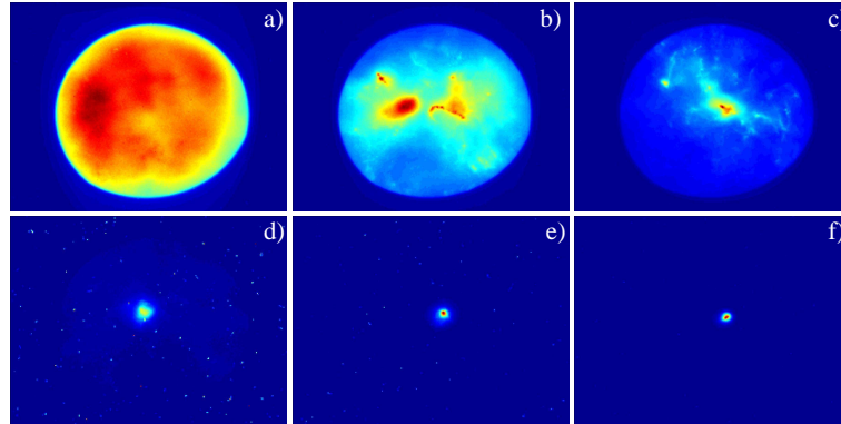
FIG. 2.3: (Couleur) Profil transverse du faisceau d'électrons en fonction de la densité électronique : a) n_e = 50 \times 10^{18} \text{cm}^{-3} ; b) 30 \times 10^{18} \text{cm}^{-3} ; c) 20 \times 10^{18} \text{cm}^{-3} ; d) 10 \times 10^{18} \text{cm}^{-3} ; e) 7.5 \times 10^{18} \text{cm}^{-3} ; f) 6.0 \times 10^{18} \text{cm}^{-3} .
