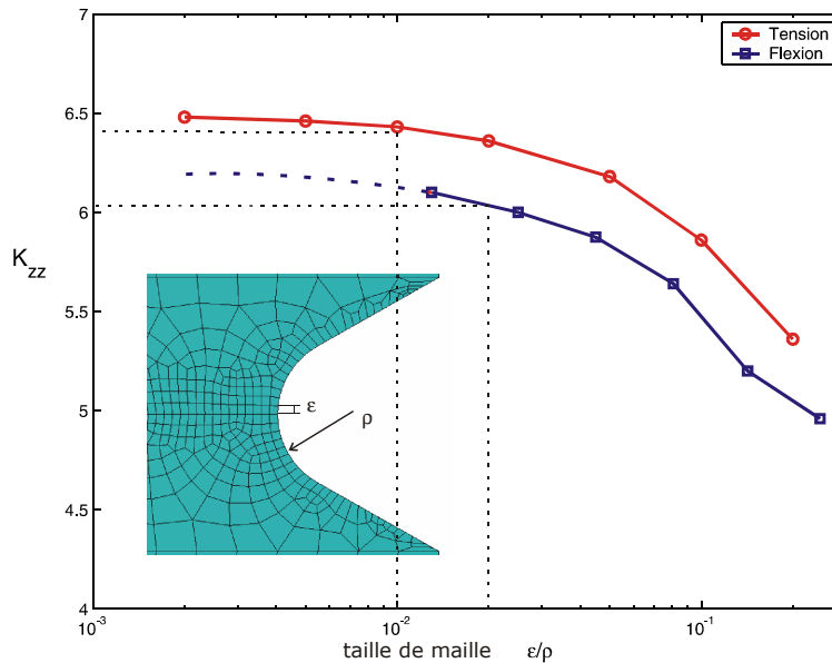
FIG. 2.8 – Analyse du maillage sur le facteur de concentration de contrainte axiale K_{ZZ} pour une entaille.
