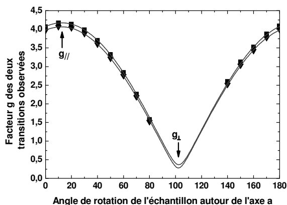
Fig. III-27 : Variation angulaire du facteur g dans le plan (100) pour le centre des deux transitions principales observées de l'ion \text{Ce}^{3+} . La courbe en trait plein est simulée par l'expression g = (g_{\perp}^2 \sin^2 \theta + g_{//}^2 \cos^2 \theta) .
