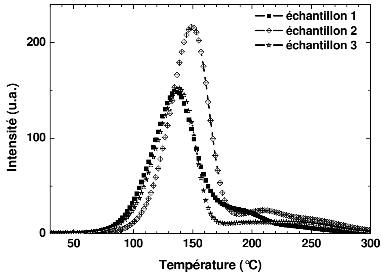
Fig. IV-40 : Courbes de thermoluminescence de trois échantillons de \text{LaCl}_3:\text{Ce}^{3+} entre 30 ^{\circ}\text{C} et 300 ^{\circ}\text{C} (vitesse de chauffage : 5 ^{\circ}\text{C}/\text{s} ; irradiation \beta^- : 512 mGy).
