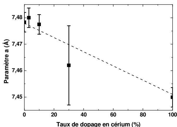
Fig. III-10 : Variation du paramètre a en fonction du taux de dopage dans \text{LaCl}_3:\text{Ce}^{3+} . La droite en pointillés indique la variation linéaire obtenue à partir des tables cristallographiques
