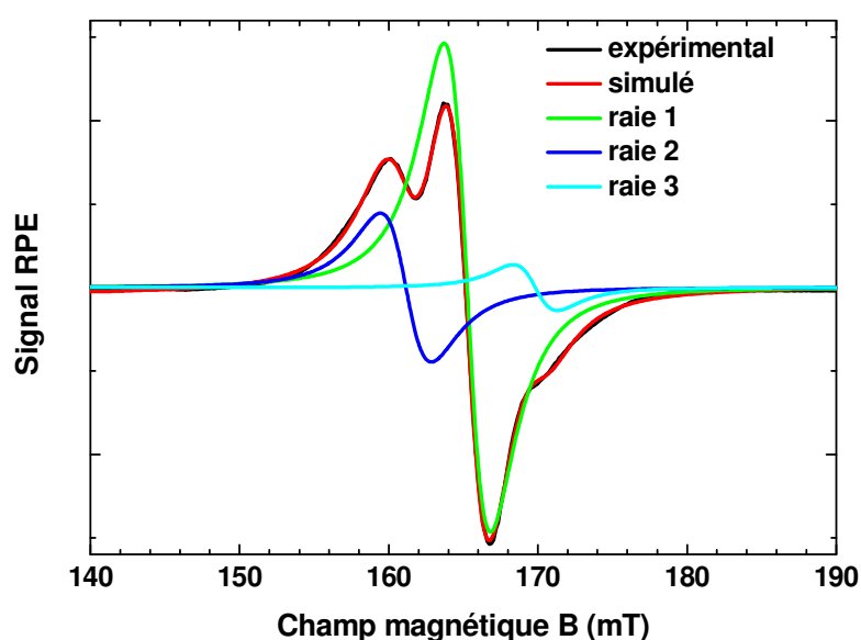
Fig. III-26 : Spectre RPE à 5 K de l'ion \text{Ce}^{3+} dans \text{LaBr}_3:\text{Ce}^{3+} tel que le champ magnétique \vec{B}_0 soit parallèle à l'axe c [001] et ajustement par trois raies dérivées de lorentziennes.
