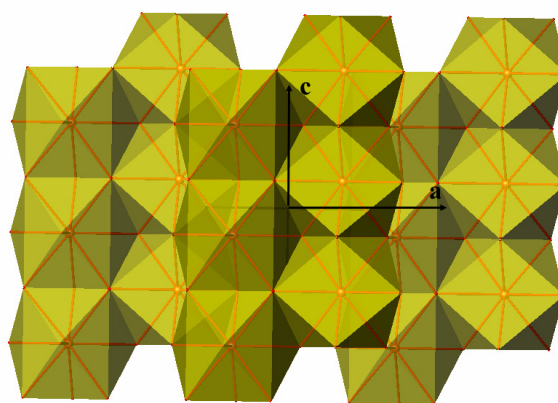
Fig. III-7 : Projection selon le plan (010) de la structure \text{UCl}_3 mettant en évidence l'enchaînement de liaisons anion-cation.
