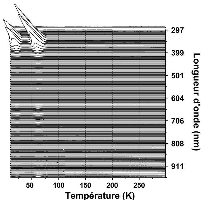
Fig. IV-18 : Courbe de thermoluminescence résolue en longueur d'onde de \text{LaCl}_3:\text{Ce}^{3+} (vitesse de chauffage : 0,1 K/s)
