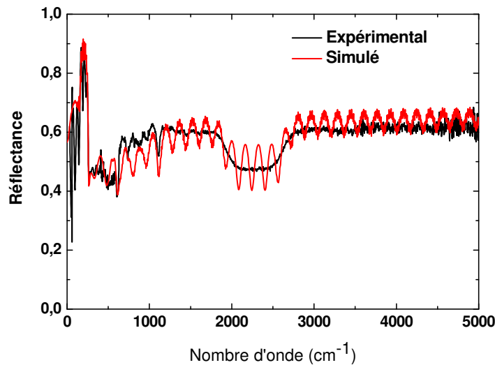
Fig. III-37 : spectres de réflectance expérimental et simulé du système multicouche à base de \text{LaCl}_3:\text{Ce}^{3+}
