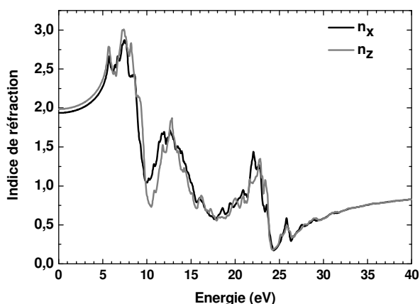
Fig. III-42 : indice de réfraction de LaBr 3 :Ce 3+ obtenu par simulation quantique (composantes axiales n_x et n_z selon les axes a et c respectivement)
