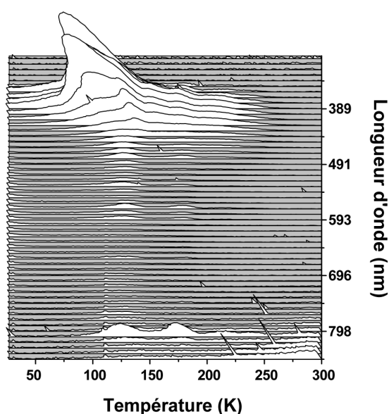
Fig. IV-19 : Courbe de thermoluminescence résolue en longueur d'onde de \text{LaBr}_3:\text{Ce}^{3+} (vitesse de chauffage : 0,1 K/s)
