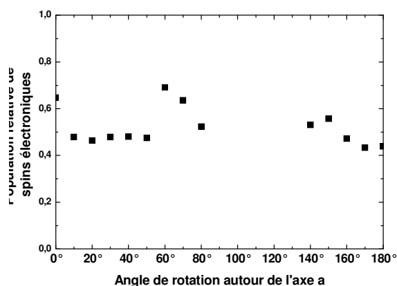
Fig. III-28 : Variation angulaire de la population de spins électronique mesurée pour la transition à champ le plus bas de l'ion \text{Ce}^{3+} (valeur relative, proportionnelle à la population réelle)
