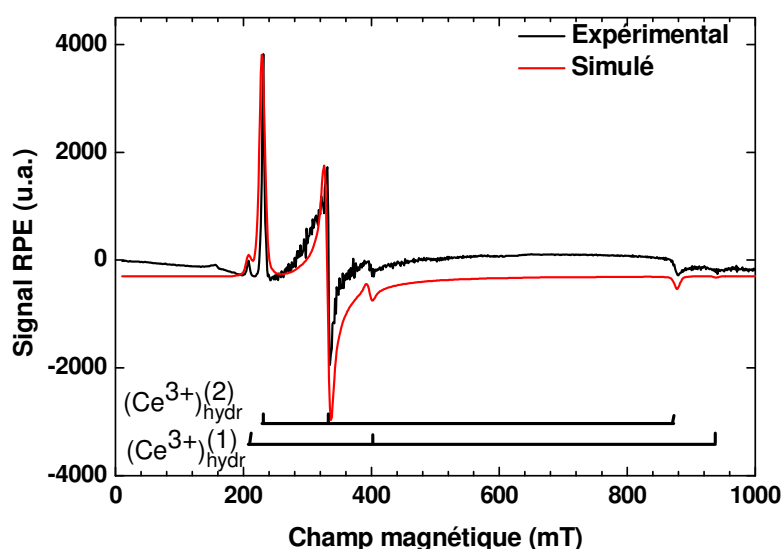
Fig. III-25 : simulation des transitions RPE dues des ions \text{Ce}^{3+} dans des couches hydratées amorphes
