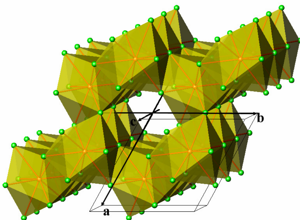
Fig. III-1 : Structure de \text{LaX}_3 ( \text{X} = \text{Cl} ou \text{Br} ) avec indication de la maille primitive
