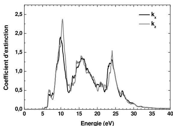
Fig. III-41 : coefficient d'extinction de LaCl 3 :Ce 3+ obtenu par simulation quantique (composantes axiales n x et n z selon les axes a et c respectivement)
