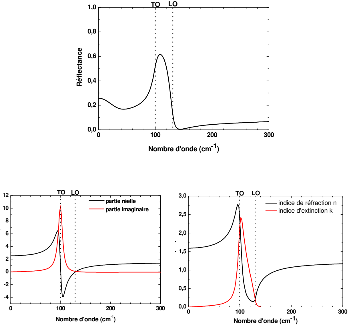
Fig. III-31 : Exemple de spectre de réflectance infrarouge d'un cristal dipolaire et fonctions optiques qui en découlent : fonction diélectrique \tilde{\epsilon}_{\sigma} , indices optiques n_{\sigma} et k_{\sigma} . Les nombres d'onde des modes TO et LO ont été précisés.
