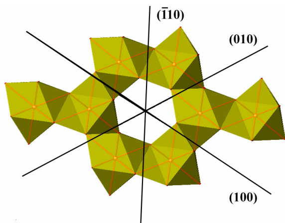
Fig. III-6 : Mise en évidence des plans de clivage dans la structure \text{UCl}_3 (projection selon le plan (001) )
