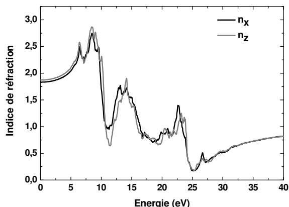
Fig. III-41 : indice de réfraction de LaCl 3 :Ce 3+ obtenu par simulation quantique (composantes axiales n_x et n_z selon les axes a et c respectivement)
