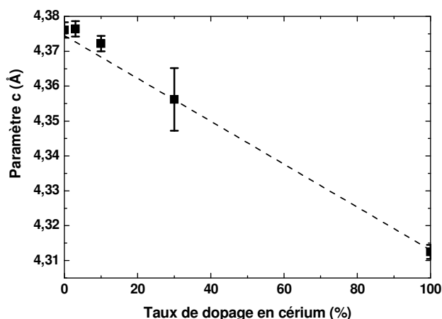
Fig. III-11 : Variation du paramètre c en fonction du taux de dopage dans \text{LaCl}_3:\text{Ce}^{3+} . La droite en pointillés indique la variation linéaire obtenue à partir des tables cristallographiques
