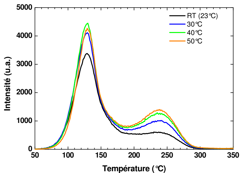
Fig. IV-53 : courbes de thermoluminescence de \text{LaCl}_3:\text{Ce}^{3+} après irradiation de 64 mGy suivie d'une pause de 350 s à température donnée
