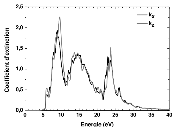
Fig. III-42 : coefficient d'extinction de LaBr 3 :Ce 3+ obtenu par simulation quantique (composantes axiales n x et n z selon les axes a et c respectivement)
