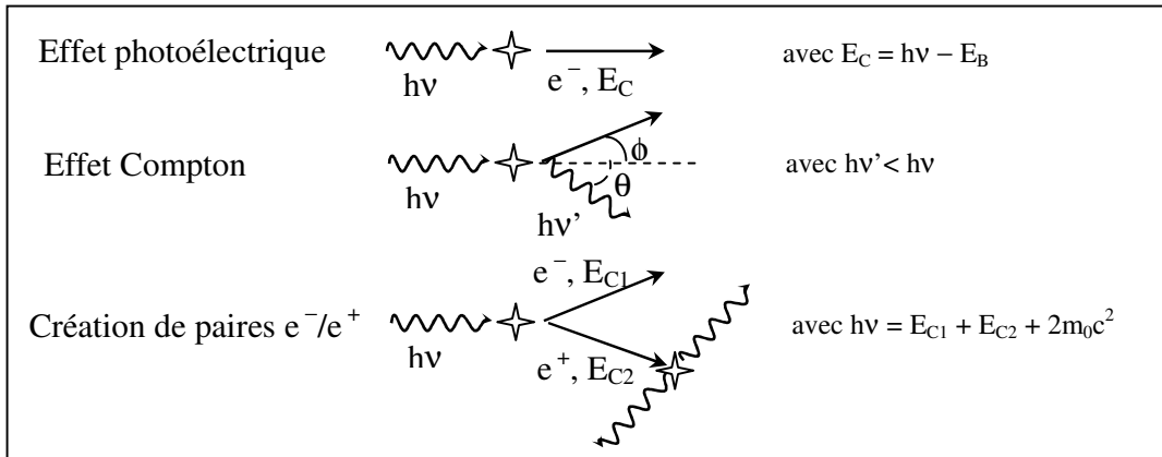
Fig. I-7 : principes des différentes interactions entre rayonnement et matière
