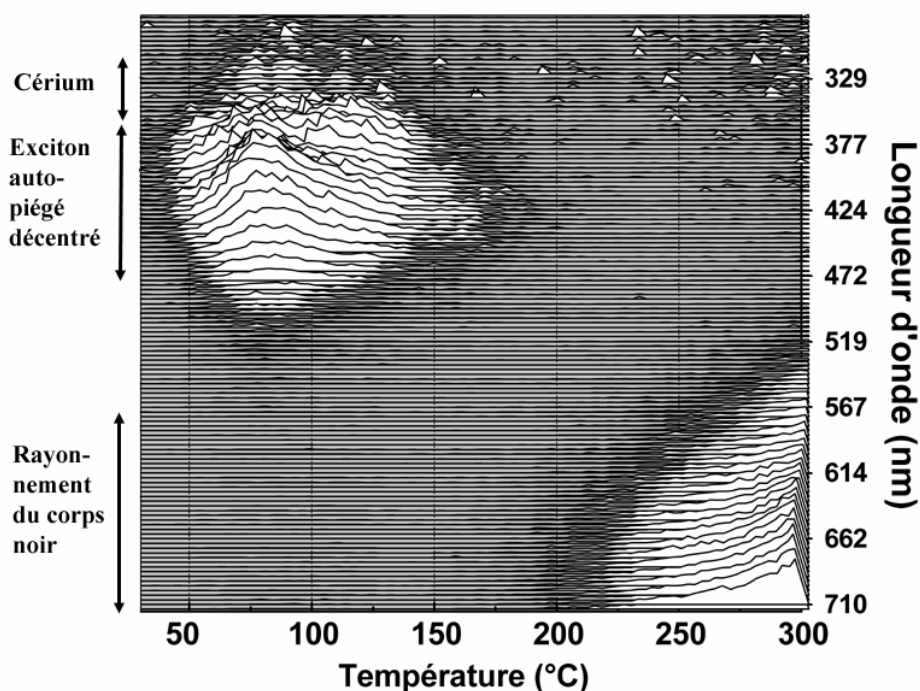
Fig. IV-33 : Courbe de thermoluminescence résolue en longueur d'onde de \text{LaCl}_3:\text{Ce}^{3+} (vitesse de chauffage : 3°C/s)
