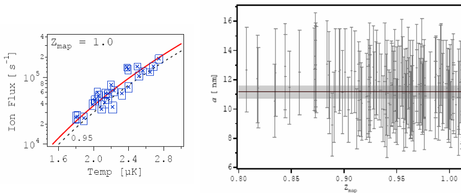
FIG. 3 – a) Signal d'ion en fonction de la température pour des nuages à T = T_c . b) les résultats finaux pour l'analyse des la détermination de la longueur de diffusion de l' \text{He}^* .
