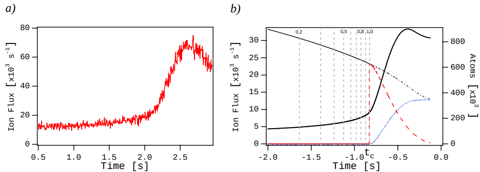
FIG. 1 – Le signal d'ion : a) signal real et b) signal simulé.
