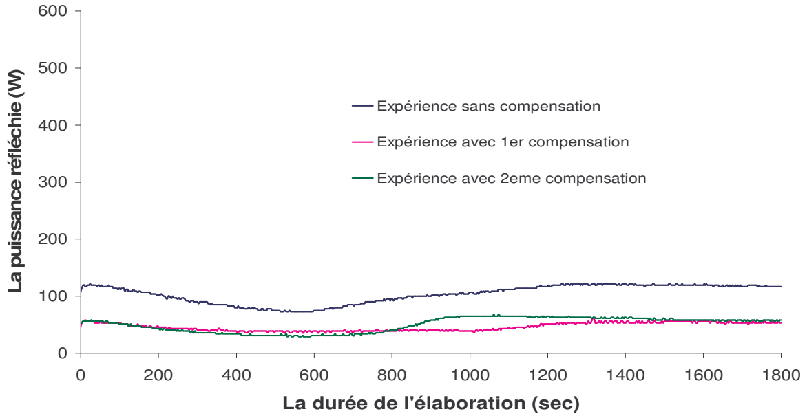
Figure III.28 : Puissances réfléchies
