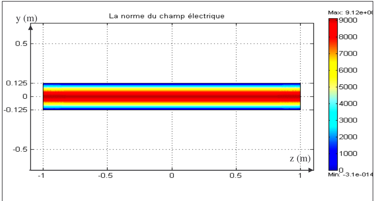
Figure II.3: Profil en 2D de la norme du champ électrique dans un guide très long
