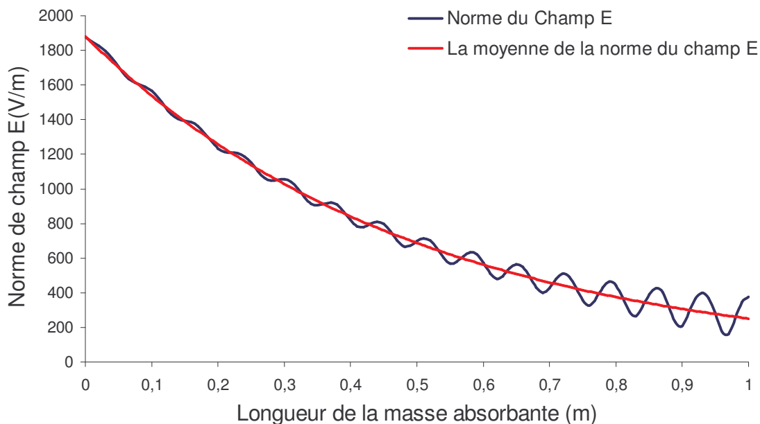
Figure II.12 : Profil de la norme du champ électrique à mi-hauteur et entre les deux limites de la masse absorbante (-0,5 et +0,5) de la figure II.11.
