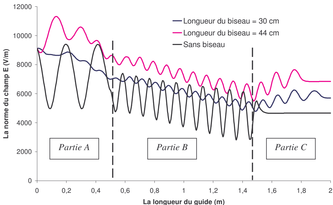
Figure II.18: Profil de la norme du champ électrique à mi-hauteur d'un guide rempli par trois diélectriques, sans et avec adaptation
