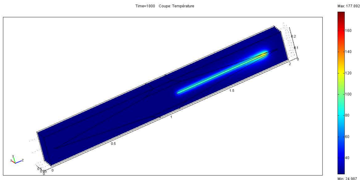
Figure IV.14 : Le champ de la température à 1800sec dans une éprouvette de 15mm et son environnement pour un chauffage uniforme
