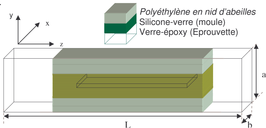
Figure II.1 : Applicateur rempli par trois diélectriques
