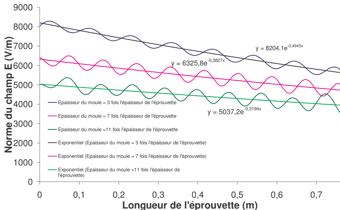
Figure A.II.10: L'évolution de la norme du champ électrique dans une éprouvette de 15 mm en fonction de l'épaisseur du moule, ainsi l'atténuation associée à chaque cas.
