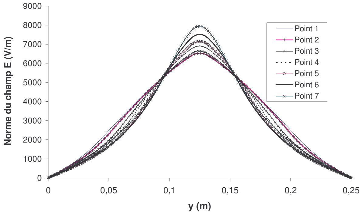
Figure II.35 : Le profil longitudinal de la norme du champ électrique aux abscisses z où le champ passe par des maxima
