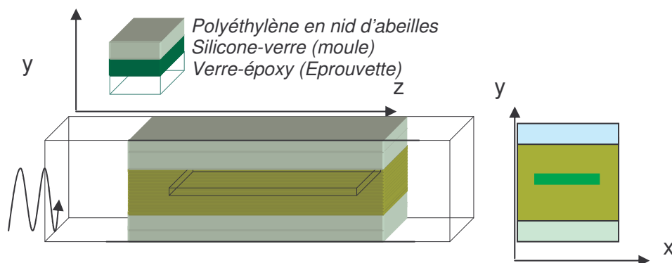
Figure III.1 : Modèle expérimental d'un applicateur rempli par trois diélectriques
