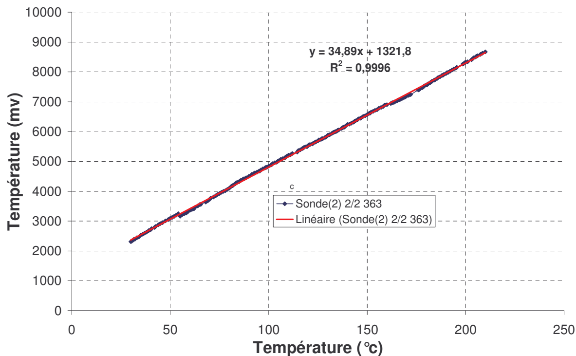
Figure B.2 : La courbe d'étalonnage de la sonde 2
