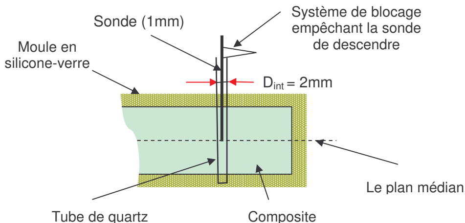
Figure III.9 : Dispositif permettant de positionner les sondes
