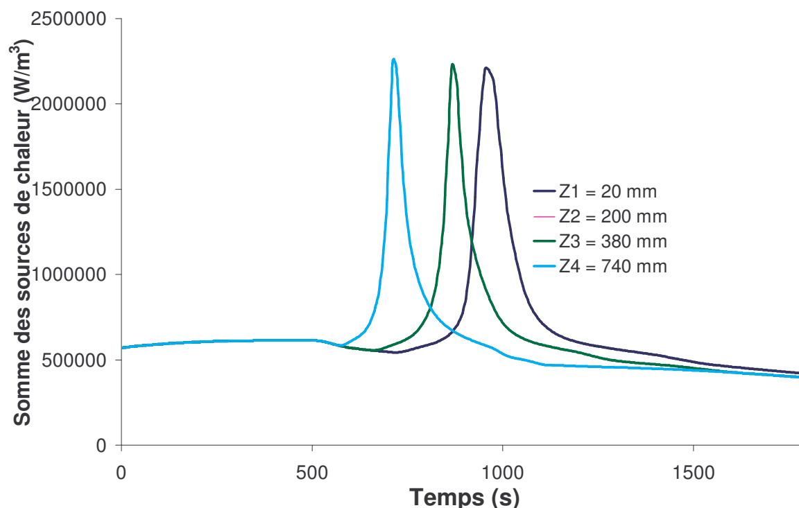
Figure IV.22 : Evolutions des sources de chaleur d'origines chimique et électromagnétique en fonction du temps
