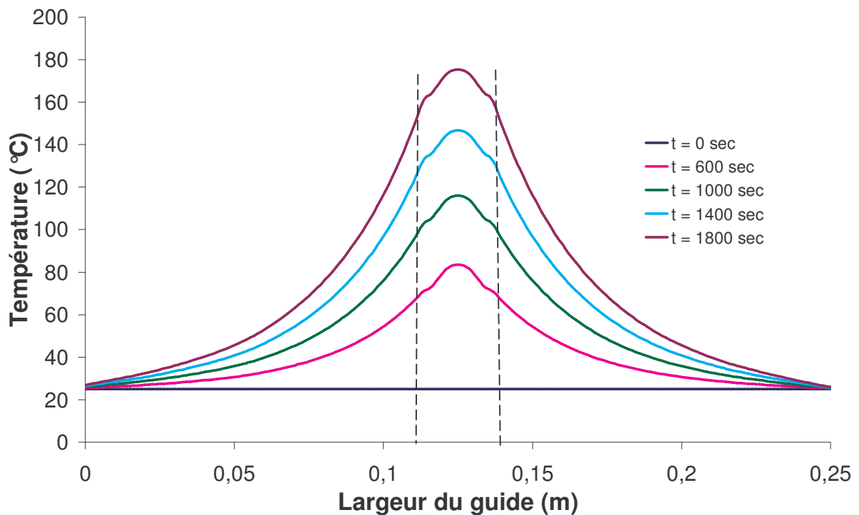
Figure IV.16 : La température transversale du composite au point z_4 = 0.74 m en fonction du temps
