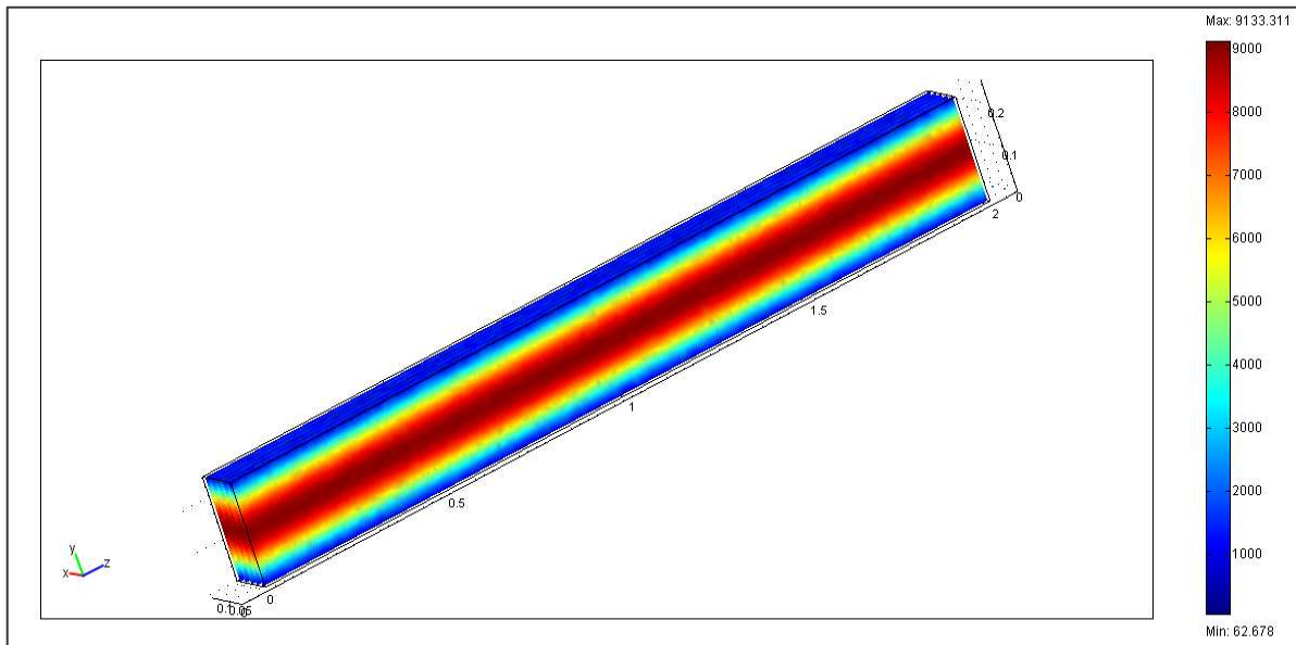
Figure II.4 : Profil en 3D de la norme du champ électrique dans un guide très long
