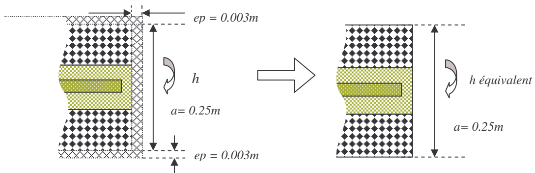
Figure IV.12 : Parois du guide et coefficient d'échange équivalent
