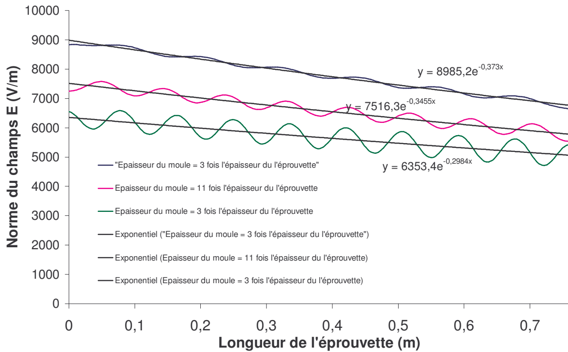
Figure A.II.9: L'évolution de la norme du champ électrique dans une éprouvette de 10 mm en fonction de l'épaisseur du moule, ainsi l'atténuation associée à chaque cas.
