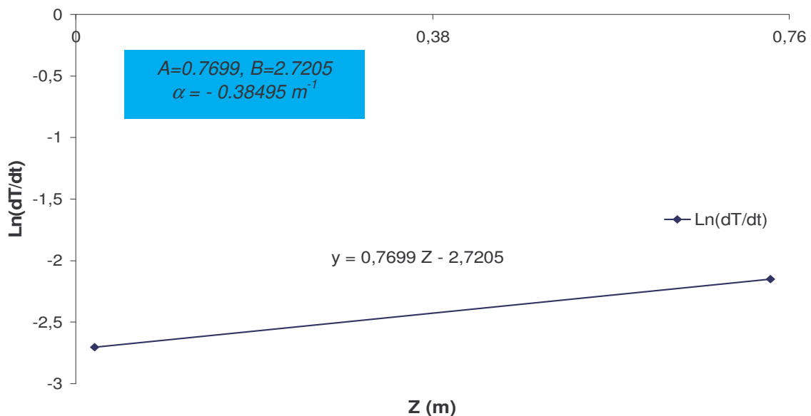
Figure III.27 : L'atténuation entre le point z_1= 0,02 \text{ m} et z_4=0,74\text{m} dans le cas d'un moule avec compensation de l'atténuation (résultat de la figure III.23)
