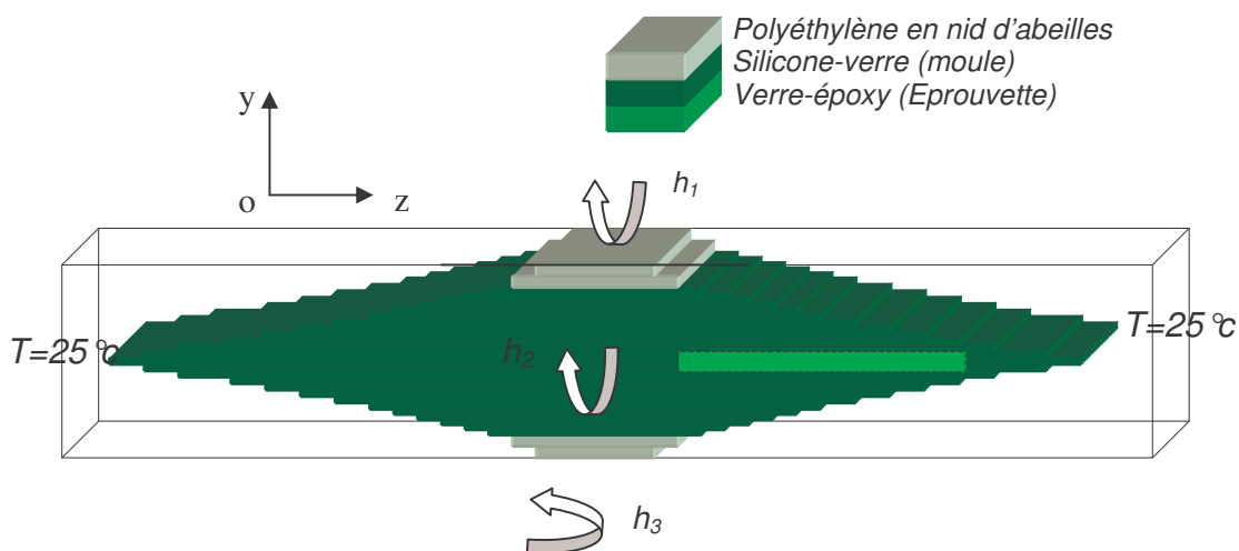
Figure IV.13 : Schéma du montage et les conditions aux limites appliquées
