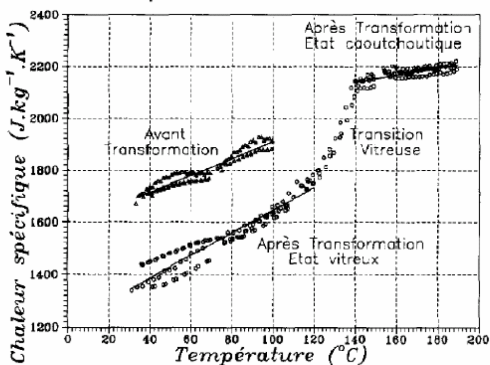
Figure IV.11 : L'évolution de la chaleur spécifique en fonction de la température d'une matrice époxydique [IV.29]
