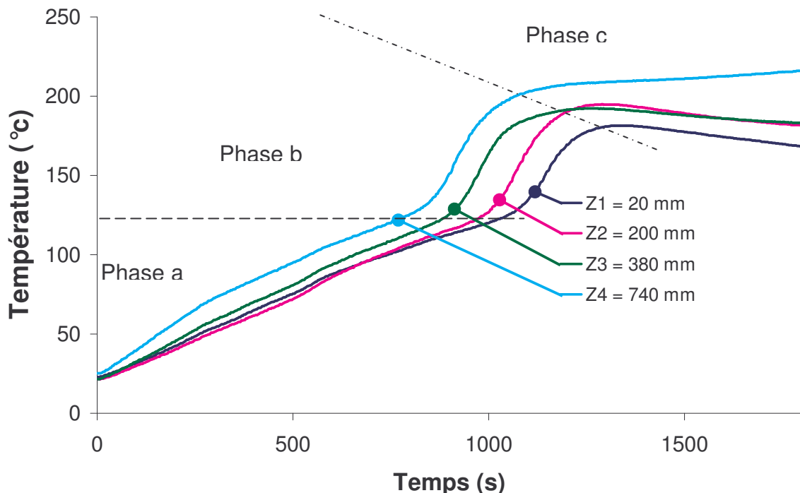
Figure III.21: Evolution des températures le long de l'éprouvette en fonction du temps, obtenue avec le premier moule sans atténuation (EDIA)
