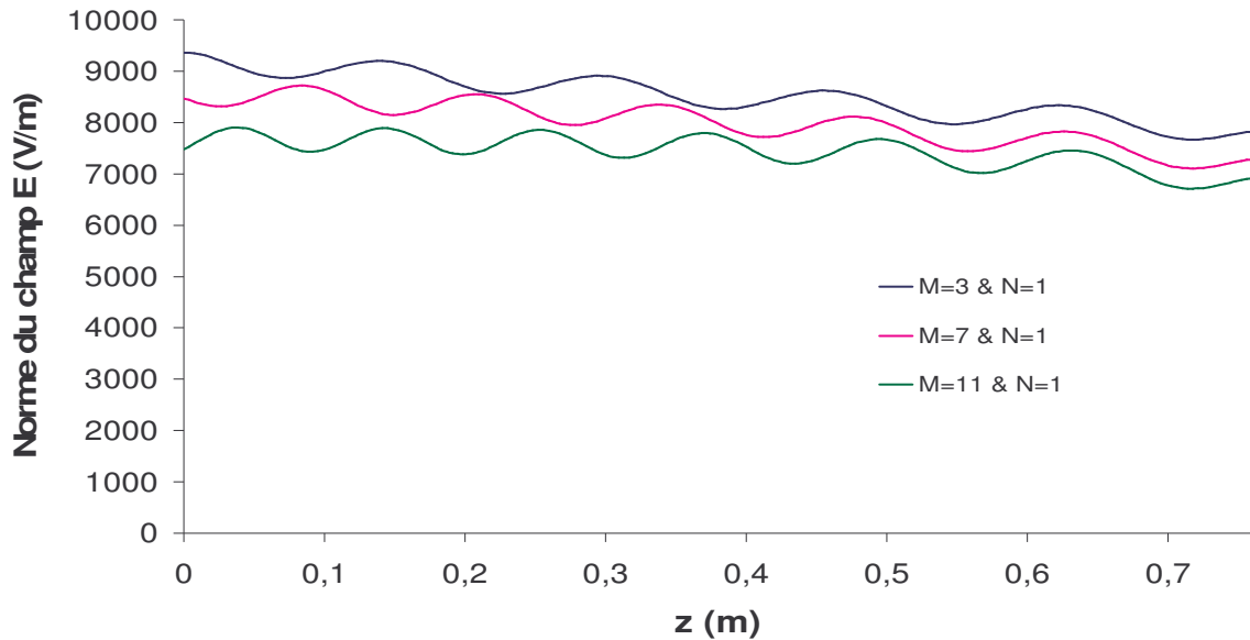
Figure II. 31: Evolution du champ électrique en fonction des dimensions du moule, le long de l'éprouvette de 5 mm d'épaisseur et de 0.30 de caractéristique d'absorption
