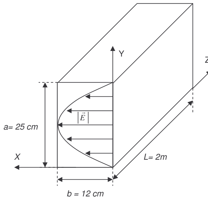
Figure I.6 : Mode TE 01 dans l'applicateur vide et ses dimensions
