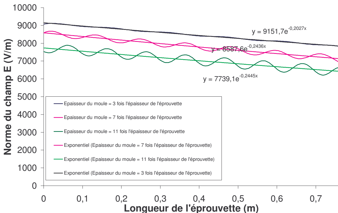
Figure A.II.8: L'évolution de la norme du champ électrique dans une éprouvette de 5 mm en fonction de l'épaisseur du moule, ainsi l'atténuation associée à chaque cas.
