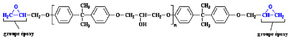
Figure I.1 : Les résines époxydes
