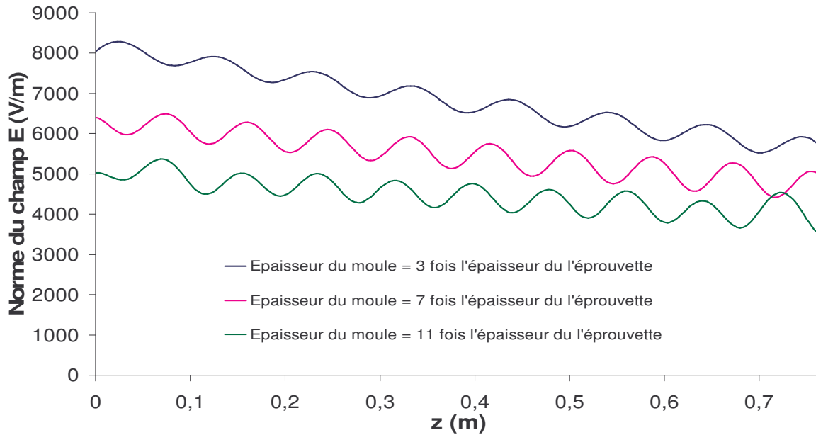
Figure II.24 : Profil de la norme du champ électrique le long de l'éprouvette d'épaisseur 15mm en fonction de l'épaisseur du moule
