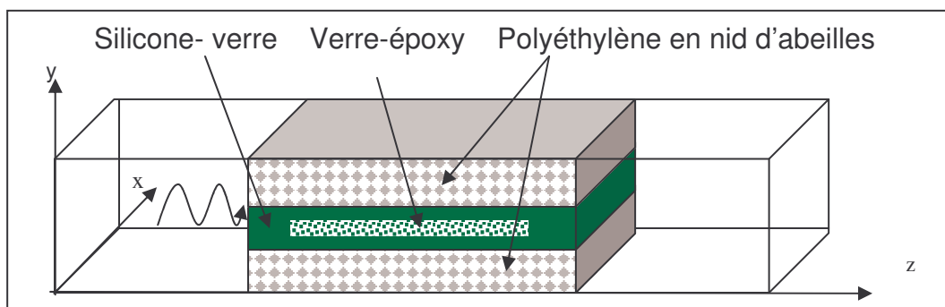
Figure II.13 : Modèle expérimental d'un applicateur rempli par trois diélectriques
