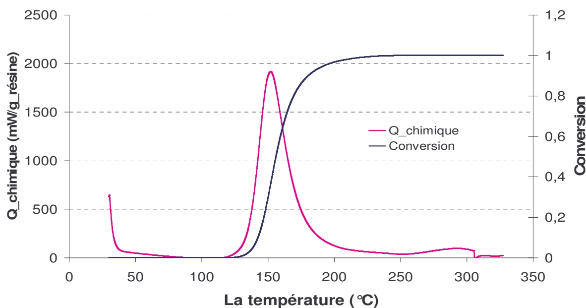
Figure IV.10 : La source chimique et conversion obtenus par DSC
