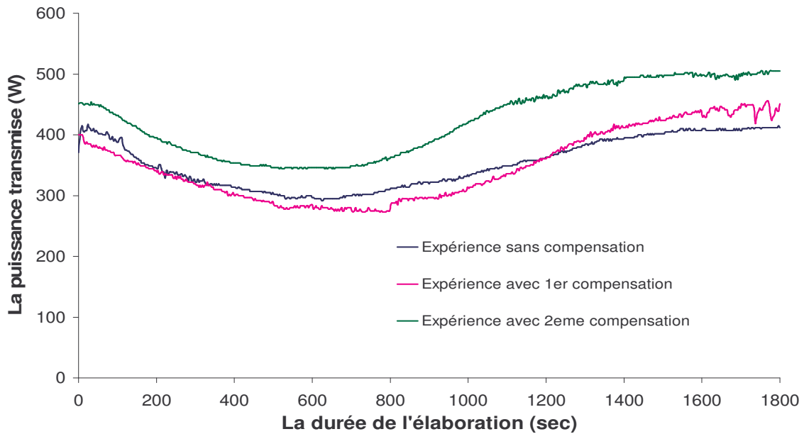
Figure III.29 : Puissances transmises
