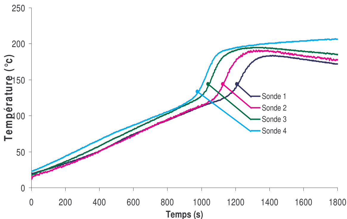
Figure B.III.1 : Evolution des températures le long de la deuxième éprouvette obtenue avec le premier moule sans atténuation (EDIA)
