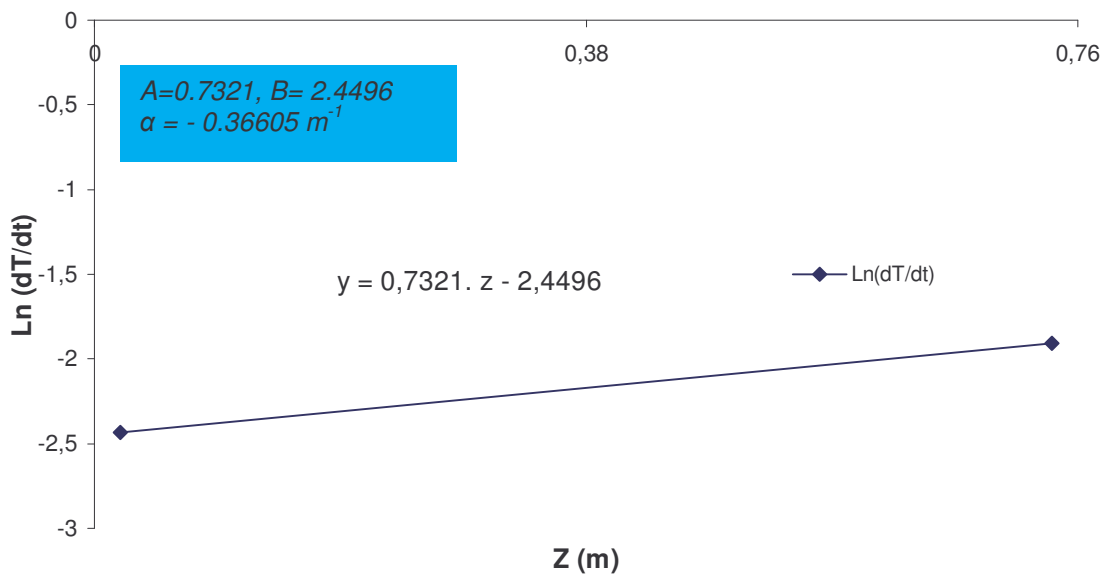
Figure III.26 : L'atténuation entre le point z_1= 0,02 \text{ m} et z_4=0,74\text{m} dans le cas d'un moule avec compensation de l'atténuation (résultat de la figure III.21)
