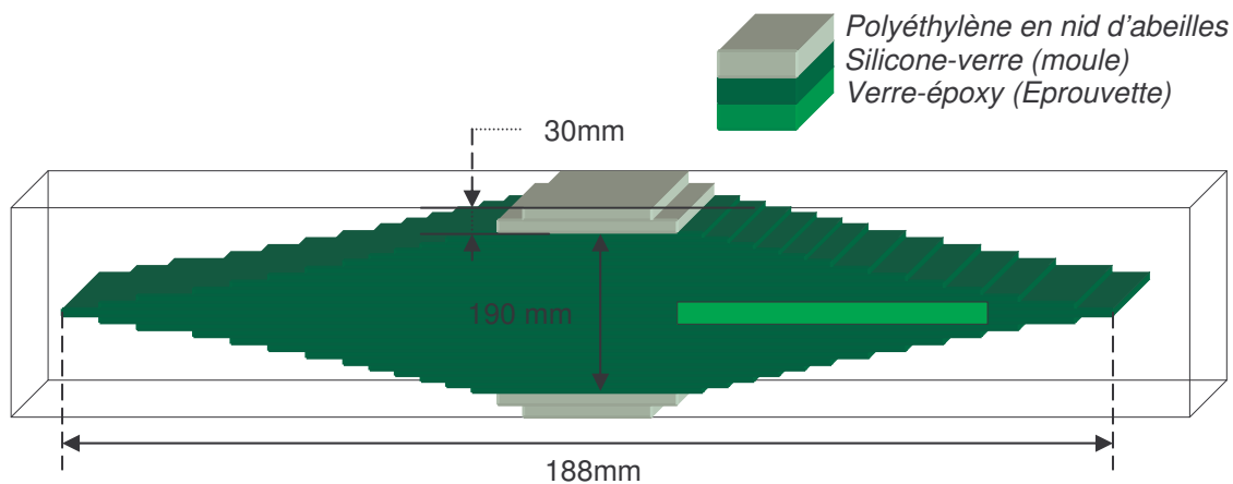
Figure III.16 : La géométrie et les dimensions de modèle du moule expérimental de la première expérience sans atténuation
