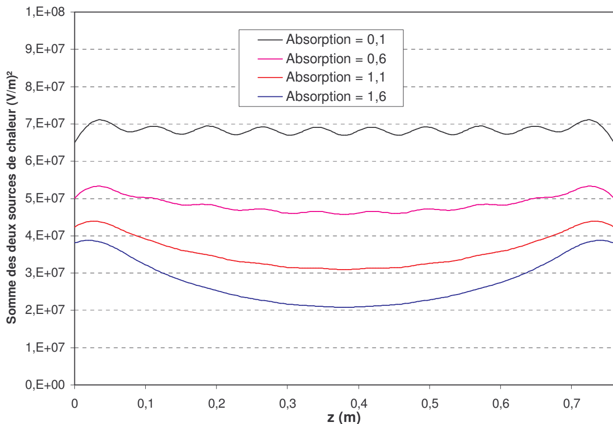
Figure II.29 : La distribution de la source micro-ondes obtenue par deux générateurs en fonction de la caractéristique d'absorption du matériau, avec 105 mm l'épaisseur du moule (l'épaisseur du moule = 7fois l'épaisseur de l'éprouvette)
