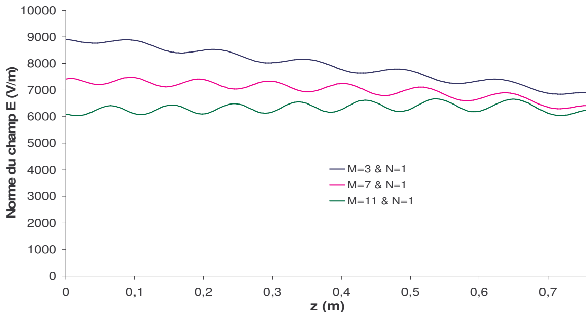
Figure II. 32: Evolution du champ électrique en fonction des dimensions du moule, le long de l'éprouvette de 10 mm d'épaisseur et de 0.30 de caractéristique d'absorption
