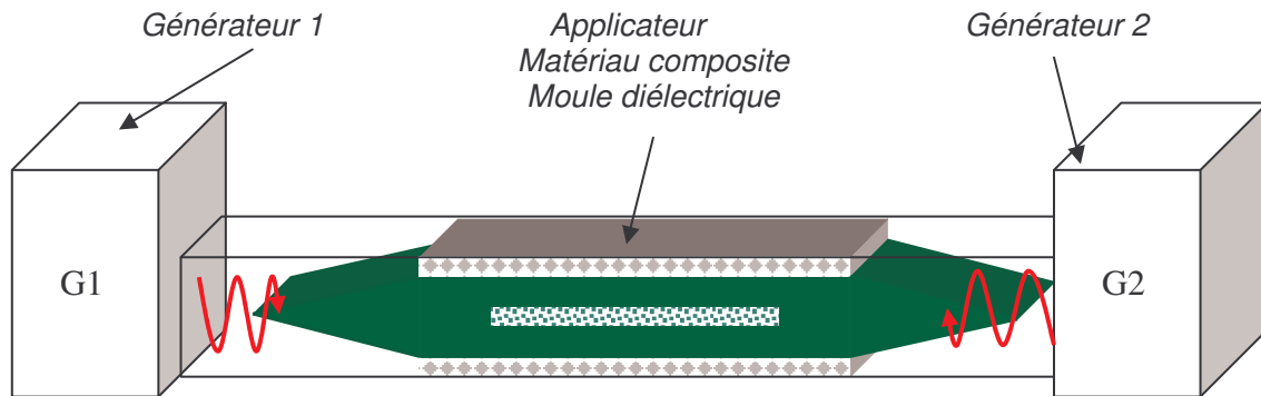
Figure II.28 : Schéma de la solution utilisant deux sources micro-ondes alternées
