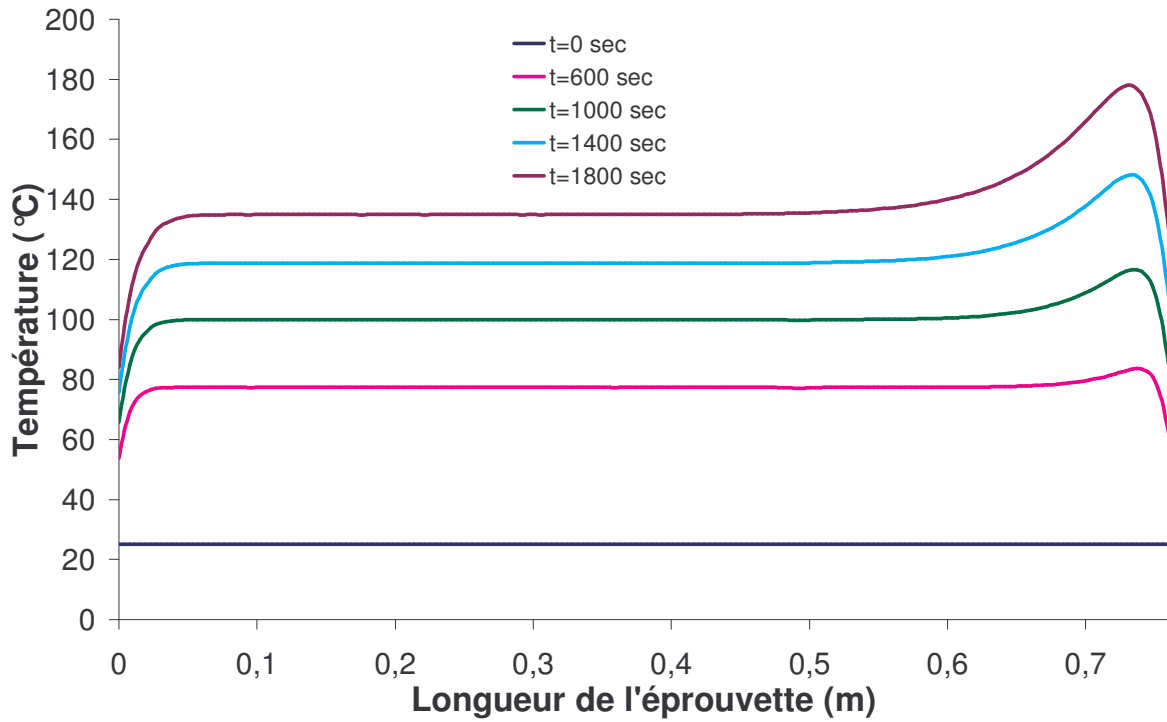
Figure IV. 15 : L'évolution de la température le long du composite en fonction du temps
