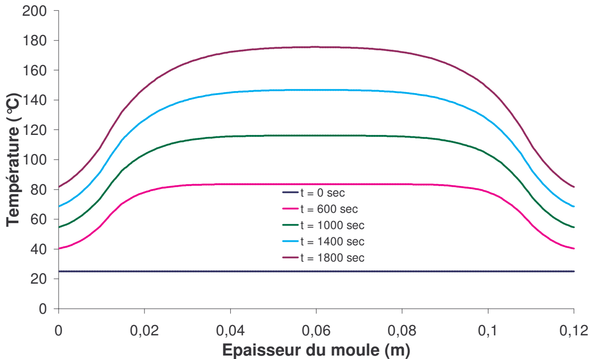
Figure IV.17 : La température suivant x du composite au point z_4 = 0.74 m en fonction du temps
