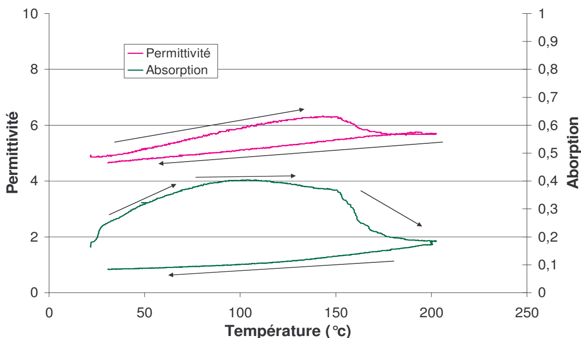
Figure IV.5 : Variation des caractéristiques diélectriques de verre-époxy en fonction de la température à 2450 MHz
