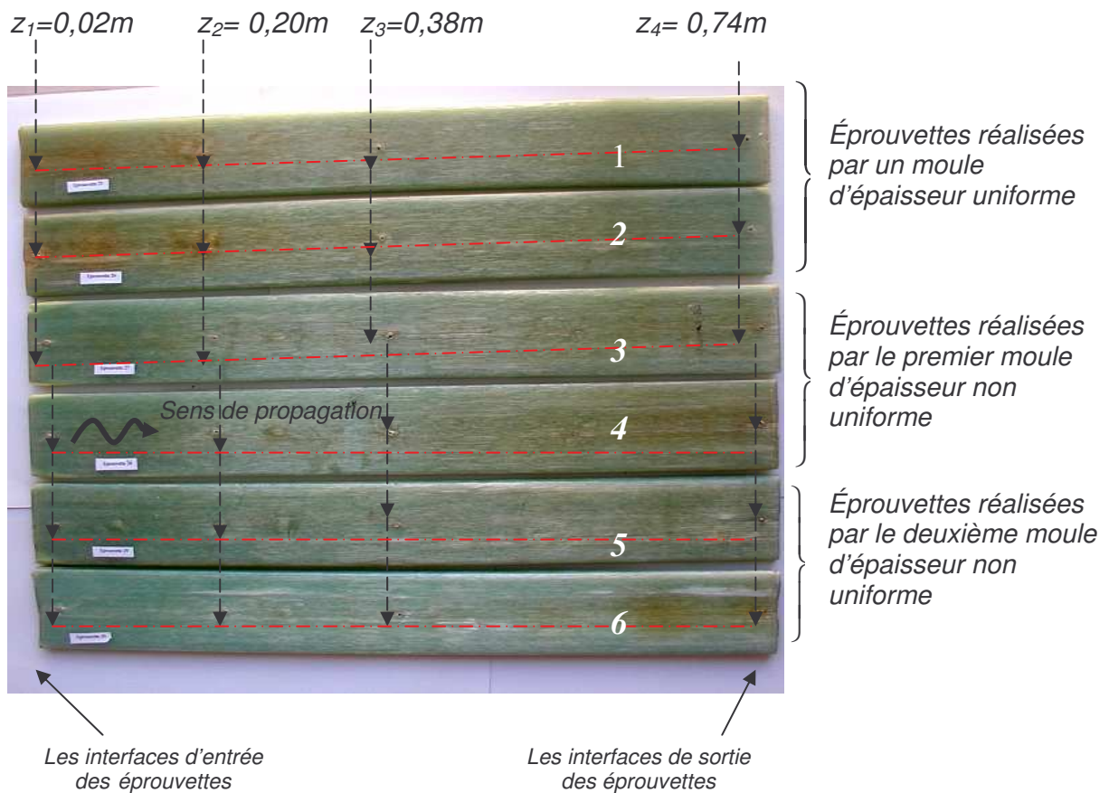
Figure III.24 : Les éprouvettes réalisées
