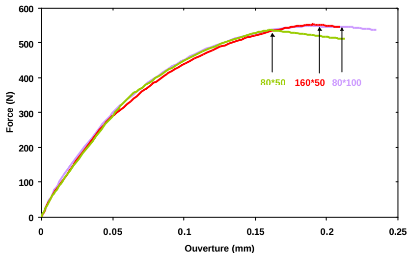
Figure V.16 Courbes force-ouverture pour les éprouvettes DENT à 20°C, en pilotage LVDT à 0.05 mm/s, pour a/B = 0.5 , et trois tailles de maille en \mu\text{m} (80-50, 160-50 et 80-100).
