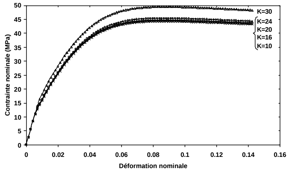
Figure IV.3 Etude de la sensibilité du paramètre K sur éprouvette lisse pour n=5 , Q=40 , b=75 , 20^\circ\text{C} , 1.5 \cdot 10^{-4} \text{ s}^{-1}
