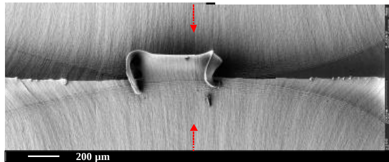
Figure III.39 Observation d'une zone de déchirement ductile pour une éprouvette DENT, traction in-situ, 3 µm/s, 20°C
