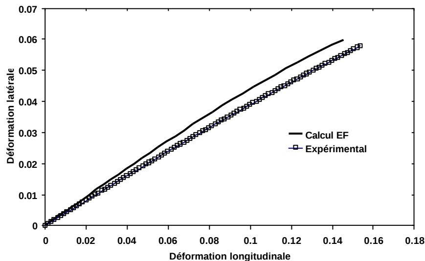
Figure IV.34 Déformation latérale en fonction de la déformation longitudinale, expérimentales et simulées, sur éprouvettes lisses, à 20°C, 1,5 \cdot 10^{-4} \text{ s}^{-1}
