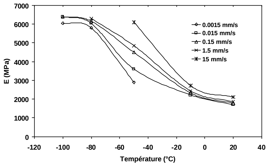
Figure II.13 Evolution du module d'Young apparent en fonction de la température (entre -100^{\circ}\text{C} et 20^{\circ}\text{C} ) et de la vitesse (entre 0.0015 mm/s et 15 mm/s)
