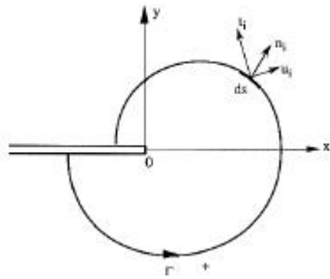
Figure A.I.4 Description de l'intégrale de contour J
