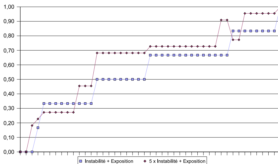
FIG. 3.5 – Comparaison des distributions normalisées des valeurs de risques calculées avec ou sans pondération, à partir des valeurs d’instabilité et d’exposition au risque (coefficients respectifs utilisés : 1 et 1, puis 5 et 1).
