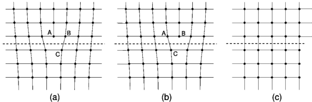
FIG. 1.3 – Déplacement d'une dislocation coin
