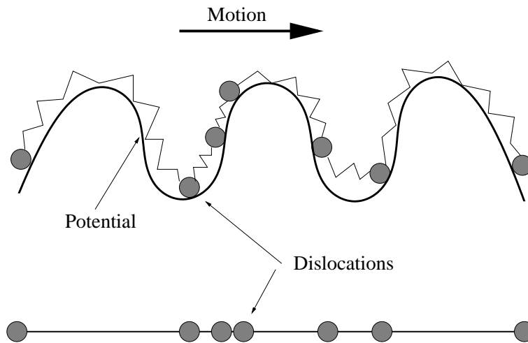
FIG. 8 – Représentation schématique d'un modèle 1D pour des dislocations reliées par des ressorts
