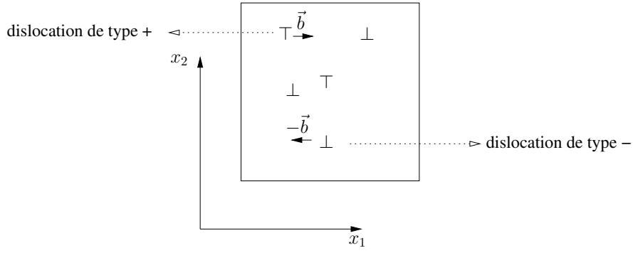
FIG. 10 – Section transversale des lignes de dislocations.
