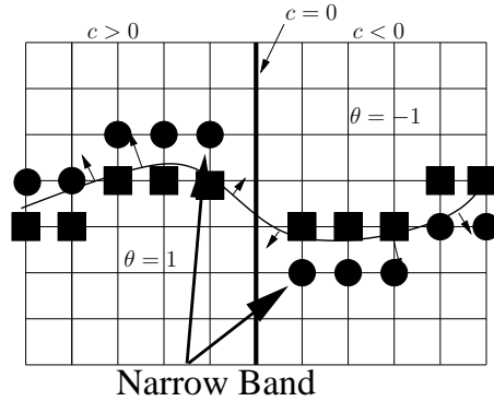
FIG. 4 – Schéma de la Fast Marching Généralisée
