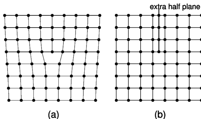
FIG. 1.1 – Géométrie d'une dislocation coin
