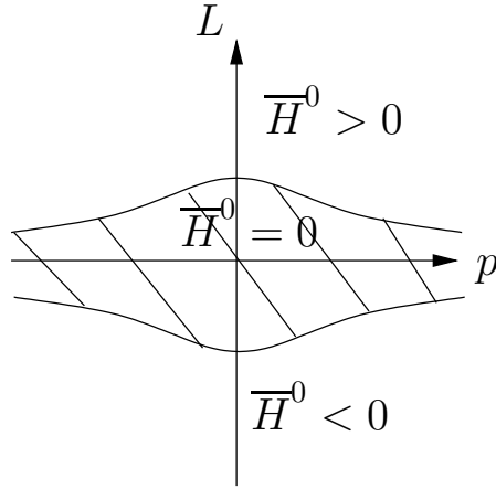
FIG. 9 – Représentation schématique de l'Hamiltonien effectif
