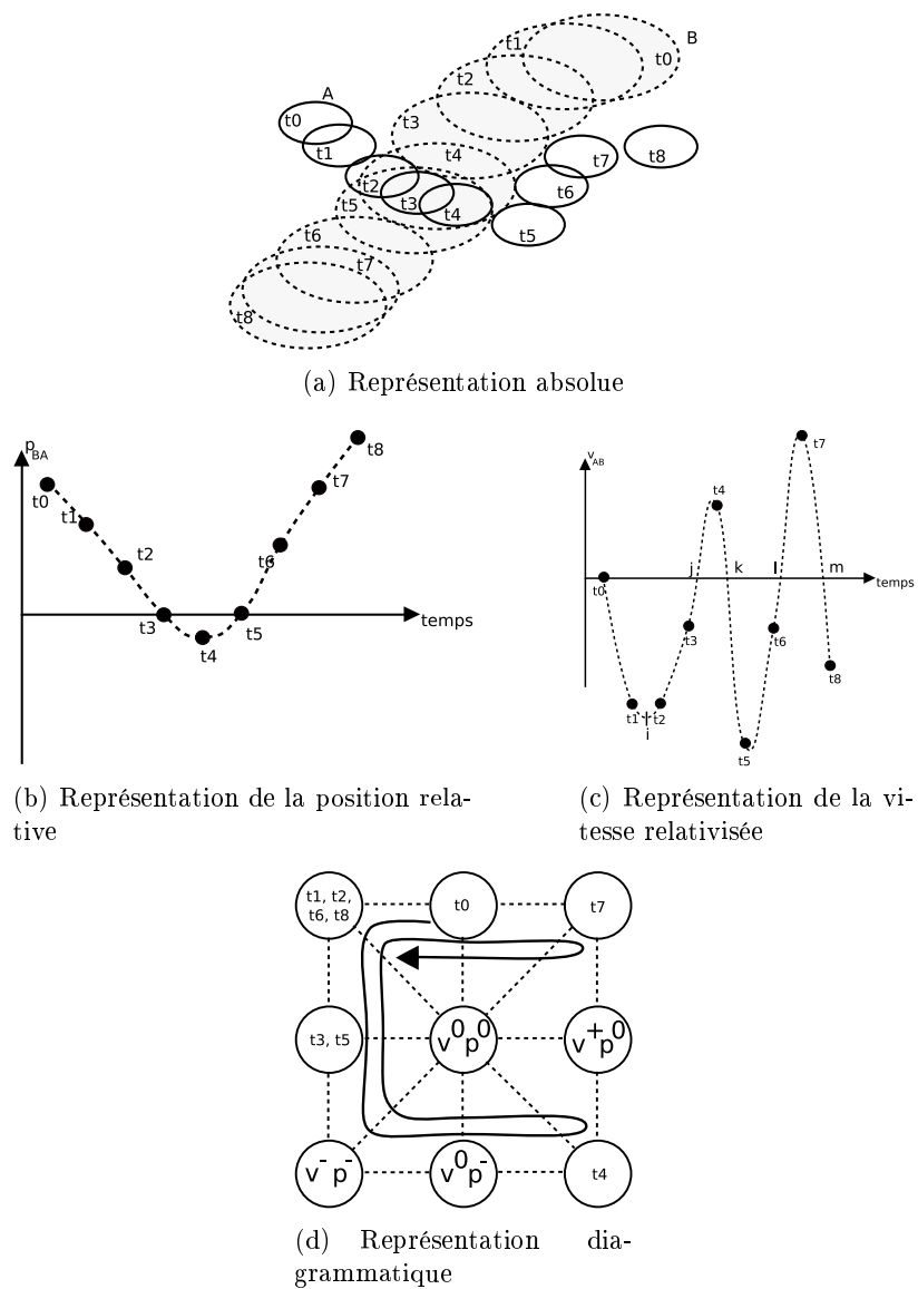
Figure B.2 — Situation : deux polygones ( A objet référent) mobiles se croisent
