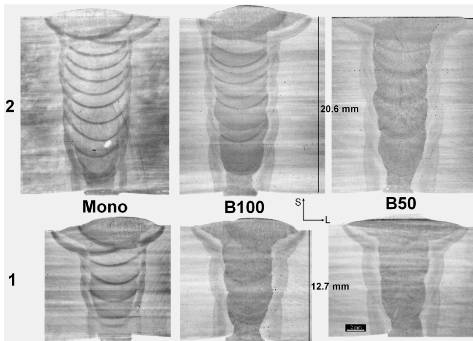
Figure II-3 : Allure des 6 soudures de raboutage coupe LS et notations en gras
