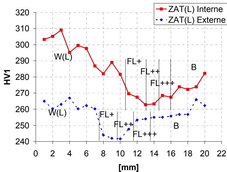
Figure II-16 : Dureté partant du centre de la soudure longitudinale W(L) en direction de la ZAT, en interne et en externe
