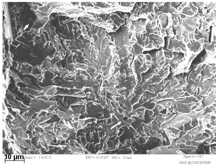
Figure III-12 : Faciès de rupture fragile à -196\text{ }^{\circ}\text{C} , ZAT F près du délaminage avec particules de TiN (flèches)
