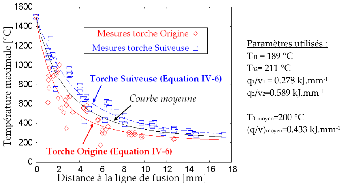
Figure IV-7. Température maximale de pic en fonction de la distance à la ligne de fusion pour un tube en acier à haute limite d'élasticité, issu des acquisitions sur cycles réels
