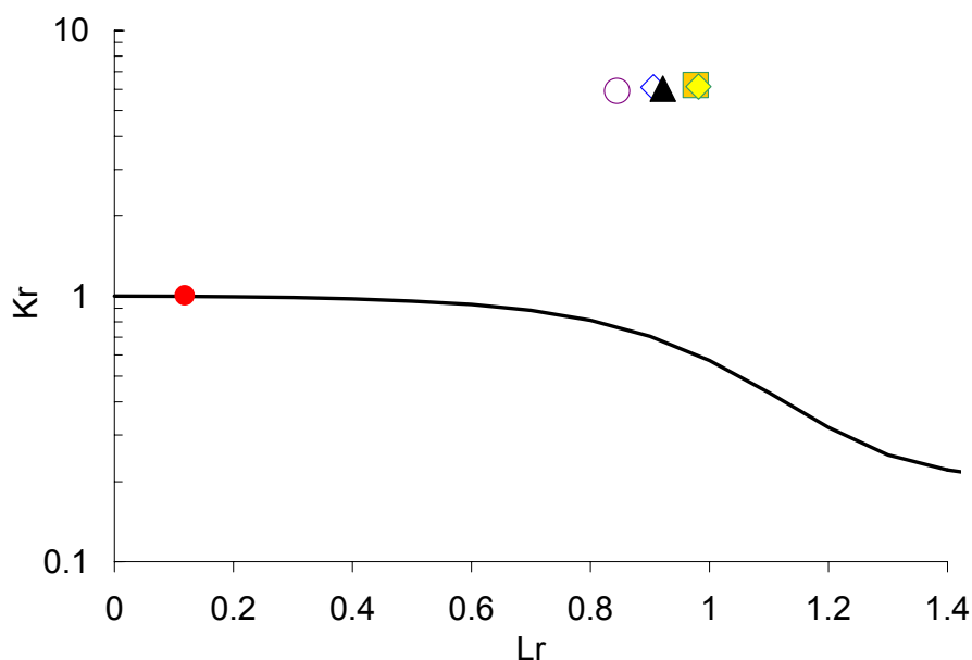
Fig. F-108 : Placements des points concernant les défauts en ligne de fusion à différentes températures (cercle à -100\text{ °C} et carré à -40\text{ °C} ). Prévission de la rupture (cercle plein) à -20\text{ °C} pour une force maximale de 2.5 kN au lieu des 20.1 kN réels.
