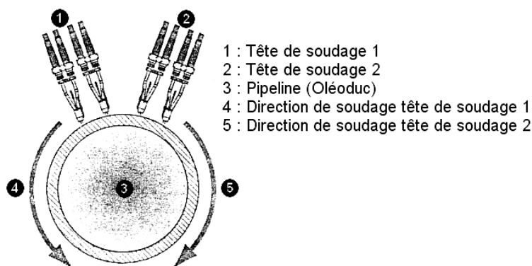
Figure I-19 : Du sommet du tuyau, les deux têtes tandem doubles soudent le pipeline de diamètre 1321 mm jusqu'au « point de rendez-vous » inférieur [M&T03]
