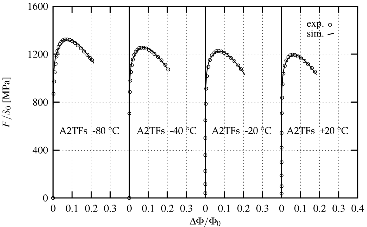
Figure V-35 : Résultats de l'identification pour la ZAT Fs sur les courbes des essais sur éprouvettes entaillées A2 entre -80 et +20 °C
