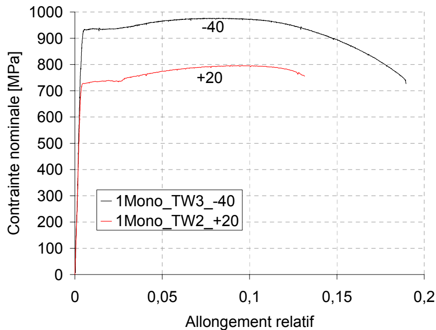
Fig. E-80 : Courbes des essais de traction sur le métal fondu du 1 Mono
