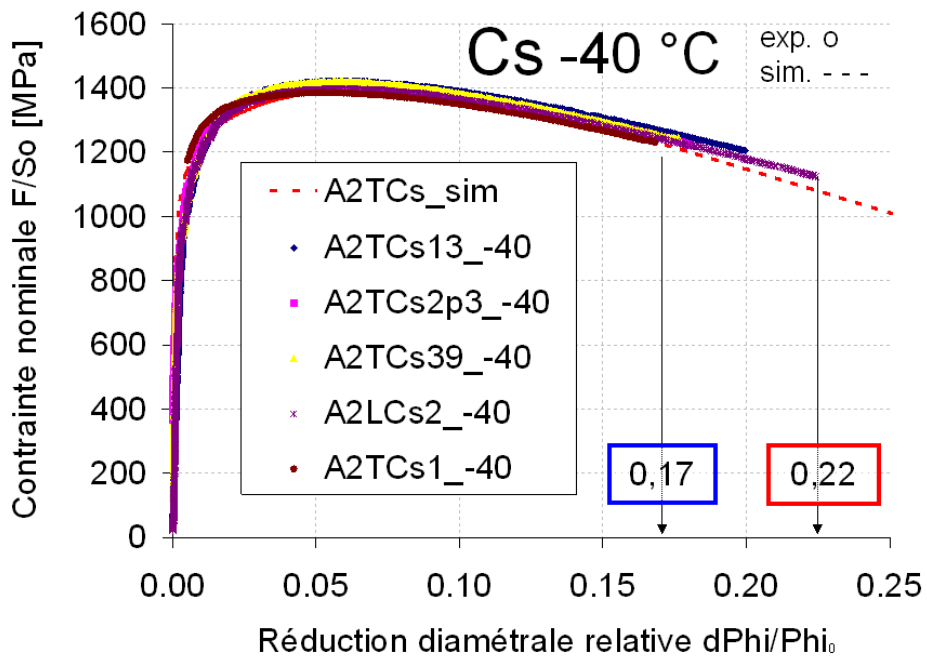
Figure V-39 : Graphique rassemblant les courbes contraintes-réduction diamétrale à -40 °C des éprouvettes de traction axisymétriques entaillées en Cs ; les déformations à rupture maximales et minimales sont utilisées ensuite pour ajuster le critère de rupture
