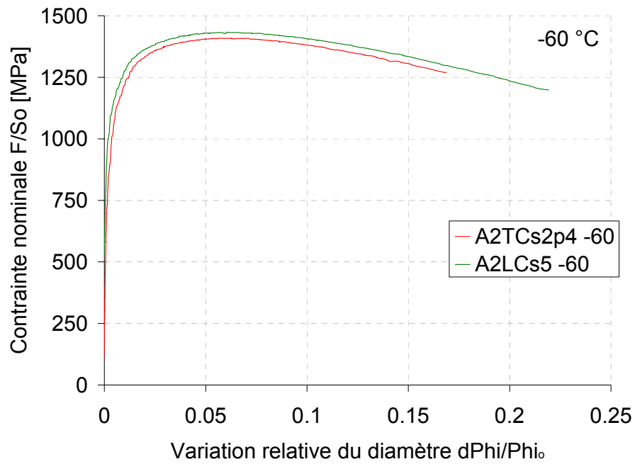
Fig. E-88 : Courbes de traction sur éprouvettes entaillées dans la ZAT Cs testées à -60\text{ °C}
