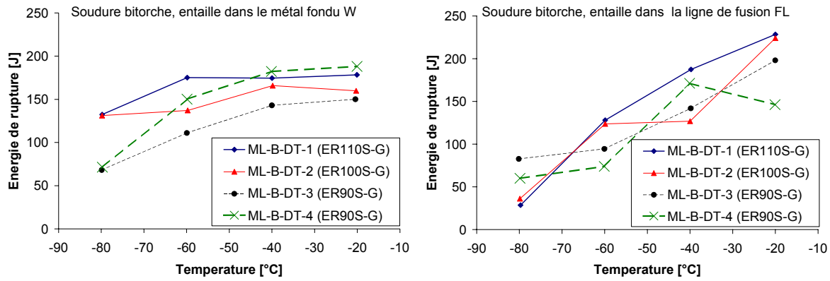
Figure I-24 : Résilience des soudures de rabotage entaillées dans le métal fondu (W) ou en ligne de fusion (FL) d'une soudure Bitorche [HAMM02-PDC]
