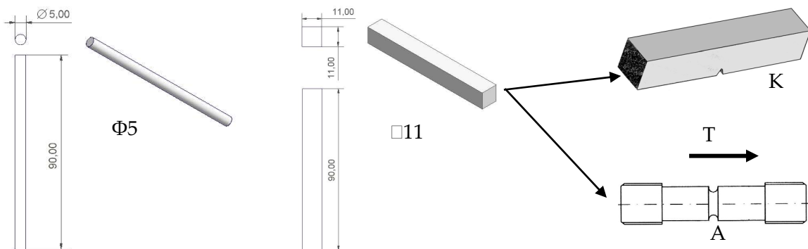
Figure IV-10 : Plans des ébauches Gleeble ( \Phi 5 , \square 11 ) et schémas des éprouvettes qui seront usinées (K, A).
