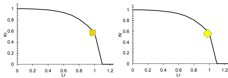
Fig. F-110 : Résultats à - 40 (carré) et -20 °C (losange)
