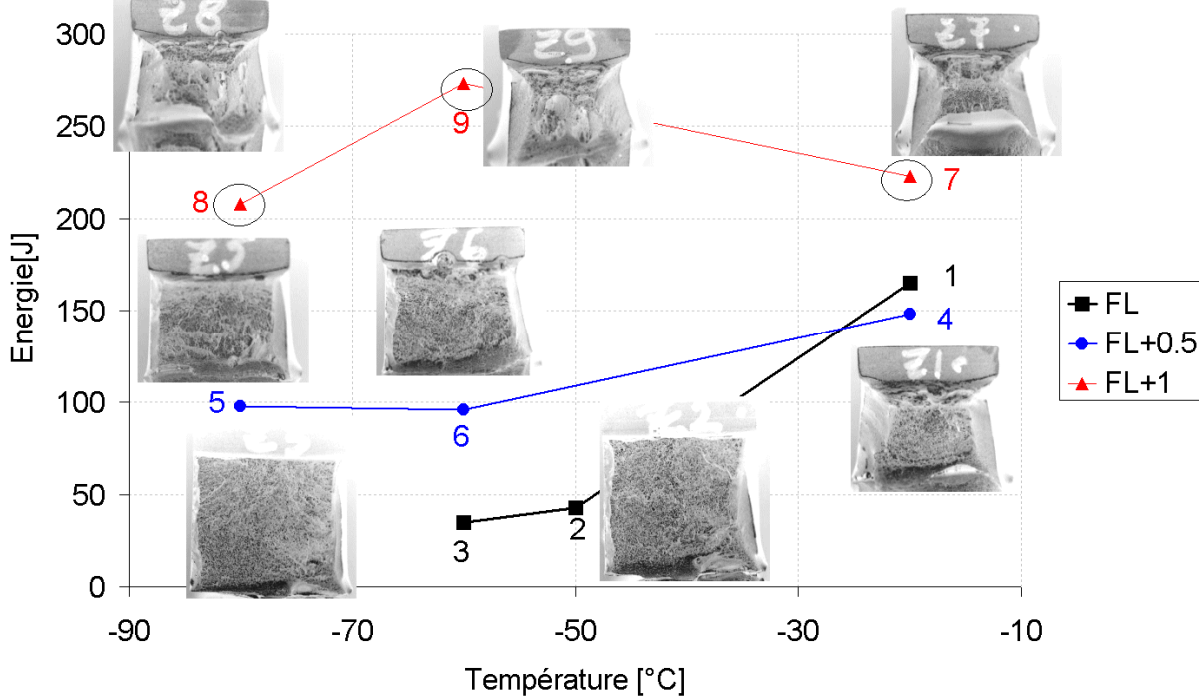
Courbes de résilience - 1B100
