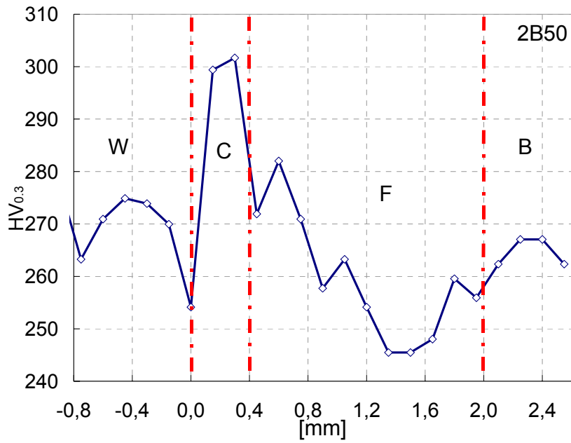
Figure II-24 : Dimensions des zones du joint, 2B50, profil à 2mm de la peau interne dans la direction L de la soudure de rabotage ; l'abscisse 0 mm correspond à la ligne de fusion
