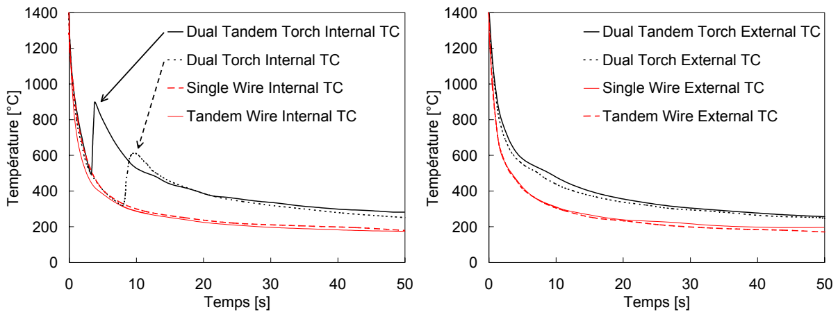
Thermocouple plac e en peau interne Thermocouple plac e en peau externe Dual Tandem : 2 tandems, Dual Torch : 2 torches, Single Wire : 1 torche, Tandem Wire : 1 tandem
