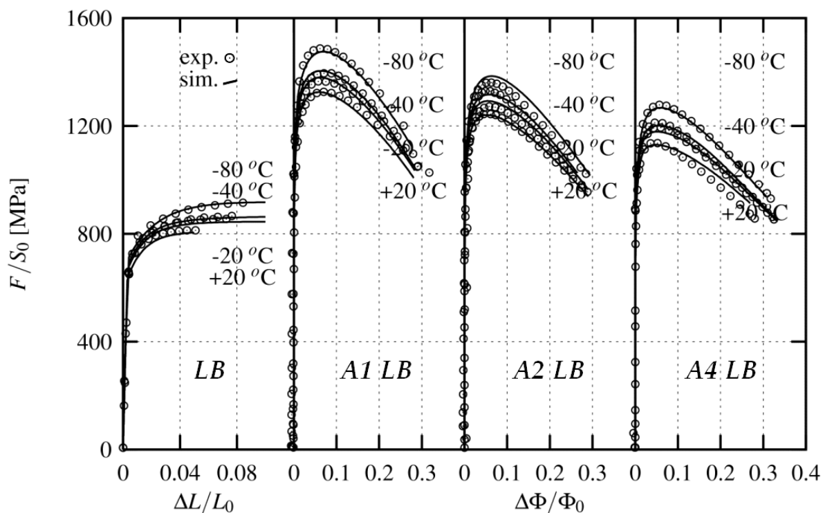
Figure V-32 : Résultats de l'identification pour le métal de base B sur les courbes des essais de traction sur éprouvettes lisses et entaillées
