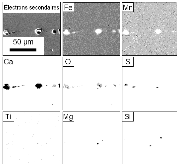
Figure II-32 : Exemples d'inclusions présentes dans le métal de base, image en haut à gauche est obtenue avec les électrons secondaires, les autres sont obtenues suite au comptage de chaque élément (noir : forte teneur, blanc : absence)
