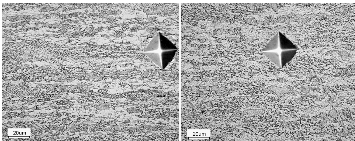
Figure II-8 : Métal de base B à 3 mm et 12 mm de la peau interne du tube (2B100).
