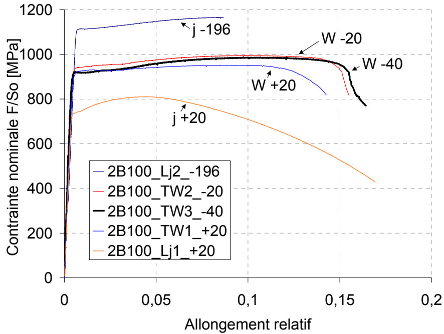
Fig. E-78 : Courbes des essais de traction sur le joint et le métal fondu du 2B100
