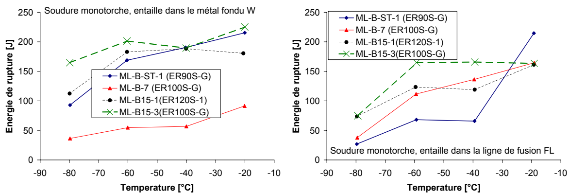
Figure I-25 : Résilience des soudures de rabotage entaillées dans le métal fondu (W) ou en ligne de fusion (FL) d'une soudure Monotorche [HAMM02-PDC]
