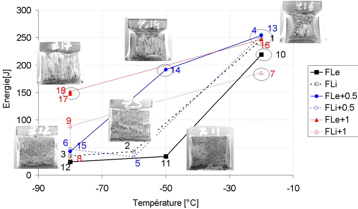
Courbes de résilience - 2B100
