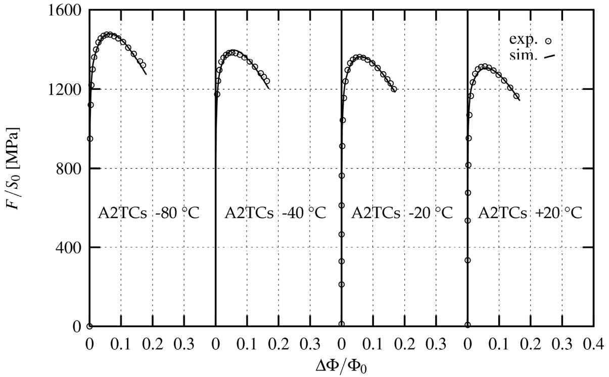
Figure V-34 : Résultats de l'identification pour la ZAT Cs sur les courbes des essais sur éprouvettes entaillées entre -80 et +20 °C
