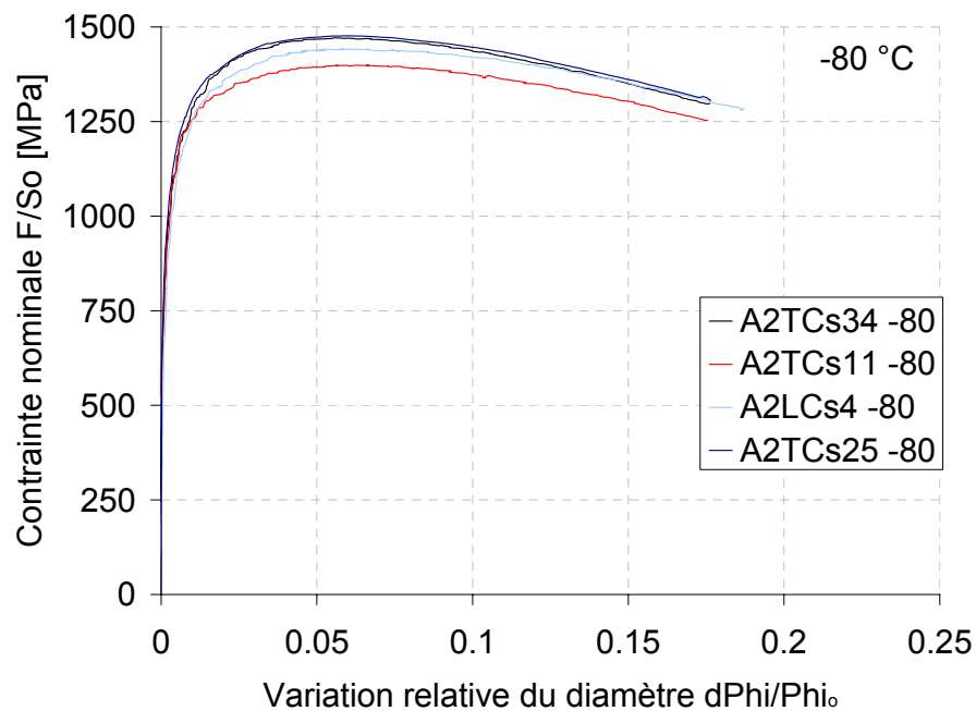
Fig. E-87 : Courbes de traction sur éprouvettes entaillées dans la ZAT Cs testées à -80\text{ }^{\circ}\text{C}
