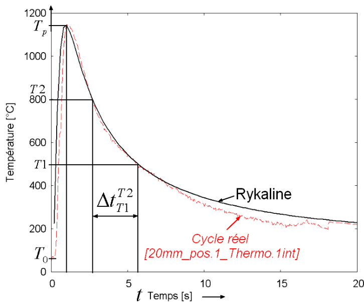
Figure IV-6 : L'équation (IV-5) de Rykaline ajustée sur la température mesurée à 1.5 mm de FL
