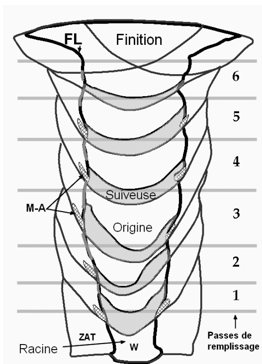
Figure II-22 : Schéma représentant les passes d'une bitorche, FL, ZAT, M-A et passes suiveuses recuites
