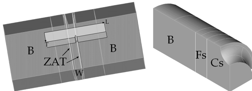
Figure V-29 : Modeler OpenCascade - création de l'éprouvette et placement de l'éprouvette entaillée dans une « boîte » dont les secteurs définiront les sous-domaines à mailler
