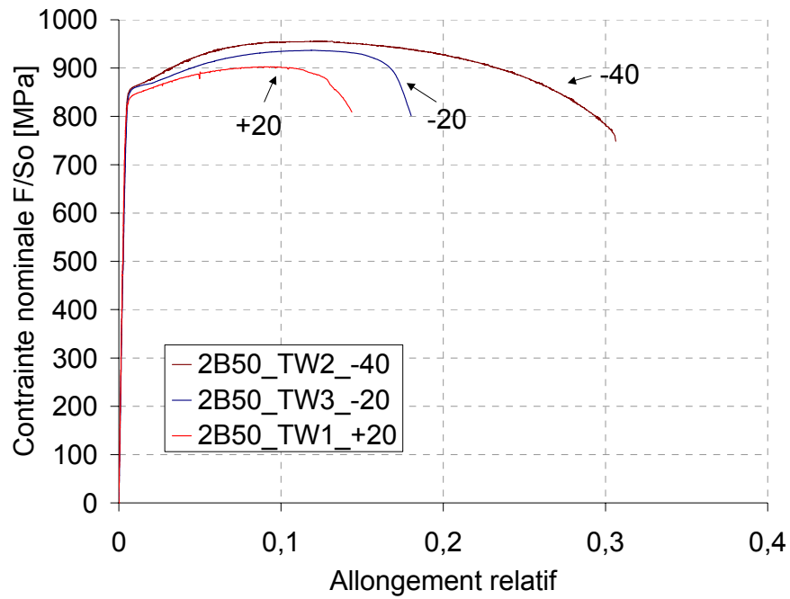
Fig. E-73 : Courbes des essais de traction sur le métal fondu du 2B50
