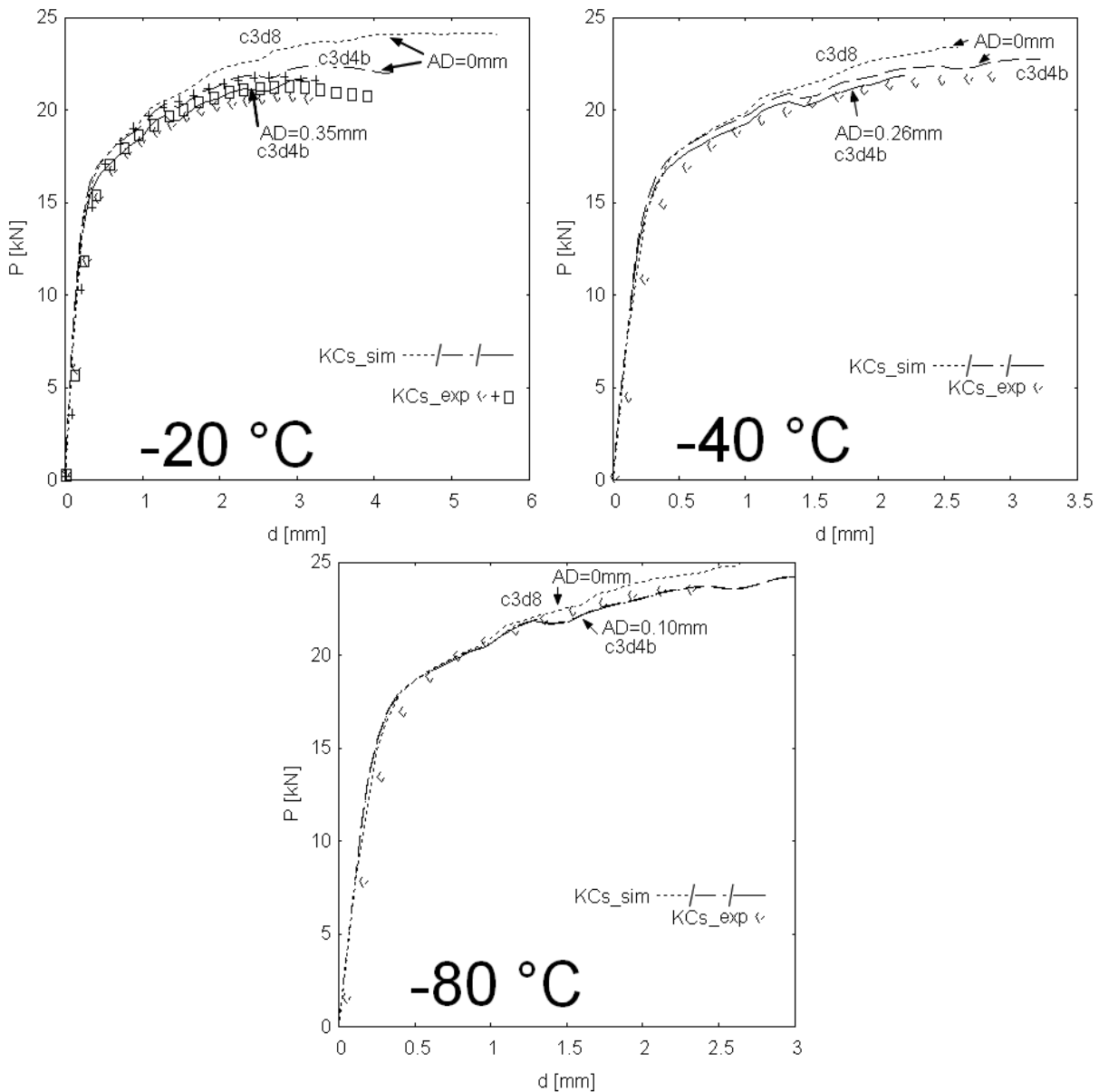
Figure V-44 : Courbes expérimentales et simulées pour KTCs à -20 , -40 et -80\text{ °C} avec avancée ductile (AD) et sans avancée ductile (AD=0mm) avec des éléments linéaires hexaèdres (c3d8) ou bulles (c3d4b)
