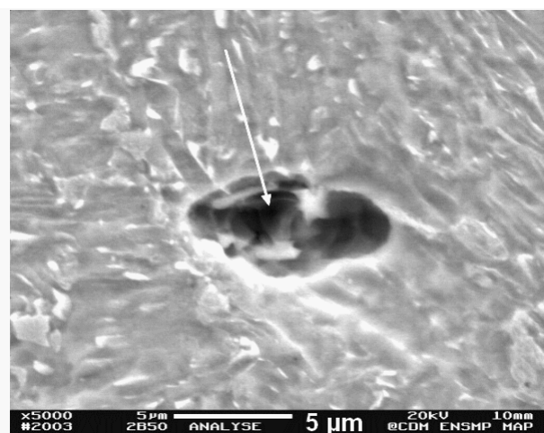
Figure II-34 : Inclusion de titane (analyse EDX) dans la zone à gros grains du 2B50
