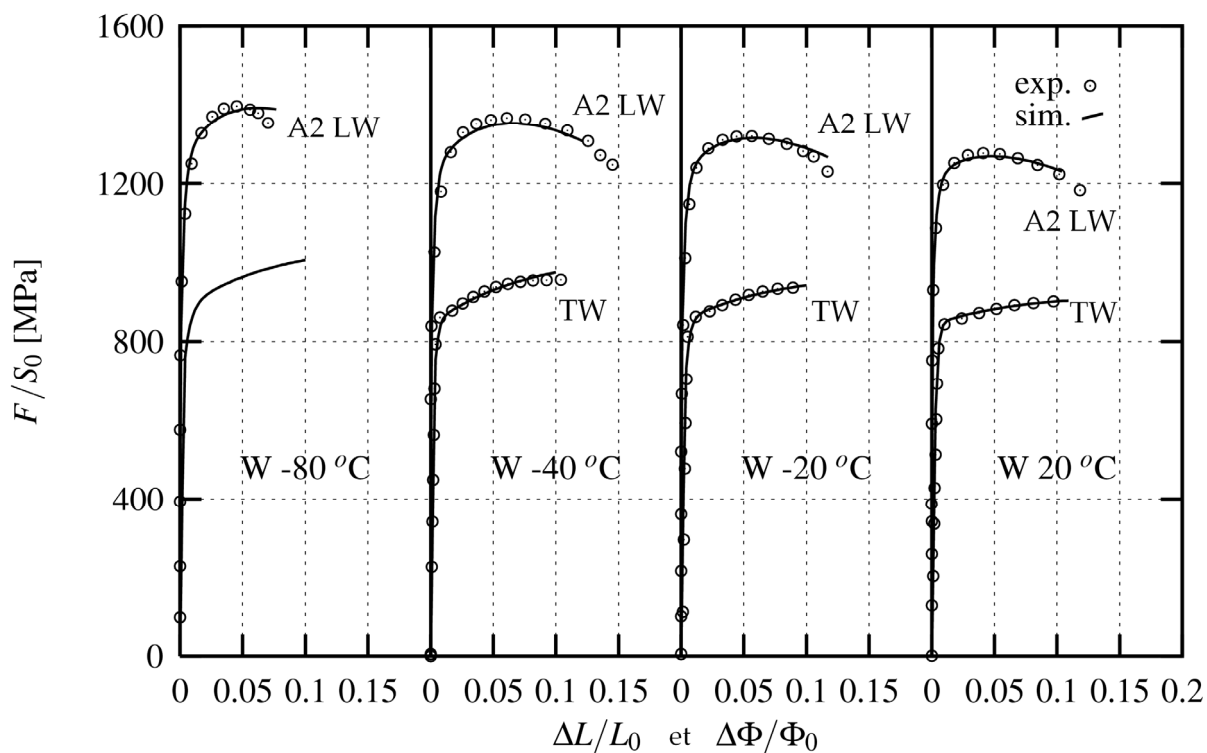
Figure V-33 : Résultats de l'identification pour le métal fondu W sur les courbes des essais sur éprouvettes de traction lisses (en bas) et entaillées (en haut) entre -80 et +20^\circ\text{C}
