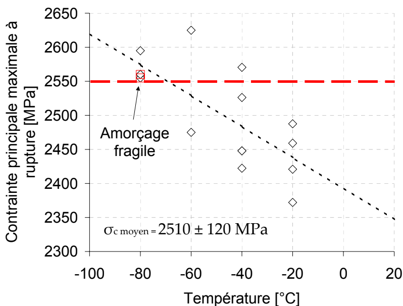
Figure V-41 : Détermination de la contrainte critique avec la contrainte relevée lorsque les amorçages sont fragiles (2550 MPa)
