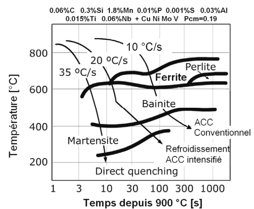
Figure I-8 : Diagramme TRC « schématisé » sur une plaque X100 de 20mm [OKAT02-PDC]
