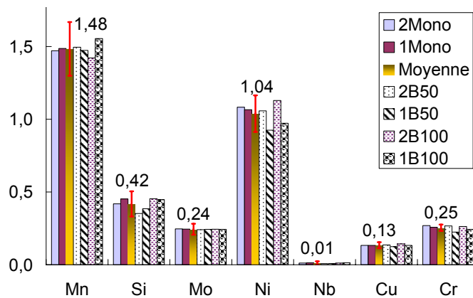
Figure II-39 : Composition du métal fondu dans toute l'épaisseur
