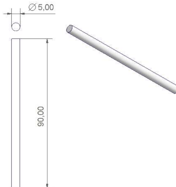
Fig. E-63 : Ebauches cylindriques, de 5 mm de diamètre (φ5) prélevées à aléatoire dans l'épaisseur
