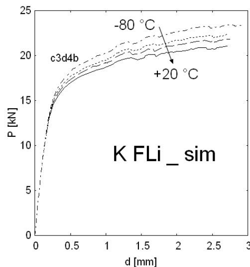
Figure V-48 : Simulations des éprouvettes de flexion 3 points entaillées en ligne de fusion entre -80 et +20\text{ °C}
