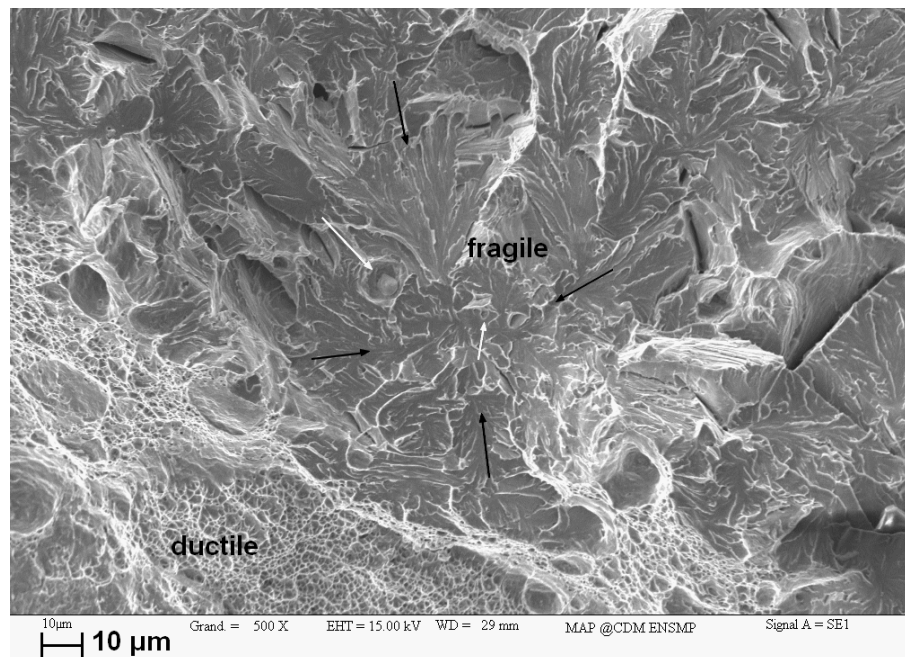
Figure V-21 : Zoom sur le faciès d'une éprouvette de traction entaillée dans le joint réel en ligne de fusion, testée à -20 °C, l'amorce ductile et les inclusions (flèches blanches) facilitent la propagation fragile
