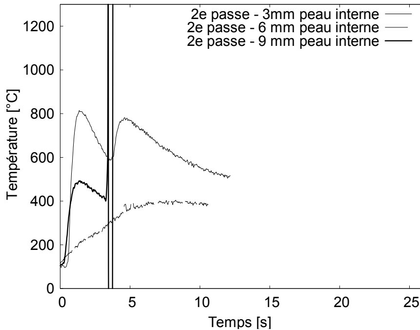
Fig. D-32 : Cycles de température, épaisseur 12 mm, position 1, 3 thermocouples, 2 ème passe
