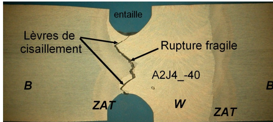
Figure V-20 : Coupe d'une éprouvette de traction entaillée dans le joint réelle en ligne de fusion, testée et rompue à -40 °C
