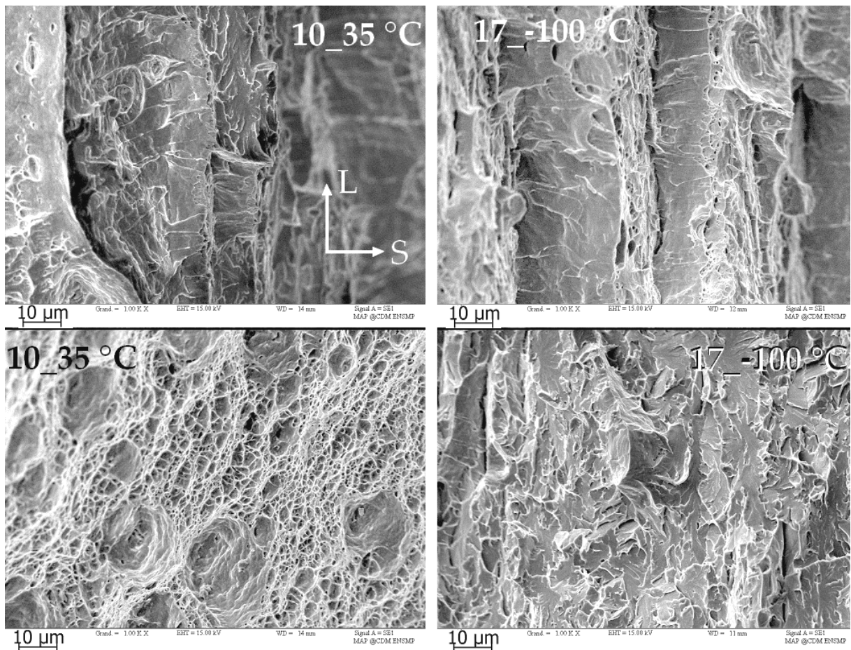
Figure III-23 : En haut, délaminage au moins partiellement fragile dans les 2 cas. En bas, rupture ductile à 35 °C et fragile à -100 °C
