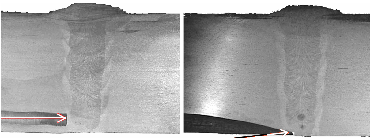
Figure IV-1 : Exemple de soudage des thermocouples au fond du meulage dans le tube de 20.6 mm. Positionnés à droite à 3 mm de la peau interne et à gauche en racine à 1.5 mm de l'axe soudure
