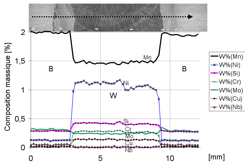
Figure II-38 : Composition massique à travers la soudure de rabotage 2B50, on traverse la passe recuite S_n entre 7 et 9 mm
