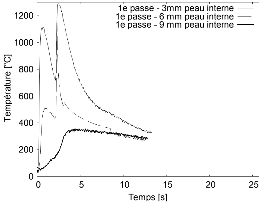
Fig. D-31 : Cycles de température, épaisseur 12 mm, position 1, 3 thermocouples, 1 ère passe
