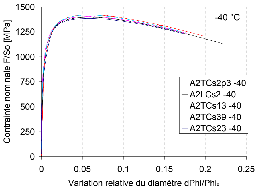
Fig. E-89 : Courbes de traction sur éprouvettes entaillées dans la ZAT Cs testées à -40\text{ °C}
