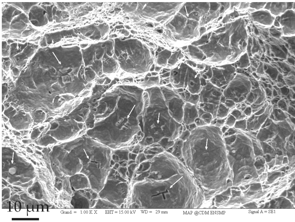
Figure V-11 : Particules de TiN multi-fissurés et de CaS (flèches blanches) au centre de grosses cupules, éprouvette de traction entaillée dans la ZAT Cs testée à 20 °C, A2TCs21_20 °C, électrons secondaires
