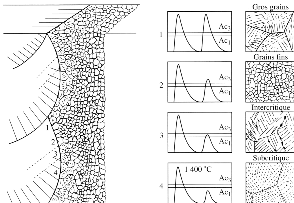
Figure I-29 : Différents types de microstructures en ZAT en fonction des cycles thermiques, d'après [TOYO89]
