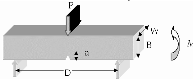
Fig. F-101 : Epreuve de flexion 3 points
