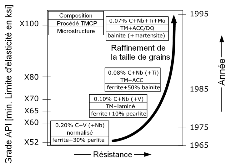
Figure I-3 : Développement des pipelines (composition, procédé TMCP, microstructure, API grade), [HEIS01]
