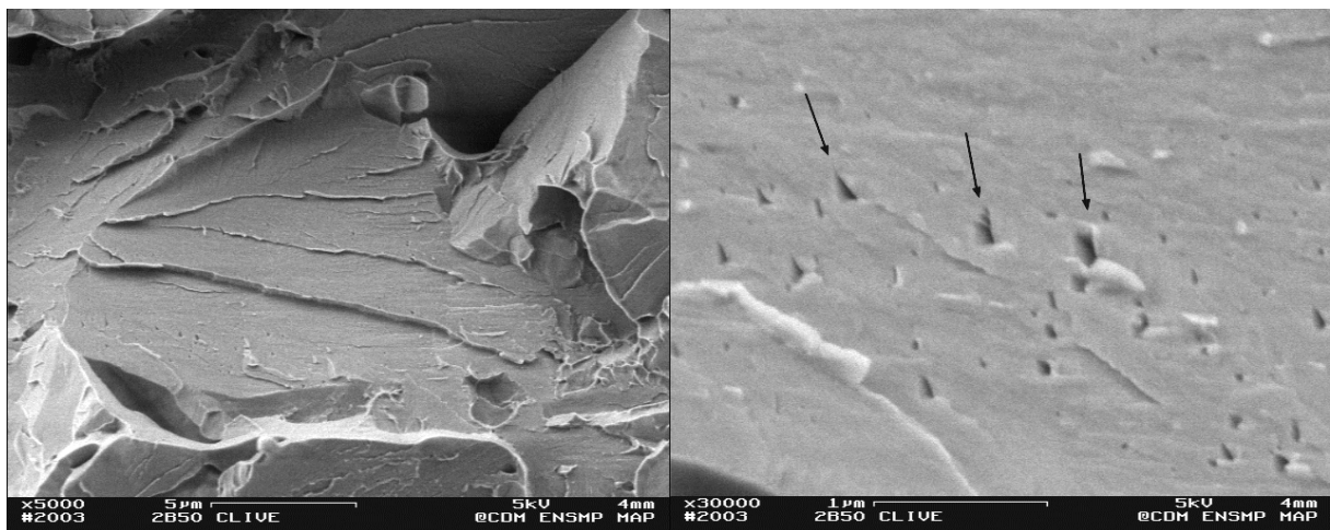
Figure III-3 : Clivage transgranulaire dans la ferrite et languettes de clivage (flèches noires)
