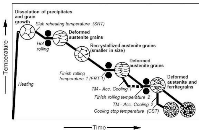
Figure I-7 : Traitement thermomécanique lors de la mise en forme de la tôle, [HILL01-43]
