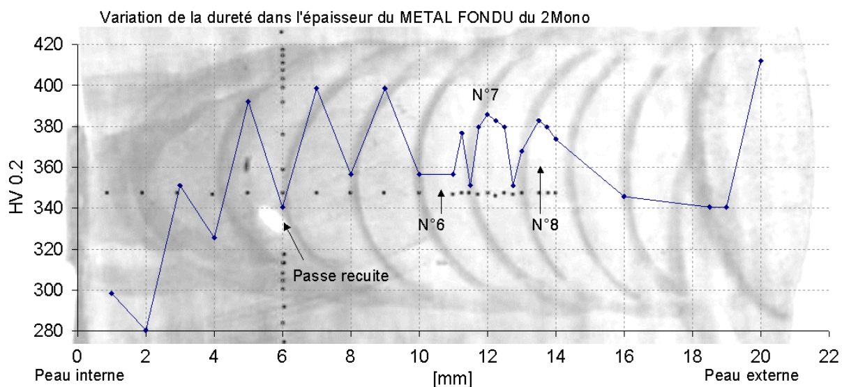
Figure II-40 : Variation de la dureté HV 0.2 dans l'épaisseur du W du 2 Mono, les points noirs sont les empreintes de mesures de dureté
