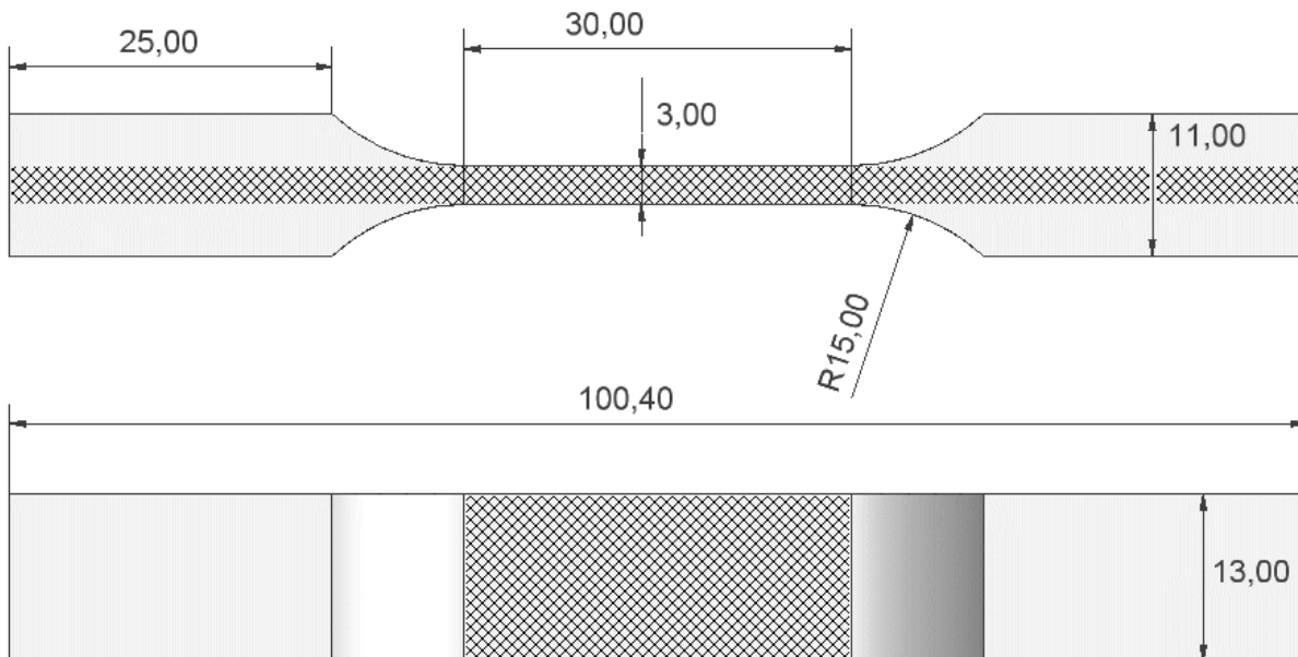
Fig. E-69 : Eprouvte de traction « Allweld » dans le métal fondu pour le tube d'épaisseur 20.6 mm
