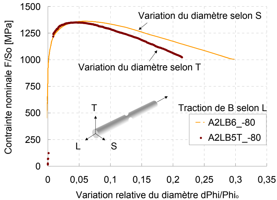
Fig. E-86 : Courbes de traction sur éprouvettes entaillées A2 dans le métal de base à -80\text{ }^{\circ}\text{C}
