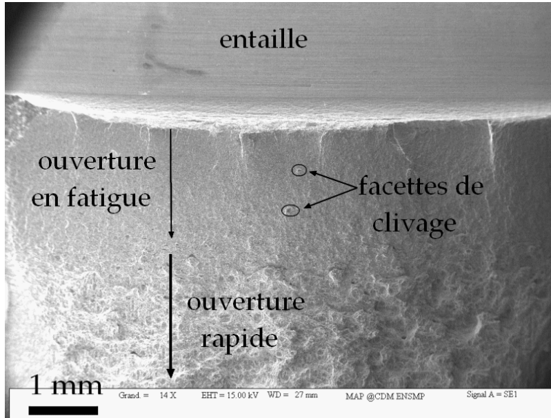
Figure V-14 : Avancée ductile, facettes de clivage arrêtées dans le front de fatigue et ouverture rapide, éprouvette de flexion 3 points KTCs_L, testée à -20 °C, interrompue et ouverte en fatigue
