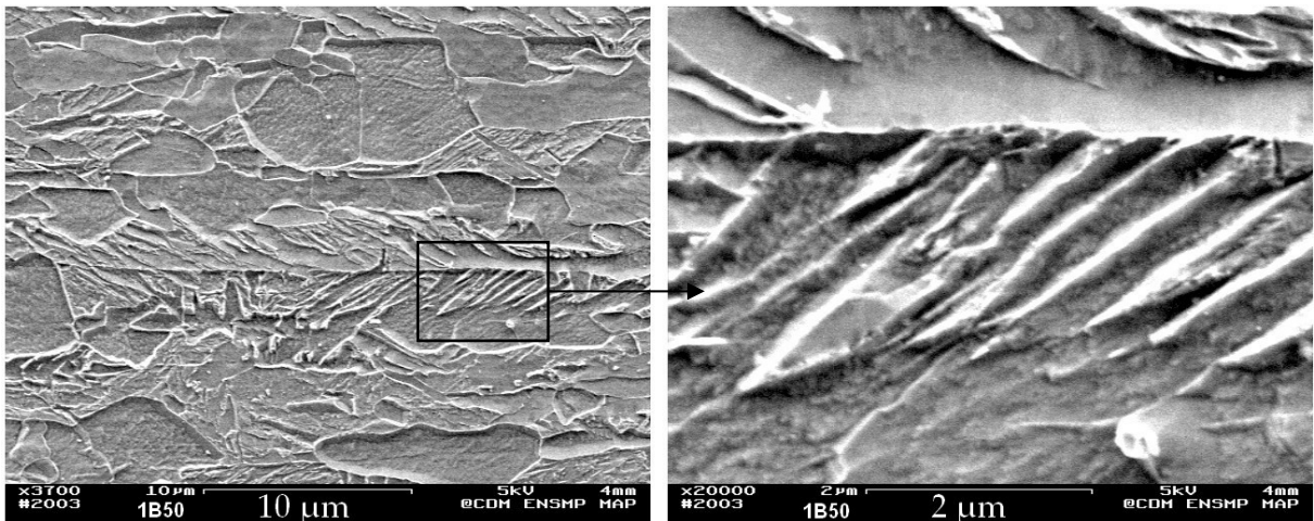
Figure II-6 : Attaque au réactif de Villela, alternance de bandes de 10 µm de large (1B50 - FEG)
