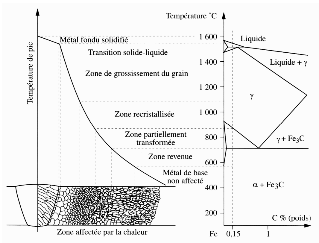
Figure I-28 : Présentation schématique des différentes parties constitutives d'un joint soudé, [BLON01] d'après [EAST83]
