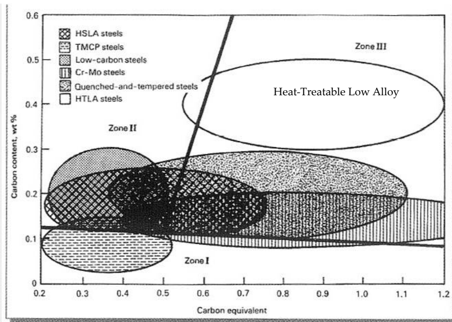
Figure I-6 : Diagramme de Graville donnant la soudabilité de l'acier en fonction de la quantité de carbone et du carbone équivalent CE IIV , [LIU-02-PDC]
