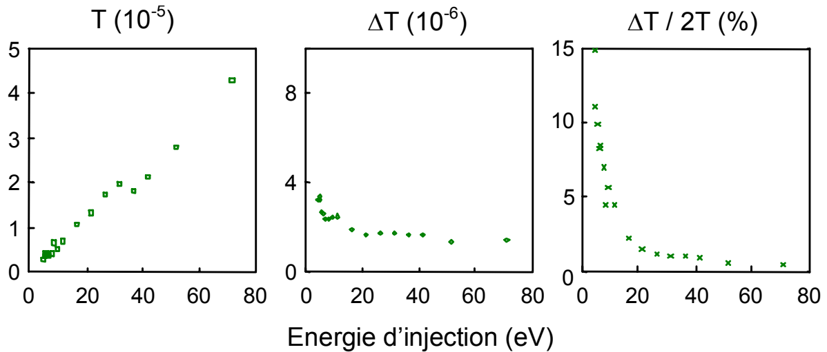
Figures I. 3 : D'après la référence 24. Transmission T, dépendance en spin de la transmission \Delta T et asymétrie A en fonction de E_p . Les surfaces d'or d'entrée et de sortie sont propres : il n'y a donc pas ici de mesure possible pour E_p < \Phi_{Au} = 4 eV.
