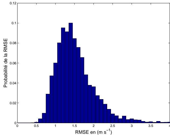
FIG. 6.7 – Distribution des RMSE. RMSE globale de 1,6 \text{ m s}^{-1} . 85 % des RMSE sont au dessous de 2 \text{ m s}^{-1} . L'histogramme est tracé avec des intervalles de 0,1 \text{ m s}^{-1} pour les RMSE.
