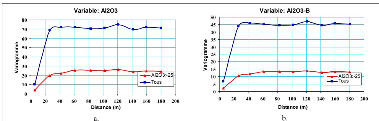
figure V.21 Variogramme d'alumine calcinée (a) et d'alumine brute (b) dans la nouvelle géométrie décompactée et mise à l'horizontale en utilisant deux surfaces qui englobent le gisement de BDR
