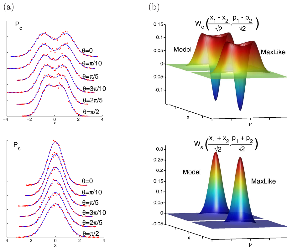
Figure 7.8: Tomographie d'un état produit avec 1,8 dB de squeezing et une réflectivité R = 5\% : (a) Distributions de quadratures mesurées, interpolées à l'aide de notre modèle. (b) Fonctions de Wigner des corrélations ( W_- = W_c ) et des anticorrélations ( W_+ = W_s ), corrigées des pertes homodynes, obtenues par maximum de vraisemblance et comparées au résultat du modèle.
