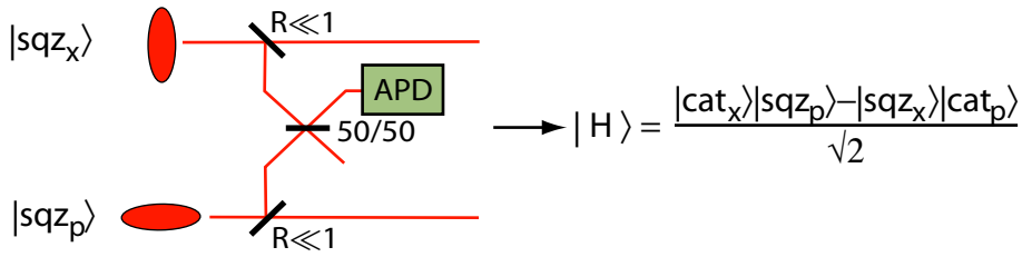
Figure 8.1: Préparations d'états "Hamlet" par soustraction cohérente d'un photon depuis deux impulsions indépendantes de vide comprimé.
