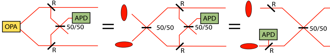
Figure 7.5: Soustraction cohérente de photons d'un état intriqué gaussien : l'état préparé avec notre dispositif peut être obtenu de manière équivalente en mélangeant un “chaton de Schrödinger” avec un mode de vide comprimé orthogonalement.
