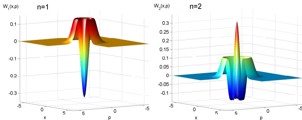
Figure 4.9: Fonctions de Wigner idéales d'états de Fock à un et deux photons.
