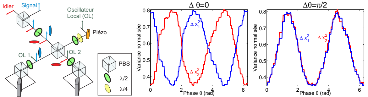
Figure 4.3: Mesure du déphasage relatif \Delta\theta entre les quadratures mesurées par les deux détections homodynes. L'interférence entre deux modes intriqués gaussiens produit deux états orthogonalement comprimés. Le déphasage relatif \phi entre les variances \Delta x_1^2 et \Delta x_2^2 donne \Delta\theta = \frac{\pi - \phi}{2} . La variance du shot noise est normalisée à 1/2.
