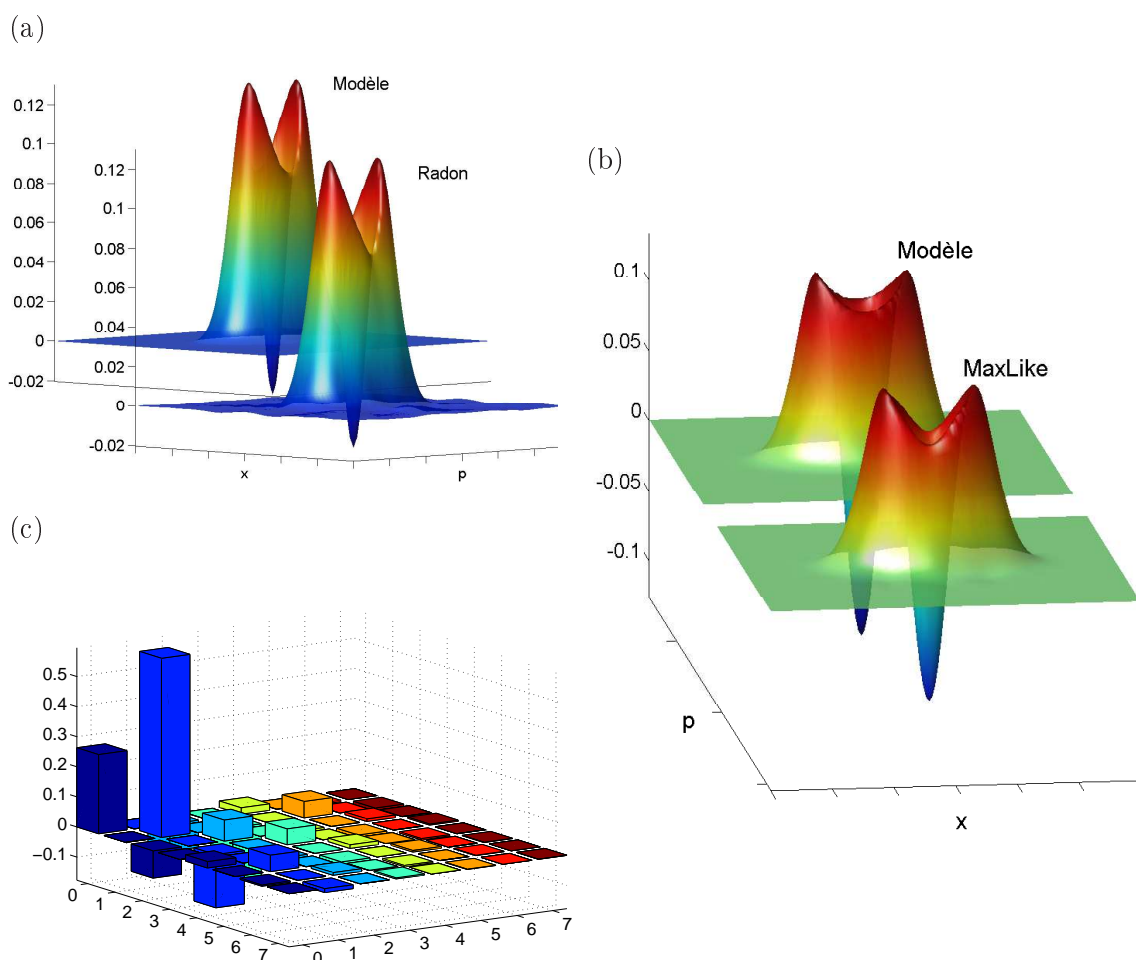
Figure 5.9: (a) Fonction de Wigner de l’état mesuré reconstruite par transformée de Radon inverse, comparée à celle obtenue à partir du modèle. (b) Fonction de Wigner de l’état généré dans l’expérience, corrigée des pertes homodynes, reconstruite par maximum de vraisemblance et comparée au résultat du modèle. (c) Matrice densité en base de Fock de l’état généré dans l’expérience, corrigé des pertes homodynes, reconstruite par maximum de vraisemblance.
