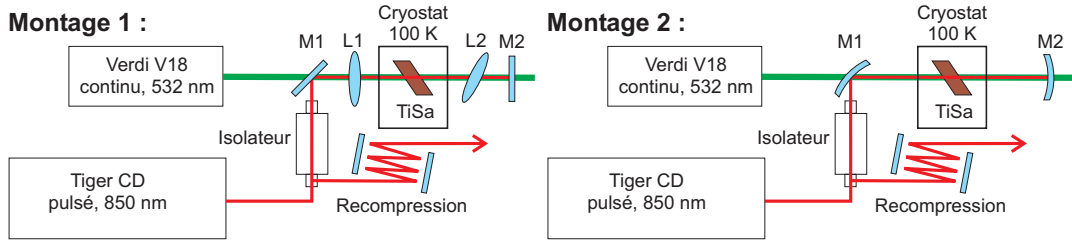
Figure 3.7: Schémas de l'amplificateur cryogénique double passage (Montage 1 utilisé pour les tests, Montage 2 pour l'implémentation finale).
