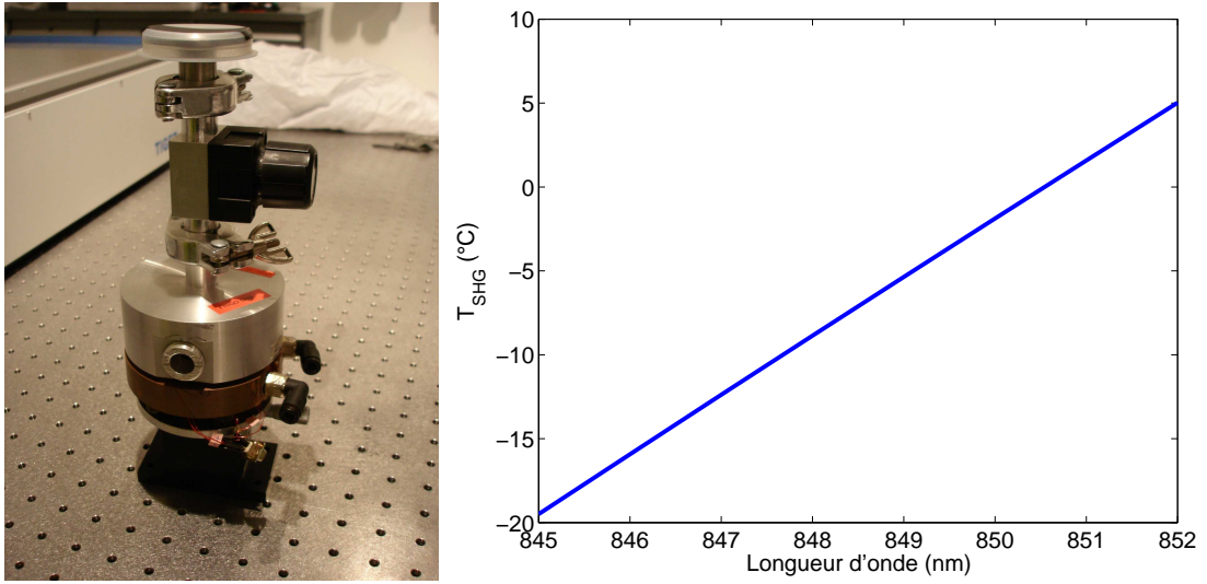
Figure 3.10: Enceintes à vide contenant les cristaux de \text{KNbO}_3 , et température d'accord de phase en fonction de la longueur d'onde (données de [68]).
