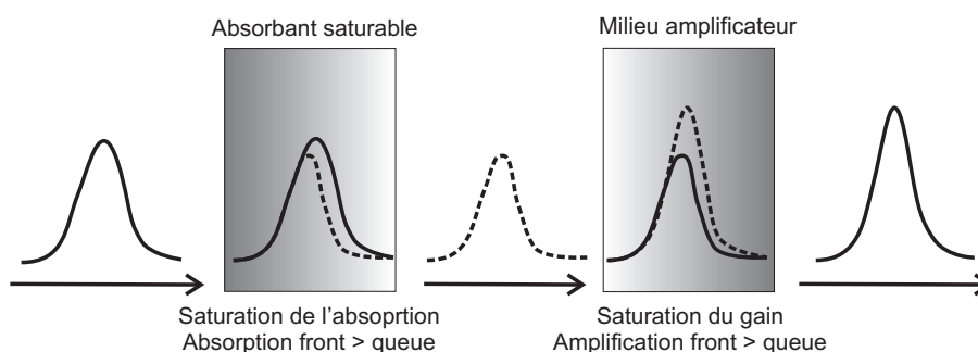
Figure 3.2: Amplification et rétrécissement temporel d'une impulsion dans un laser verrouillé par un absorbant saturable.
