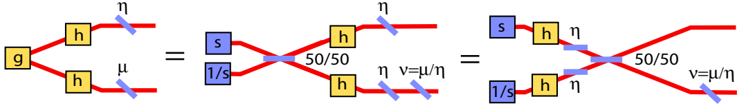
Figure 4.11: Modélisation du bruit OPA et des pertes en ligne. Pour simplifier les calculs, on suppose que l'état intriqué initial est créé non pas avec un OPA non-dégénéré avec un gain g mais par interférence de deux vides comprimés monomodes produits par deux OPAs dégénérés avec des facteurs de compression s et 1/s . On peut alors faire “remonter” avant cette séparatrice le bruit OPA, ajouté par deux amplificateurs non-dégénérés avec des gains h . Il en est de même pour les pertes homodynes (lame de transmission \eta ), en divisant en deux parties les pertes APD \mu = \eta\nu .
