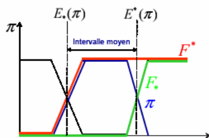
Figure 135 : Exemple de F^* , F_* , E^* , et E_*
