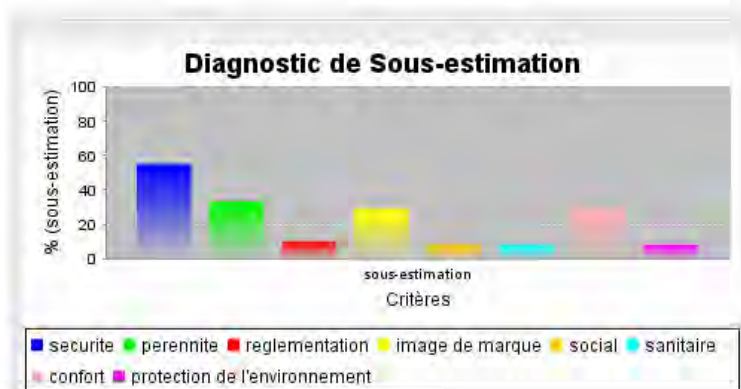
Figure 128 : analyse du risque d'erreur d'évaluation global (au maximum 2 erreurs)
