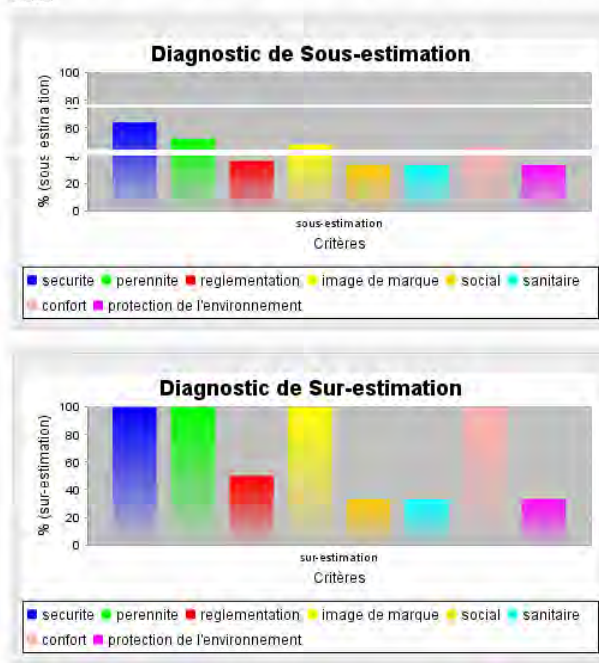
Figure 127 : analyse du risque d'erreur d'évaluation global
