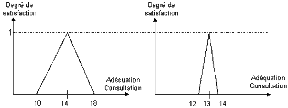
Figure 68 : exemple de scores flous pour deux prestataires concurrents
