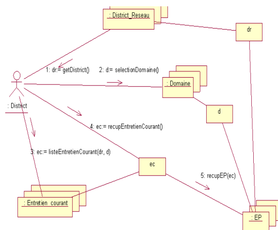
Figure 26 : consulter une fiche entretien courant
