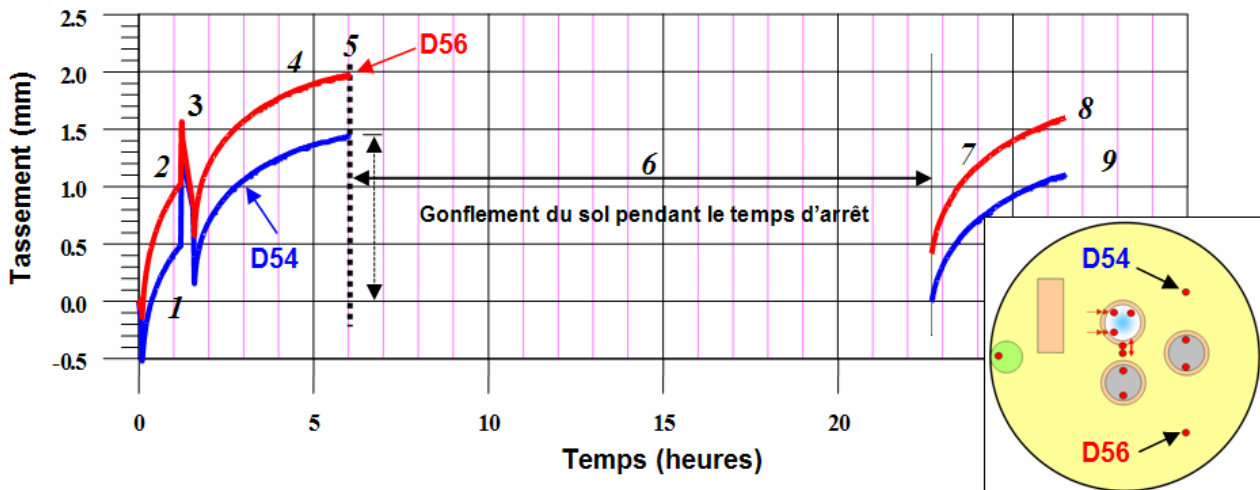
(b) Tassements de la superstructure
