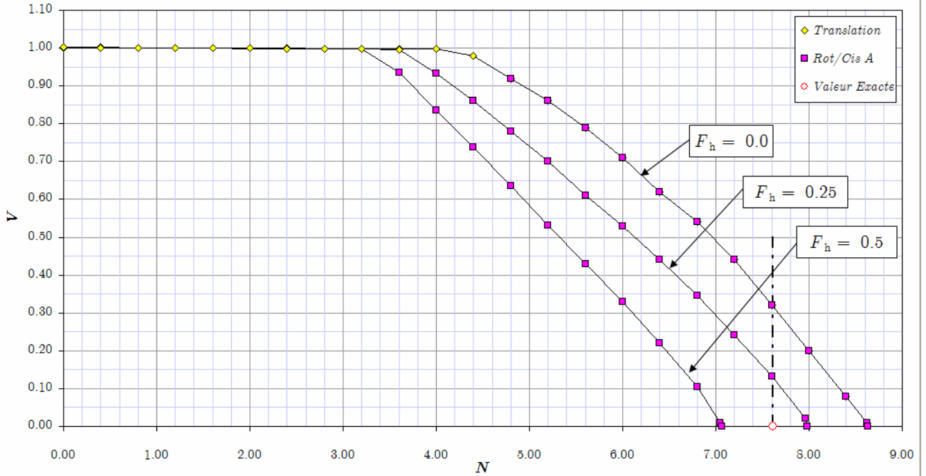
k=1 , Diagramme d'interaction V-N
