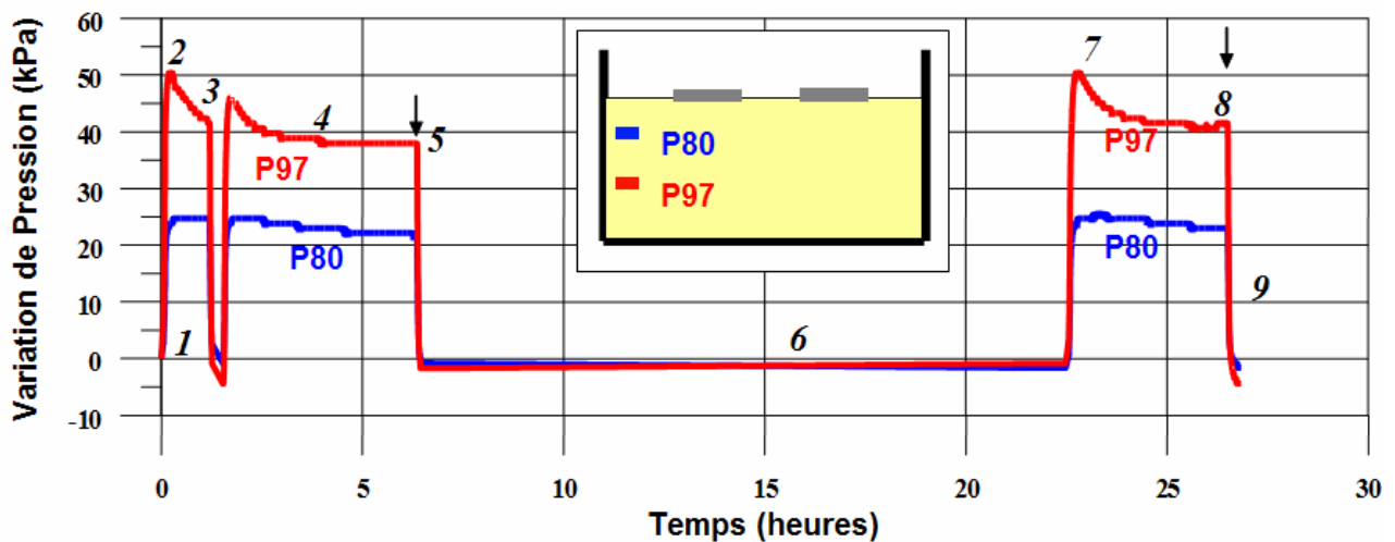
Figure 3.15 – Deuxième séance d'essais. Résultats pertinents pour la consolidation du sol. 1. Montée à 40g. 2. Phase de consolidation. 3. Problème rencontré – arrêt. 4. Reprise de la phase de consolidation. 5. Premier essai sous force horizontale, essai sous force verticale. 6. Arrêt – préparation du deuxième essai. 7. Deuxième phase de consolidation. 8. Deuxième essai sous force horizontale. 9. Arrêt définitif.
