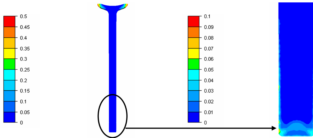
Figure 5.21 : Critère de Latham et Cockroft normalisé (OP3 - lopin de diamètre 13 mm)
