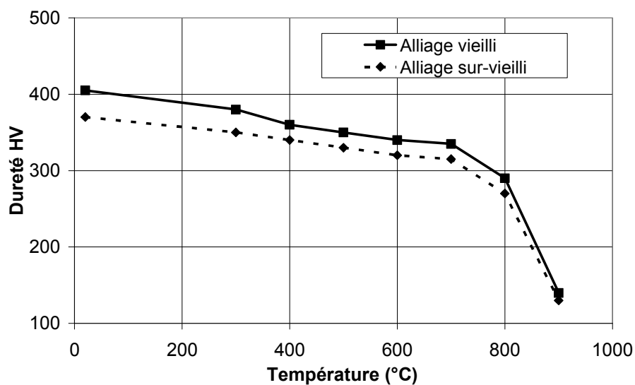
Figure 2.17 : Dureté à chaud de l'alliage NCF2415C [UET 1 ]
