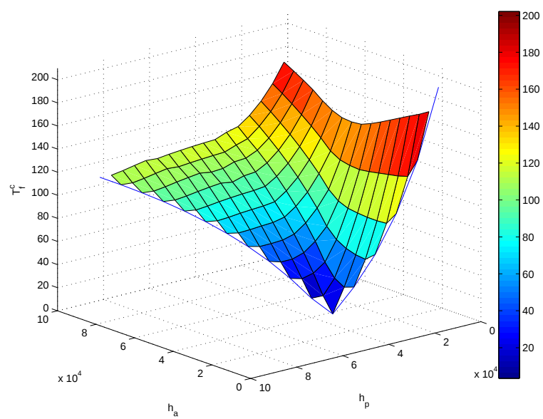
FIG. 5.15 – Temps T_f^c (en jours)
