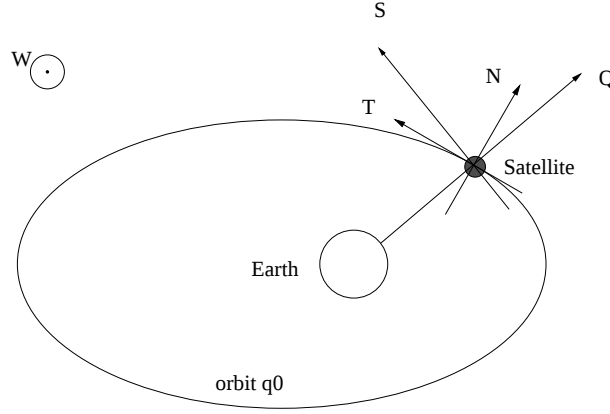
FIG. 1.2 – Les repères othonormés QSW et NTW
