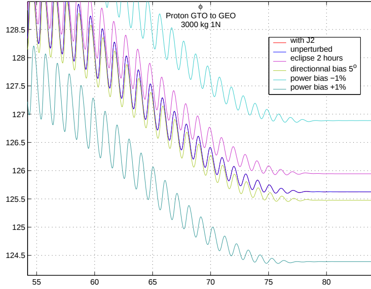
FIG. 6.3 – Sensibilité du déphasage \phi à diverses perturbations sur un transfert GTO-GEO
