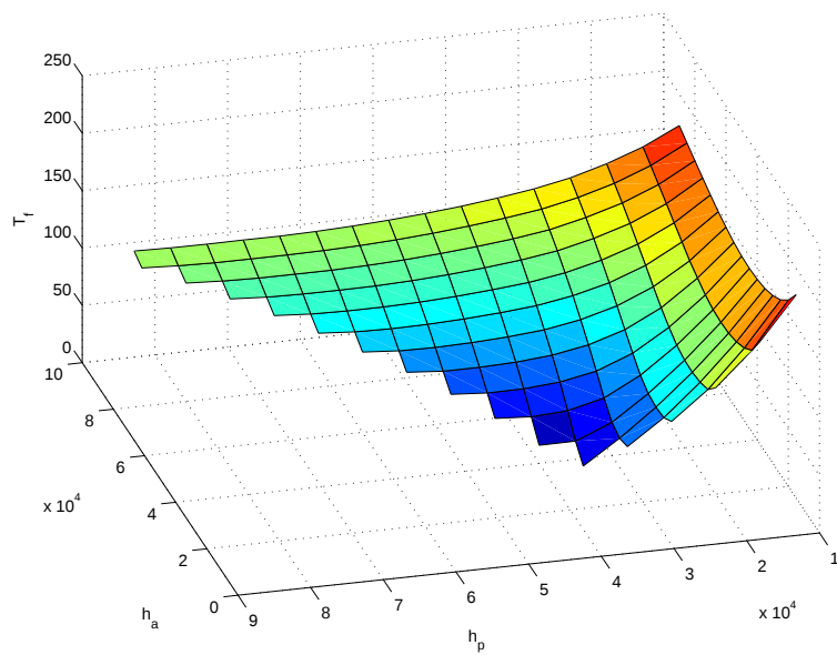
FIG. 5.8 – Temps de transfert de la meilleurs interpolation en fonction de l'orbite initiale.
