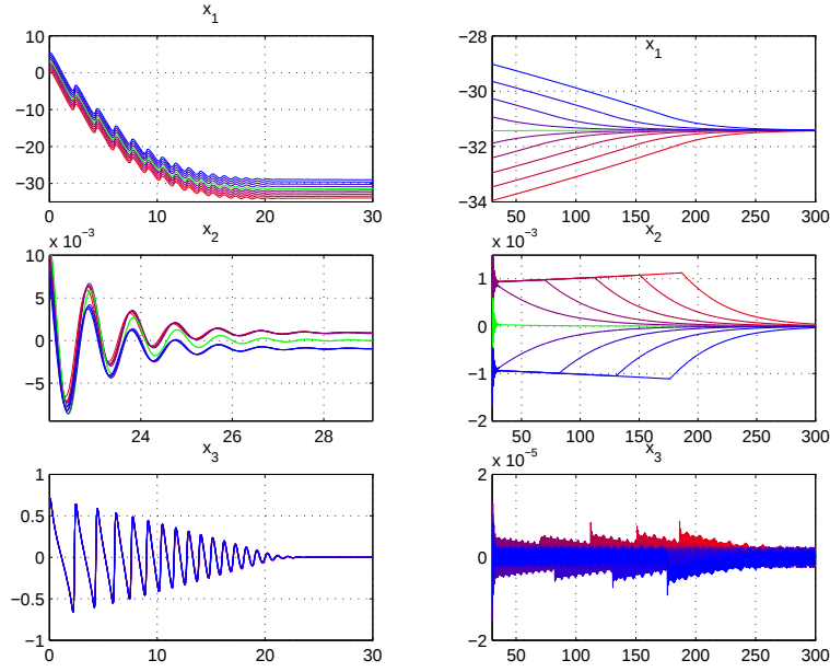
FIG. 6.1 – Sensibilité du feedback Kellett Praly à la longitude initiale
