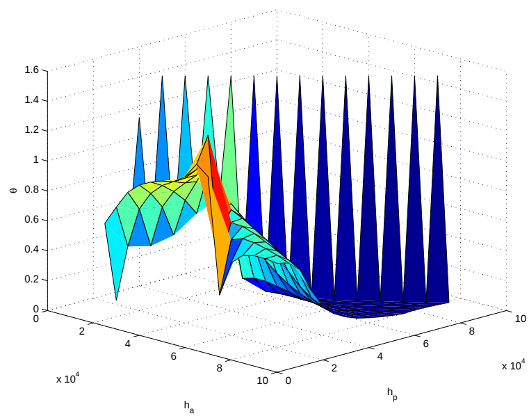
FIG. 5.10 – Meilleur interpolation de Lyapunov
