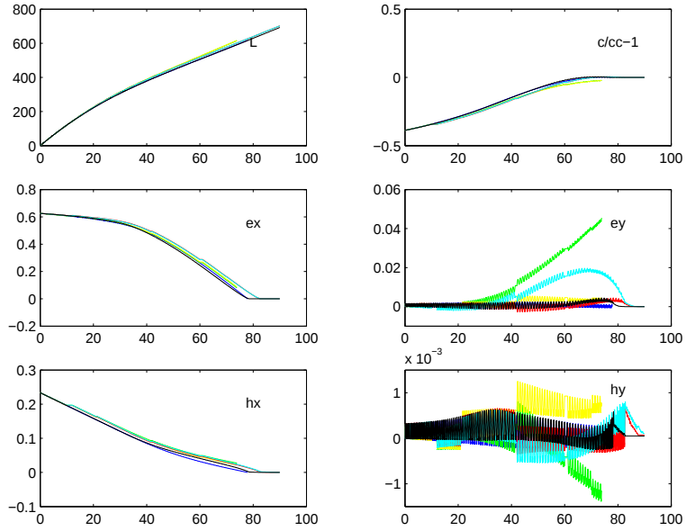
FIG. 5.4 – Contrôle optimal contre contrôle stabilisant, un transfert Proton-GTO vers GEO, masse initiale 3000kg, module maximal de poussée 1N
