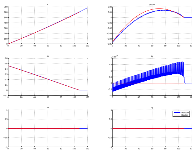
FIG. 5.12 – Evolution des paramètres orbitaux pour le transfert ha=60000 hp=20000
