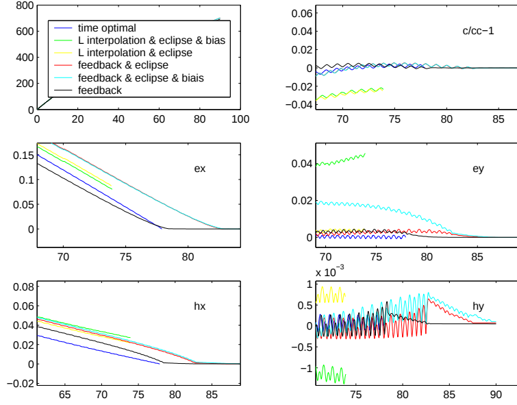
FIG. 5.3 – Contrôle optimal contre contrôle stabilisant, un transfert Proton-GTO vers GEO, masse initiale 3000kg, module maximal de poussée 1N, détail de la fin
