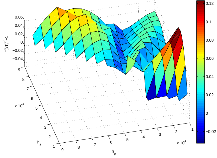
FIG. 5.16 – Erreur relative \frac{T_f^c}{T_f^{ref}} - 1
