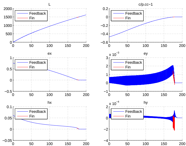
FIG. 5.1 – Evolution des paramètres orbitaux pour le transfert 1
