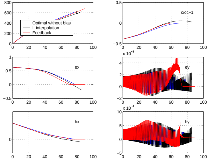
FIG. 5.5 – Biais sur le module maximal de poussée de +10%, Proton GTO vers GEO, 3000kg 1N
