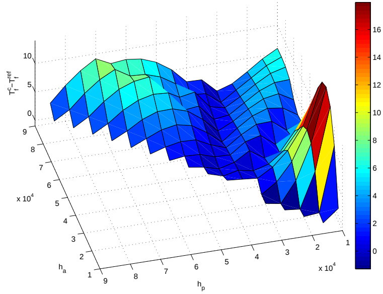
FIG. 5.17 – Erreur absolue T_f^c - T_f^{ref}
