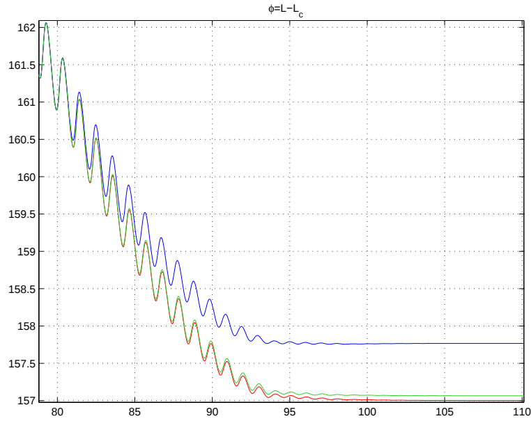
FIG. 6.4 – Synchronisation par changement de condition initiale
