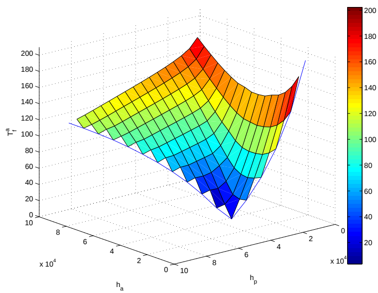
FIG. 5.19 – Temps T_f^a (en jours)
