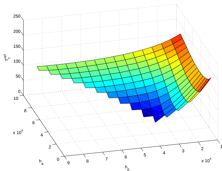
FIG. 5.7 – Temps de référence calculé avec MIPELEC
