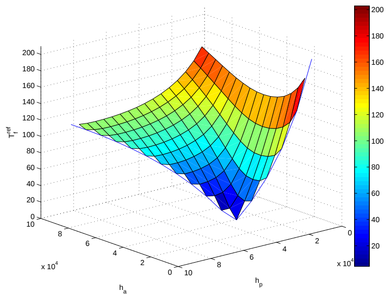
FIG. 5.14 – Temps de référence T_f^{ref} (en jours)
