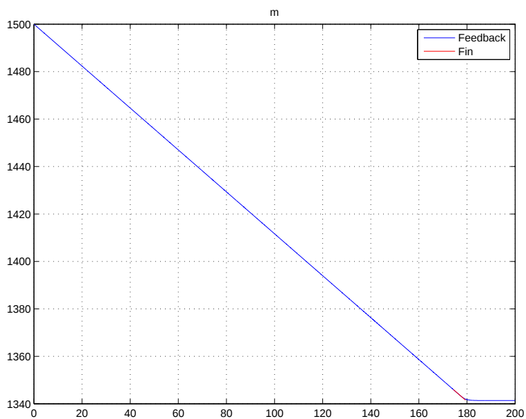
FIG. 5.2 – Evolution de la masse pour le transfert 1
