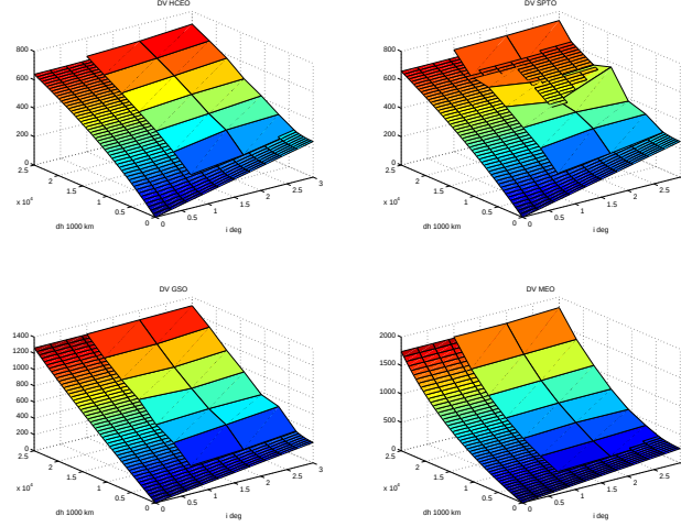
FIG. 5.23 – \Delta V : grille fine transferts optimaux, grille large algorithme naïf \Phi .
