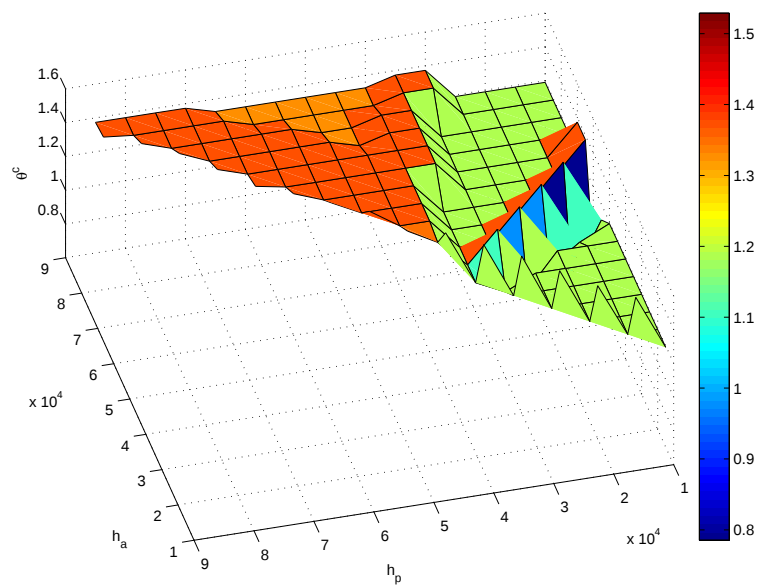
FIG. 5.18 – L'argument de l'optimisation naïve : \theta_c
