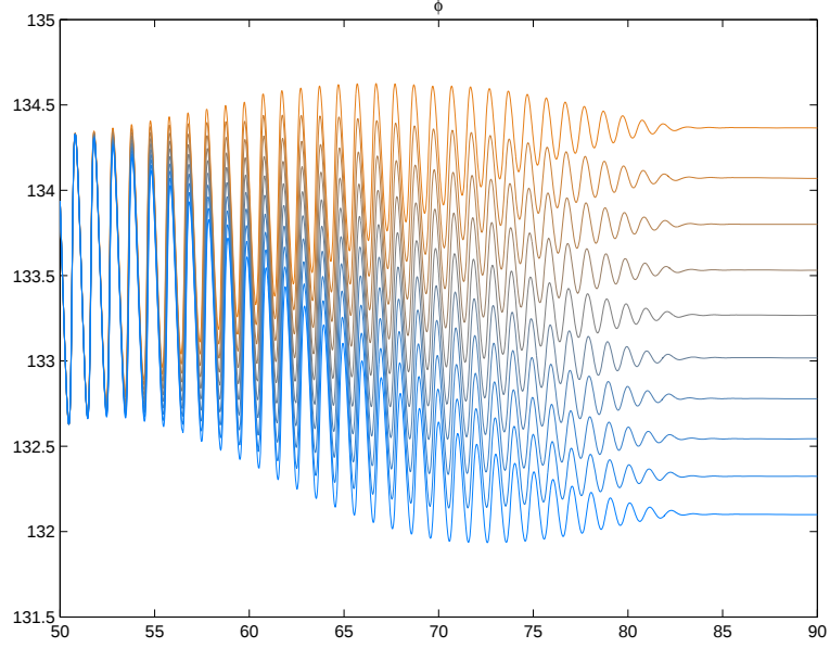
FIG. 6.5 – Sensibilité du déphasage \phi au paramètre k_a
