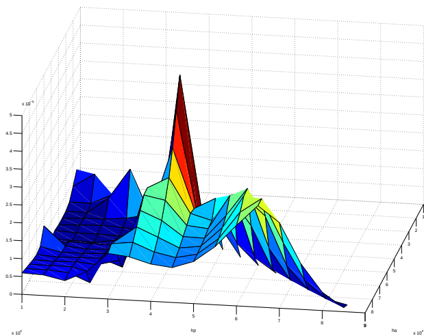
FIG. 5.11 – Le coût d'interpolation
