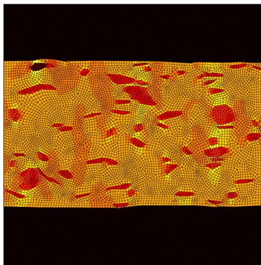
FIG. 4.20 – Répartition des contraintes de von Mises à la suite d'un refroidissement de 180 \text{ } ^\circ\text{C} à 20 \text{ } ^\circ\text{C} . Plus la couleur est foncée, plus le domaine concerné est sollicité.
