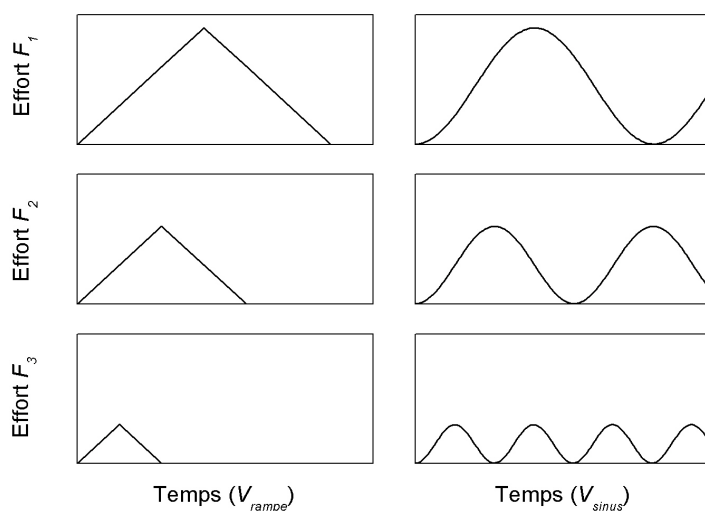
FIG. 8.2 – La vitesse de charge maximale induite par le signal sinusoïdale est maintenue constante.
