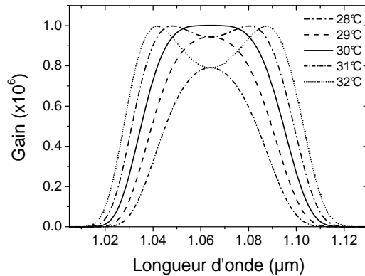
FIG. 3.2 – Courbes de gain dans le PPKTP pour différentes températures. La période de retournement du cristal est de 6,739 \mu\text{m} .
