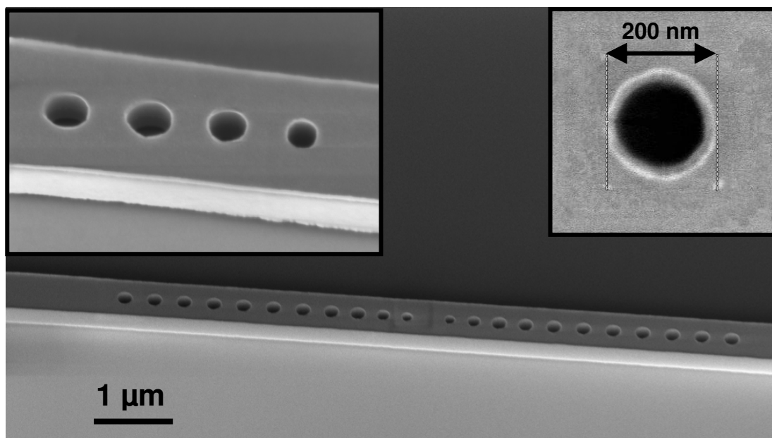
Figure 29 - Photo MEB d’une cavité après fabrication. En insert, détail de 4 trous fabriqués à gauche et détails d’un trou de 200 nm vue de dessus.
