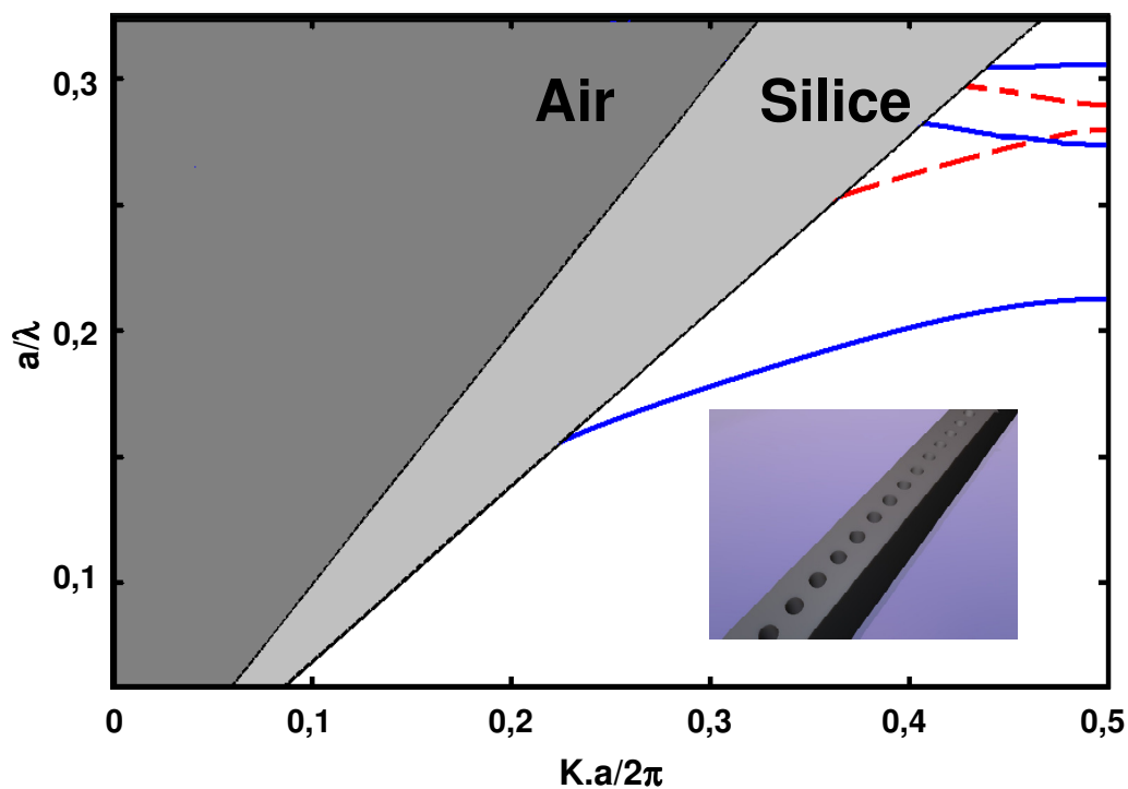
Figure 12 - Diagramme de bande ou de dispersion d'un réseau de trous périodique de période 370 nm et de 180 nm de diamètre le long d'un guide ruban. En bleu le mode fondamental et en pointillé rouge le second mode possédant une symétrie différente.
