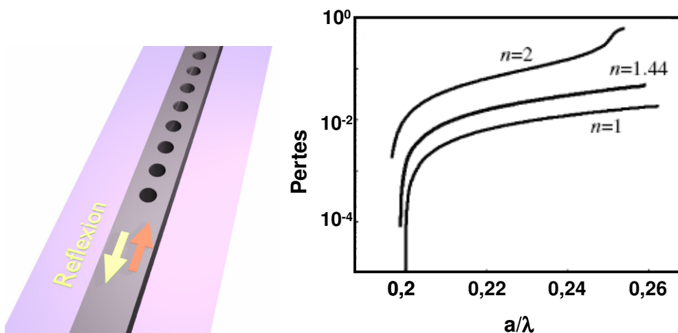
Figure 14 - A gauche, schéma d'un miroir semi-infini composé de trous de diamètre 180 nm et espacés d'une période de 370 nm dans un guide ruban de 520 nm de large sur 340 nm de hauteur. A droite, graphique des pertes calculées pour un miroir semi-infini avec différents substrats d'indice n ( \lambda=1,6 \mu\text{m} ).
