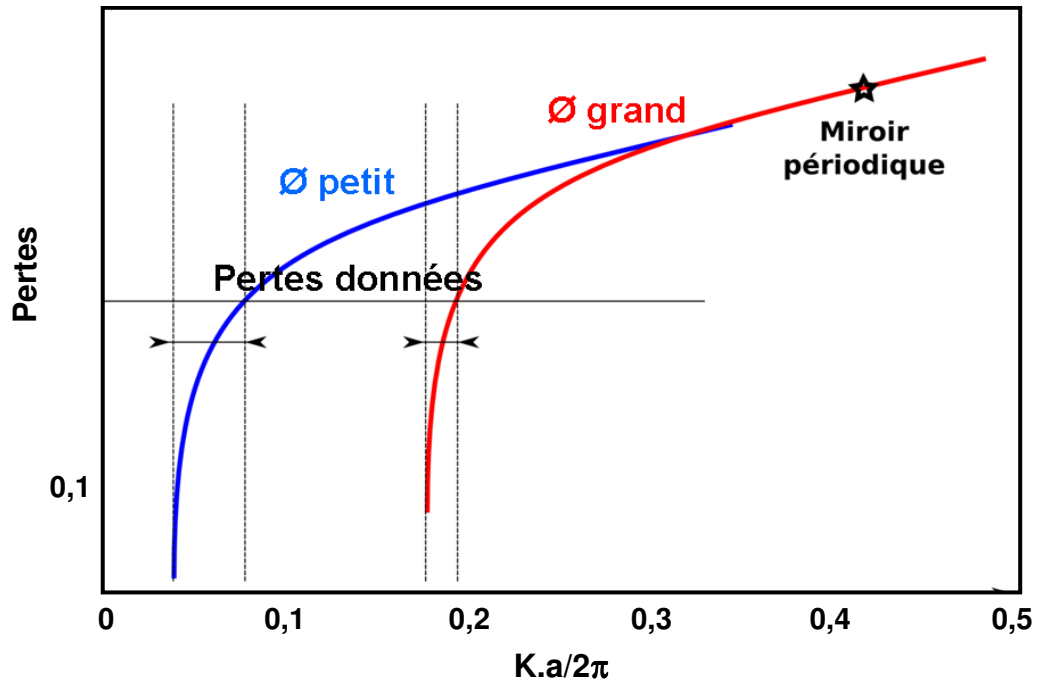
Figure 16 - Schéma illustrant l'intervalle opérationnel de longueur d'onde pour deux diamètres différents pour une valeur de pertes données.
