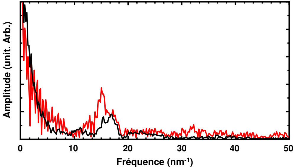
Figure 49 - Transformée de Fourier en amplitude des spectres de la Figure 48.
