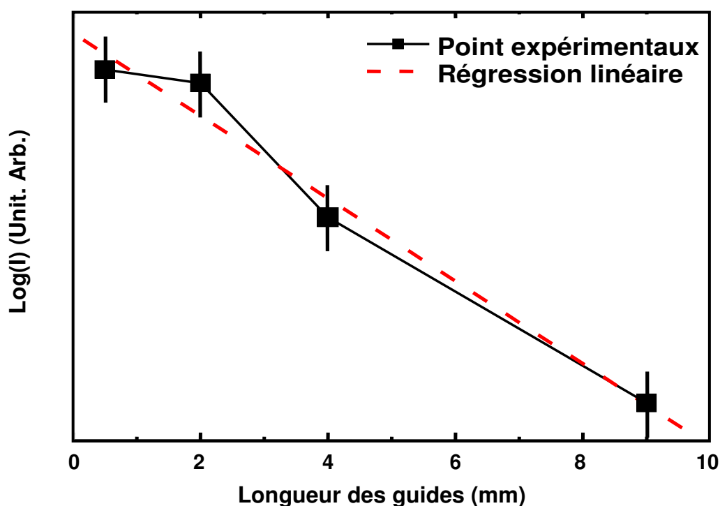
Figure 32 - Intensités transmises pour différentes longueurs du guide à une longueur d'onde 1550 nm pour un guide 450 nm de large. En noir, les points expérimentaux. En pointillé rouge, la régression linéaire. Ici la pente est de 6 dB/cm.
