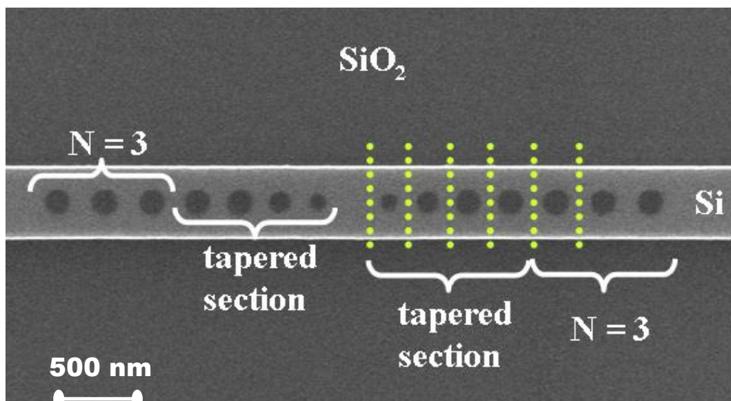
Figure 40 - Photo MEB d'une cavité avec N=3 trous dans la partie périodique des miroirs.
