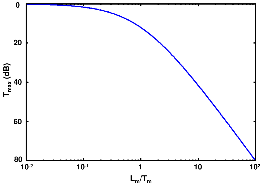
Figure 8 - Transmission maximum d'une cavité en fonction du rapport entre les pertes L_m et la transmission T_m des miroirs.
