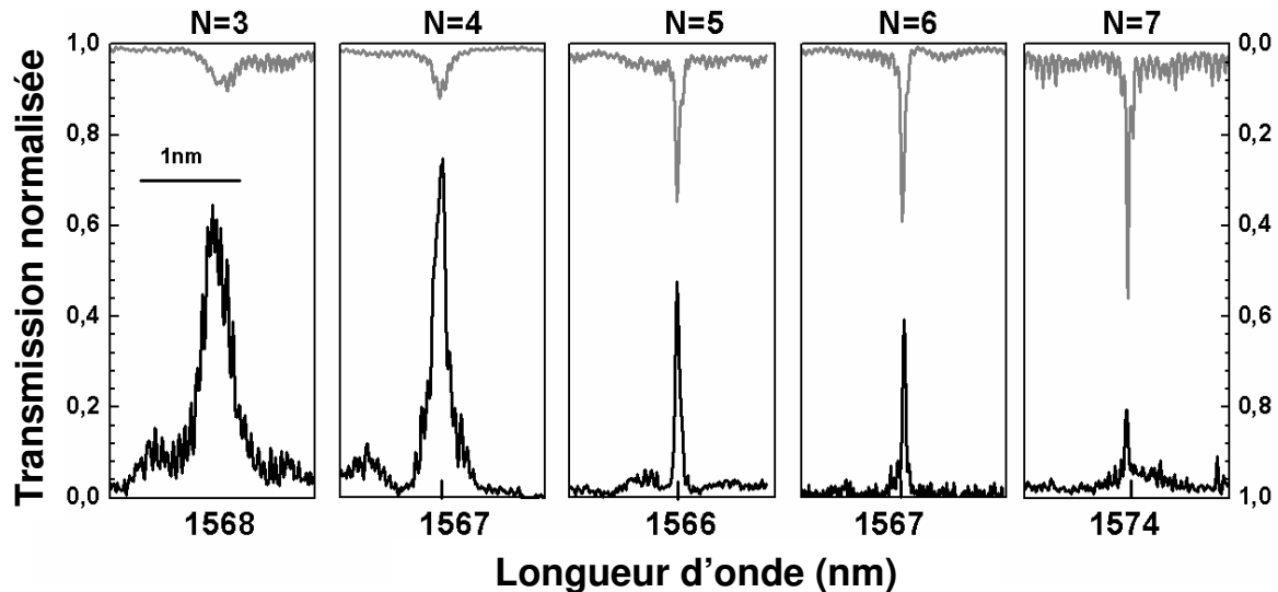
Figure 60 – Spectres obtenus en mesurant par-dessus (axe inversé) et spectres en transmission (axe normal) pour les différents N considérés.
