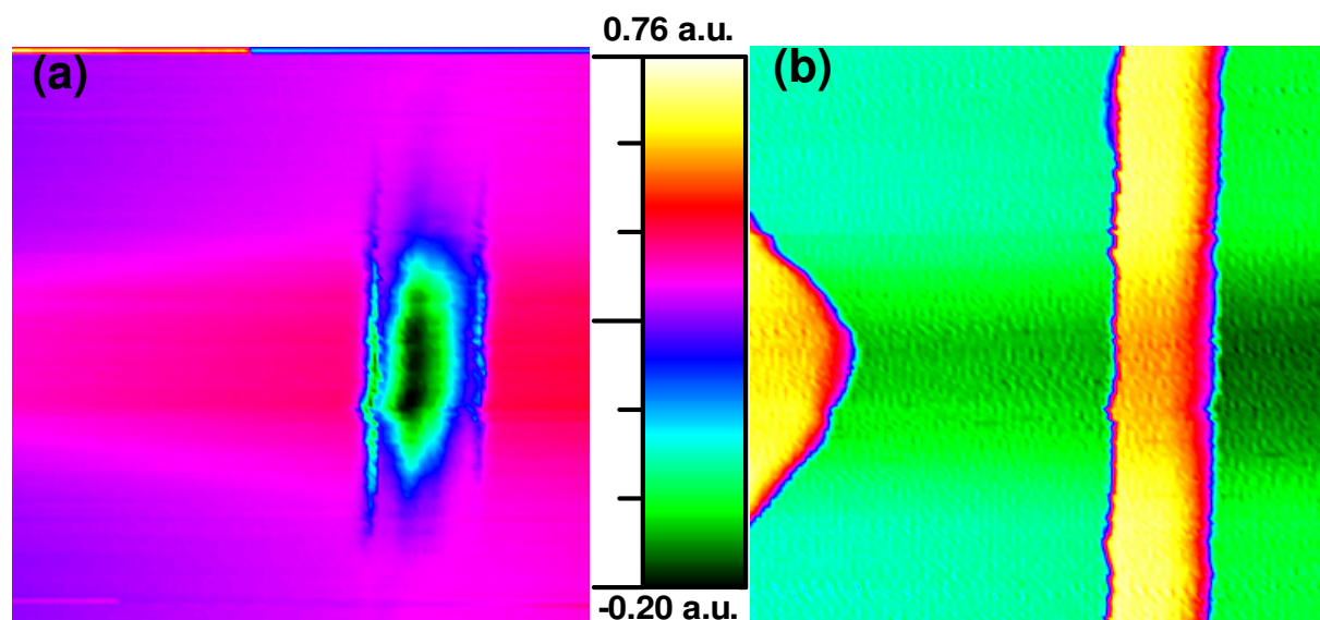
Figure 88 – (a) cartographie de la transmission transmise en fonction de la position de la pointe au-dessus de la cavité. (b) Image topographique de la structure.
