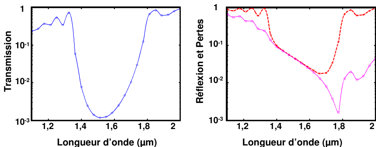
Figure 39 – A gauche, la transmission et à droite les pertes (ligne continue) et 1-R (ligne pointillé) pour un miroir à N=7.
