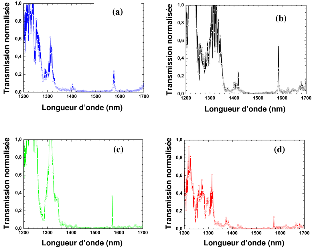
Figure 44 - Spectre en transmission des cavités adaptées avec un nombre croissant de trous périodiques dans le miroir. (a) N=1, (b) N=2, (c) N=3, (d) N=4.
