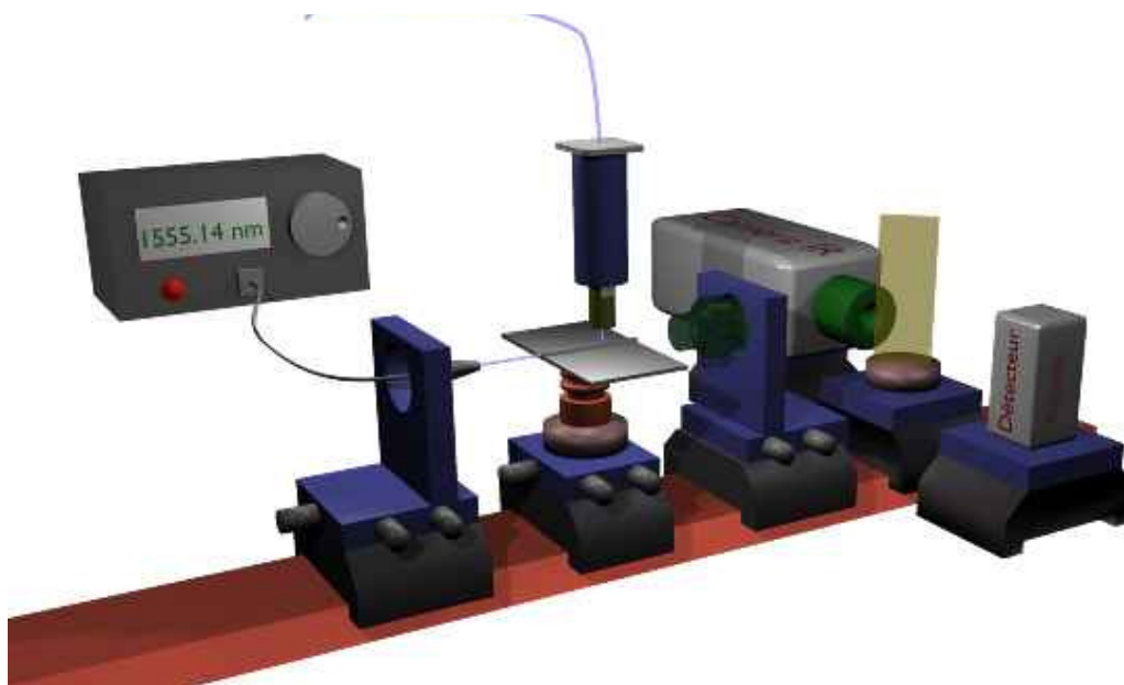
Figure 69 - Schéma du banc de transmission couplé avec un SNOM.
