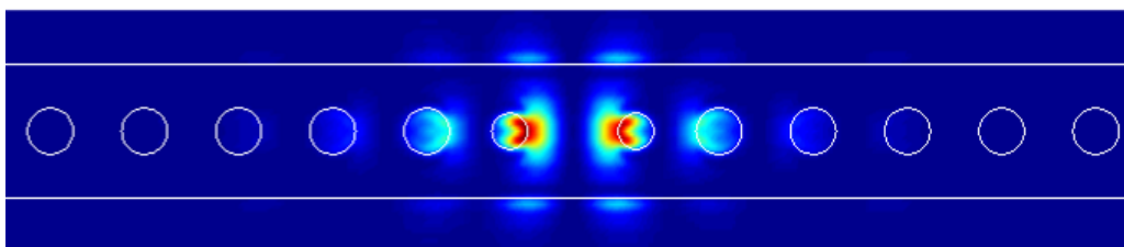
Figure 71 - Calcul 3D du champ à la surface d'une micro-cavité.
