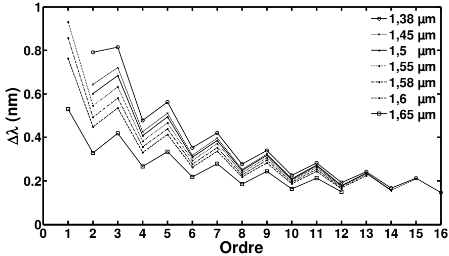
Figure 81 - Evolution du décalage en longueur d'onde en fonction de l'ordre de la cavité pour différentes longueurs d'onde de résonance avec une pointe en silice de dimension 0,4 \mu\text{m} .
