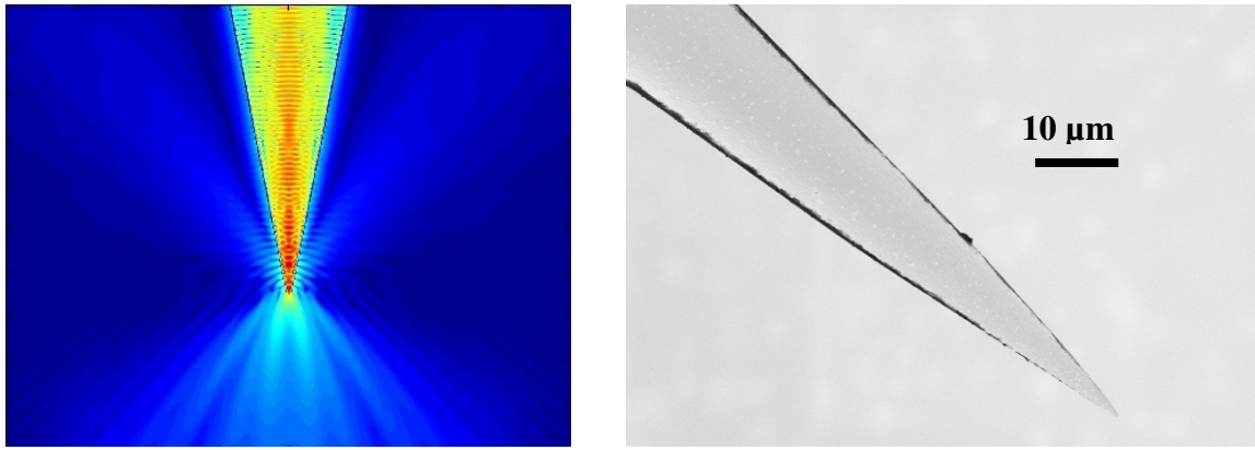
Figure 46 - À gauche, calcul du champ dans une pointe en silice tirée des travaux de Fadi Baida. À droite, photo MEB d'une pointe en silice réalisée par attaque chimique
