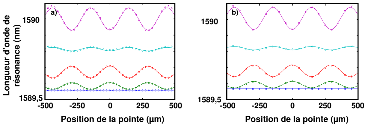
Figure 83 - Longueur d'onde de résonance en fonction de la position de la pointe pour deux cavités présentant des facteurs de qualité différents. (a) Q=6700 et (b) Q=250000 . Les différentes courbes donnent le décalage pour des dimensions de pointe de 400, 300, 200, 100, 0 nm (courbes de haut en bas). Les courbes en trait plein sont calculées avec le modèle Fabry-Perot et les points avec le calcul vectoriel complet du système cavité-pointe.
