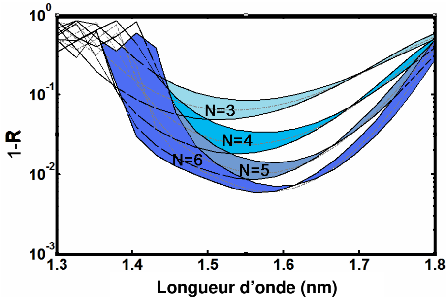
Figure 65 - Evolution de la réflexion ( 1-R sur la figure) d'un miroir optimisé pour le recyclage en fonction du nombre de trous dans la partie périodique du miroir. En pointillé la courbe pour les tailles nominales et en grisée l'intervalle possible pour une incertitude de \pm 10 nm sur les dimensions.
