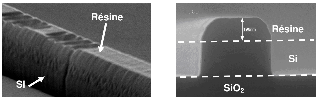
Figure 27 - Photos MEB d'une structure gravée avec le masque de résine dessus. À droite, profil de gravure et hauteur restante de résine.
