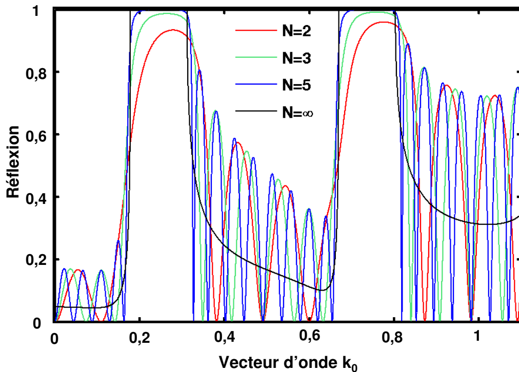
Figure 4 - Réflexion d'un miroir de Bragg quart d'onde (l'épaisseur de chaque couche vaut \lambda/4n ) de période a=0,37 \mu\text{m} comportant 2, 3, 5 et une infinité de paires de silicium ( n=3,48 ) et de silice ( n=1,44 ).
