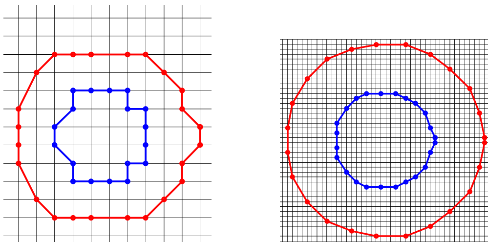
Figure 23 - Cercles de 100 nm (en bleu) et de 200 nm (en rouge) défini sur un maillage de 20 nm (à gauche) et de 5 nm (à droite)
