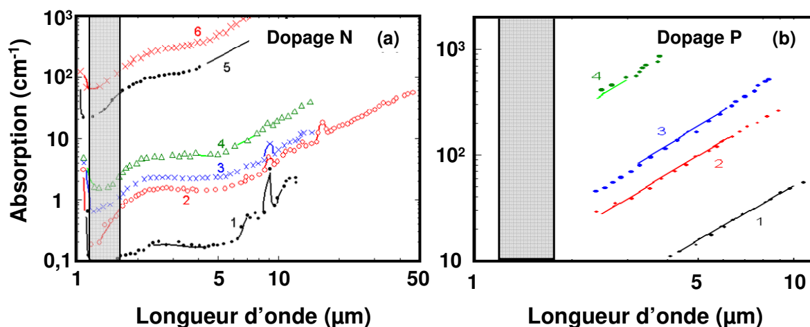
Figure 30- Spectre d'absorption en \text{cm}^{-1} en fonction de la longueur d'onde et du niveau de dopage N du silicium (à gauche) et P (à droite). Les courbes vont du dopage le plus faible ( 1.4 \cdot 10^{16} \text{ cm}^{-3} , courbe 1) vers le dopage le plus élevé ( 1 \cdot 10^{19} \text{ cm}^{-3} , courbe 6). Extrait de (SPI57) (a) et (HAR66) (b). En gris la zone d'intérêt en longueur d'onde autour de 1,55 \mu\text{m} .
