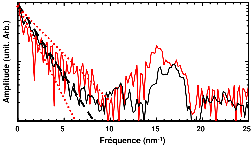
Figure 50 - même courbe que la Figure 49 en échelle logarithmique. En pointillé les régressions linéaires possible pour les deux courbes.
