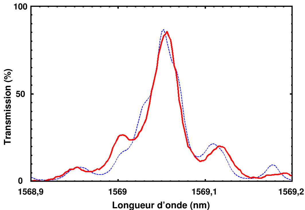
Figure 56 - Comparaison entre le résultat du modèle par ajustement (en pointillé bleu) et la courbe expérimentale (trait continu rouge) pour une cavité avec N=5 . Les résultats de la simulation donnent un facteur de qualité de 20 000 et des longueurs de 5 et 4 mm.
