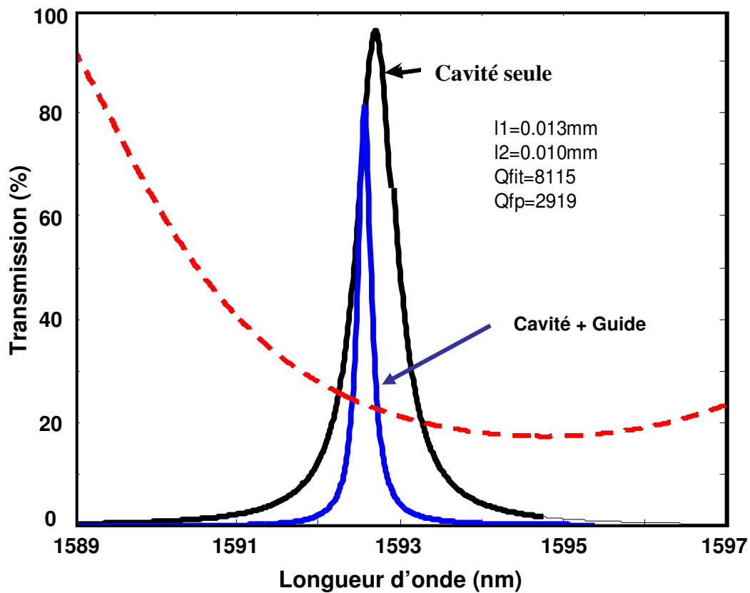
Figure 53 - Comparaison entre le pic de résonance en transmission de la cavité (courbe noire) et celui transmis par le système des trois cavités (courbe bleue). En pointillé rouge, représentation d'une frange Fabry-Perot.
