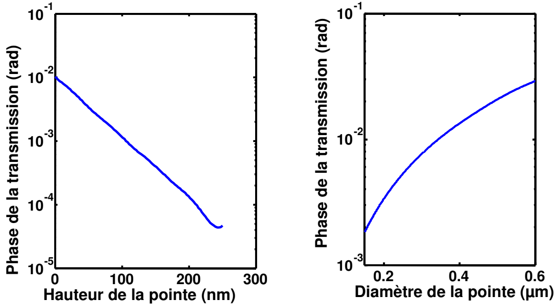
Figure 80 - Evolution de la phase de la transmission (rad) d'une pointe en silice ( n=1,5 ) en fonction de sa hauteur (à gauche) et de sa dimension (à droite).
