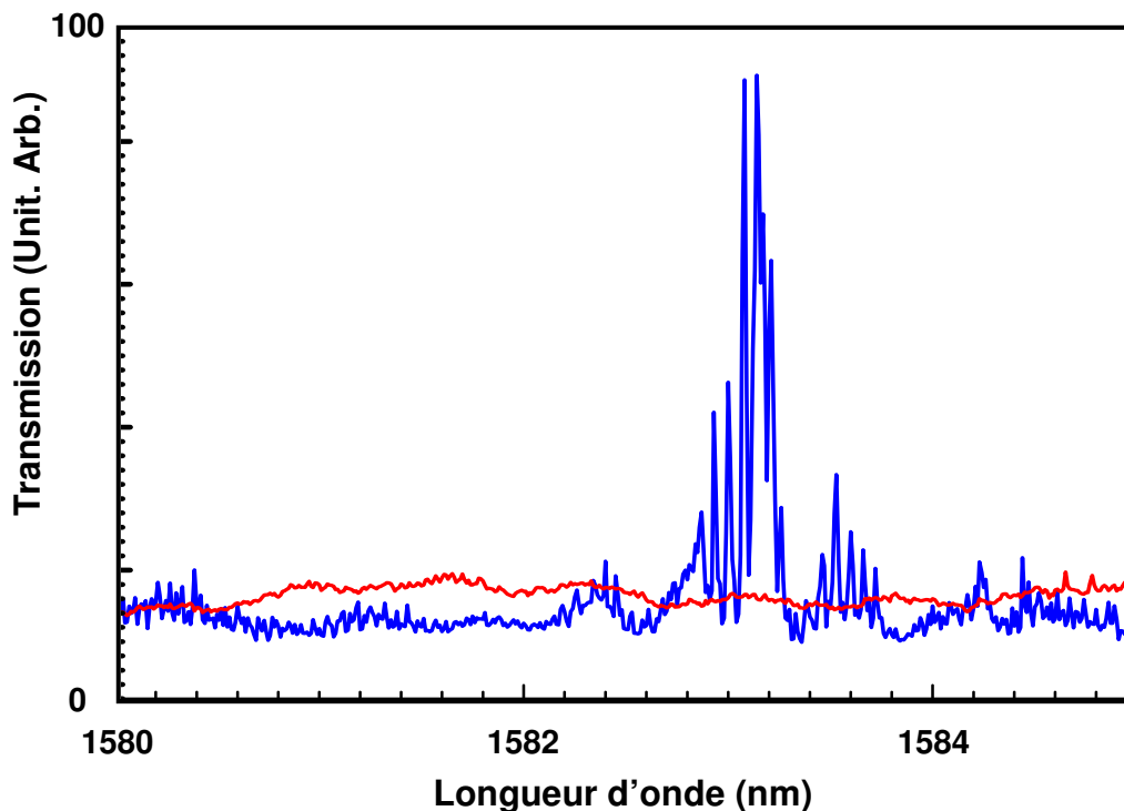
Figure 57 - Spectre du fond continu obtenu en se découplant du guide d'onde en rouge en comparaison d'un spectre en transmission (N=5) en bleu.
