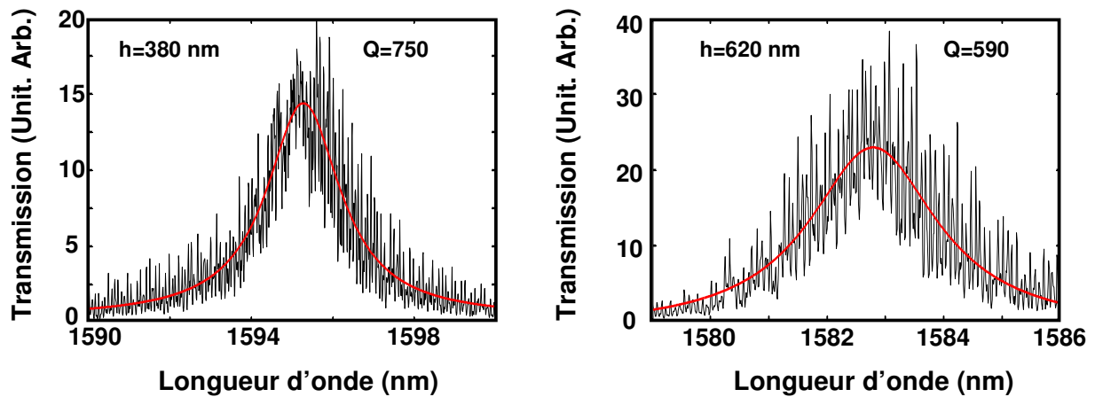
Figure 67 - Spectre en transmission de cavités à recyclage conçues pour le 2 e et le 3 e ordre pour N=4 . L'ajustement (courbe rouge) est effectué par la méthode bicarrée.
