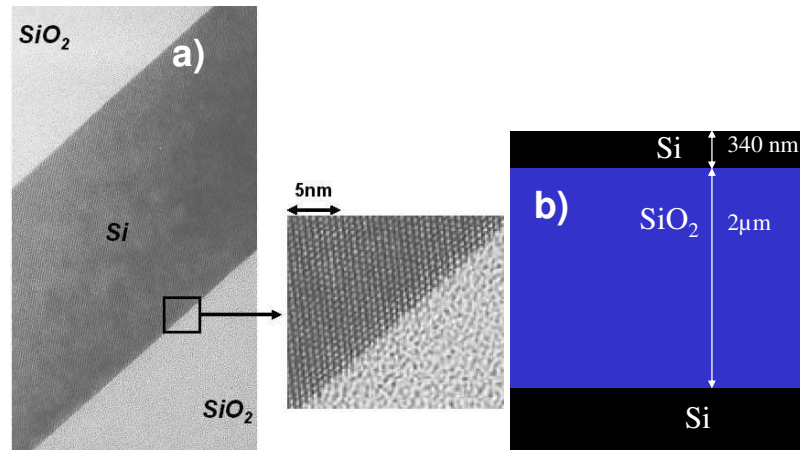
Figure 20 – Une coupe de l’empilement de SOI. (a) photo TEM d’une plaque de SOI commercial. (b) schéma de l’empilement du SOI choisi.
