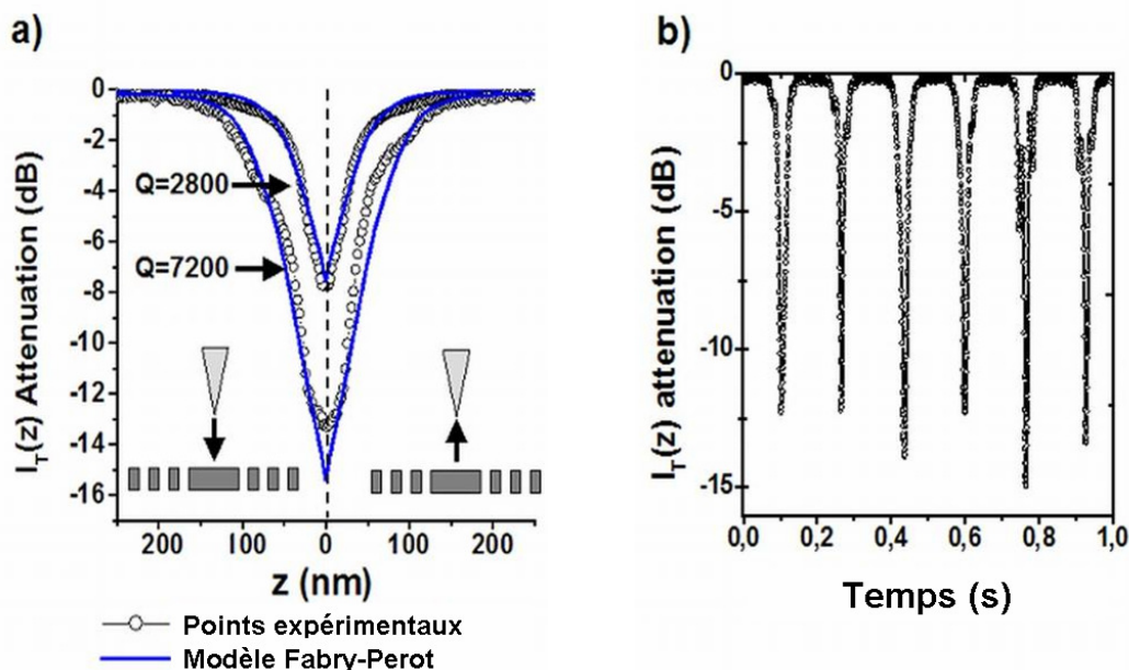
Figure 73 - Evolution de l'intensité transmise à longueur d'onde fixe en fonction de la hauteur de la pointe. a) Confrontation des résultats expérimentaux et du modèle Fabry-Perot développé dans la suite de ce chapitre pour les deux cavités. b) Succession de cycles de descentes et montées de la pointe en fonction du temps.
