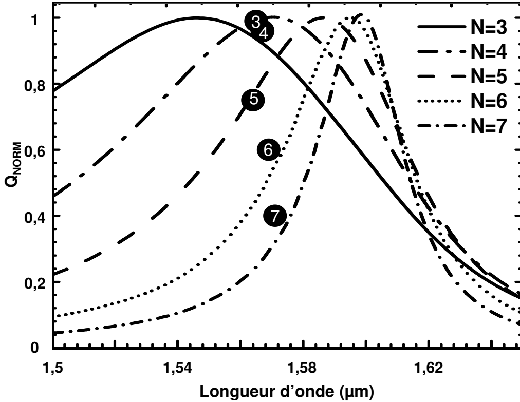
Figure 63 – Evolution du facteur de qualité normalisé ( Q_{NORM}=Q/Q_{max} ) en fonction de la longueur d'onde de résonance pour des cavités avec différents N.
