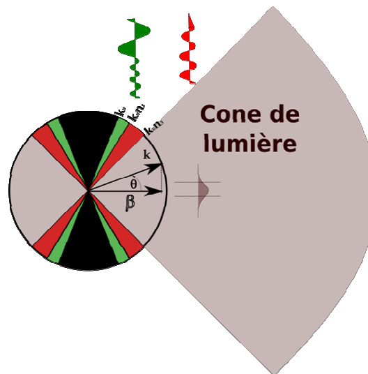
Figure 9 - Schéma illustrant les différents cônes de lumière. En gris le cône de lumière du substrat. En rouge, celui de l'indice n_1 . En vert celui de l'air. Pour chaque zone des profils de champ sont représentés.
