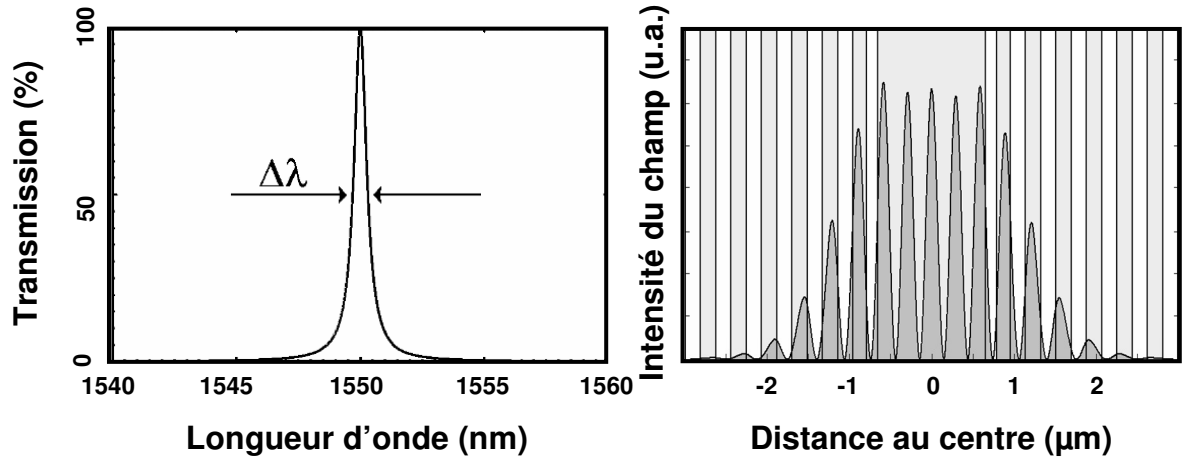
Figure 1 - a) Pic de résonance d'une cavité b) Distribution du champ électrique dans une cavité en fonction de la distance au centre de la cavité
