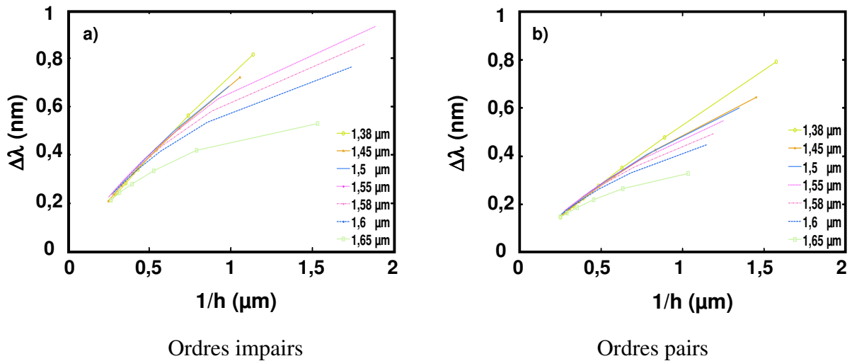
Figure 82 - Evolution du décalage en longueur d'onde ( \Delta\lambda = \lambda - \lambda_0 ) en fonction de la longueur de la cavité (ici 1/h ) pour les ordres impairs (à gauche) et les ordres pairs (à droite) pour différentes longueurs d'onde de résonance avec une pointe en silice de dimension 0,4 \mu\text{m} .
