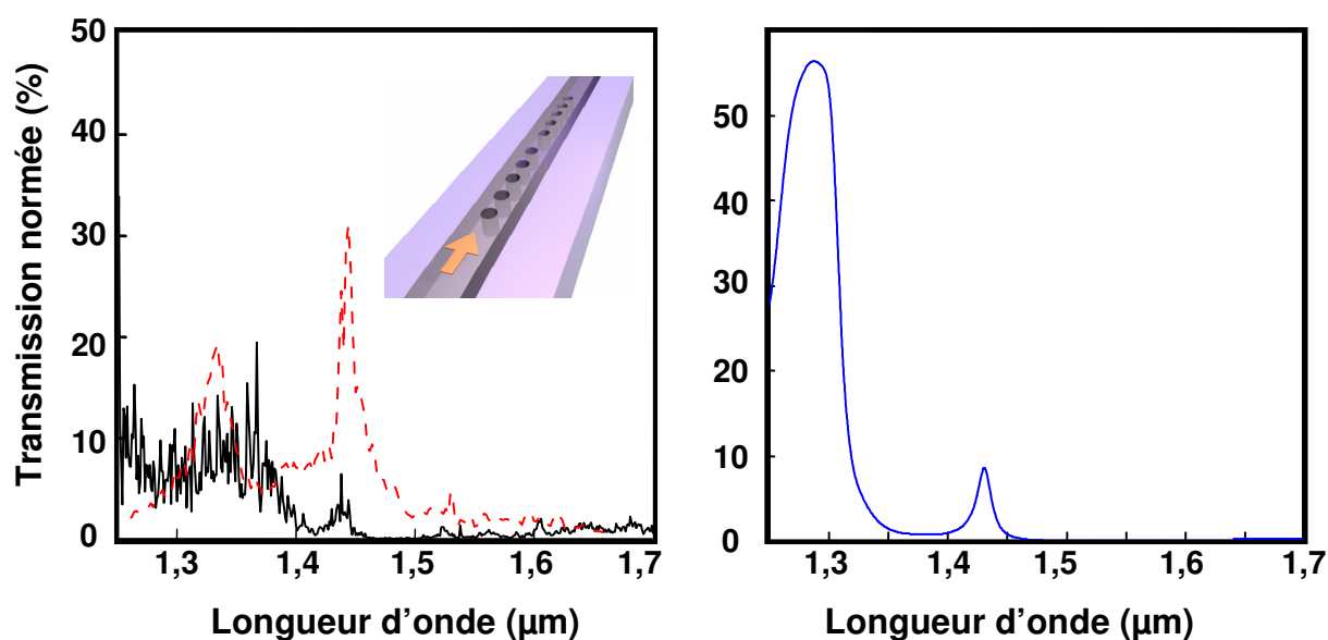
Figure 38 – A gauche, Transmission normalisée d'une cavité avec N=5 et en pointillés une mesure par-dessus la cavité. La section du guide est de 500 nm par 340 nm. Le diamètre des trous est 180 nm et la période 370 nm. En insert, schéma d'une cavité avec N=5 . A droite, simulation 3D de cette cavité
