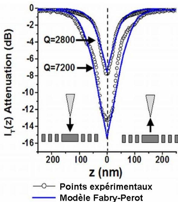
Figure 87 - Evolution de l'intensité transmise à longueur d'onde fixe en fonction de la hauteur de la pointe. Confrontation des résultats expérimentaux et du modèle Fabry-Perot pour les deux cavités sur un cycle de descente et de remontée.
