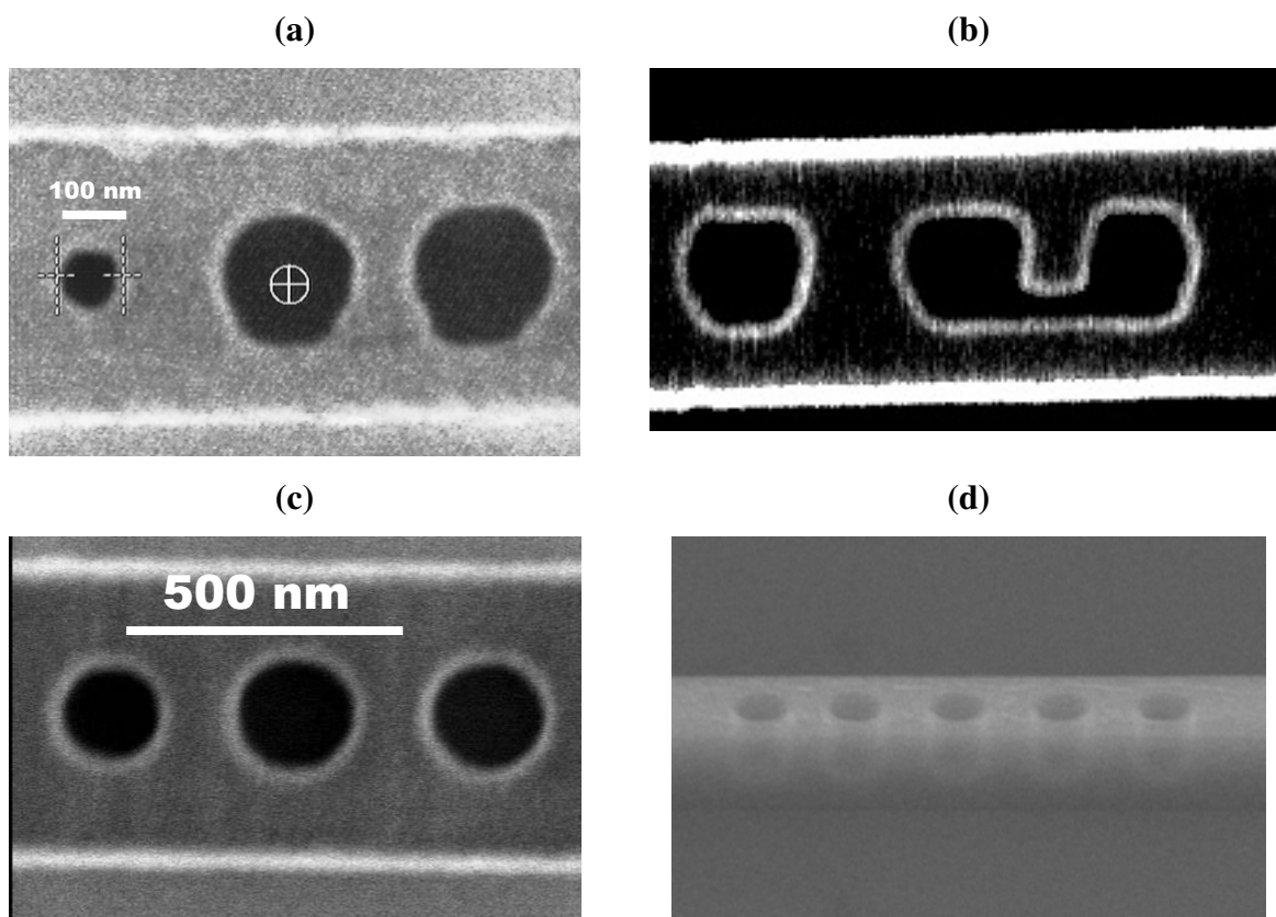
Figure 24 – Images MEB de la résine après insolation et développement montrant les défauts des trous insolés. (a) et (b) avec le masqueur à grille 20 nm. (c) avec une grille de 5 nm. (d) vue en perspective du niveau résine.
