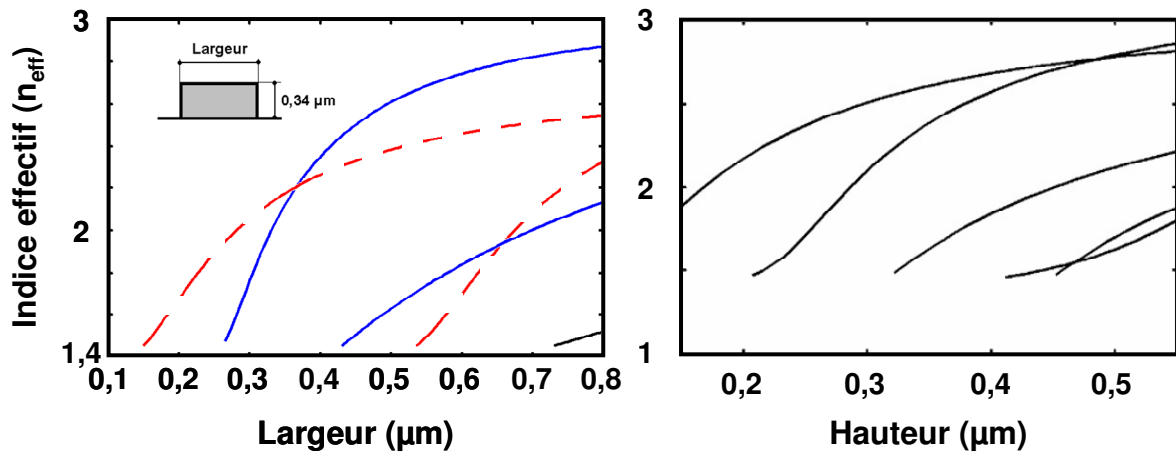
Figure 10 - Diagramme des modes existants en fonction de la largeur (à gauche) et de la hauteur (à droite, largeur de 500 nm) du guide ruban : en tiret rouge les modes TM-like et en bleu les modes TE-like. Les modes sont calculés à \lambda=1,6 \mu\text{m} .
