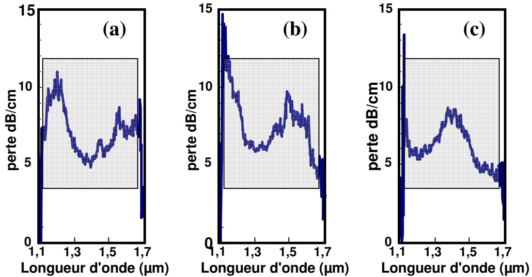
Figure 33 - Pertes en ligne en dB/cm fonction de la longueur d'onde pour différente largeur de guide d'onde. (a) Guides de largeur 450 nm. (b) Guides de largeur 500 nm. (c) Guides de largeur 550 nm. En grisé, les longueurs d'onde où la régression fonctionne.
