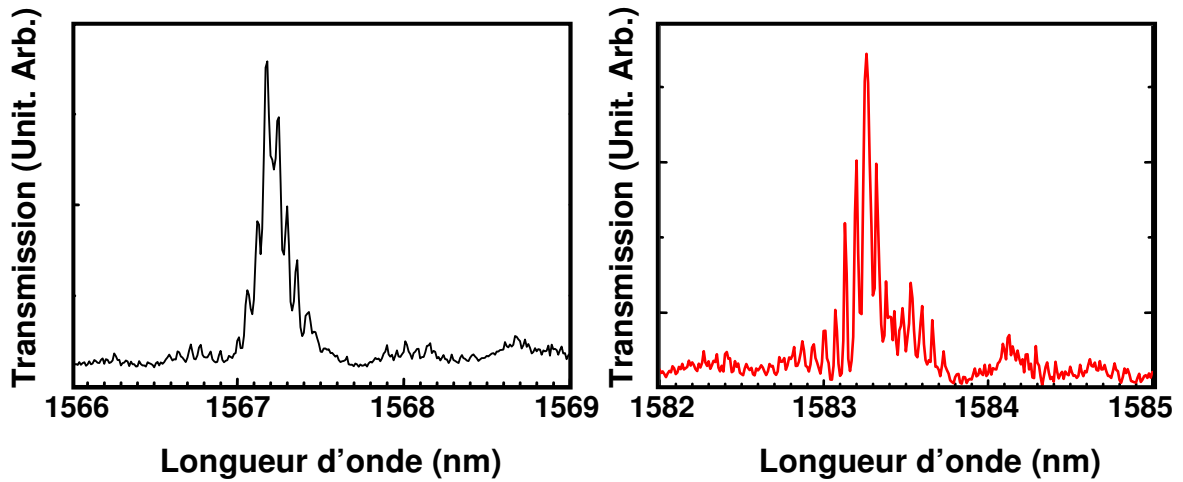
Figure 48 – Exemple de deux spectres en transmission de cavités mesurées sur des puces différentes.
