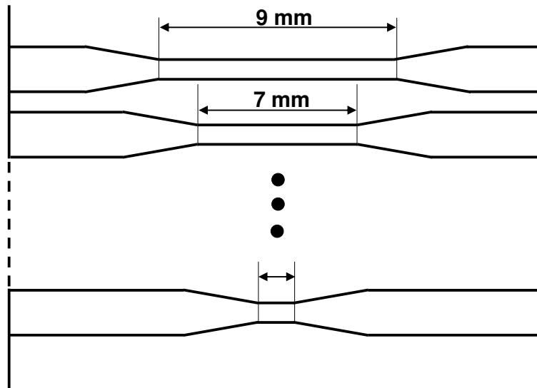
Figure 31 - Schéma des guides utilisés pour mesurer l'atténuation. De part et d'autre du guide de 450, 500 ou 550 nm de large se trouve un guide large de 8 \mu m. La transition entre les deux guides se fait par une zone d'adaptation de 500 \mu m de long.
