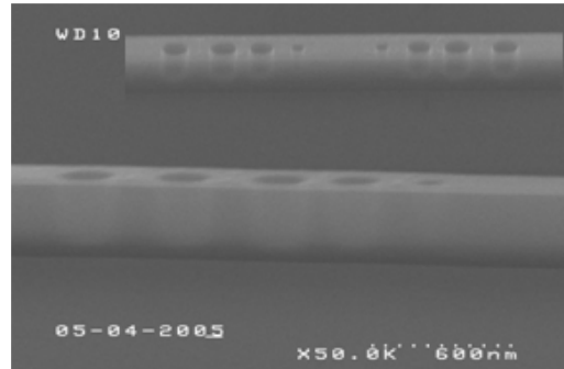
Photo MEB d'une micro-cavité après développement de la résine négative
