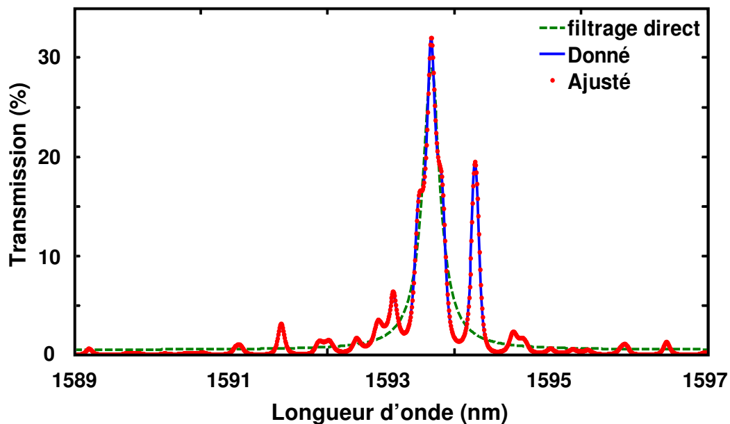
Figure 55 - Comparaison entre le résultat du calcul donné par le modèle avec un jeu de paramètres standard ( L_1=4\text{mm} , L_2=5\text{mm} , Q=25\,000 , contraste élevé – en bleu) et l'estimation par ajustement (en point rouge). La courbe en pointillés verts donne le résultat du filtrage direct.
