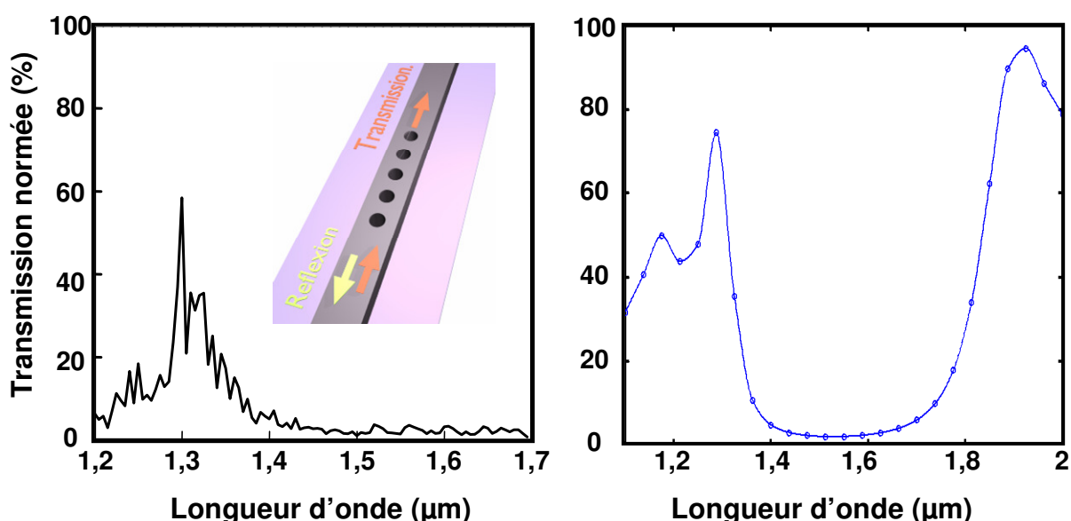
Figure 37 – À gauche, la transmission du miroir avec N=4 normalisée par une référence. À droite, calcul 3D de la transmission de la même structure. Le guide d'onde en silicium a une hauteur de 340 nm et de 500 nm. Le miroir périodique est formé d'une série de trous de 180 nm de diamètre et de 370 nm de période.
