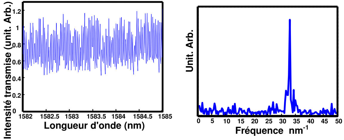
Figure 34 - Spectre en transmission d'un guide ruban de 10 mm de long. A droite, transformée de Fourier de ce spectre.
