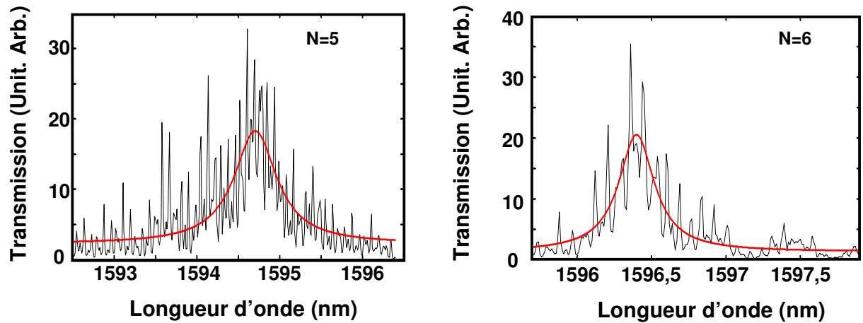
Figure 68 - Spectre en transmission de deux cavités à recyclage du second ordre. A droite, spectre obtenu pour N=5 et à gauche pour N=6.
