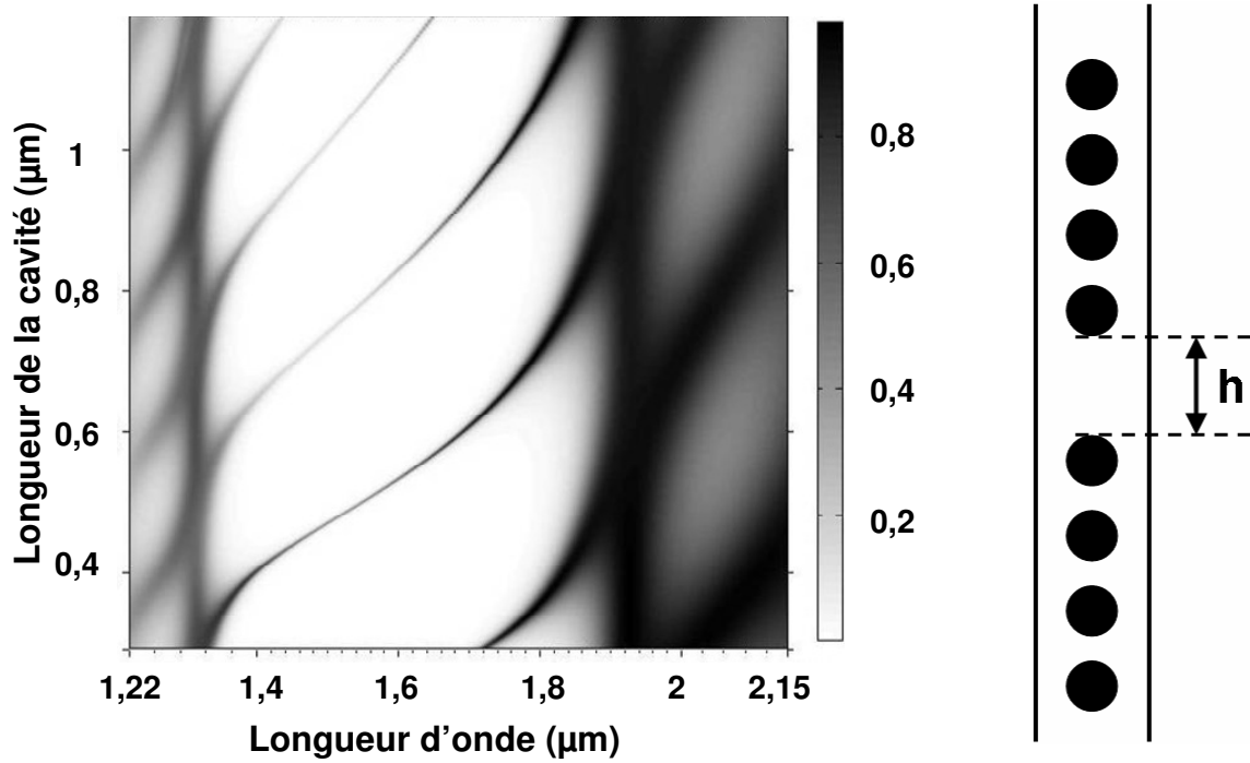
Figure 18 - Transmission d'une cavité à miroir périodique ( N=4 ) complète sur substrat \text{SiO}_2 , en fonction de la longueur de cavité ( h ) et de la longueur d'onde, obtenue par calcul 3D. Le schéma de droite montre la géométrie considérée.
