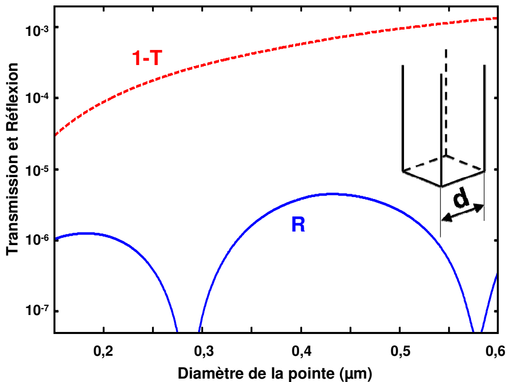
Figure 77 - Evolution de la transmission T (1-T en pointillé rouge) et de la réflexion R (courbe bleue) en fonction de la dimension de la pointe en silice ( n=1,5 ). A droite, schéma de la pointe à section carrée. Le guide en silicium est de largeur 500 nm et de hauteur 340 nm. Le calcul est effectué à 1,6 \mu\text{m} .
