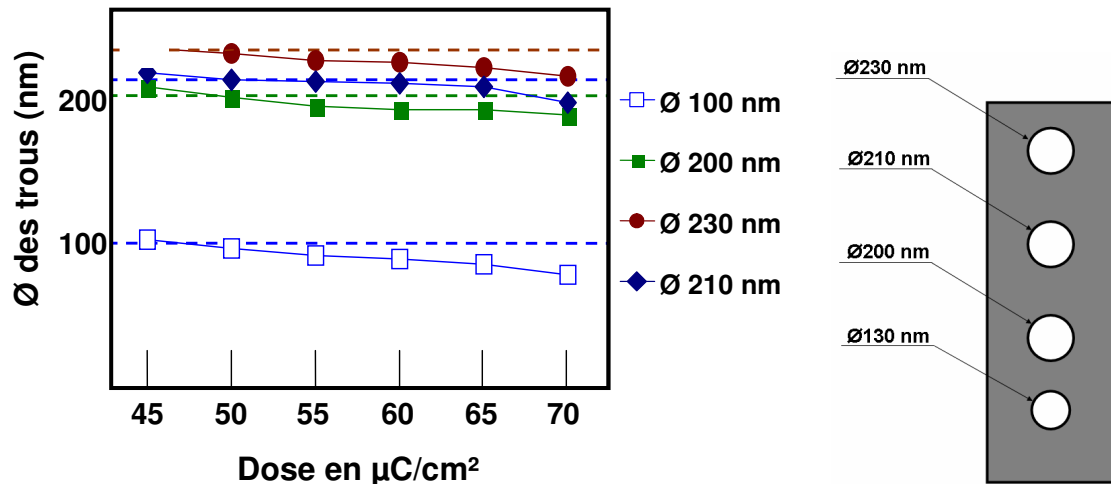
Figure 22 - Evolution des tailles des trous en fonction de la dose d'insolation. A droite, schéma des motifs insolés. En gris, partie de la résine exposée.
