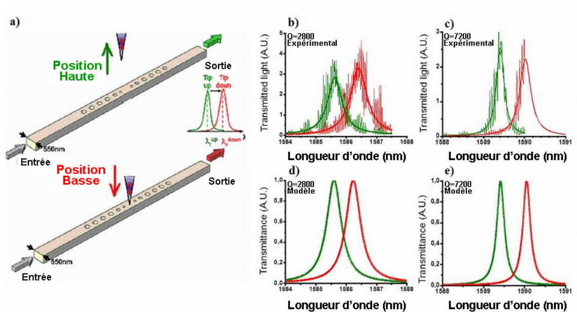
Figure 86 - Comparaison entre le modèle et les mesures pour l'expérience de la Figure 72. En d) (respectivement e)) le calcul avec le modèle Fabry-Perot correspondant à la mesure en b) (respectivement c)).
