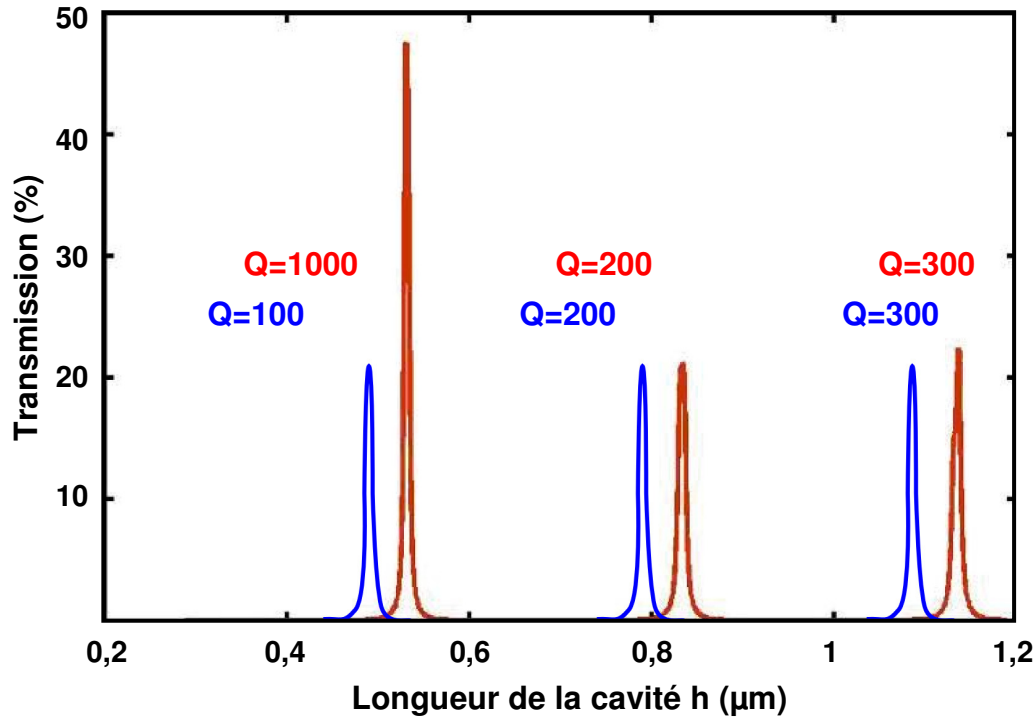
Figure 19 – Coupe en longueur d’onde ( \lambda=1,6\mu\text{m} ) de la Figure 18 montrant les résonances de la cavités en fonction de la longueur de la cavité. En bleu le modèle Fabry-Perot et en rouge le calcul a-FMM. Les deux courbes sont décalées pour plus de lisibilité.
