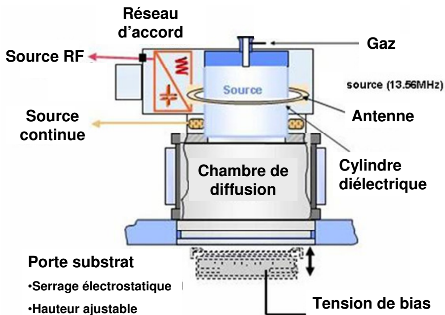
Figure 26 -Schéma d'un bâti de gravure sèche ICP. Ce schéma est issu de (@EPFL).
