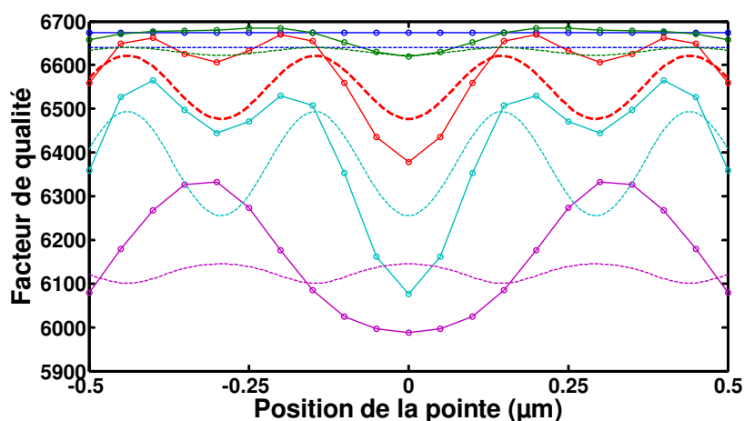
Figure 84 - Evolution du facteur de qualité en fonction de la position de la pointe dans le plan pour différentes dimensions de pointe. Les courbes en pointillé sont obtenues à partir du modèle analytique et les courbes continues avec des points sont obtenues par calcul numérique 3D.
