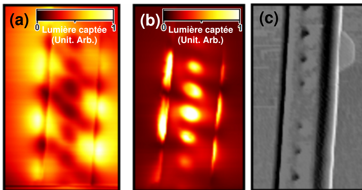
Figure 70 –Cartographie SNOM de la lumière captée par la pointe à la surface de l'échantillon à la longueur d'onde de résonance de la cavité (a) et à une longueur d'onde légèrement plus élevée (b). (c) Image topographique de l'échantillon obtenue pendant le balayage de la pointe.
