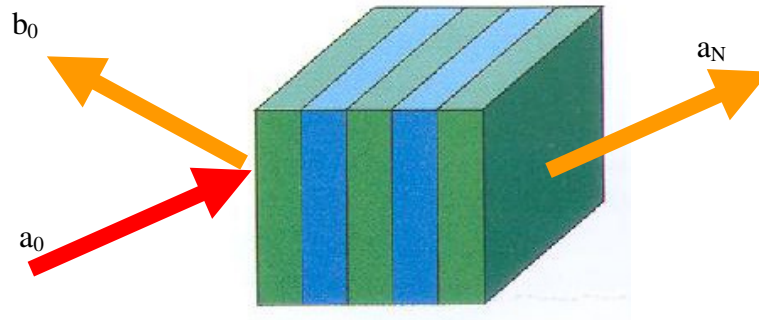
Figure 3 - Schéma d'un miroir de Bragg constitué d'un empilement de N couches périodiques de 2 matériaux différents. Une onde incidente d'amplitude a_0 réfléchi une onde d'amplitude b_0 et transmet une onde d'amplitude a_N .
