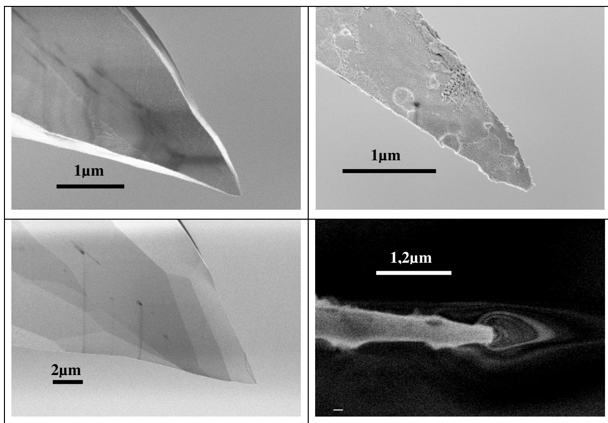
Figure 76 - Photos MEB de 4 pointes de fibre en silice fabriquée par attaque chimique dans des conditions identiques.
