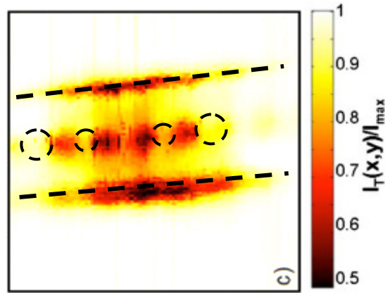
Figure 74 - Mesure de la transmission de la cavité en fonction de la position de la pointe au-dessus de la cavité.
