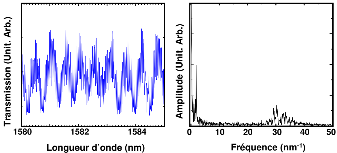
Figure 47 – À gauche, transmission d'un guide ruban échantillonné à 10 pm. A droite, Transformée de Fourier de ce spectre en transmission.
