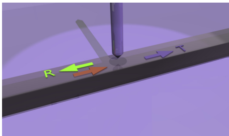
Figure 75 - Vue schématique d'une pointe au-dessus d'un guide ruban. L'onde incidente (flèche rouge) est réfléchie avec un coefficient R=|r|^2 (flèche verte) et transmise avec un coefficient T=|t|^2 (flèche bleue).
