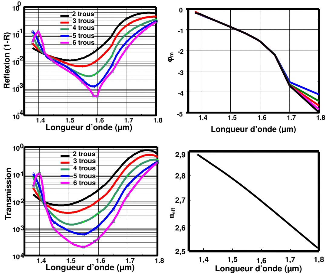
Figure 61 - Caractéristiques principales d'un miroir adapté en fonction de la longueur d'onde pour différents N. En haut à gauche : réflexion du miroir. En haut à droite : évolution de la phase à la réflexion. En bas à gauche : transmission, à droite : évolution de l'indice effectif n_{\text{eff}} du mode M1.
