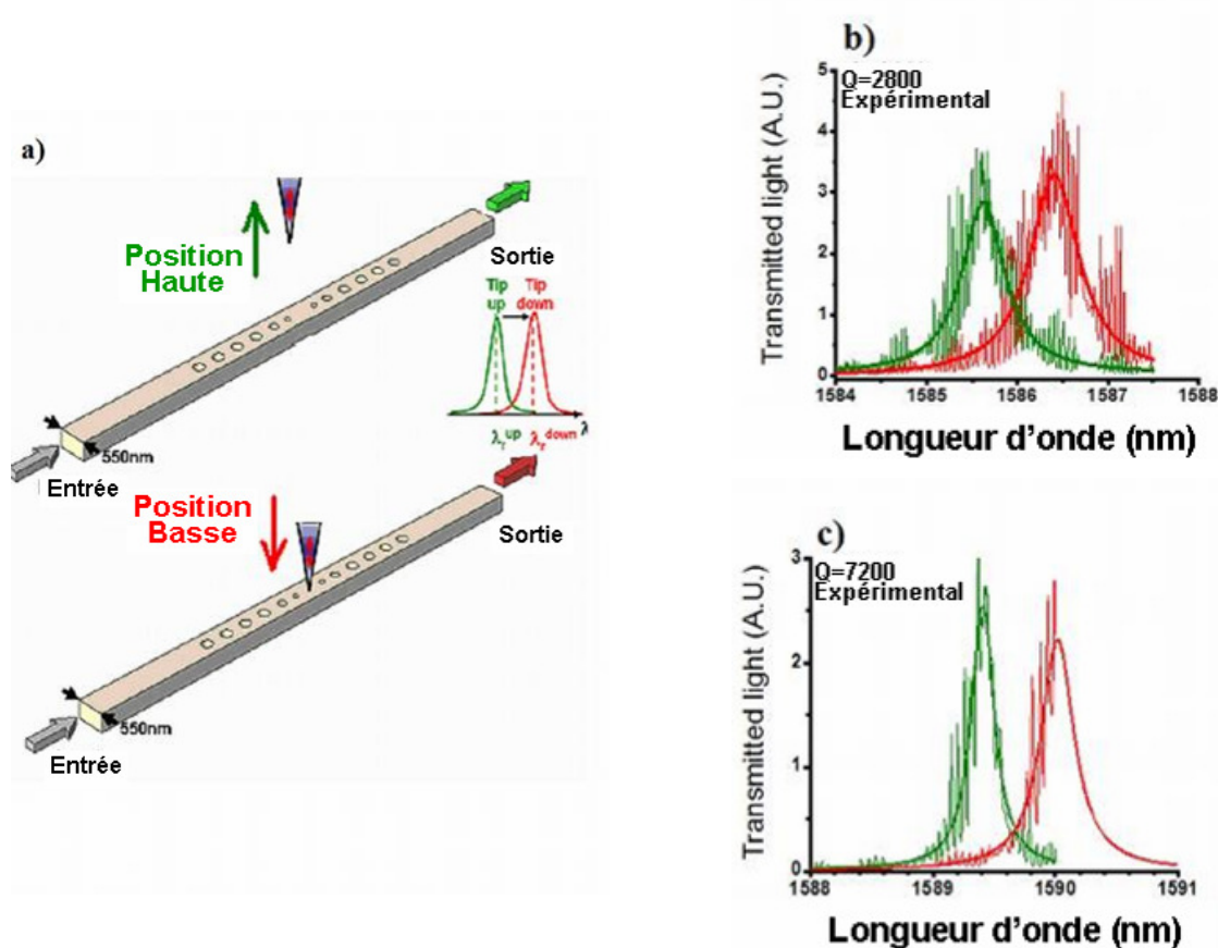
Figure 72 - Résultats obtenus en approchant une pointe de silice de deux cavités de facteurs de qualité de 2800 et 7200. a) Schéma de l'approche de la pointe. b) et c) Spectres en transmission obtenus sans la pointe (courbe verte) et avec la pointe (en rouge). Figure tirée de (LAL07a).
