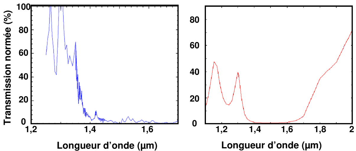
Figure 43 - A gauche, Spectre en transmission d'un miroir adapté avec N=4 . A droite, calcul 3D de la structure correspondante.
