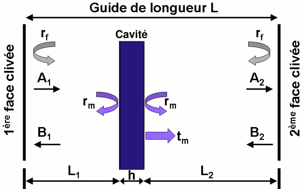
Figure 51 - Schéma du modèle d'une cavité dans un guide d'onde. Les différentes interfaces sont considérées comme des plans possédant une réflectivité et une transmission modale. La cavité (en bleue) est placée à une distance L_1 de la première face clivée et à une distance L_2 de la deuxième face clivée. r_f est la réflectivité modale et t_f la transmission modale des faces clivées ; r_m et t_m représentent la réflectivité et la transmission modale des miroirs de la cavité test. La cavité de longueur h est placée à une distance L_1 de la première face clivée et L_2 de la deuxième face clivée
