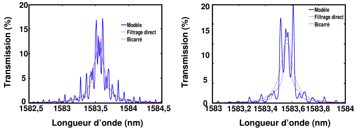
Figure 54 - Deux exemples d'application de la méthode bicarré sur deux cavités modèles avec Q=9250 (à gauche) et Q=23560 (à droite). Les courbes bleues représentent les transmissions données par le modèle et les courbes en pointillé vert donne le résultat du filtrage direct. Les courbes magenta donnent le filtrage par résolution de l'équation bicarré.
