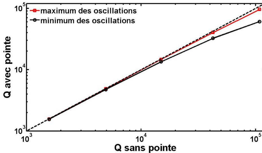
Figure 85 - Variation du facteur de qualité induite par une pointe en silice de 300 nm en fonction du facteur de qualité de la cavité sans pointe. Q varie en fonction de la position de la pointe et il n'a été reporté sur cette figure que le minimum (courbe en rouge) et le maximum de ces oscillations (courbes en noir). En pointillé, la référence d'une cavité sans pointe.
