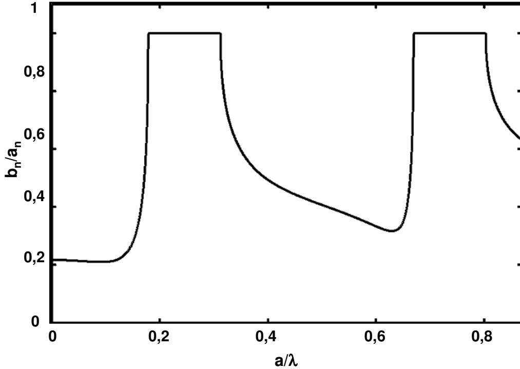
Figure 5 - Evolution du rapport b_n/a_n en fonction de a/\lambda pour la géométrie de la Figure 6.
