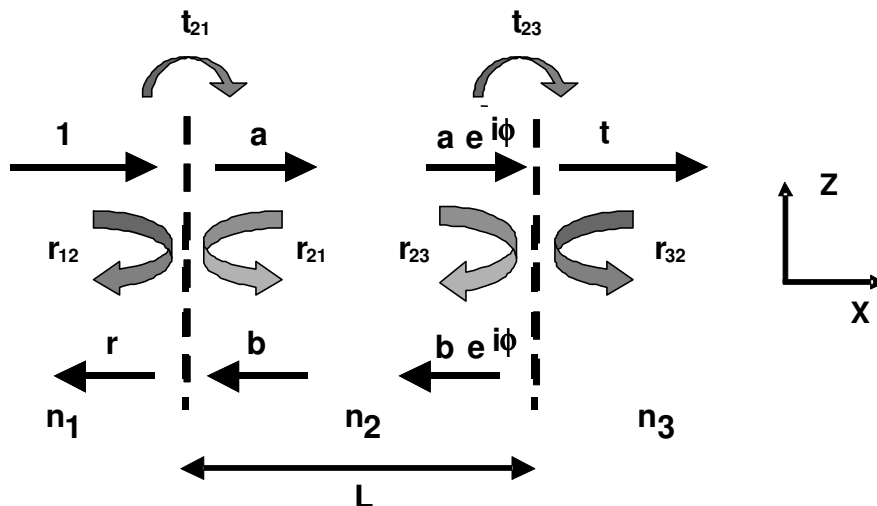
Figure 2 - Schéma de principe d'un interféromètre Fabry-Perot
