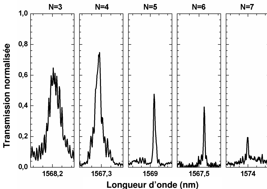
Figure 58 – Spectres en transmission de cavités avec N=3, 4, 5, 6, 7 en unité normalisée (la normalisation est discutée plus loin) sur un intervalle de 1 nm en longueur d'onde.
