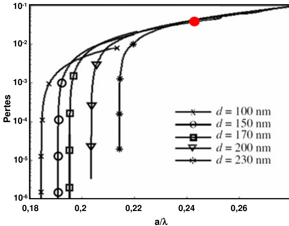
Figure 15 - Calcul des pertes pour différents diamètres de trou dans le miroir périodique en fonction de a/\lambda . Le point rouge représente les pertes du miroir périodique que nous avons choisi.
