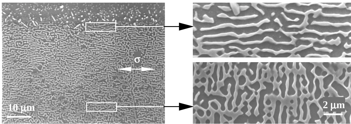
Figure IV.38: coalescence des précipités \gamma dans le substrat de l'éprouvette sollicitée en cycle triangle sous \Delta\epsilon_m=1,6\% jusqu'à la durée de vie. Coupe attaquée à l'eau régale: 66% vol. acide chlorhydrique, 33% vol. acide nitrique.
