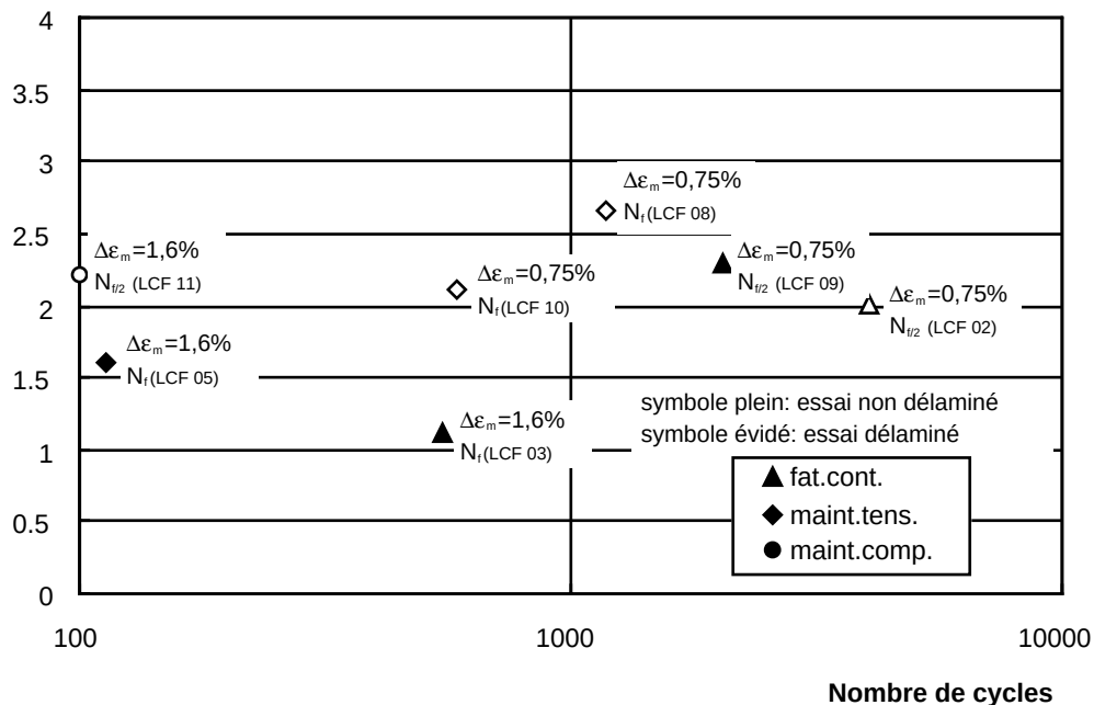
Figure IV.40: épaisseur moyenne de la couche d'alumine en fonction du nombre de cycles de fatigue oligocyclique isotherme. (La valeur relative à l'essai LCF09, \Delta\epsilon_m = 0,75\% , N_{t/2} , est mesurée en zone non délamination)
