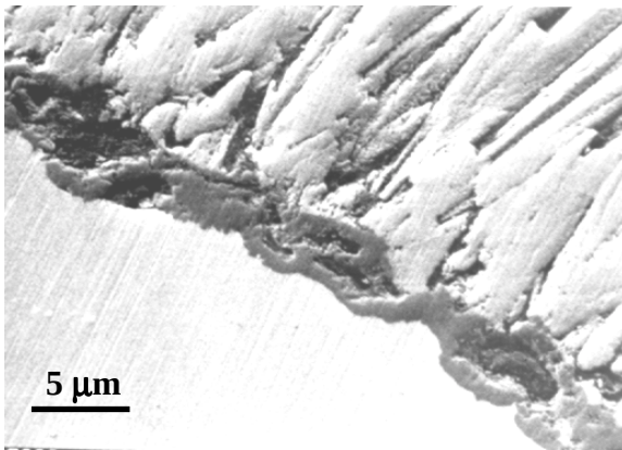
Figure IV.55: éprouvette de fatigue mécano-thermique sollicitée pendant 247 cycles.
