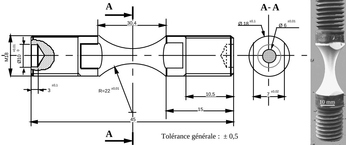
Figure III.9: dessin de définition de l'éprouvette AG2C et photographie après dépôt de la barrière thermique.
