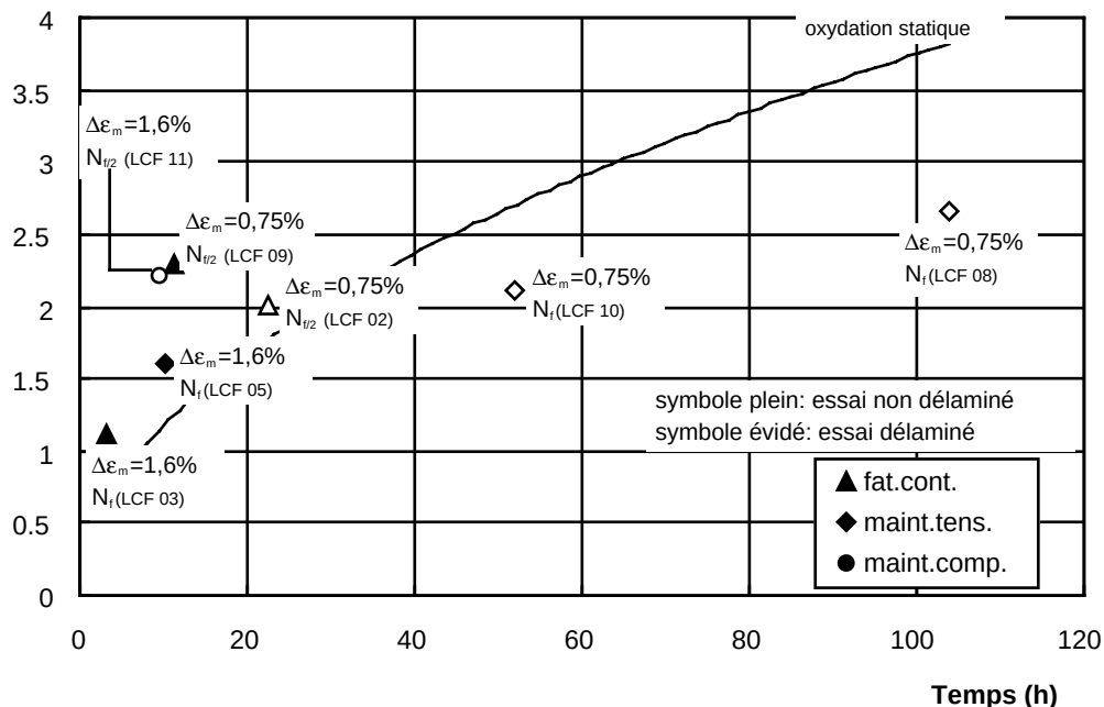
Figure IV.41: épaisseur moyenne de la couche d'alumine en fonction du temps passé à 1100^\circ\text{C} par l'éprouvette. (La valeur relative à l'essai LCF09, \Delta\epsilon_m = 0,75\% , N_{f/2} , est mesurée en zone non délaminée)
