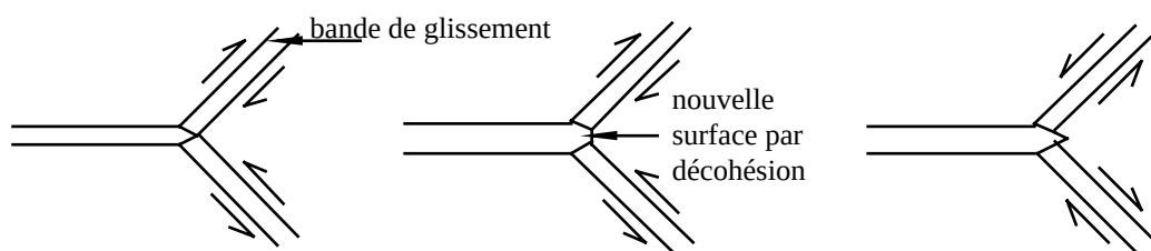
Figure II.51: création de nouvelles surfaces sous l'action des contraintes de tension. D'après Tomkins (1968). Schéma de gauche: début de la phase en tension. Schéma du milieu: la contrainte de rupture est atteinte en pointe de fissure. Schéma de droite: début de la phase de compression.
