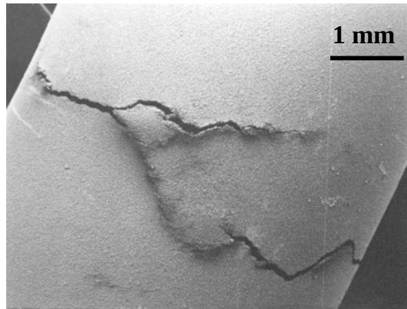
Figure IV.21: partie utile de l'éprouvette sollicitée en cycle triangle sous \Delta\epsilon_m = 1,6\%
