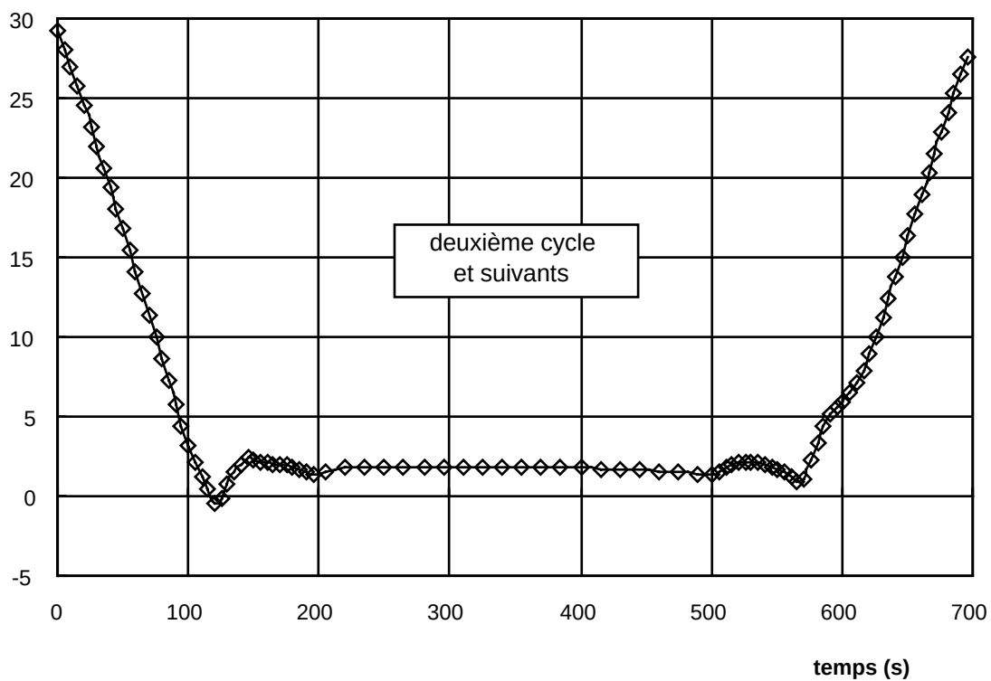
Figure V.31: évolution de la contrainte normale interfaciale d'origine thermique et mécanique au cours d'un cycle de fatigue mécano-thermique sur une éprouvette tubulaire de 5,5mm de rayon et d'une épaisseur d'oxyde 15 \mu m.
