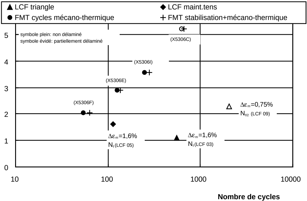
Figure IV.64: épaisseur moyenne de la couche d'alumine en fonction du nombre de cycles de fatigue mécano-thermique (FMT) et de fatigue isotherme (LCF). (Symbole plein: aucun délaminage, symbole évidé: délaminage ou écaillage).
