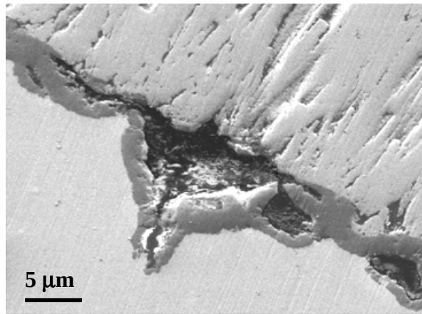
Figure IV.56: éprouvette de fatigue mécano-thermique sollicitée pendant 247 cycles.
