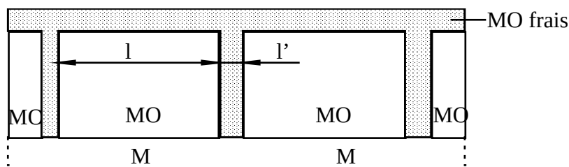
Figure V.42: schématisation de l'oxydation aux joints de grains de l'oxyde.
