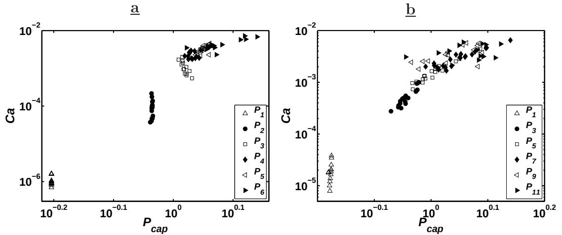
FIG. 3.5: Terme capillaire pour les liquides partiellement mouillants. a- LPM 1. b- LPM 2. Les propriétés des liquides sont prises à T = 30 °C et les pressions sont les mêmes que celles des courbes de la figure 2.11.
