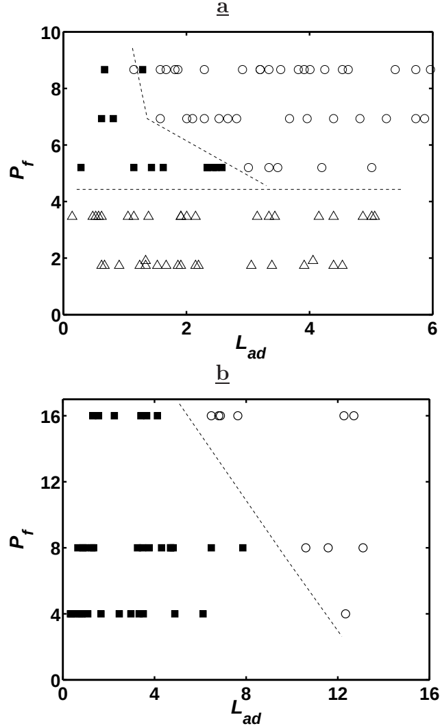
FIG. 2.24: Diagrammes L_{ad} - P_f expérimentaux. On reporte les cas observés qualitativement [division (O), éclatement (■) et blocage ( \Delta )] en fonction de la longueur initiale des bouchons et de la pression de forçage adimensionnalisées. a - Première géométrie - La valeur de la pression de blocage adimensionnalisée se situe autour de 4-5, et le blocage est indépendant de la longueur des bouchons. b - Deuxième géométrie - Le blocage n'est pas observé, les expériences ayant été commencées à une pression de forçage certainement supérieure à la pression de blocage \mathcal{P}_{blocage} . La transition entre l'éclatement et la division est similaire à celle obtenue pour la première géométrie : plus la pression de forçage est grande, plus la longueur requise pour obtenir deux bouchons fils est faible.
