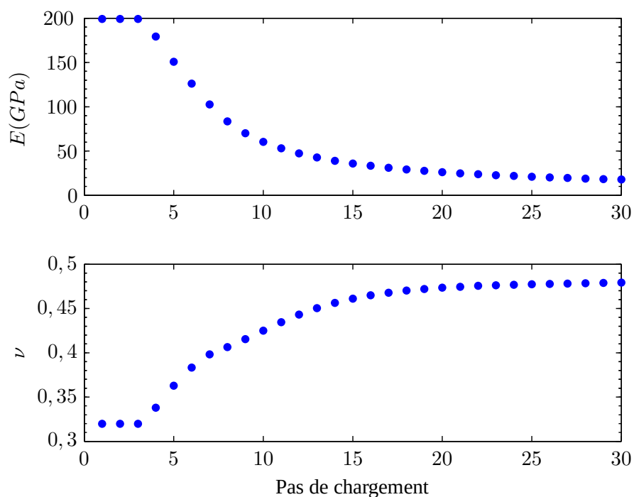
FIG. 5.6: Évolution des paramètres élastiques identifiés avec la MCV sans prise en compte de la plasticité.
