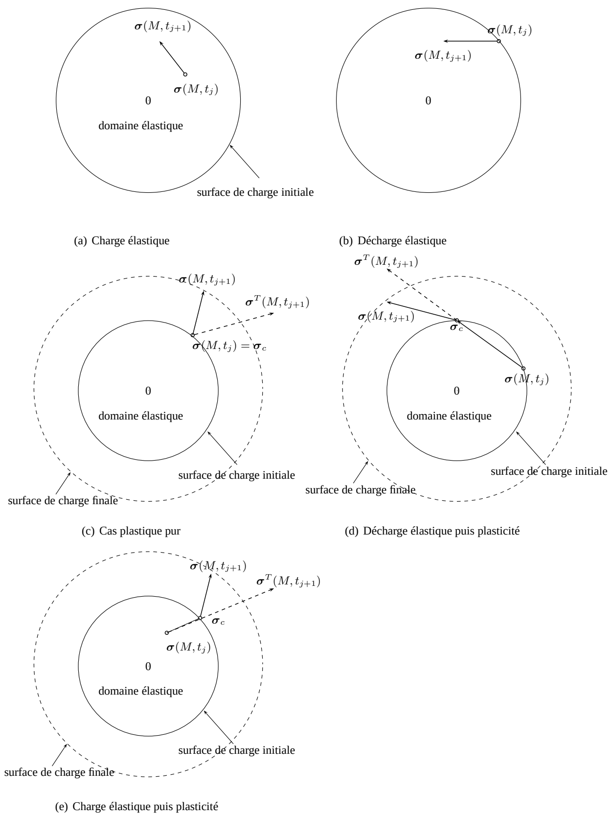
FIG. 3.4: Les cinq cas considérés pour le calcul de la plasticité 2D.
