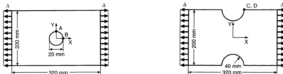
FIG. 1.6: Éprouvettes de traction proposées par Aoki et al. (1997) pour identifier deux paramètres d'un modèle élastoplastique par recalage éléments finis des champs de déplacements.
