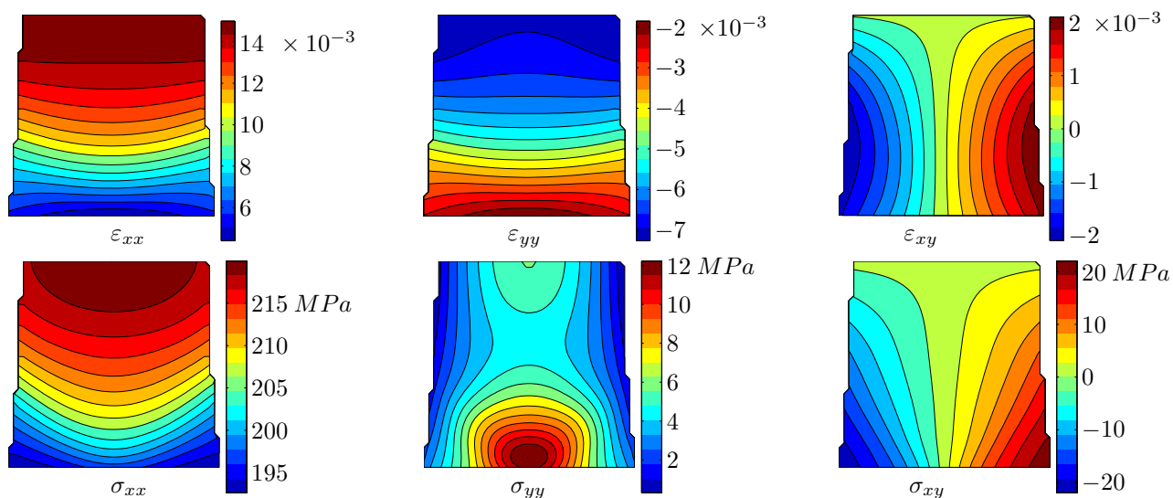
FIG. 5.4: Champs simulés de déformation et de contrainte après apparition de la plasticité ( F = 8930 \text{ N} ), avec le modèle de Voce (tableau 2.2)
