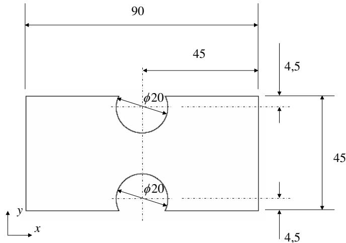
FIG. 6.2: : Géométrie de l'éprouvette de traction plane bi-entallée. Les dimensions sont en mm et seule la partie entre les mors est représentée.
