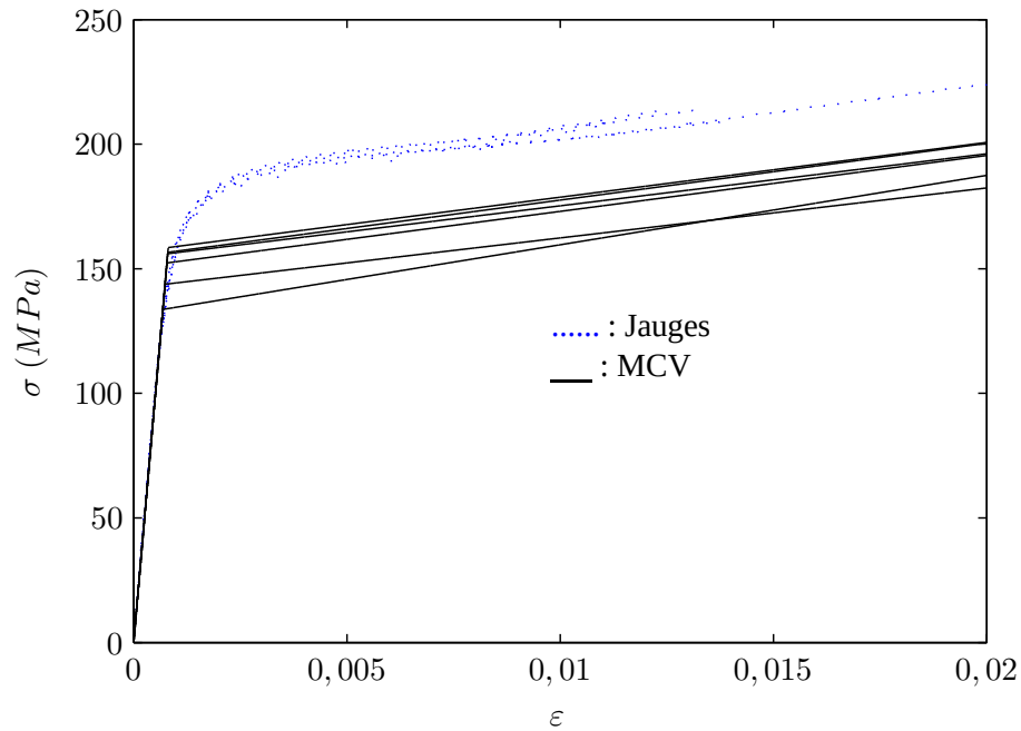
FIG. 6.30: Courbes tracées en supposant une loi d'écrouissage bi-linéaire et à partir des paramètres identifiés (voir tableau 6.10) avec la fonction C_{tot} .
