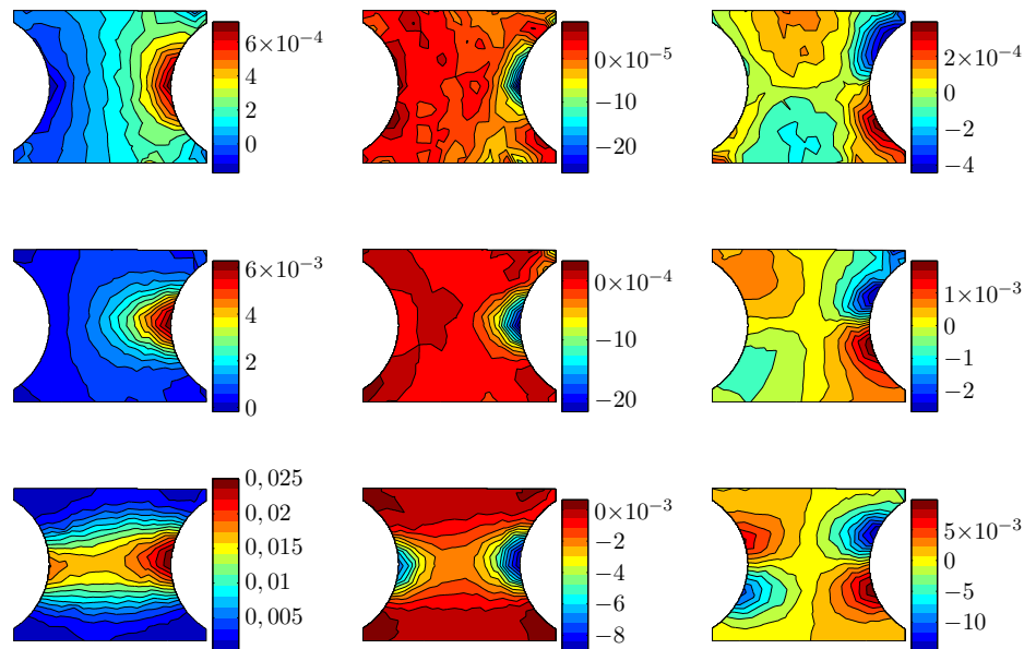
FIG. 6.22: Champs de déformation obtenus après lissage type élément fini de taille 15 pixels de côté au cours du chargement.
