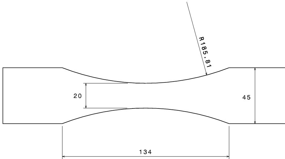
FIG. 5.1: Géométrie de l'éprouvette plane de traction à section variable utilisée pour réaliser un essai quasi uniaxial hétérogène.
