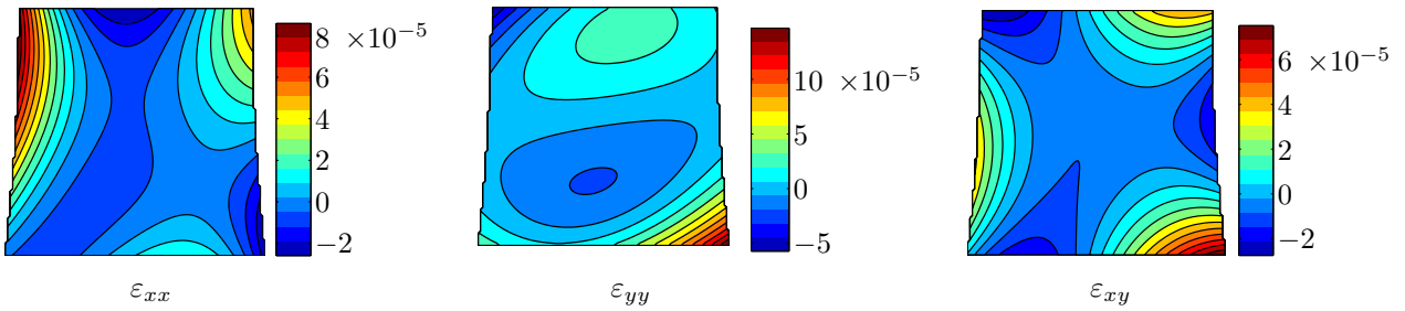
FIG. 5.14: Dérivation des champs polynomiaux de la figure 5.13 afin d'estimer la résolution en déformation.
