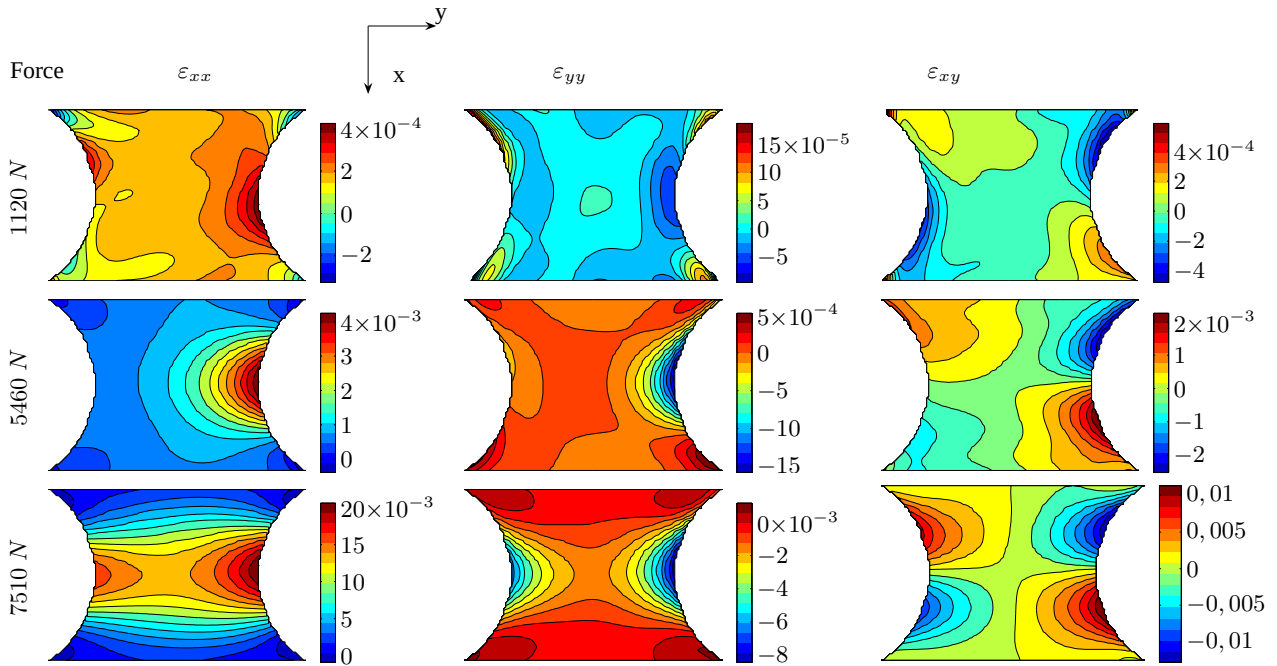
FIG. 6.12: Essai n°1 : champs de déformation obtenus après dérivation d'un polynôme de degré 10 pour trois pas de chargement.
