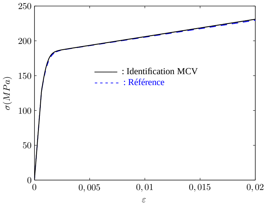
FIG. 5.9: Courbe identifiée à partir des déformations directement issues du calcul par éléments finis et en utilisant la procédure de calcul des contraintes 2D.
