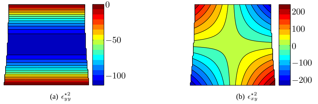
FIG. 3.2: Composantes non nulles du champ de déformation virtuel \epsilon^{*2} .
