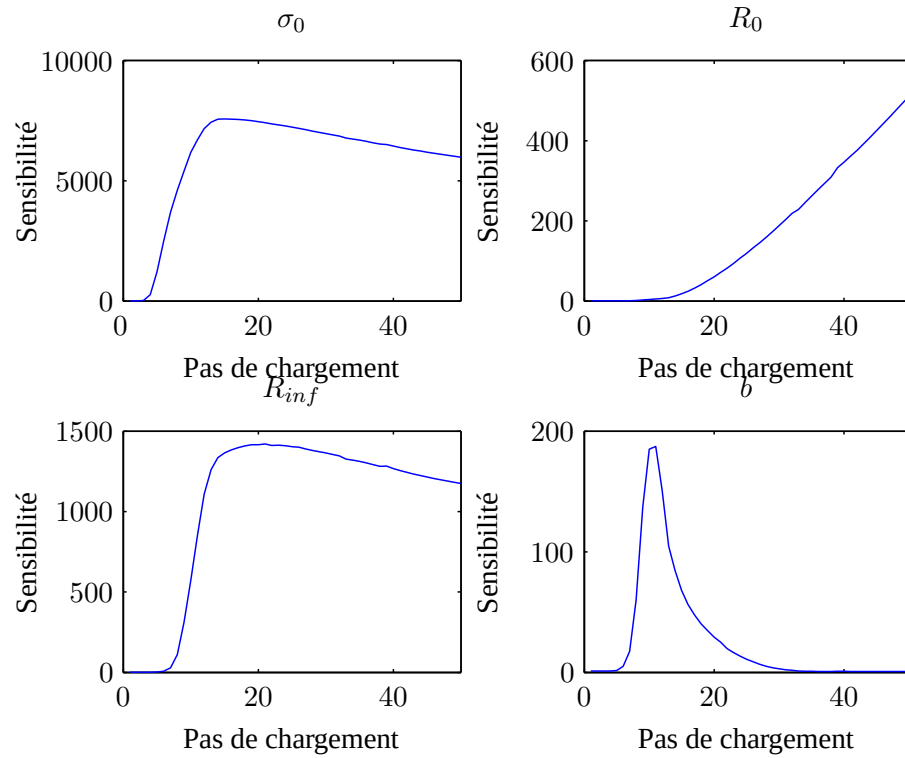
FIG. 6.9: Évolution des sensibilités de la fonction coût aux différents paramètres de la loi d'écrouissage en fonction du pas du chargement.
