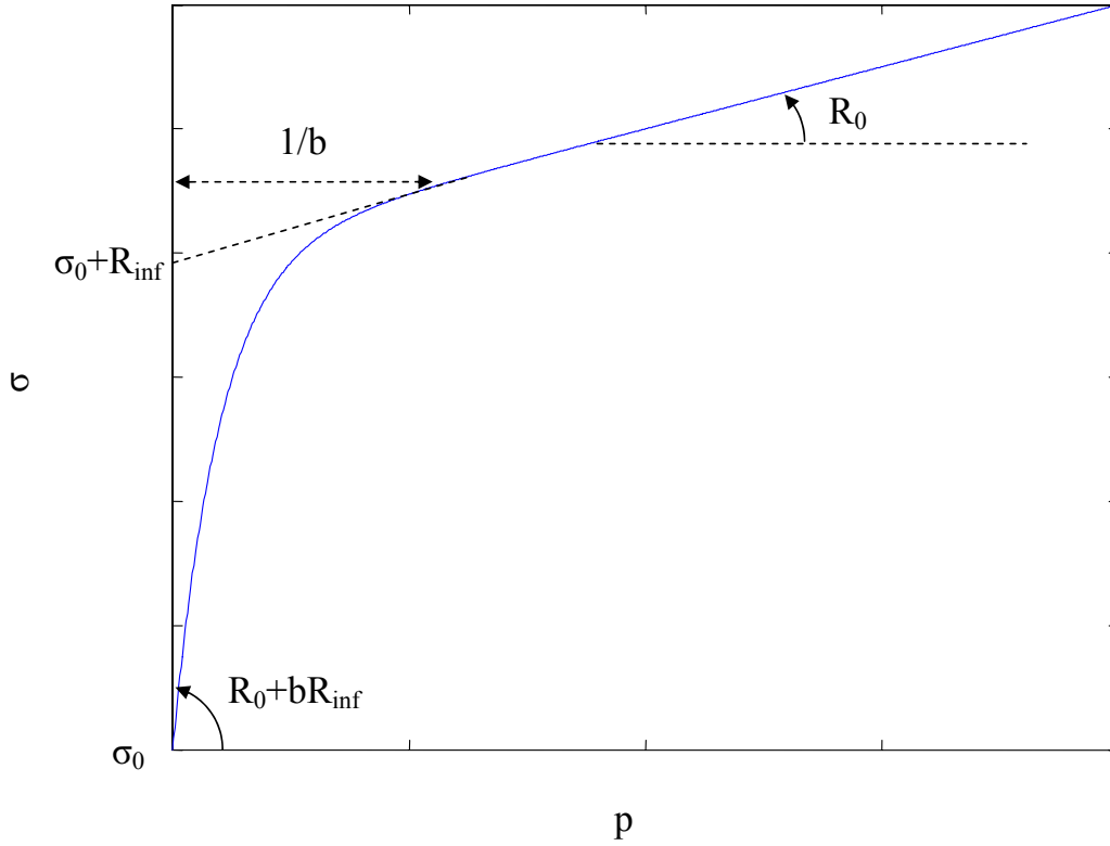
FIG. 2.3: Loi d'écrouissage de Voce : \sigma_s = \sigma_0 + R_0 p + R_{inf}[1 - \exp(-bp)] .
