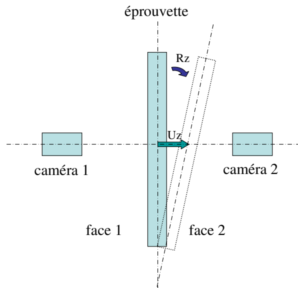
FIG. 4.1: Dispositif à deux caméras et mouvements hors-plan.
