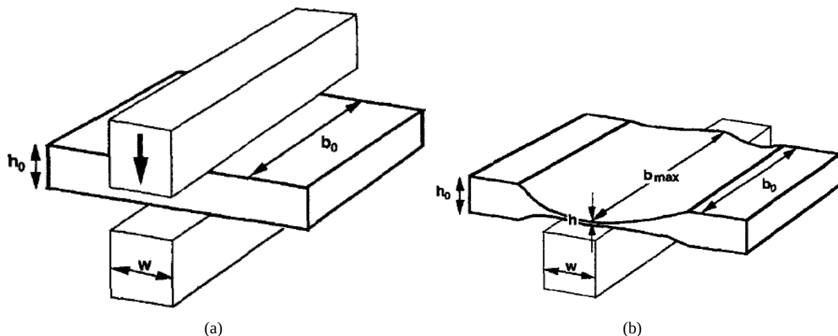
FIG. 1.4: Schéma de l'essai de bipoinçonnement, avant (a) et après (b) déformation (d'après Gelin et Ghouati (1996)).
