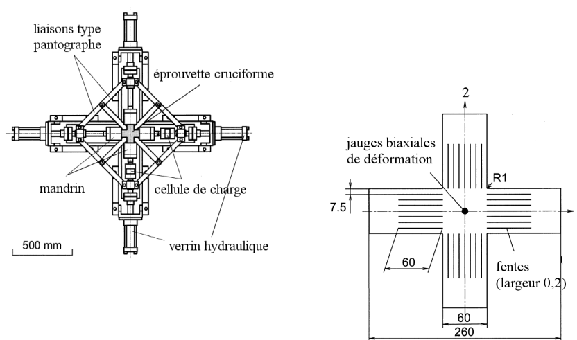
FIG. 1.2: Dispositif de traction biaxiale et éprouvette cruciforme (Kuwabara et al. (2000)).
