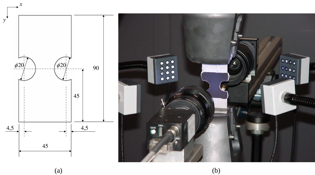
FIG. 6.11: (a) Géométrie (en mm ) de l'éprouvette de traction plane bi-entaillée. (b) Dispositif expérimental : éprouvette en traction (distance entre les mors 90 mm ) munie de grilles de pas 100 \mu m sur les deux faces, caméras alignées et éclairage.
