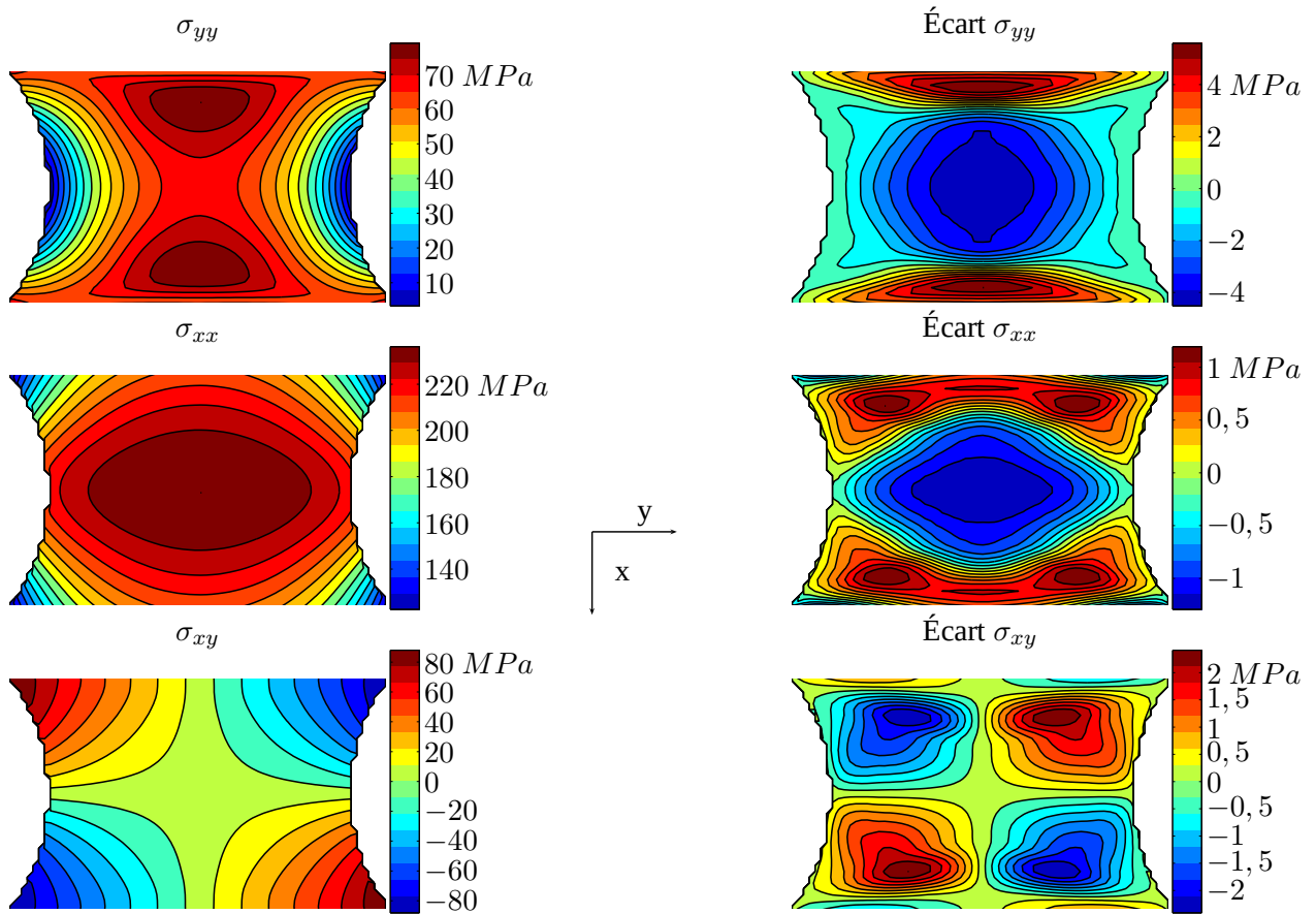
FIG. 6.5: Contraintes calculées avec l'algorithme de calcul de contraintes 2D à partir des déformations directement issues du calcul par éléments finis aux points de Gauss (à gauche) et écarts avec les contraintes directement issues du calcul élément fini aux points de Gauss (à droite).
