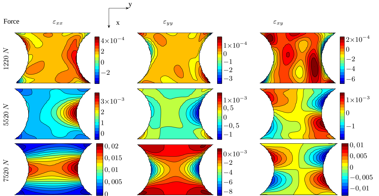
FIG. 6.14: Essai n°3 : champs de déformation obtenus après dérivation d'un polynôme de degré 10 pour trois pas de chargement.
