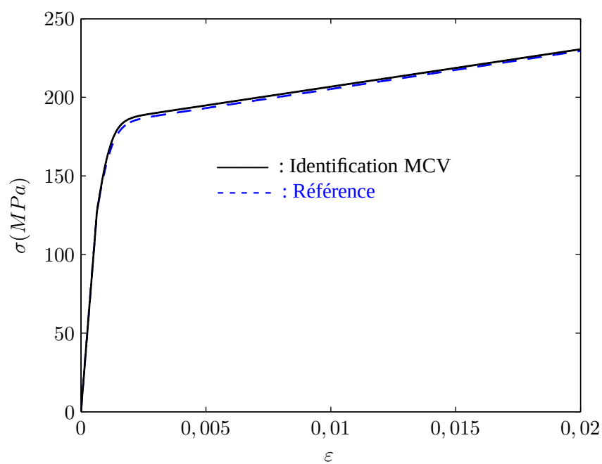
FIG. 5.10: Courbe identifiée à partir de la réponse en déplacement simulée plus un bruit blanc d'écart type 1 \mu m lissée par un polynôme de degré 4.
