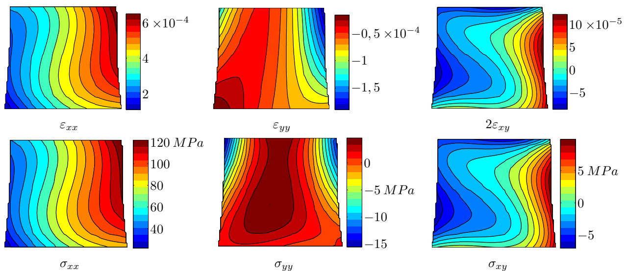
FIG. 5.16: Champs de déformations obtenus après un lissage de degré quatre avant l'apparition de la plasticité (3120 N) et champs de contrainte calculés avec les paramètres élastiques identifiés.
