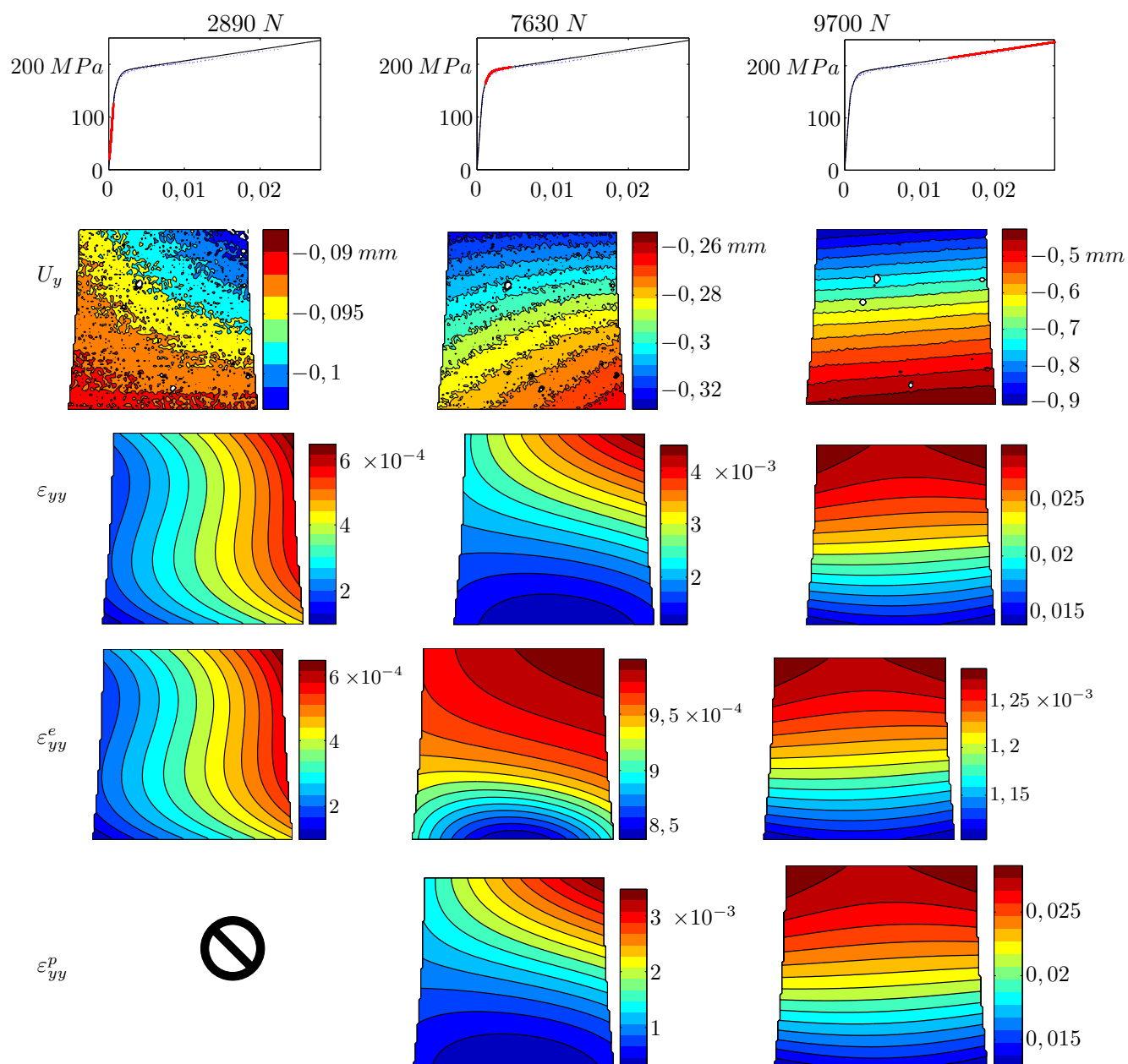
FIG. 5.18: Champs de déplacement mesurés et champs de déformation calculés après un lissage de degré quatre, puis séparation des déformations élastiques et plastiques au cours du chargement à partir des paramètres identifiés (voir tableau 5.8).
