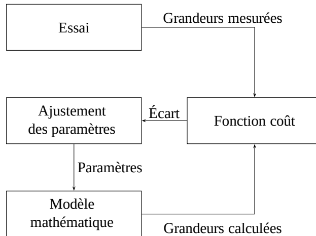
FIG. 1.3: Diagramme de la procédure d'identification par recalage (d'après Hendricks (1991)).
