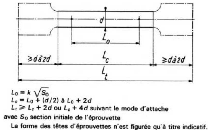
FIG. 2.4: La norme NF A 03-151 précise la forme et les dimensions de la partie calibrée des éprouvettes de traction.
