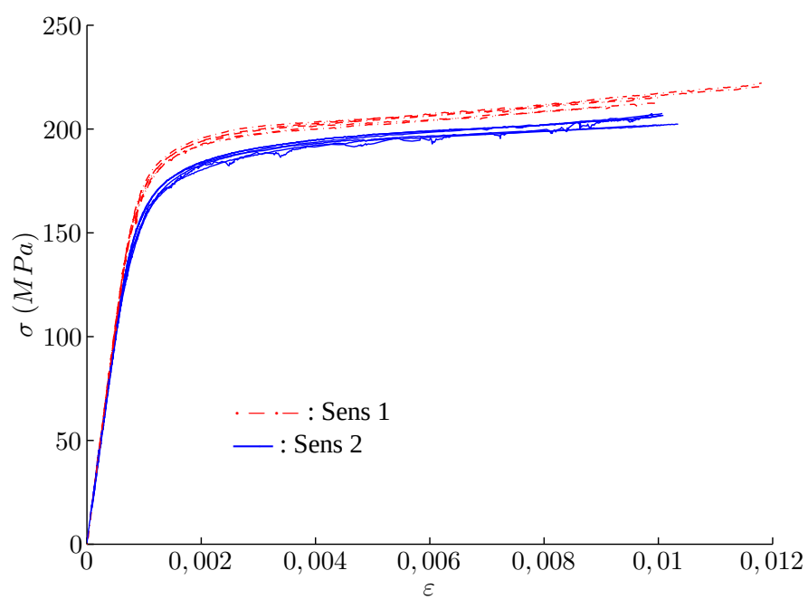
FIG. 2.6: Courbes contrainte-déformation issues des essais homogènes dans les deux directions de la tôle.
