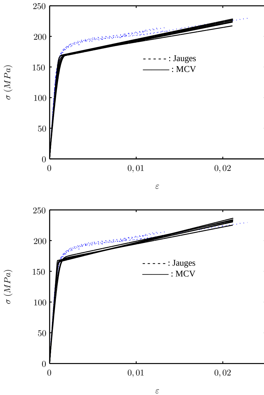
FIG. 6.21: Superposition du faisceau de courbes uniaxiales issues de essais homogènes avec jauges et des courbes calculées à partir des paramètres identifiés sur chacun des six essais sur éprouvette bi-entaillée (de haut en bas, degré 10 et degré 11).
