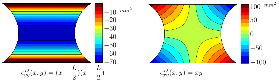
FIG. 6.25: Composantes non nulles du champ de déformation virtuel numéro 2.
