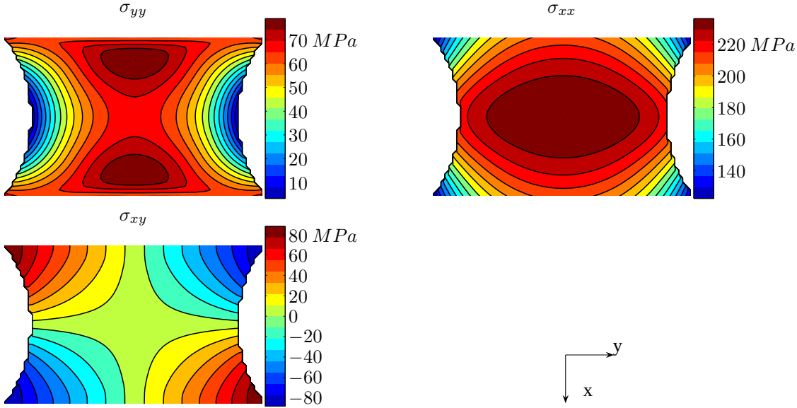
FIG. 6.3: Champ de contraintes entre les entailles issu du calcul par élément fini (points de Gauss) en fin de chargement.
