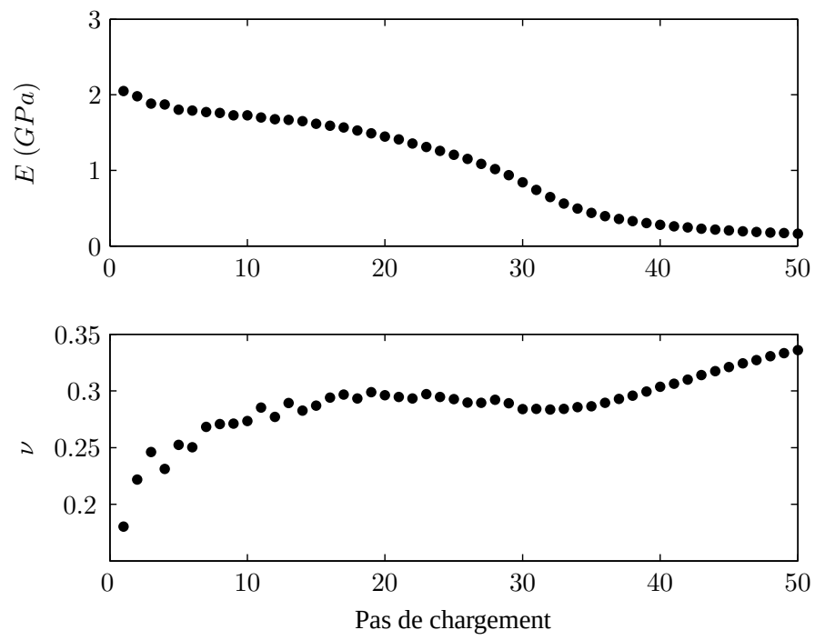
FIG. 6.18: Évolution des paramètres élastiques apparents identifiés au cours du chargement sans prise en compte de la plasticité (essai n^o1 , degré 8).
