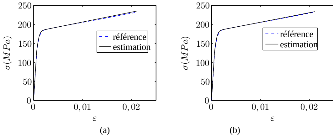
FIG. 6.8: Superposition des courbes uniaxiales de référence et des courbes tracées avec les paramètres identifiés à partir des champs de déformation directement issus du calcul par éléments finis, pour 30 pas (a) et 50 pas (b) de chargement.
