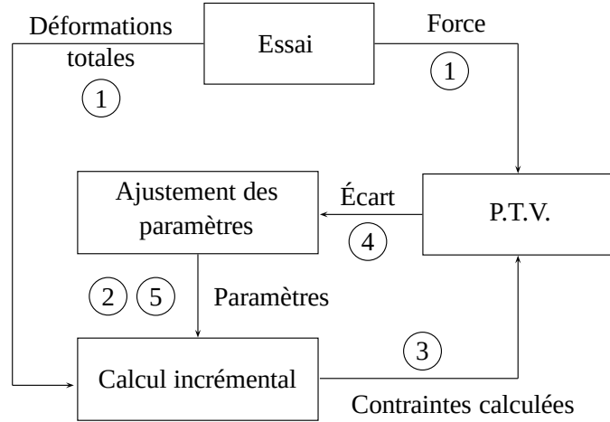
FIG. 5.7: Diagramme de déroulement de la Méthode des Champs Virtuels Non Linéaire (numérotation : voir texte). Les déformations peuvent être mesurées directement ou obtenues par dérivation des déplacements.
