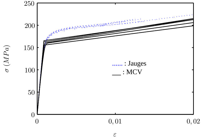
FIG. 6.29: Courbes tracées avec les paramètres identifiés (voir tableau 6.9) à partir de la fonction \mathcal{C}_{tot} .
