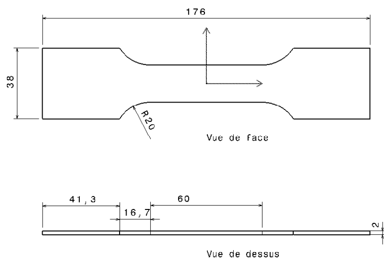
FIG. 2.5: Dimensions des éprouvettes de traction uniaxiale.
