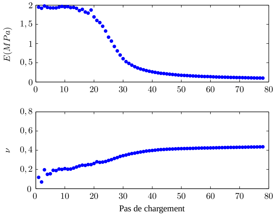
FIG. 5.15: Évolution des paramètres élastiques sans prise en compte de la plasticité.
