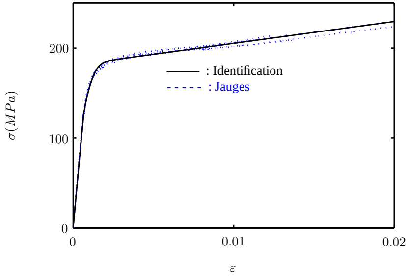
FIG. 5.19: Courbe de Voigt identifiée au sens des moindres carrés sur les réponses des jauges.
