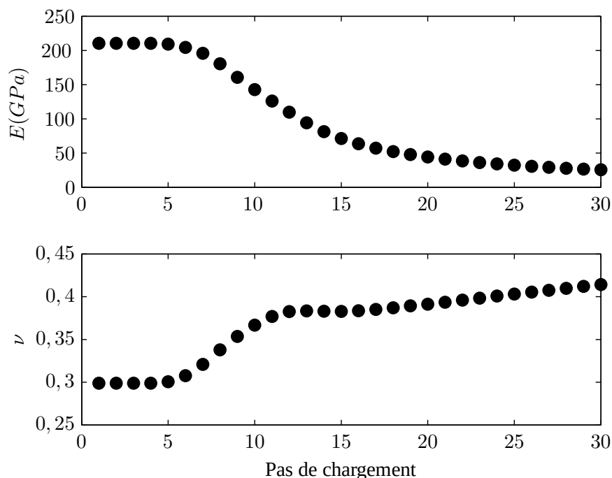
FIG. 6.6: Paramètres élastiques apparents au cours du chargement identifiés avec la MCV linéaire.
