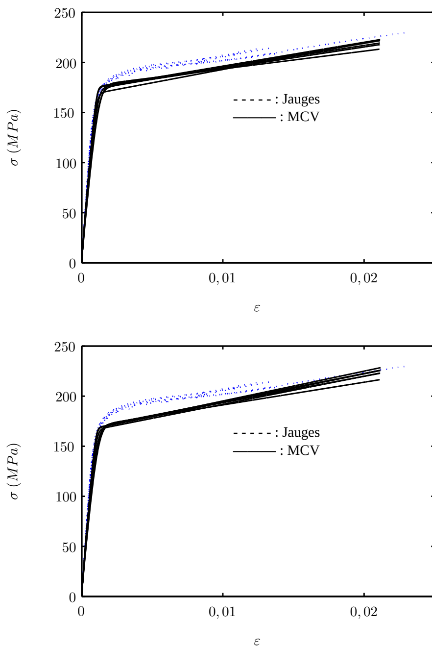
FIG. 6.20: Superposition du faisceau de courbes uniaxiales issues des essais homogènes avec jauges et des courbes calculées à partir des paramètres identifiés sur chacun des six essais sur éprouvette bi-entaillée (de haut en bas, degré 8 et degré 9).
