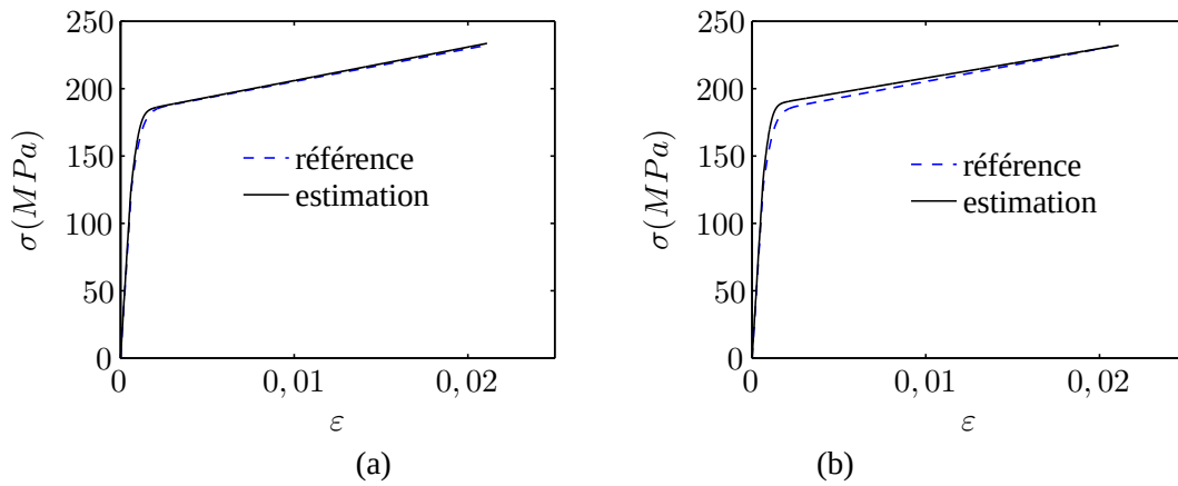
FIG. 6.10: Comparaison des courbes uniaxiales de référence et des courbes tracées à partir des paramètres identifiés avec un polynôme de degré 9 en présence d'un bruit blanc d'écart type 0,1 \mu m (a) et 0,5 \mu m (b).
