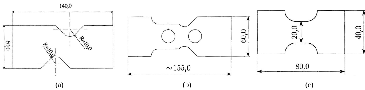
FIG. 1.7: Éprouvettes planes de traction bi-entaillée (a), trouée (b) et de cisaillement (c) utilisées par Meuwissen et al. (1998); Meuwissen (1998) (cotes en mm).
