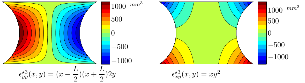
FIG. 6.26: Composantes non nulles du champ de déformation virtuel numéro 3.
