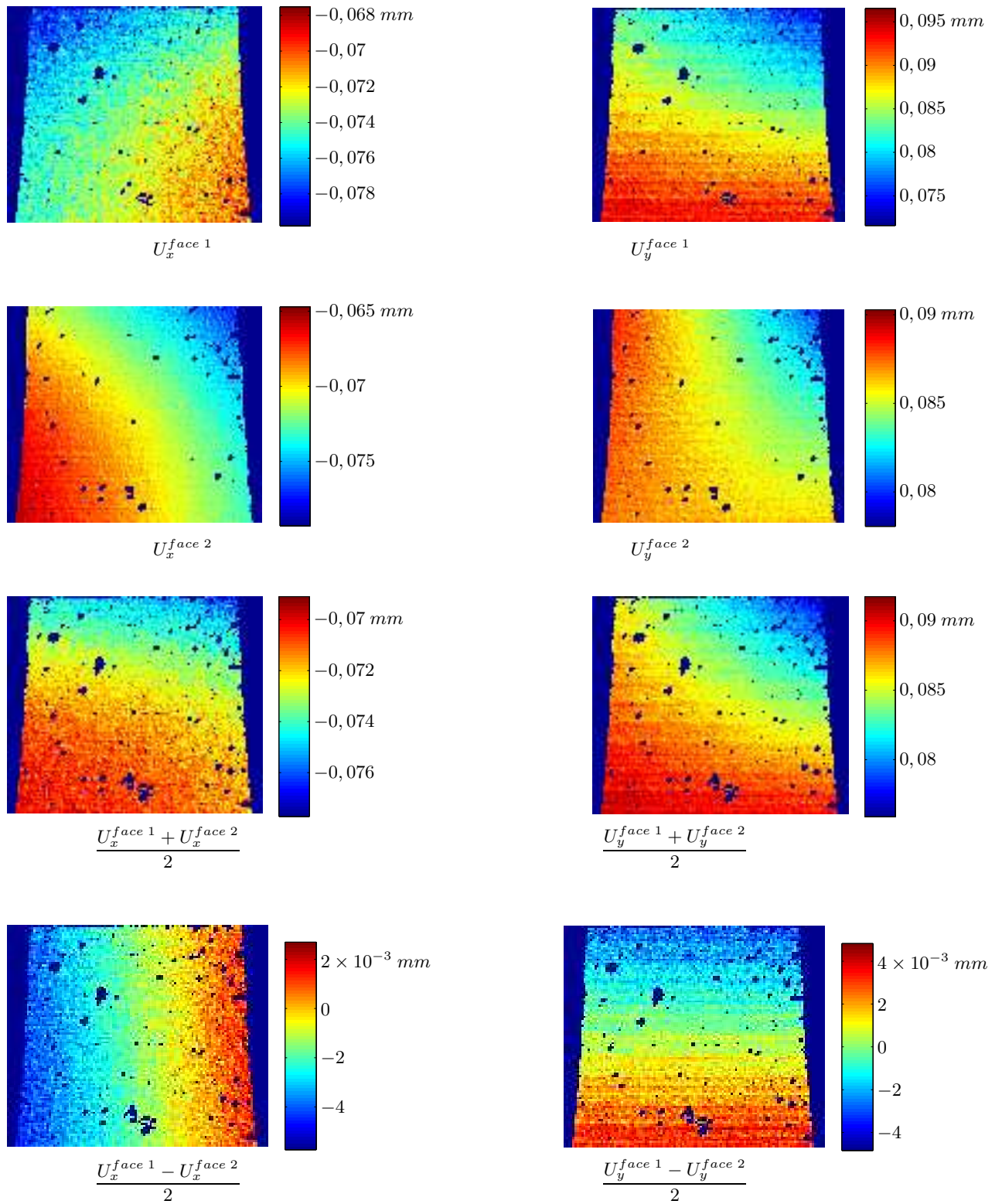
FIG. 5.12: Champs de déplacement mesurés sur les deux faces, moyennes et demi-différences avant l'apparition de la plasticité (3300 N).
