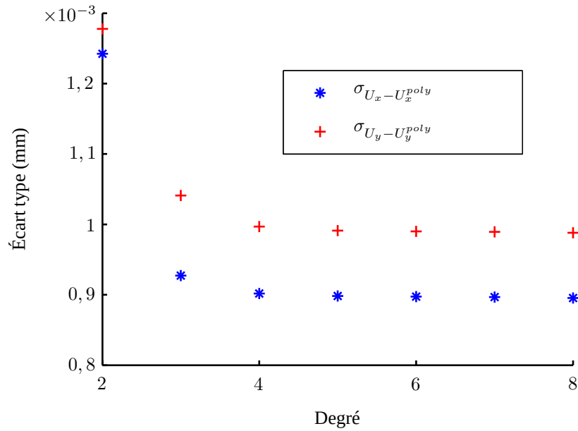
FIG. 5.20: Écarts quadratiques moyens entre le déplacement mesuré et l'approximation polynomiale en fonction du degré du polynôme.
