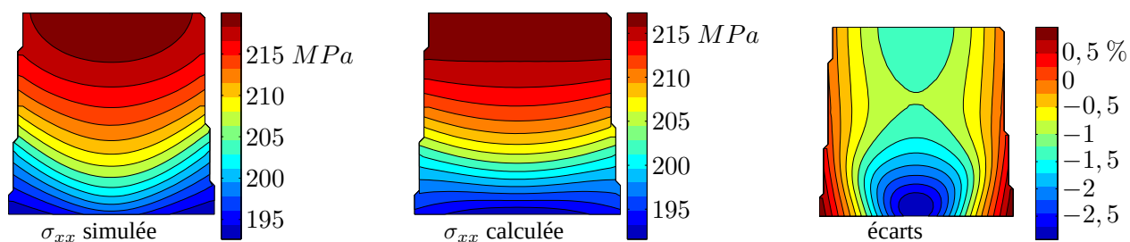
FIG. 5.5: Comparaison d'un champ de contrainte simulé avec un champ de contrainte calculé par la procédure uniaxiale ( F = 8760 \text{ N} , modèle de Voce, paramètres : tableau 2.2).
