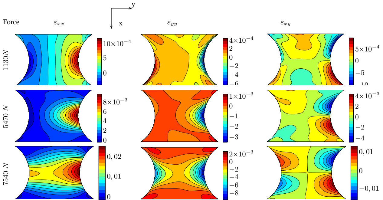
FIG. 6.16: Essai n°5 : champs de déformation obtenus après dérivation d'un polynôme de degré 10 pour trois pas de chargement.
