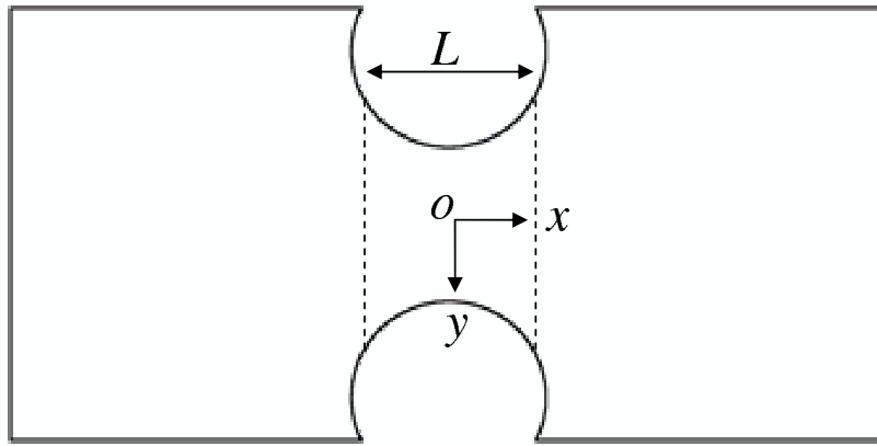
FIG. 6.23: Région d'intérêt et repère orthonormé pour l'écriture des champs virtuels
