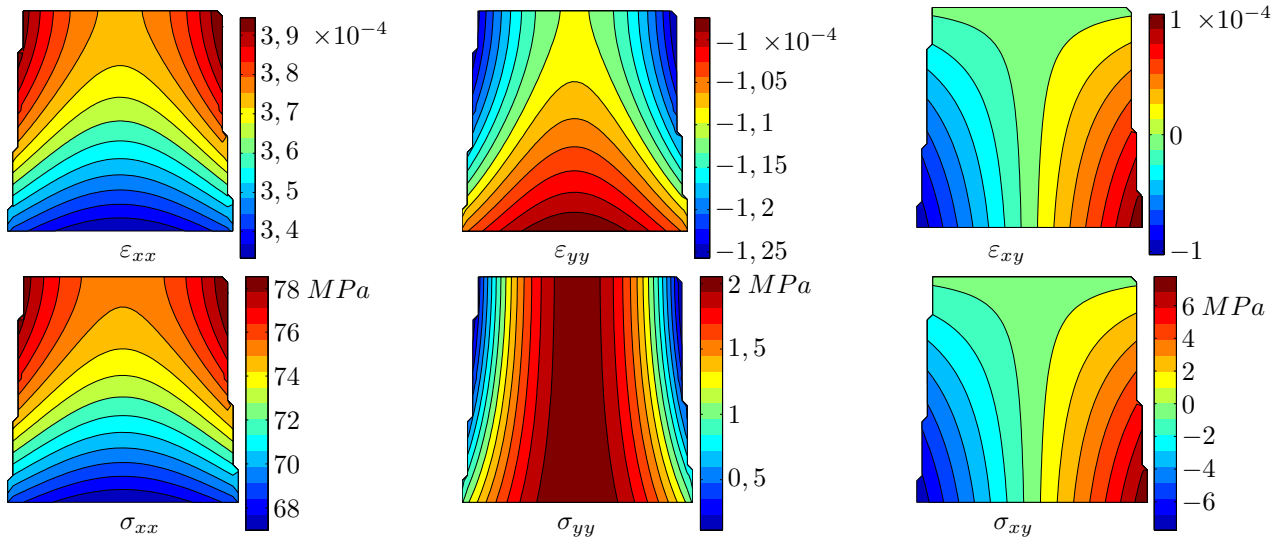
FIG. 5.3: Champs simulés de déformation et de contrainte avant l'apparition de la plasticité ( F = 3050\text{N} ), avec le modèle de Voce (tableau 2.2).
