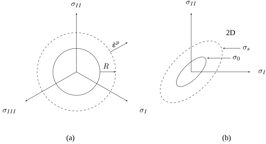
FIG. 2.2: (a) Surface de charge axée sur la trisectrice du repère ( \sigma_I = \sigma_{II} = \sigma_{III} ) dans l'espace des contraintes principales, écoulement normal \dot{\epsilon}^p et écrouissage isotrope R ; (b) projection des surfaces de charge initiale et écrouie en contraintes planes ( \sigma_{III} = 0 ).
