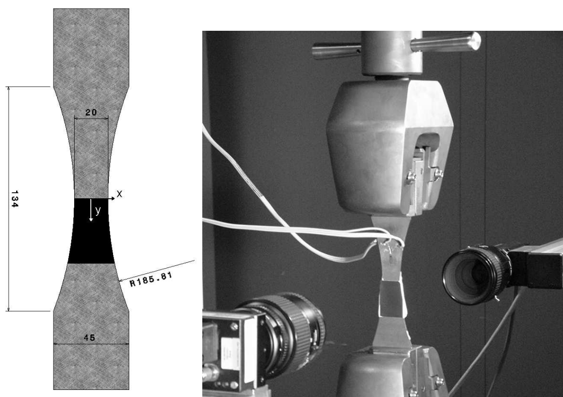
FIG. 5.11: Dispositif d'essai de traction de l'éprouvette plate à section variable.
