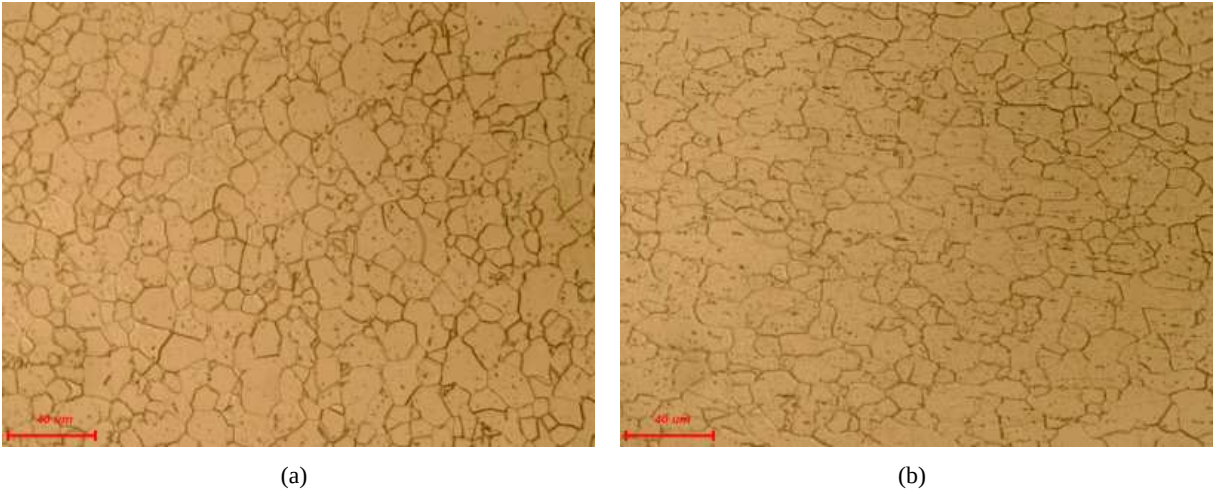
FIG. 2.1: Micro-structure d'un échantillon de la tôle. La photo (a) ne montre pas d'orientation privilégiée des grains dans le plan de la tôle, tandis que dans l'épaisseur (b), les grains sont légèrement écrasés en raison du procédé de laminage.
