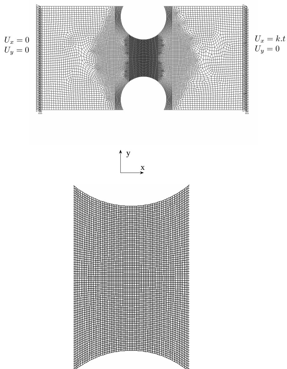
FIG. 6.4: (a) : Modèle éléments finis de l'essai de traction sur éprouvette bi-entallée (élément PLANE182). (b) : Région utilisée pour l'identification (environ 5000 éléments).
