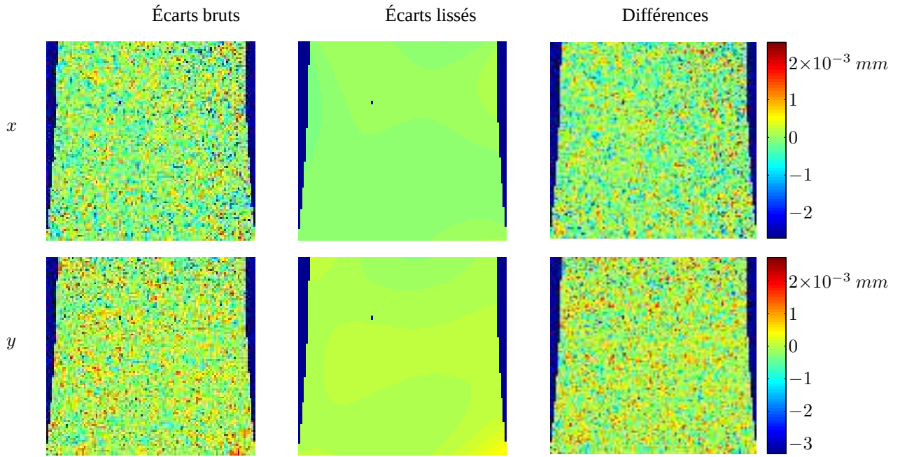
FIG. 5.13: Distributions (x, y) d'écarts entre deux mesures successives du même état cinématique, lissage polynomial de degré quatre de ces distributions et différences entre les deux.
