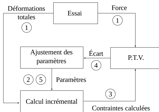
FIG. 6.7: Diagramme de déroulement de la méthode des champs virtuels dans le cas non linéaire. Les déformations peuvent être mesurées directement ou obtenues par dérivation des déplacements.
