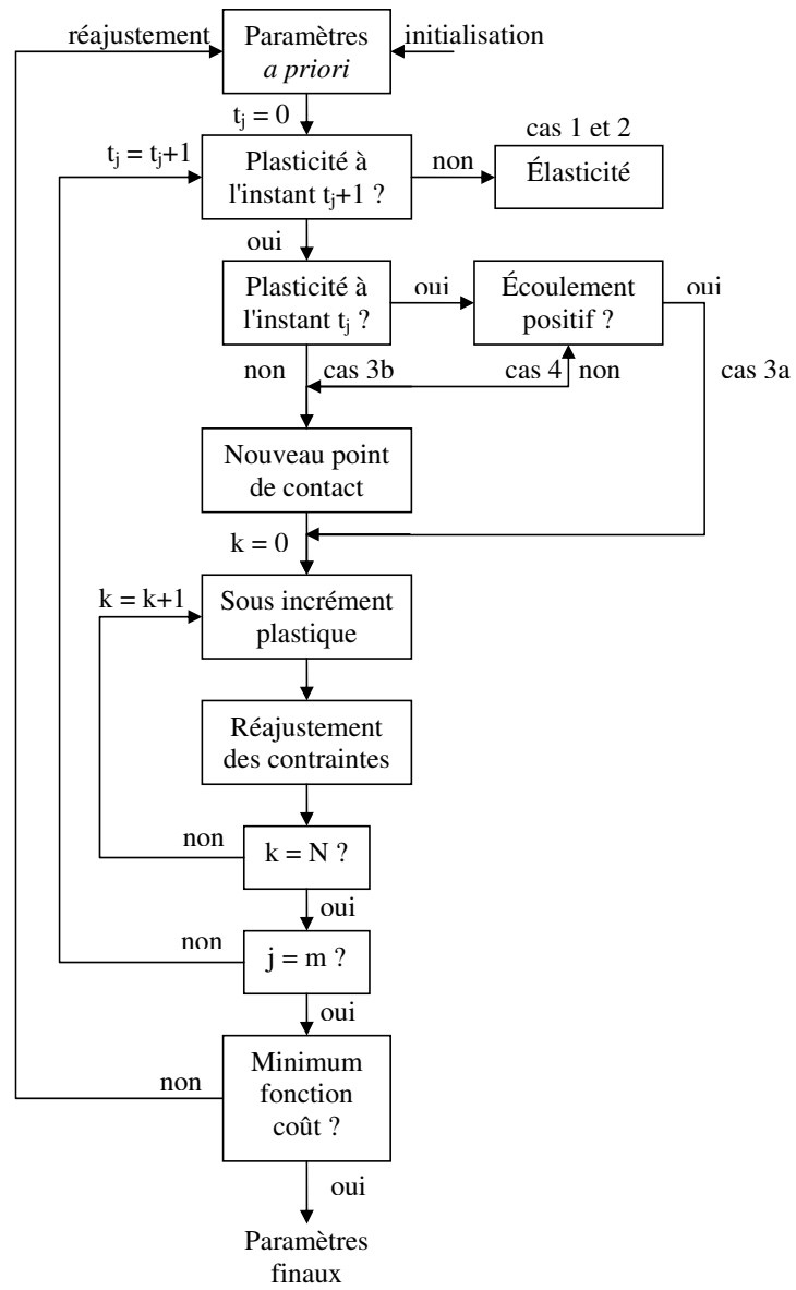
FIG. 3.5: Diagramme de la procédure de minimisation et de calcul des contraintes dans le cas 2D.
