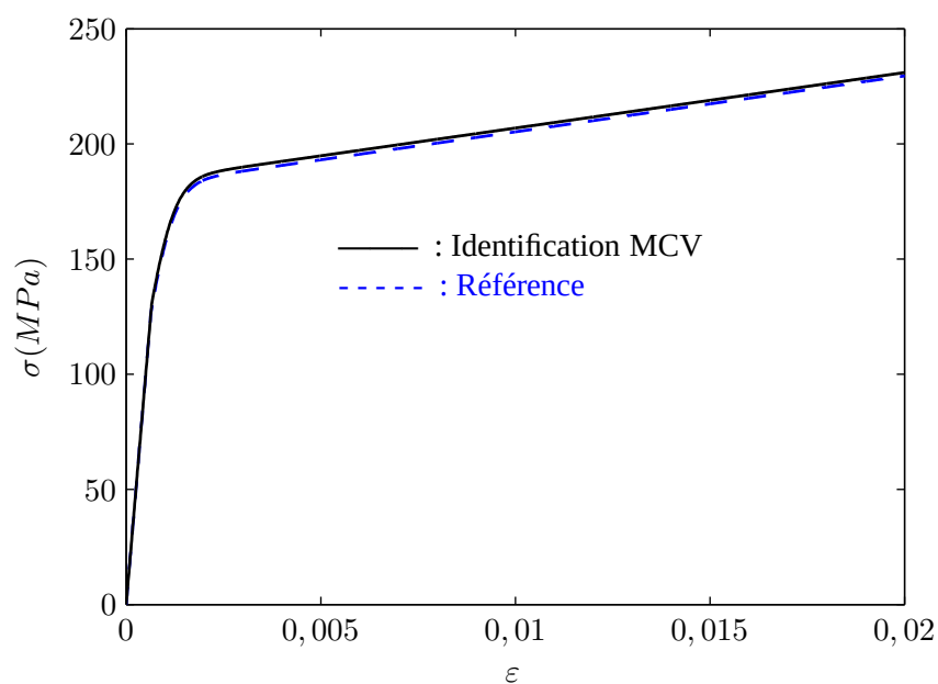
FIG. 5.8: Courbe référence et courbe identifiée avec la MCV à partir des déformations directement issues du calcul par éléments finis.
