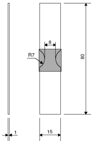
FIG. 1.8: Éprouvette de traction utilisée par Kajberg et Lindkvist (2004) pour identifier un modèle d'érouissage en grandes déformations.
