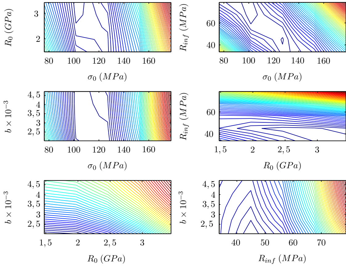
FIG. 6.24: Courbes de niveaux de la fonction coût autour des valeurs de référence pour un de essais.
