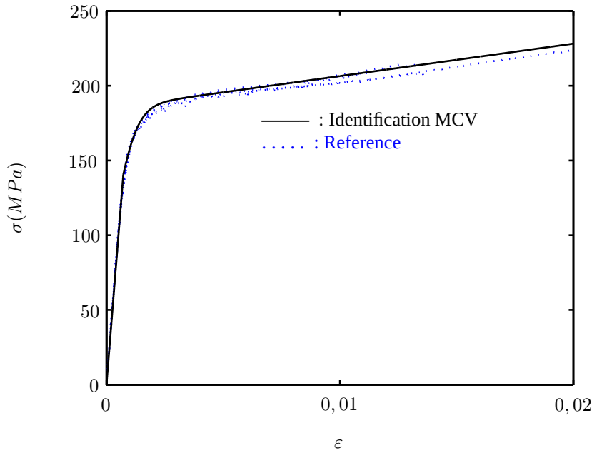
FIG. 5.17: Comparaison des courbes contrainte/déformation issues des essais de référence avec jauges et de la courbe calculée à partir des paramètres identifiés avec la MCV (voir tableau 5.8).
